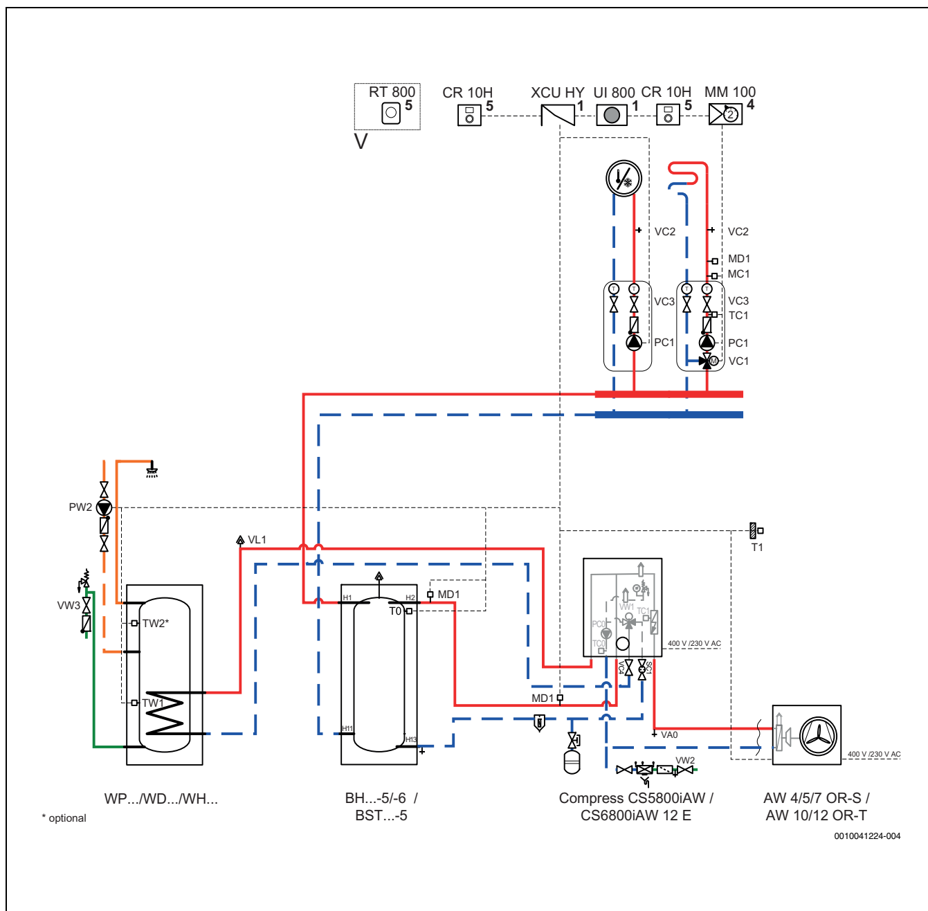
Afb. 39 Warmtepomp, twee cv-circuits, binneneenheid, buffervat en boiler
