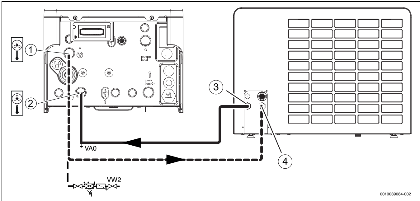
Afb. 19 Aansluiting binneneenheid op de warmtepomp
