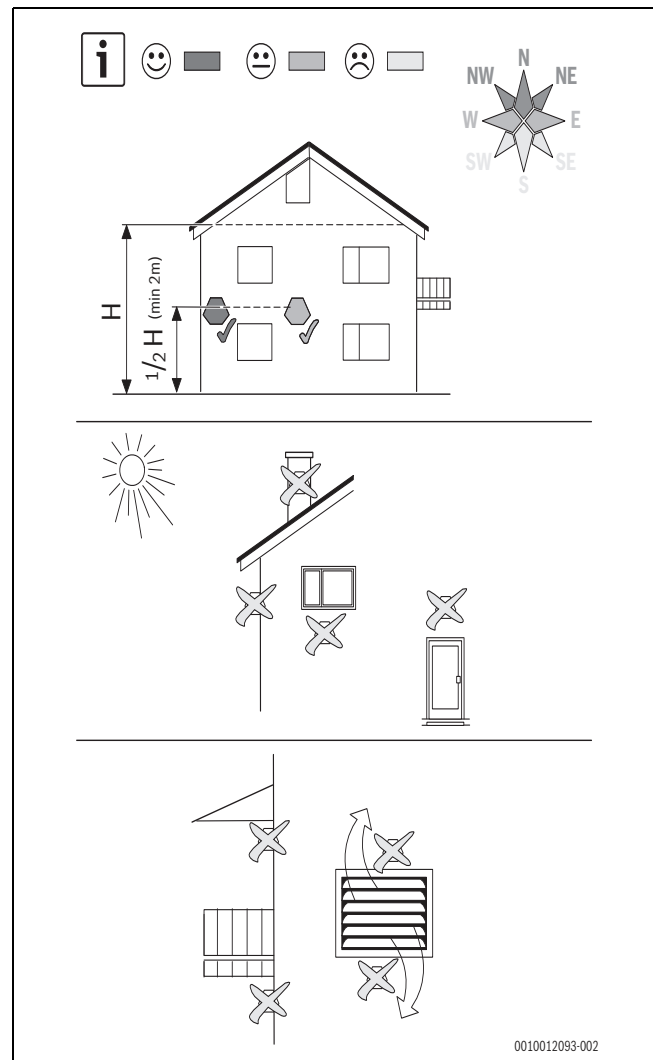
Afb. 27 Positie van de buitentemperatuursensor
