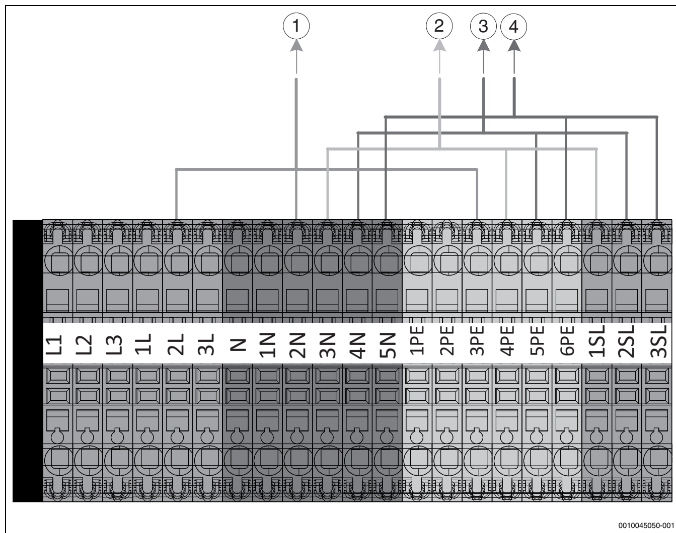
Afb. 32 Elektrische aansluitingen voor toebehoren
