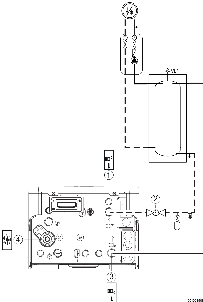
Afb. 20 Aansluiting van de binneneenheid op het verwarmingssysteem
