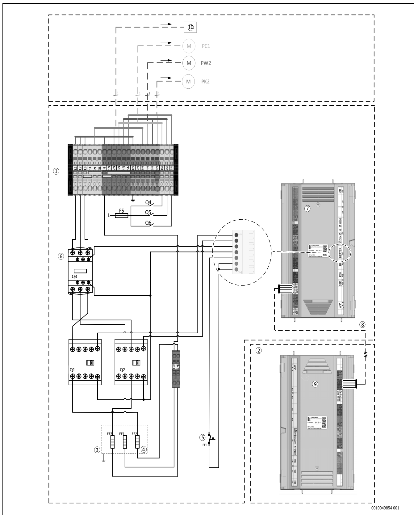
Afb. 42 Stroomvoorziening binneneenheid standaard
