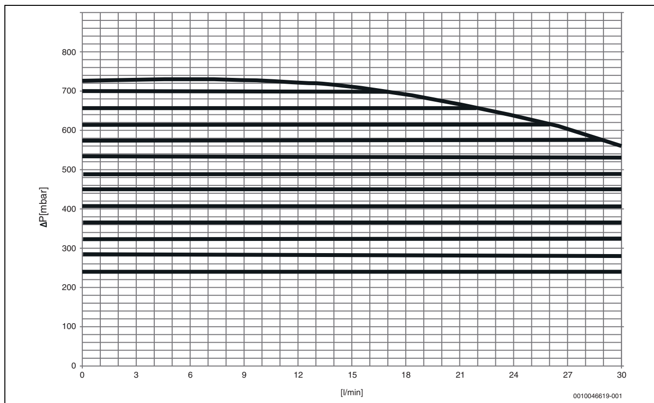
Afb. 40 Prestatieoverzicht voor PC0
