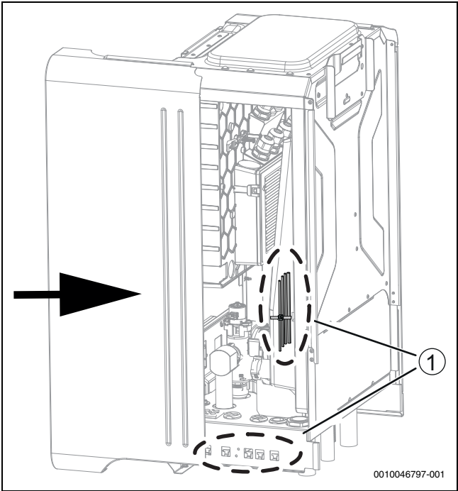
Afb. 29 Plaats de zijafdekking
