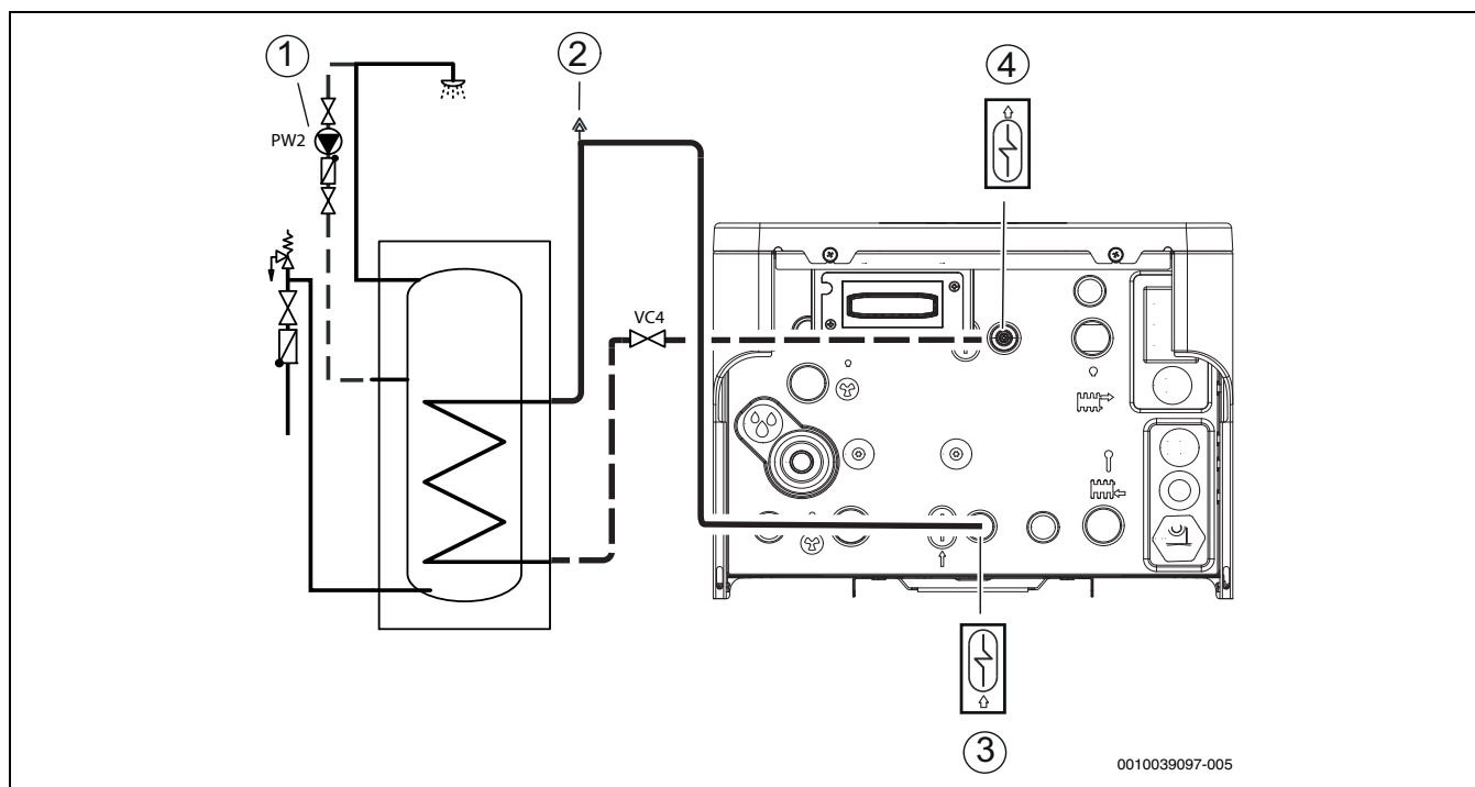
Afb. 21 Aansluitingen van de binneneenheid voor warm water
