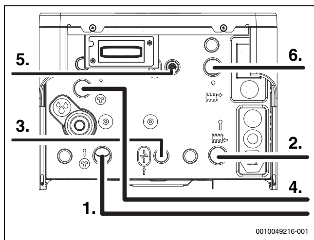
Afb. 17 Leidingaansluitingen
