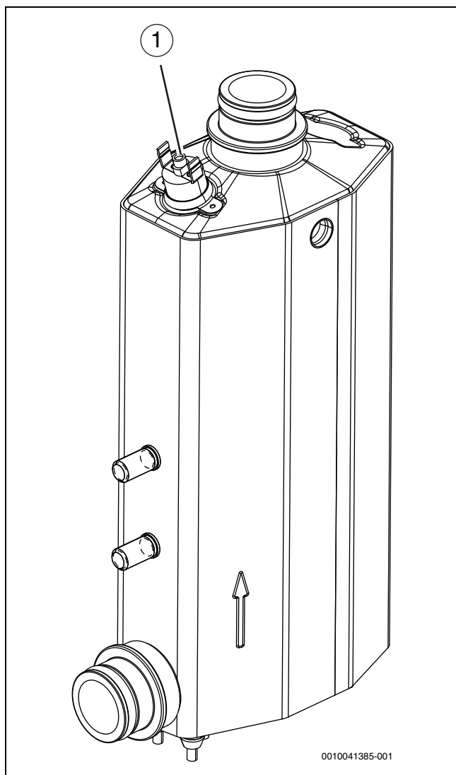
Afb. 35 Elektrische verwarming
