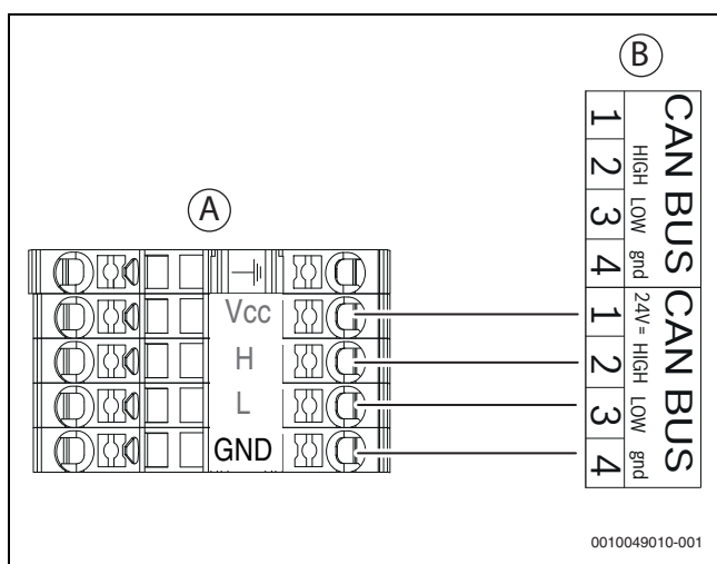
Afb. 24 CAN-BUS warmtepomp - binneneenheid
