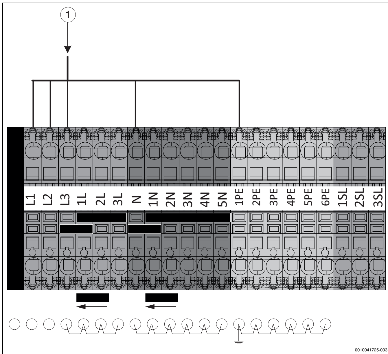
Afb. 30 Elektrische aansluitingen
