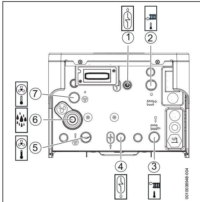
Afb. 6 Leidingaansluitingen
