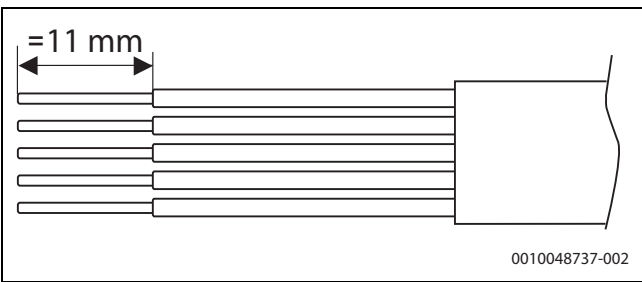
Afb. 28 Striplengte ader voedingsaansluiting
