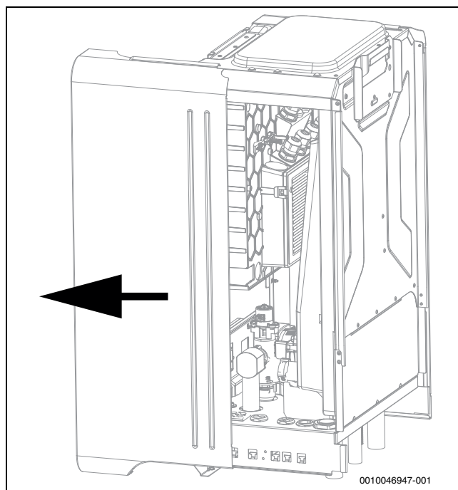
Afb. 16 Verwijder de zijafdekking
