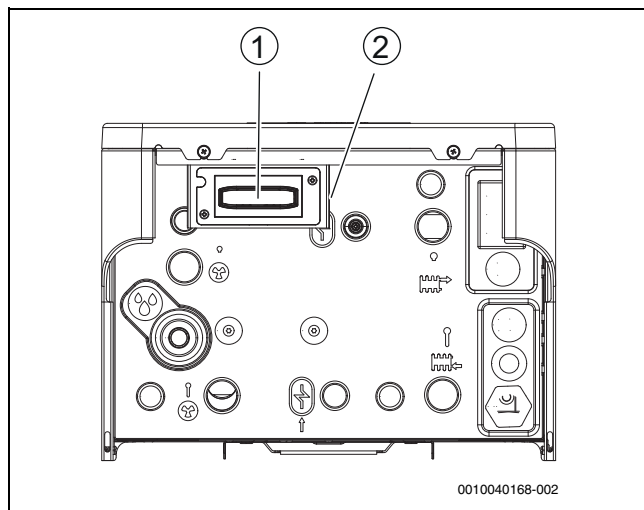
Afb. 12 Plaatsen Connect-Key
