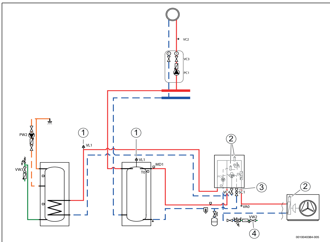
Afb. 22 Binneneenheid, warmtepomp, boiler en verwarmingssysteem met buffervat
