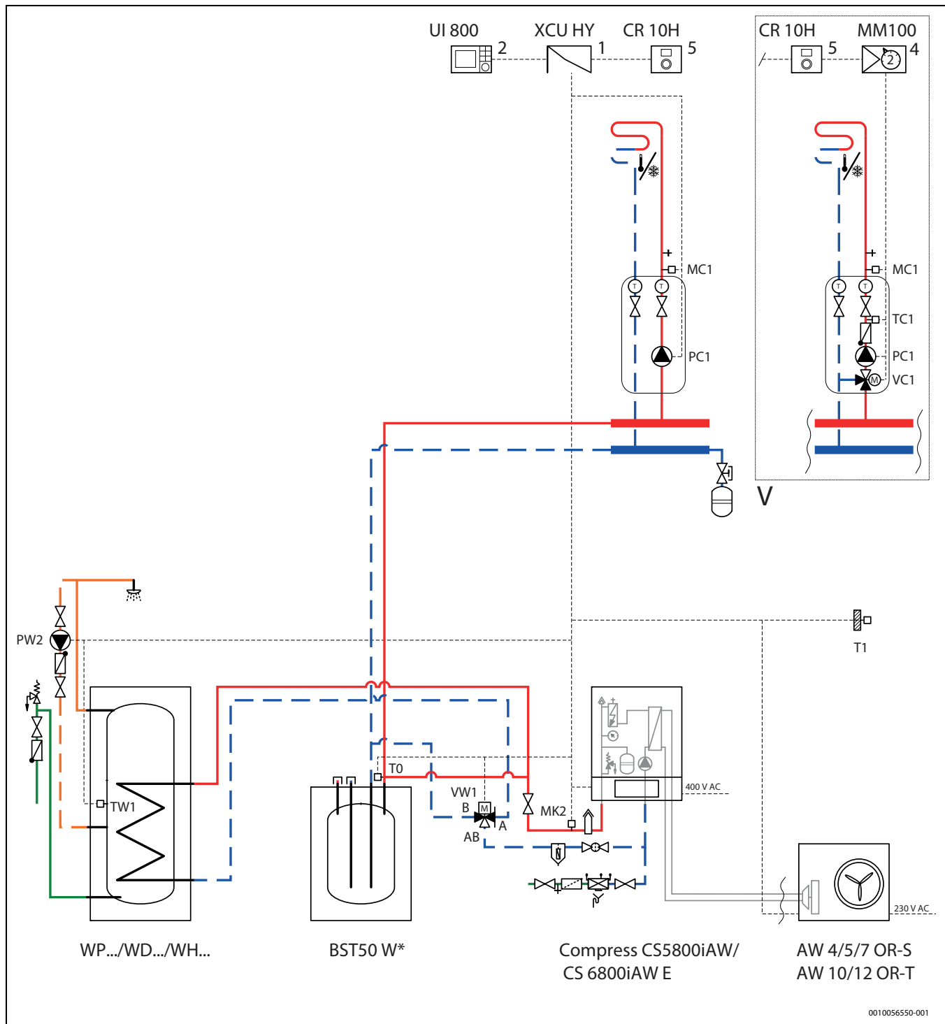
Afb. 37 Warmtepomp met binnenunit, klein buffervat en warmwatertoestel
