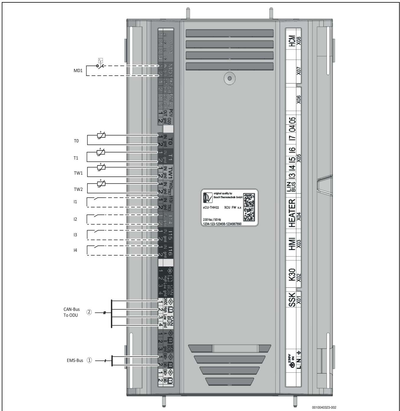
Afb. 33 Aansluitingen
