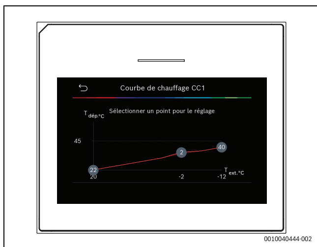
Fig. 1 Écran de démarrage pour le réglage de la courbe de chauffage pour le type de régulation de la température extérieure avec pied de courbe (et point de confort)
