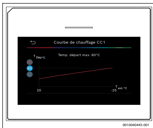
Fig. 5 Régler la température maximale de départ
