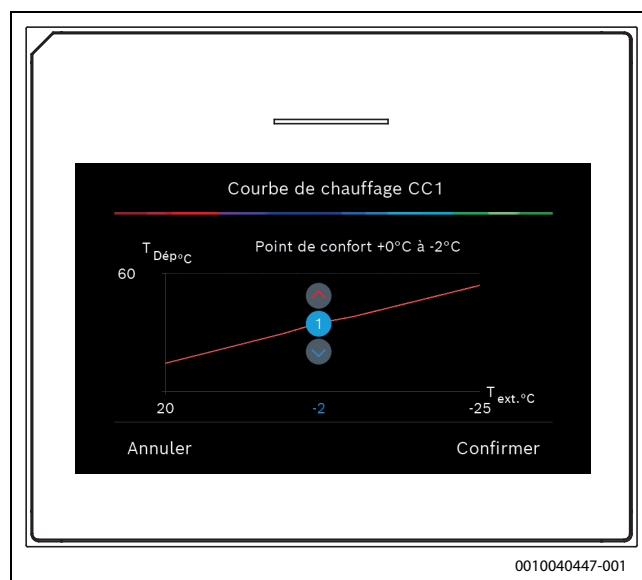
Fig. 4 Régler le point de confort (uniquement si le type de réglage est défini sur la température extérieure avec pied de courbe)
