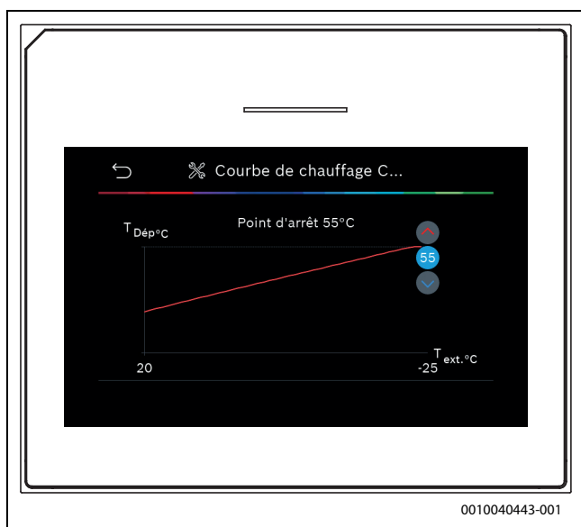
Fig. 2 Régler le point d'arrêt (uniquement si le type de réglage est défini sur la température extérieure avec pied de courbe)
