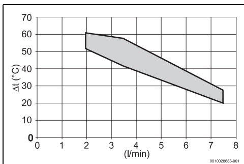
Afb. 30 Type 9 liter
