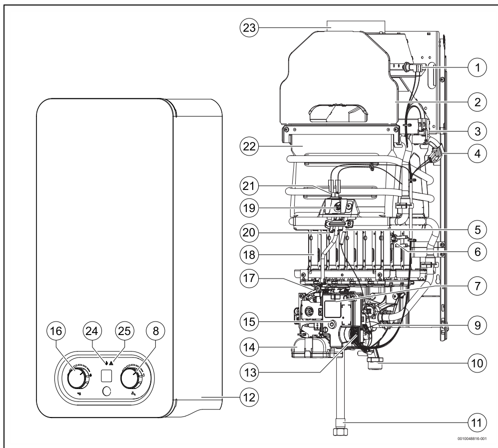
Afb. 2 Toestelontwerp
