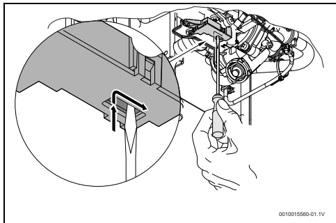
Afb. 27 Reset de microschakelaar
