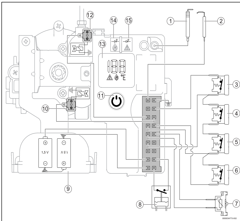
Afb. 29 Elektrisch schema
