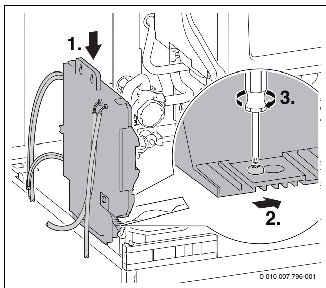
Afb. 56 Besturing op de boiler bevestigen
