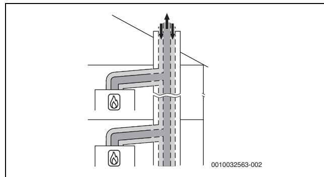
Afb. 32 Collectief systeemconform C (10)3x met concentrisch luchttoevoer/rookgasafvoersysteem in opstellingsruimte
