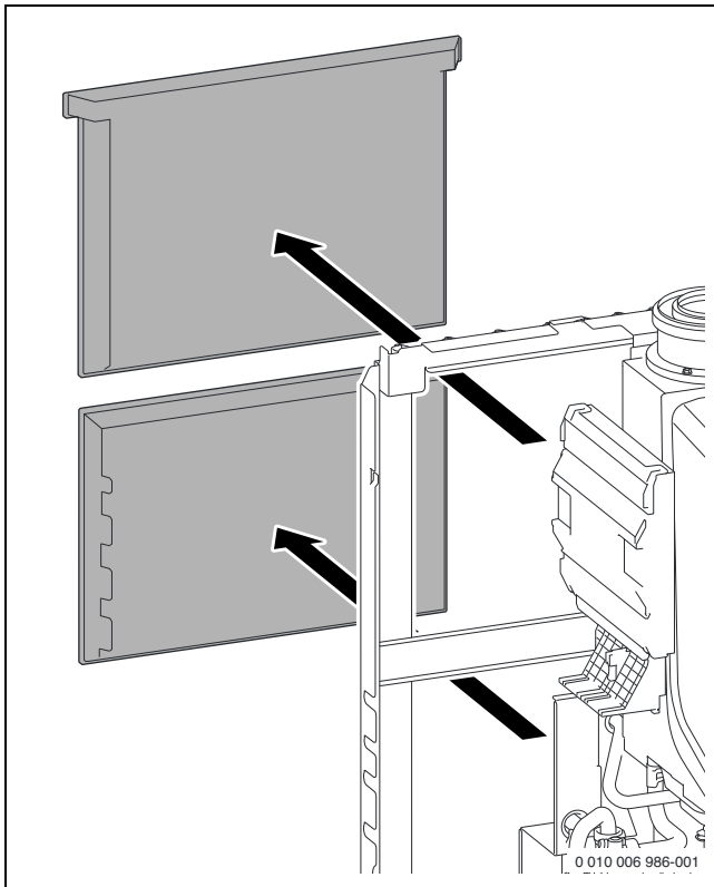
Afb. 64 Warmte-isolatie aan de achterzijde afnemen
