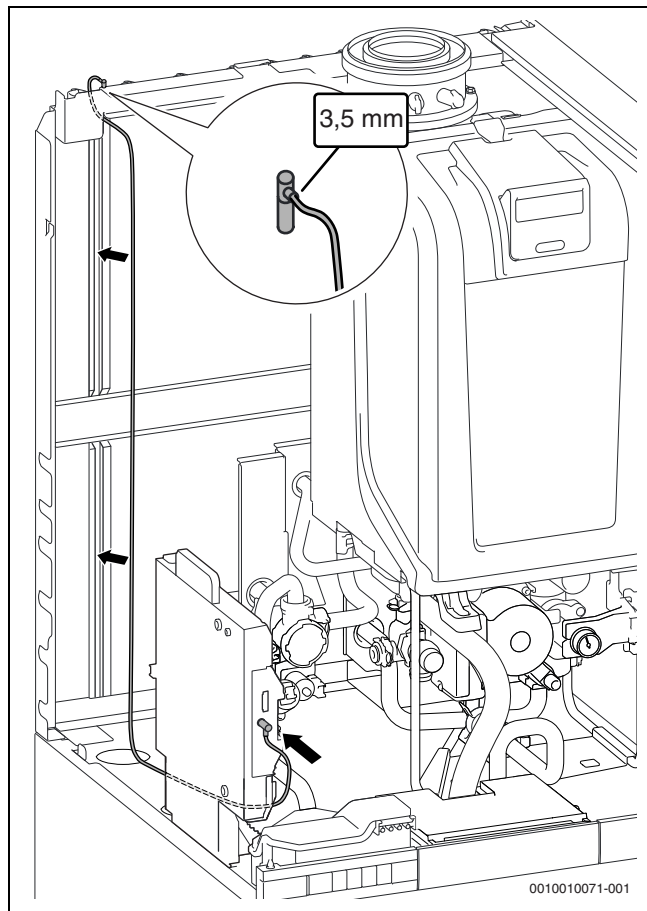
Afb. 70 Aansluiting en installatie van de kabel
