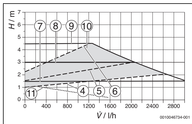
Afb. 113 Pompkarakteristiek voor proportionele druk en constante druk
