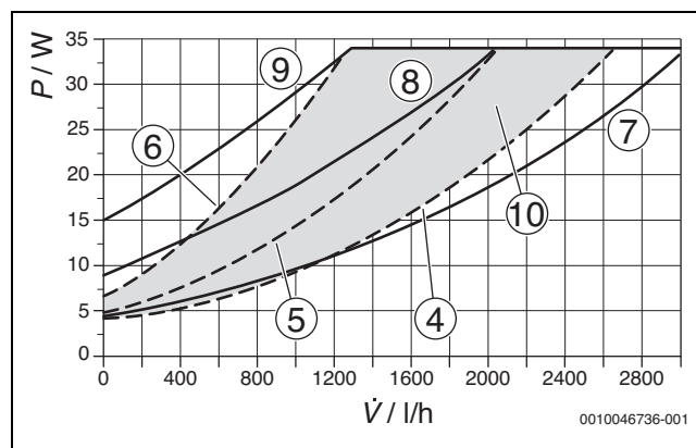
Afb. 115 Opgenomen vermogen voor proportionele druk en constante druk
