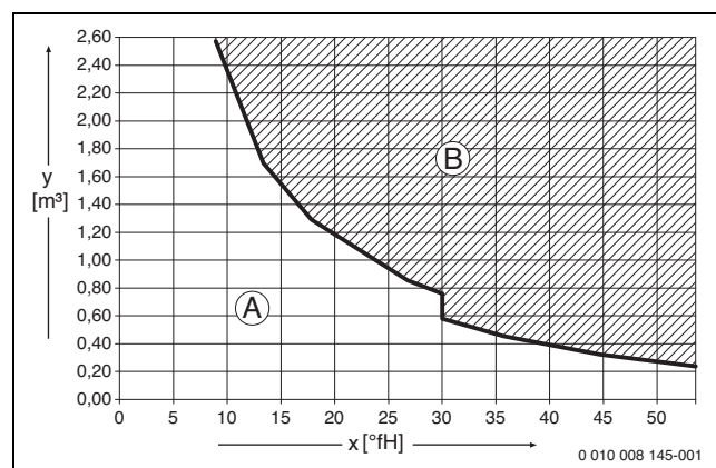
Afb. 40 Eisen aan het vul- en bijvulwater in °fH voor toestellen < 50 kW
