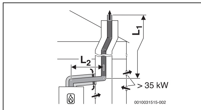
Afb. 31 Flexibel rookgasafvoer door de schacht B 33 met open luchttoevoer via het concentrisch luchttoevoer/rookgasafvoersysteem in opstellingsruimte
