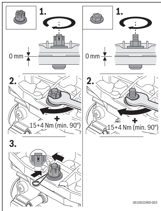
Afb. 89 Draai de moer op het branderdekseel vast
