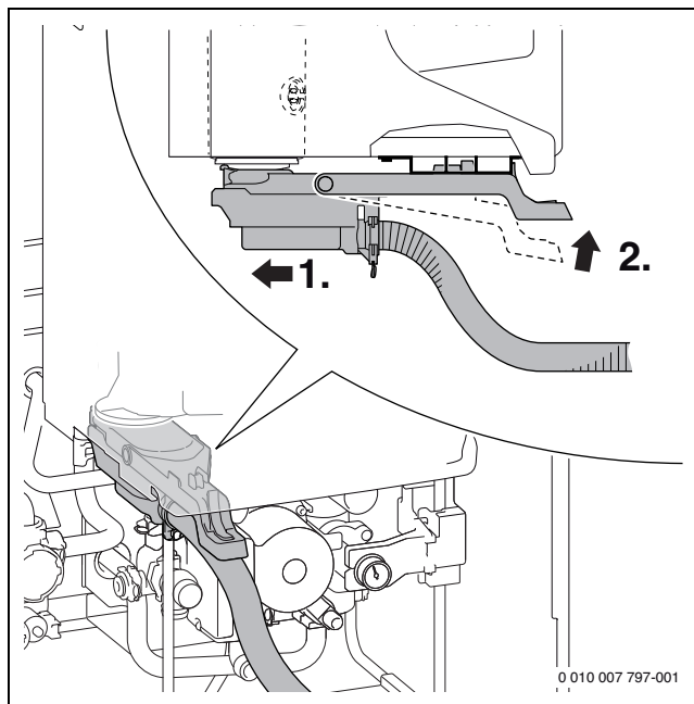
Afb. 50 Vuilfilter monteren
