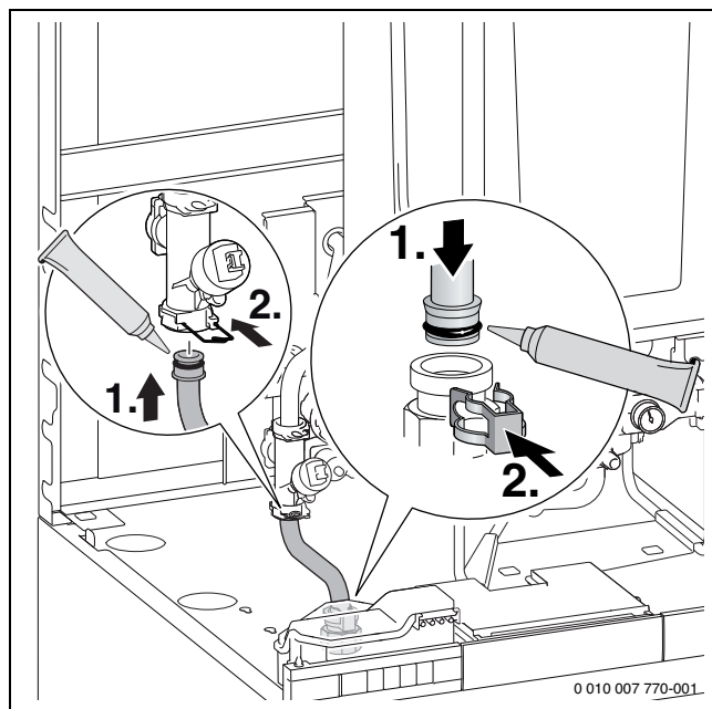
Afb. 53 Buisverbinding tussen 3-wegklep en boileraanvoer maken
