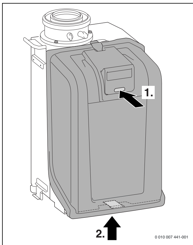
Afb. 81 Branderkap verwijderen
