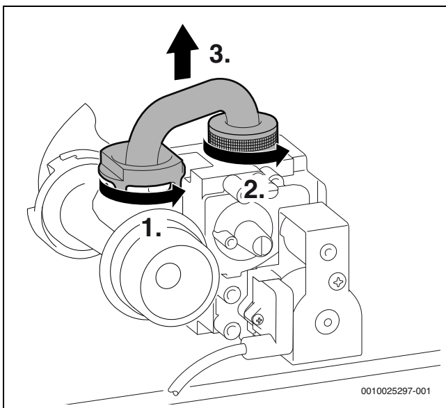
Afb. 100 Gasleiding demonteren
