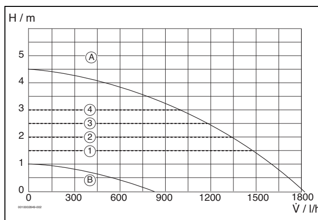
Afb. 106 Pompkarakteristieken en pompcurven
