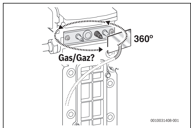
Afb. 86 Controleren op lekken
