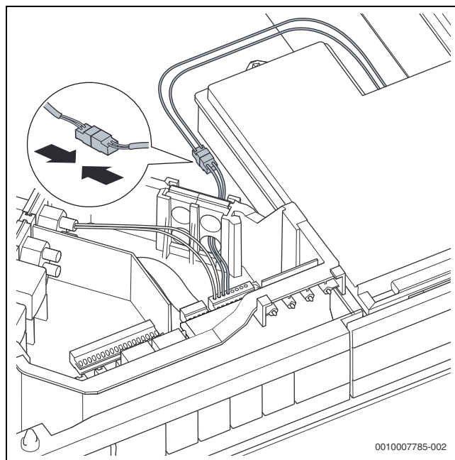
Afb. 62 Schuiflade voor de regelaar op de aansluitbox aansluiten
