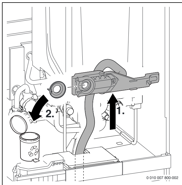
Afb. 49 Vuilfilter uit de onderhoudspositie nemen en beschermdeksel afnemen
