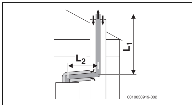
Afb. 26 Star rookgasafvoertraject conform C 93x in een schacht en concentrisch luchttoevoer/rookgasafvoersysteem in opstellingsruimte
