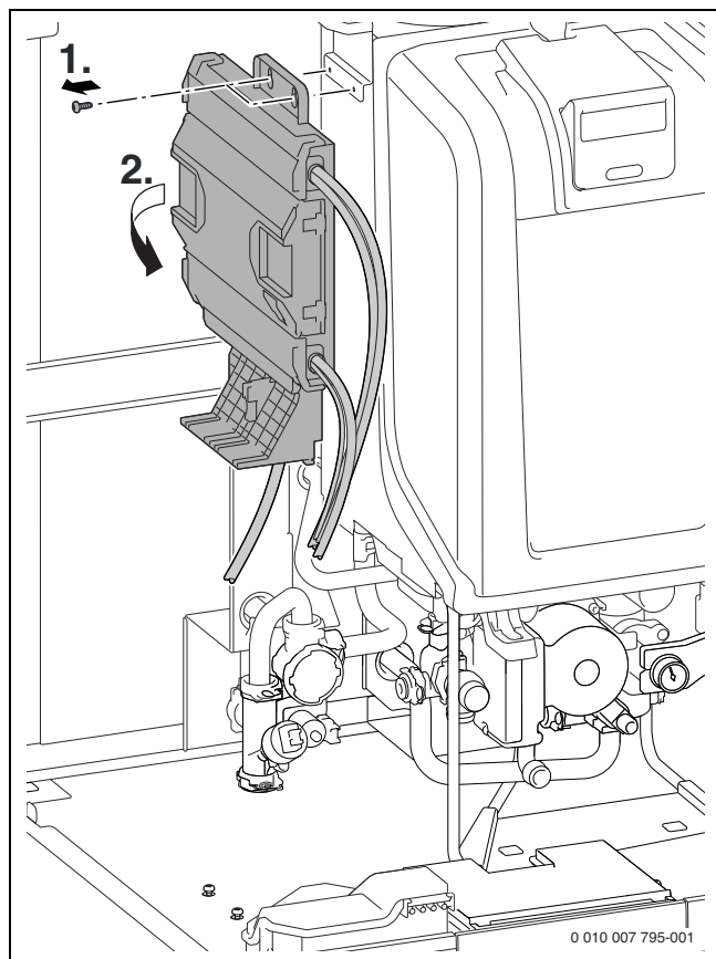
Afb. 55 Besturing afnemen
