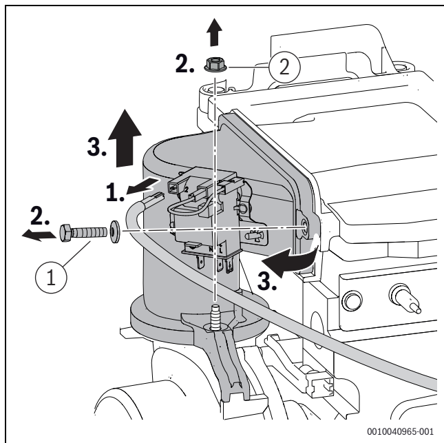
Afb. 97 Menginrichting demonteren
