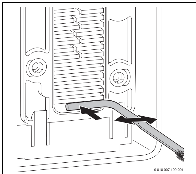
Afb. 94 Condensopvang reinigen
