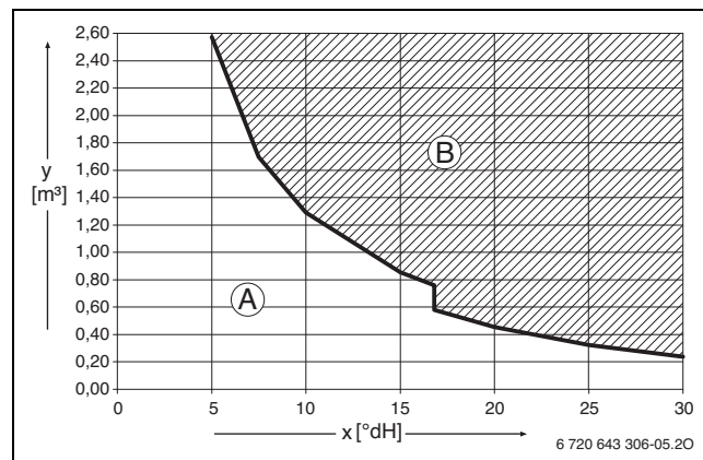
Afb. 39 Eisen aan het vul- en bijvulwater in °dH voor toestellen < 50 kW
