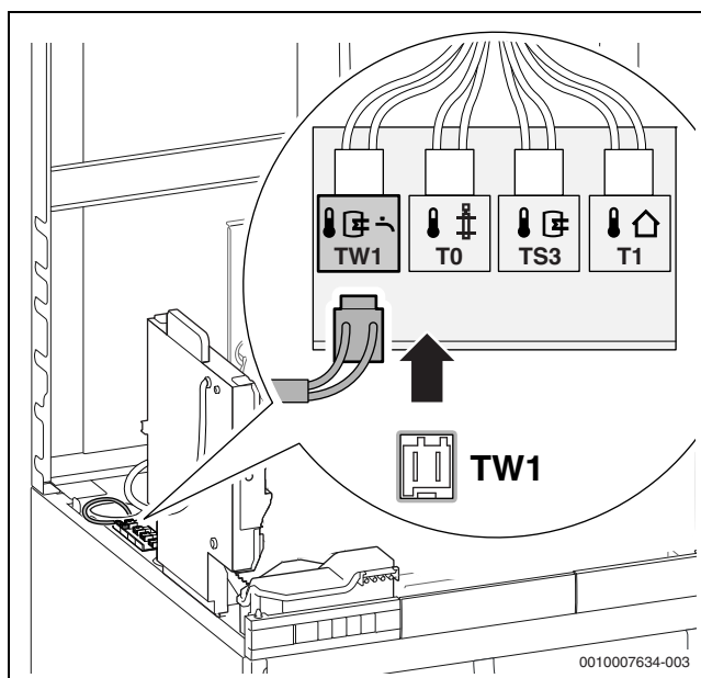
Afb. 58 Boilertemperatuursensor aansluiten
