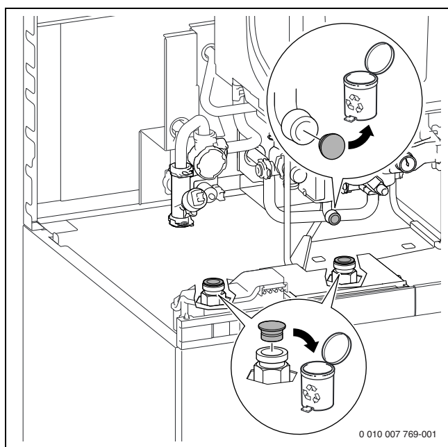
Afb. 52 Stop op verwarmingslichaam en op de boileraanvoer en -retour verwijderen
