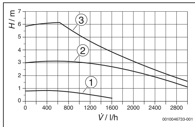
Afb. 112 Pompcurve voor de pompstanden I tot III
