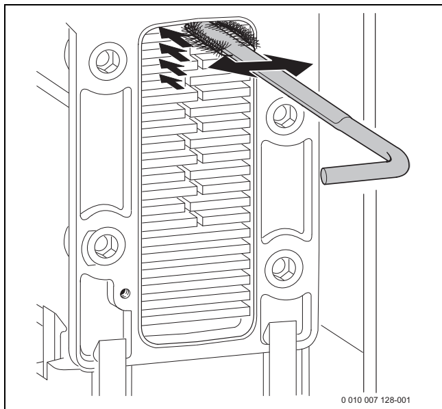
Afb. 92 Reinig het verwarmingslichaam met de borstel
