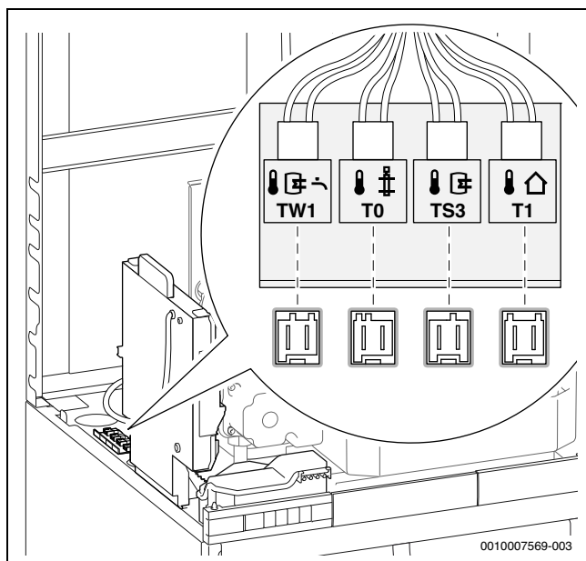
Afb. 69 Stekker op besturing
