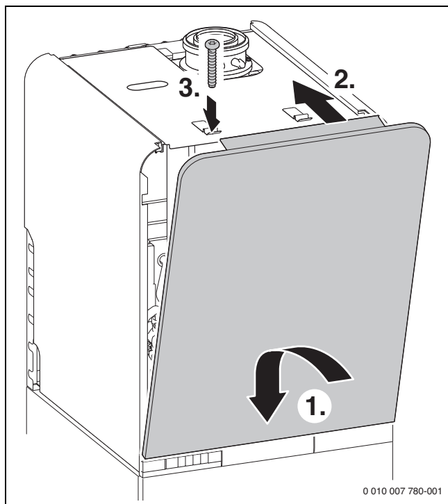
Afb. 75 Voorste mantel inhangen en met de schroef uit de leveringsomvang borgen
