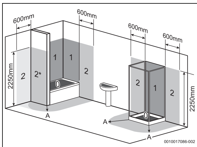
Afb. 38 Veiligheidszone (voorbeeldweergave)
