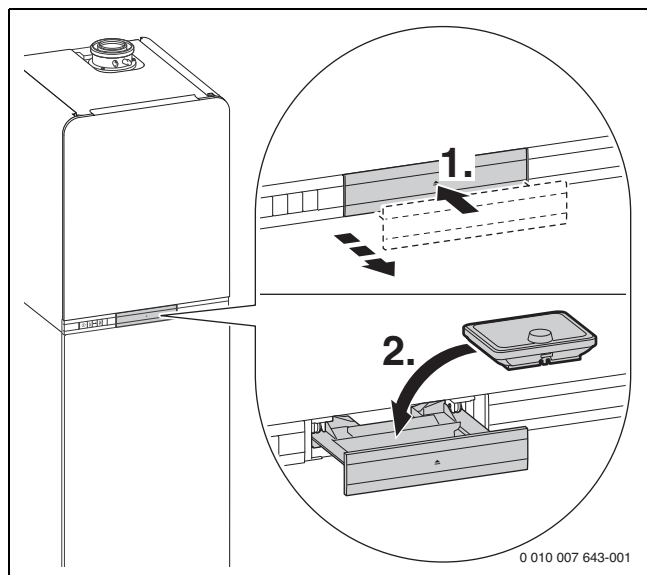
Afb. 71 Plaats de verwarmingsregelaar
