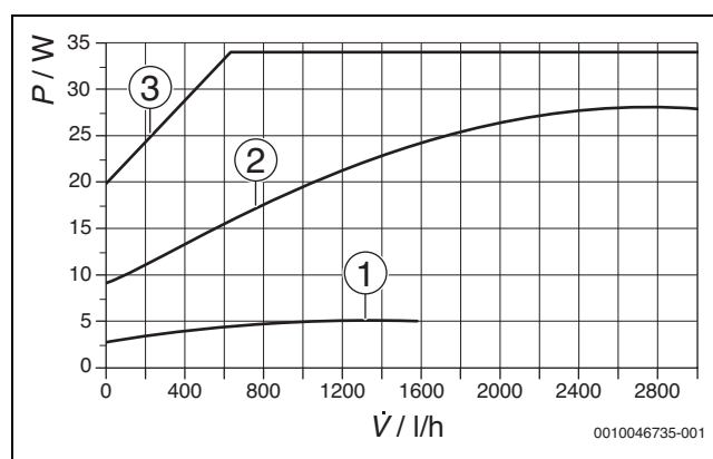
Afb. 114 Opgenomen vermogen voor de pompstanden I tot III
