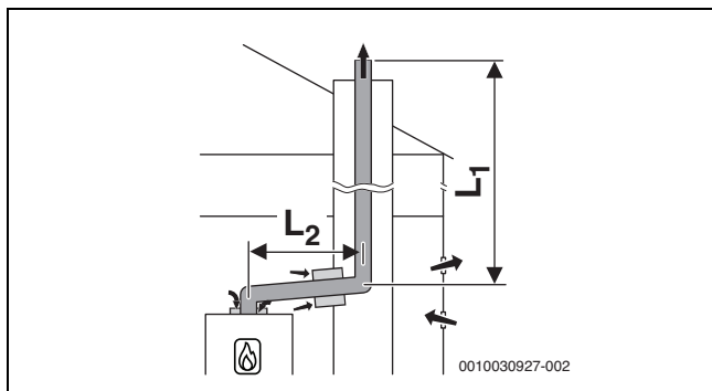
Afb. 28 Starre rookgasafvoer door de schacht conform B 23p /B 53p met open luchttoevoer aan toestel en concentrisch verbindingstuk tussen opstellingsruimte en schacht
