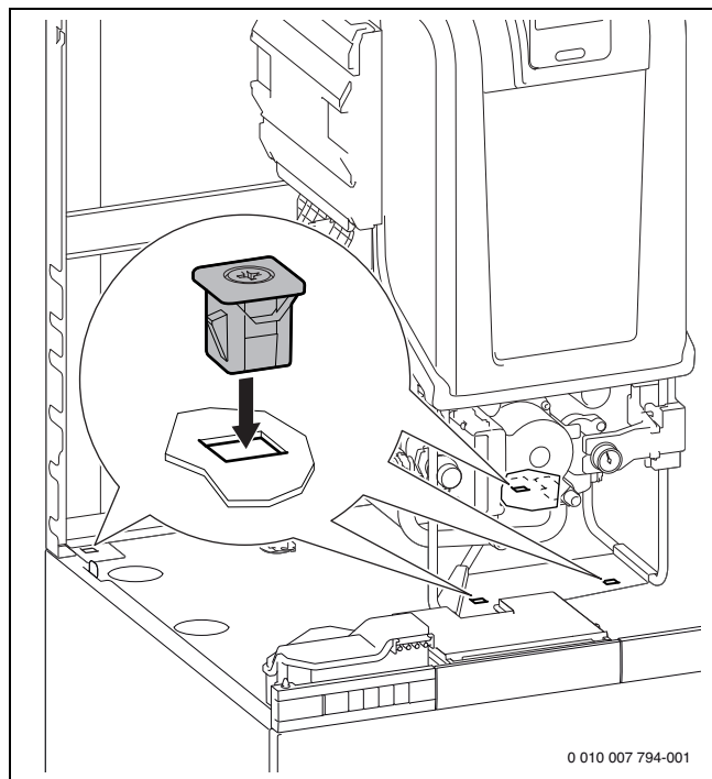
Afb. 48 Ketel met de 4 meegeleverde clips op de boiler fixeren
