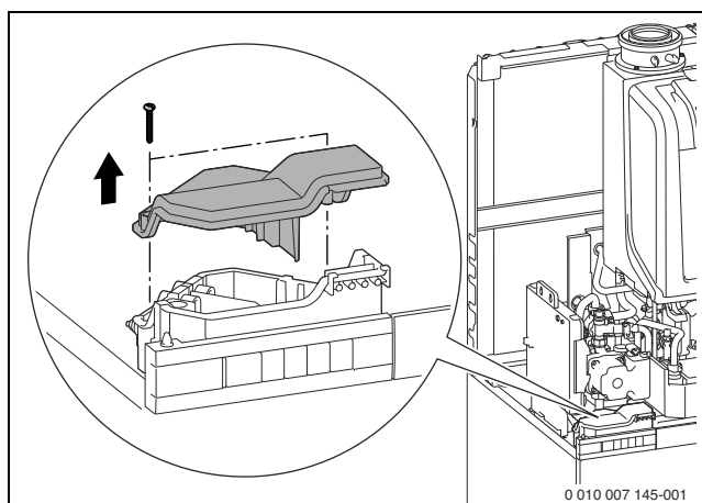
Afb. 59 Afdekking van de aansluitbox verwijderen
