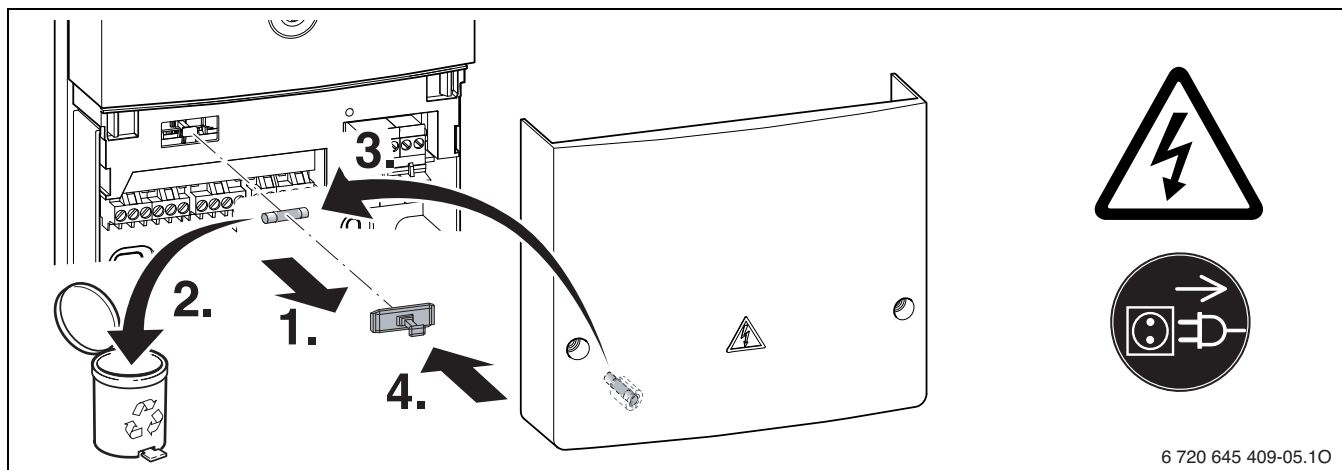
Afb. 105 Zekering van module vervangen
