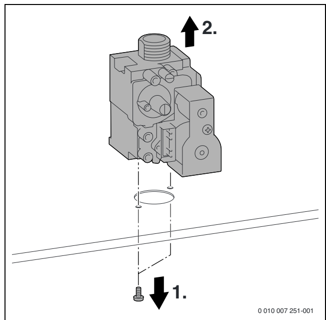
Afb. 102 Demoneren gasblok
