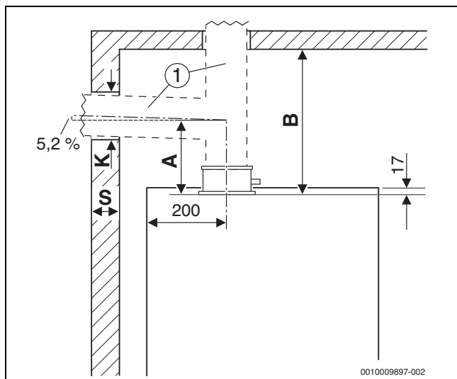
Afb. 15 Afmetingen
