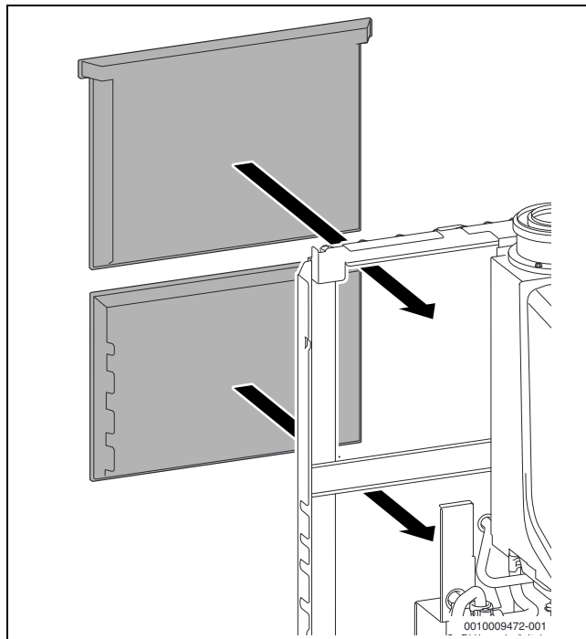
Afb. 72 Warmte-isolatie aan de achterzijde monteren
