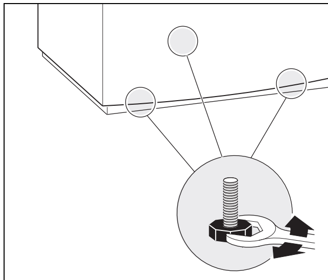
Afb. 46 Boiler uitlijnen
