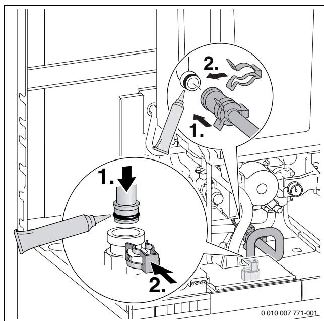
Afb. 54 Buisverbinding tussen boilerretour en verwarmingslichaam maken
