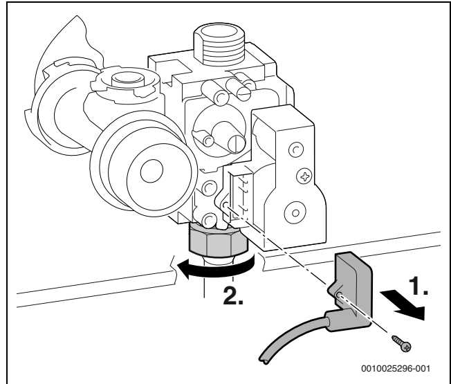
Afb. 101 Trek de stekker los en maak de wartelmoer los
