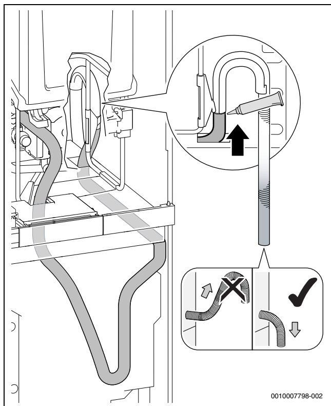
Afb. 51 Sifonslang op eindstuk steken
