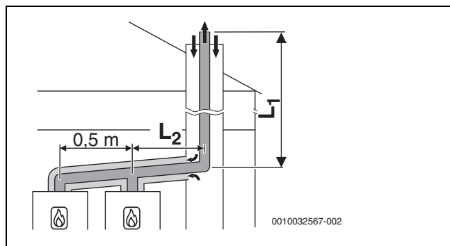
Afb. 37 Cascade met 2 toestellen: star rookgasafvoertraject conform C 93x in een schacht en concentrisch luchttoevoer/rookgasafvoersysteem in opstellingsruimte
