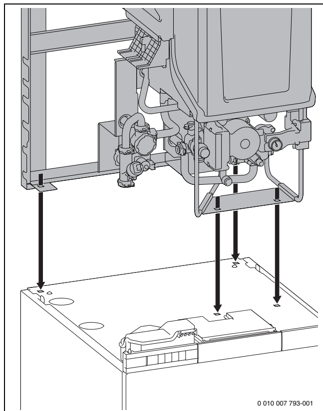
Afb. 47 Ketel op de boiler plaatsen
