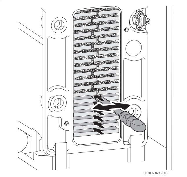
Afb. 91 Reinigingsgereedschap
