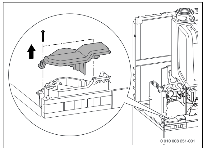
Afb. 65 Afdekking van de aansluitbox verwijderen
