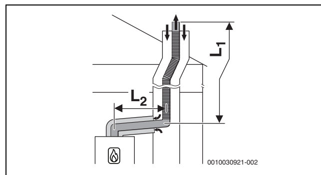
Afb. 27 Flexibel rookgasafvoertraject conform C 93x in een schacht en concentrisch luchttoevoer/rookgasafvoersysteem in opstellingsruimte
