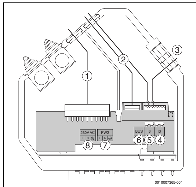
Afb. 67 Aansluitbox
