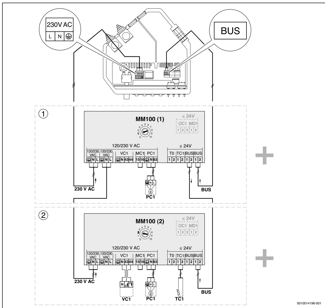
Afb. 68 Aansluiting van de module MM 100, indien aanwezig
