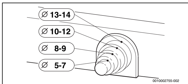
Afb. 66 Aanpassen trekontlasting aan de kabeldiameter
