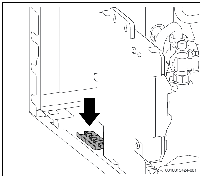
Afb. 57 Stekkerstrook op de boiler bevestigen
