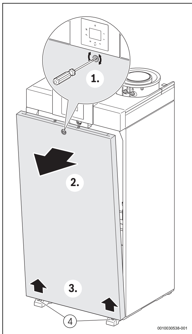
Afb. 6 Openen voorpaneel
