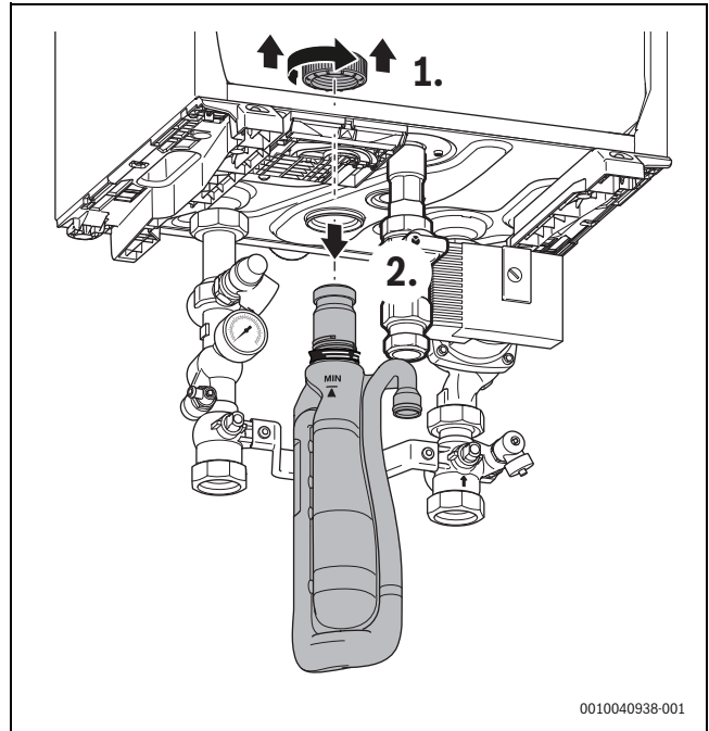
Afb. 45 Verwijderen toestelsifon
