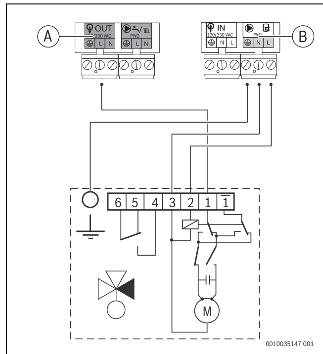
Afb. 29 Aansluitschema voor 230 V 3-wegklep
