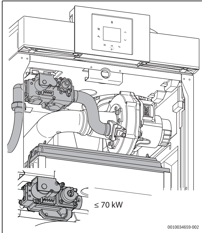
Afb. 36 Controleren gastraject
