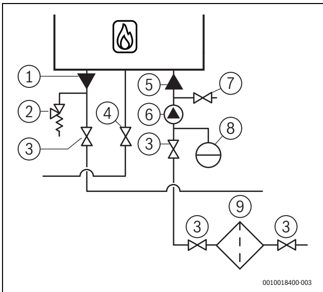
Afb. 18 Aansluiten cv-leidingen
