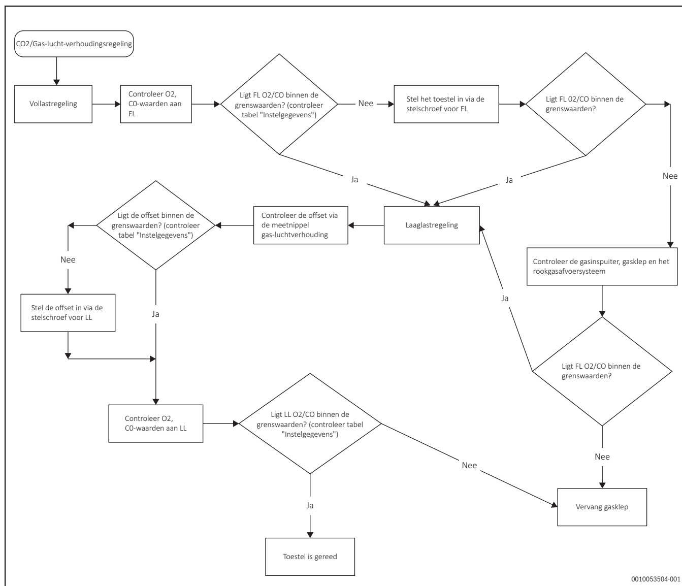
Afb. 35 Flowchart instelinstructies
