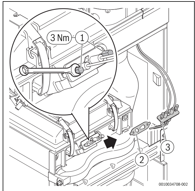
Afb. 48 Vervangen ontstekingsunit
