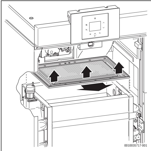
Afb. 43 Verwijderen brander
