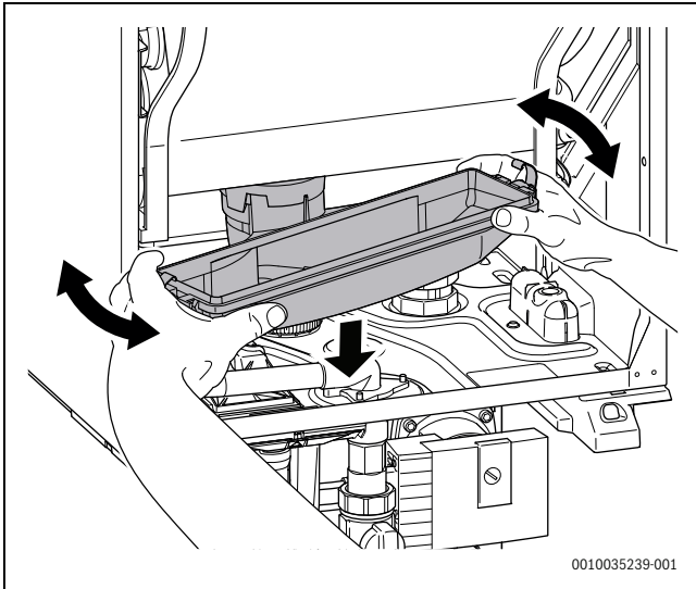
Afb. 47 Verwijderen condensbak
