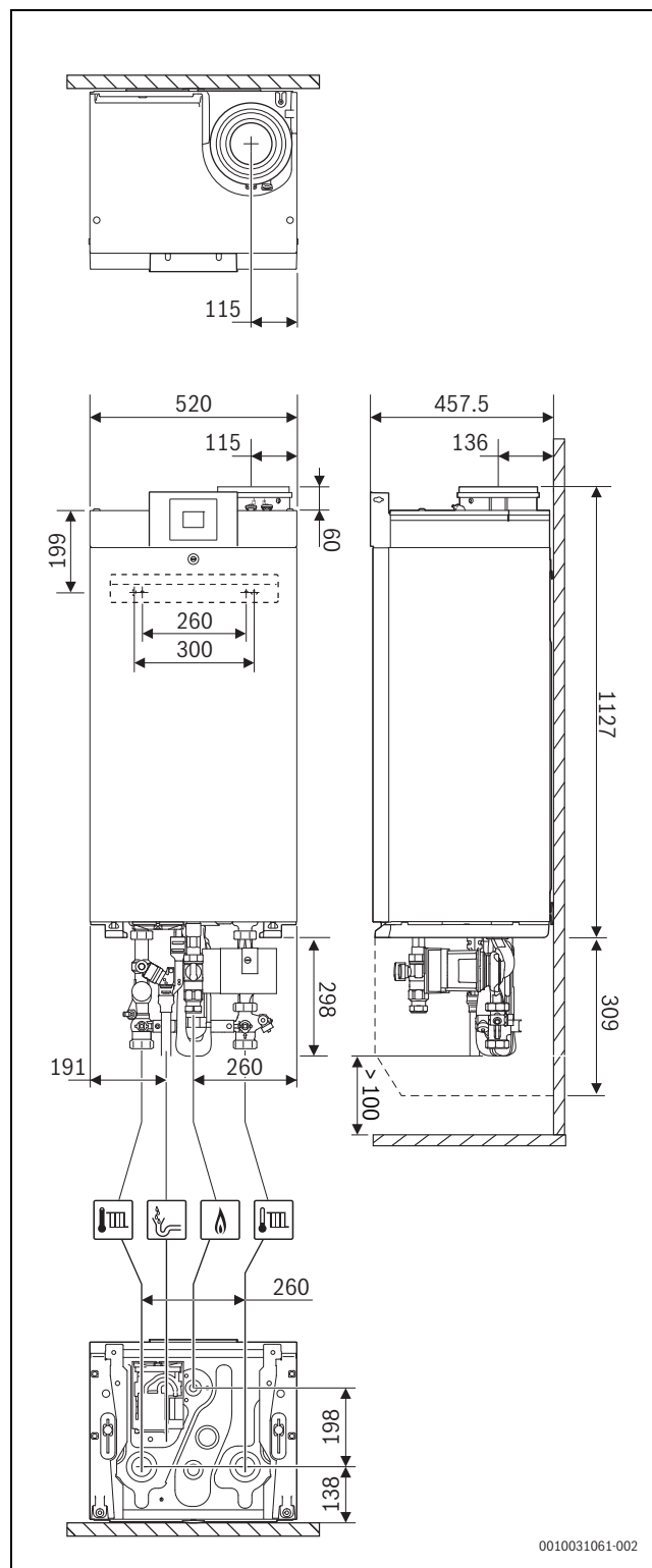
Afb. 3 Afmetingen aan de wand [mm]
