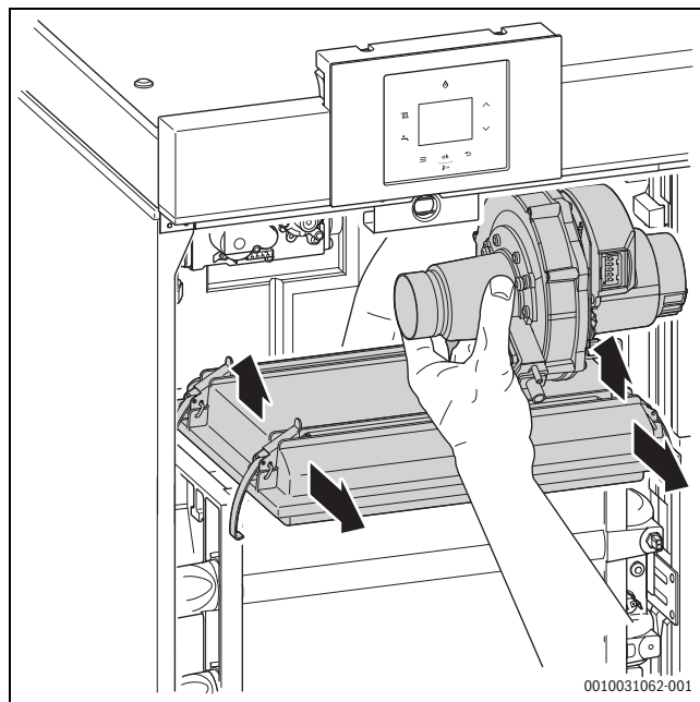
Afb. 41 Verwijderen gas-luchtunit met branderdekseel
