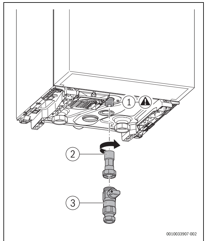
Afb. 13 De gasklep installeren
