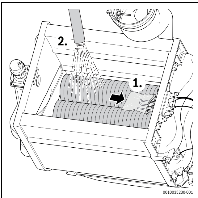
Afb. 44 Reinigen warmtewisselaar
