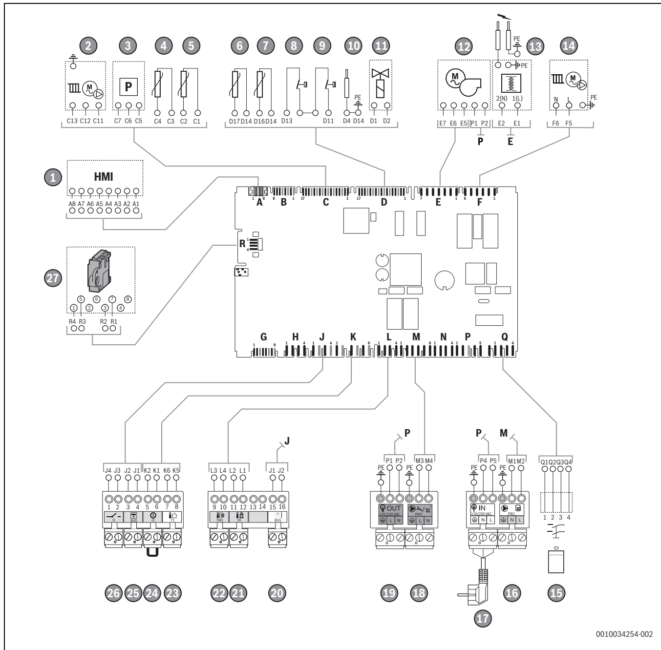
Afb. 51 Elektrisch schema
