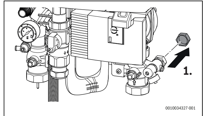
Afb. 20 Aansluiten expansievat
