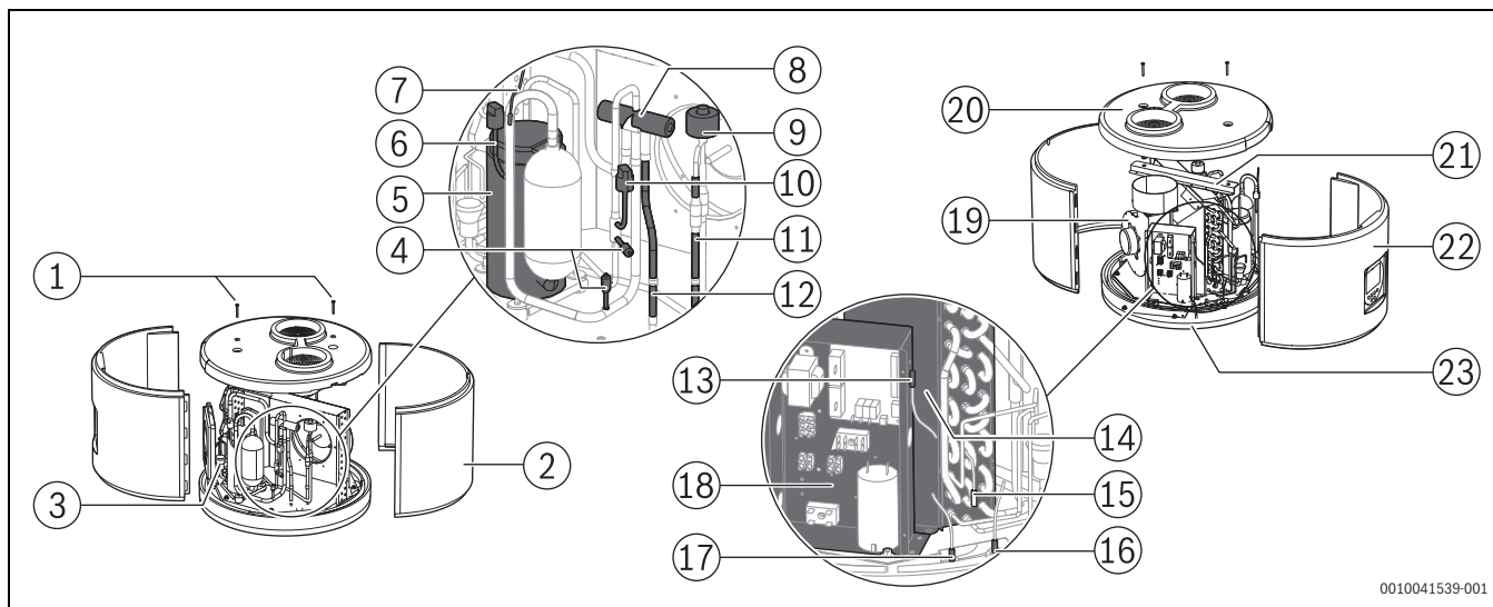
Bild 4 Product overview
