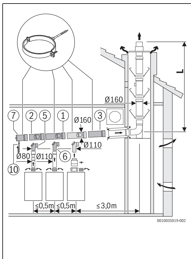
12 DN160 - DN160
