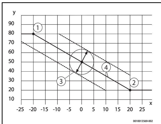
Fig. 4 Courbe de chauffage en fonction de la température extérieure
