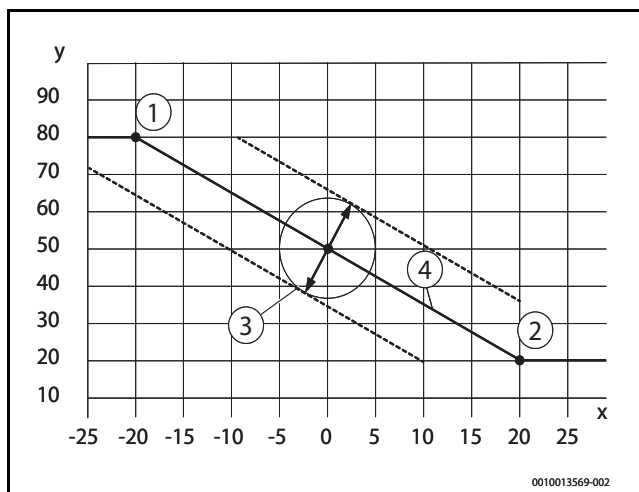
Afb. 4 Weersafhankelijk geregelde stooklijn
