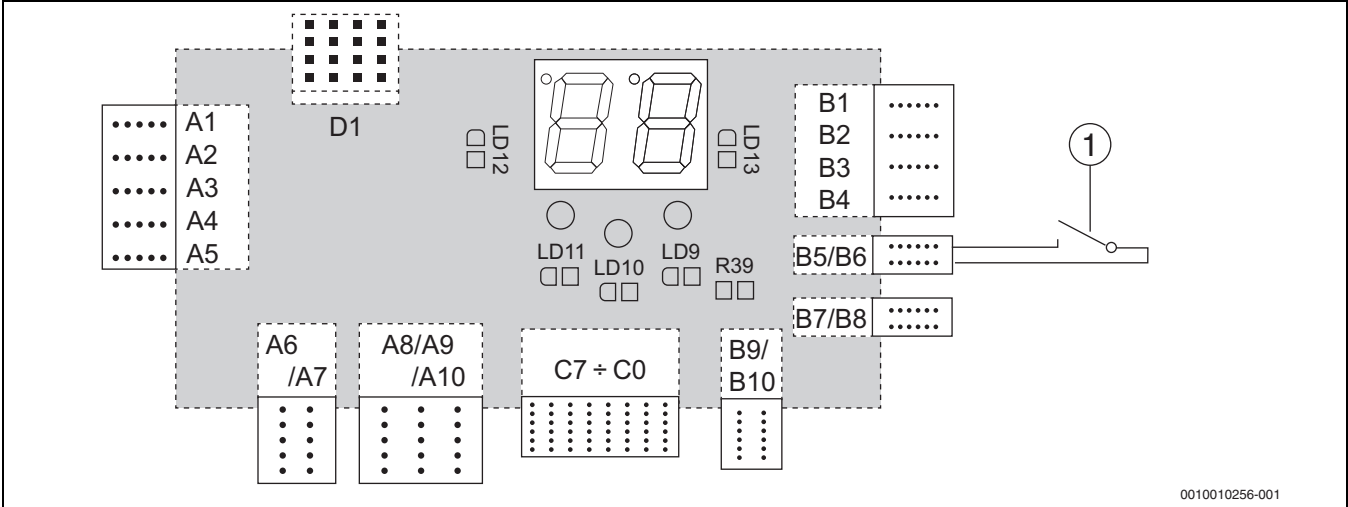
Afb. 23 Aansluiting kamerthermostaat
