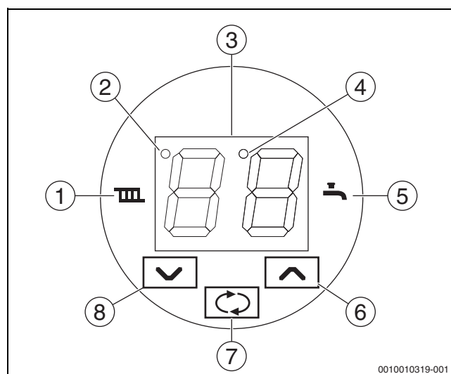
Afb. 34 Bedieningspaneel
