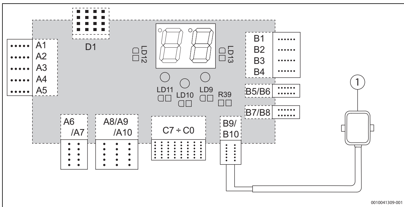
Afb. 33 Een buitentemperatuursensor aansluiten voor equithermische regeling
