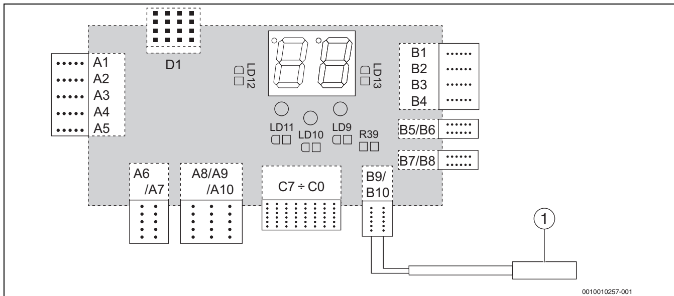
Afb. 32 Aansluiting van een externe temperatuursensor voor de minimale kamertemperatuur of een extra kamerthermostaat
