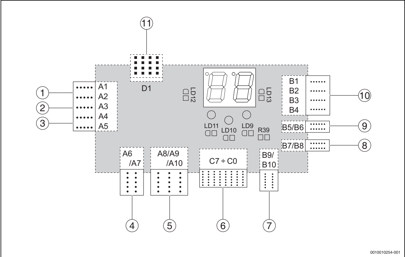
Afb. 22 Elektronica cv-toestel
