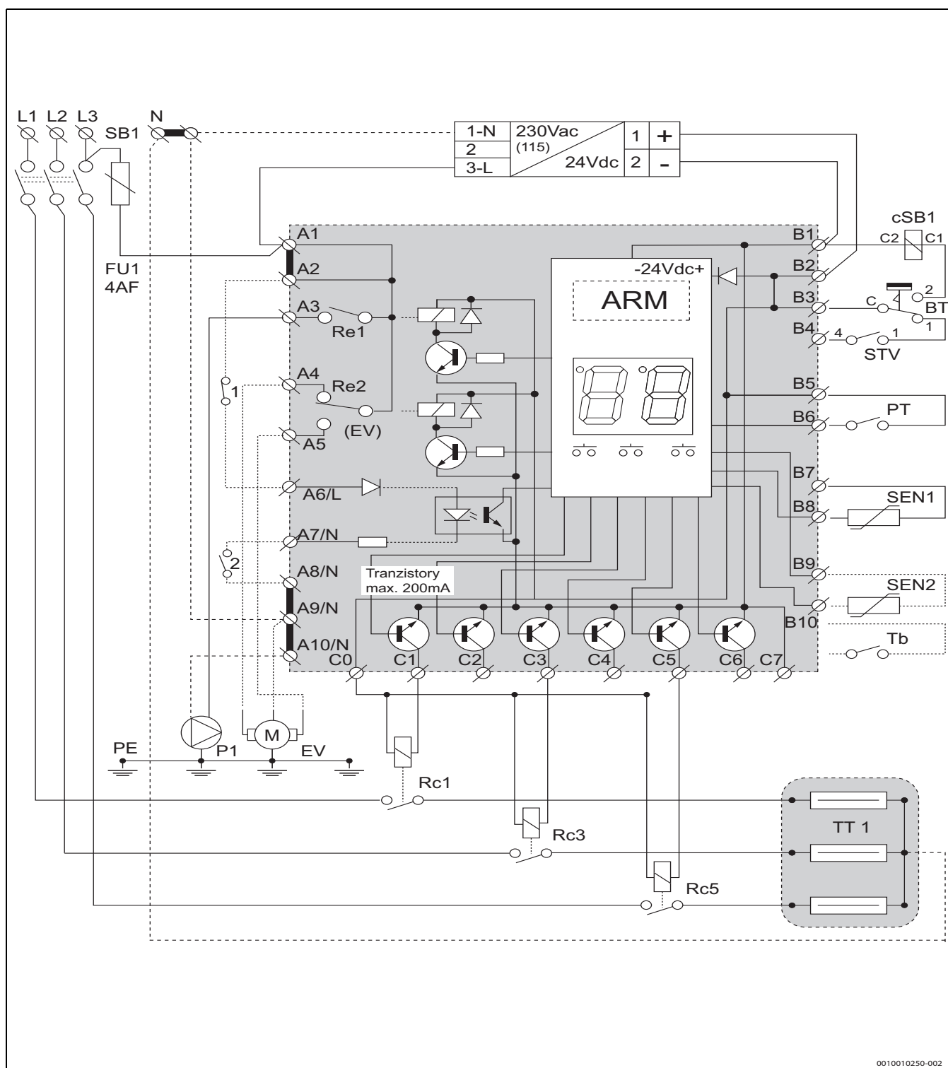
Afb. 20 Bedieningsschema van het cv-toestel Tronic Heat 3500 (4-12 kW), 3x 400/230 VAC
