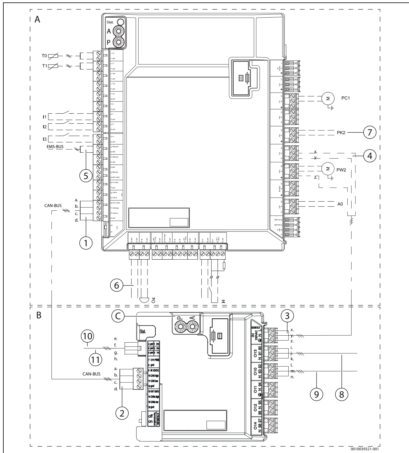
Afb. 9 Aansluitschema uitbreidingsprintplaat (koelstation) en installatieprintplaat (warmtepomp)
