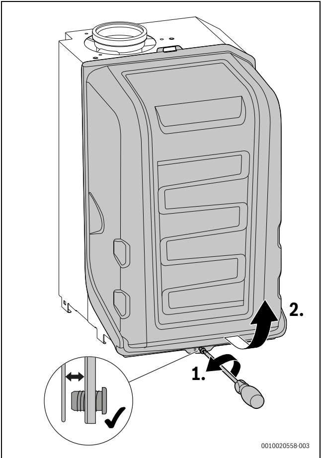
Afb. 37 Branderkap verwijderen
