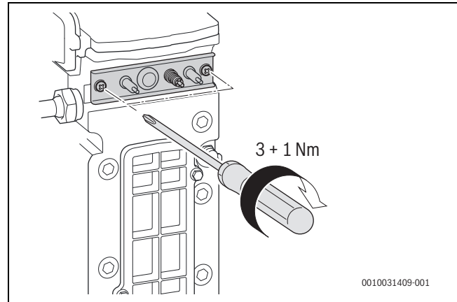
Afb. 42 Elektrodenset inbouwen
