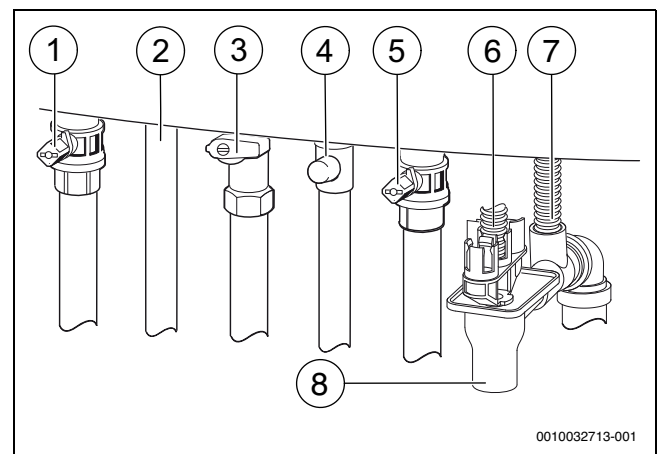
Afb. 31 Gas- en waterzijdige aansluitingen (toeberehen)
