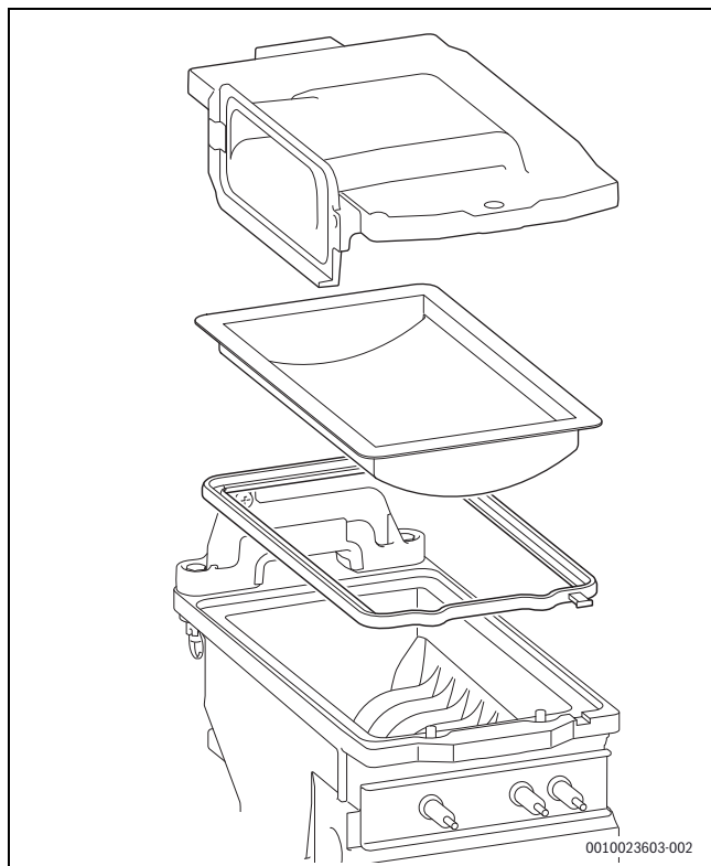
Afb. 45 Brander
