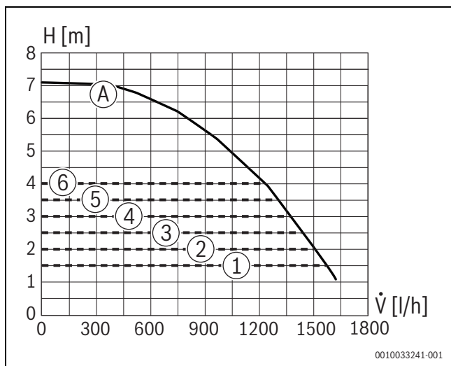
Afb. 68 Pompkarakteristieken en pompcurven
