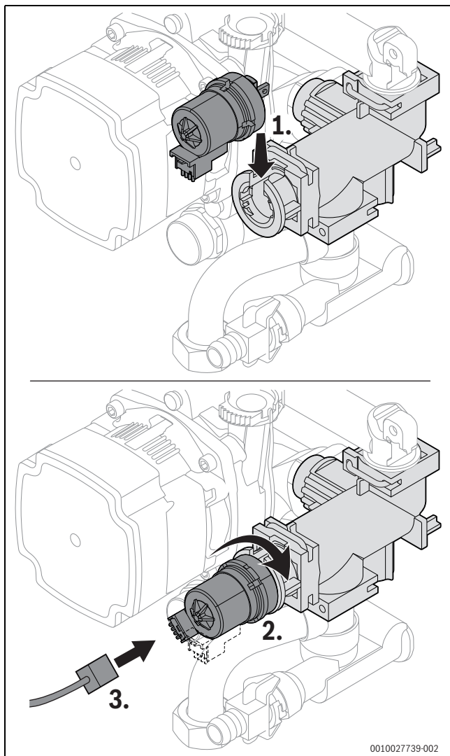
Afb. 65 Motor van de 3-wegklep inbouwen (variant zonder schroeven)
