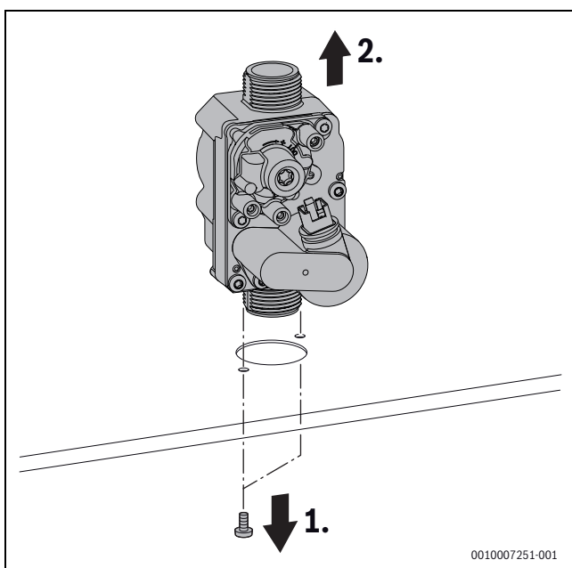
Afb. 63 Gasblok demonteren
