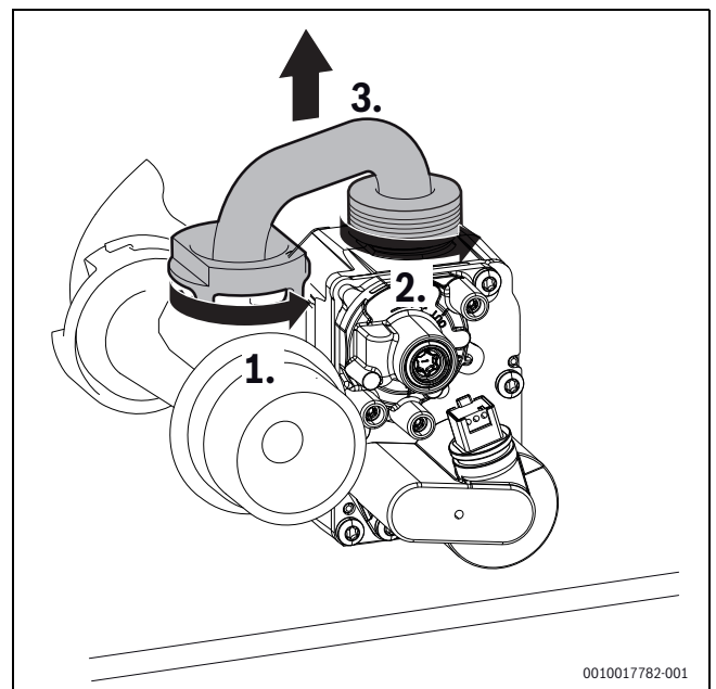
Afb. 61 Gasbuis demonteren
