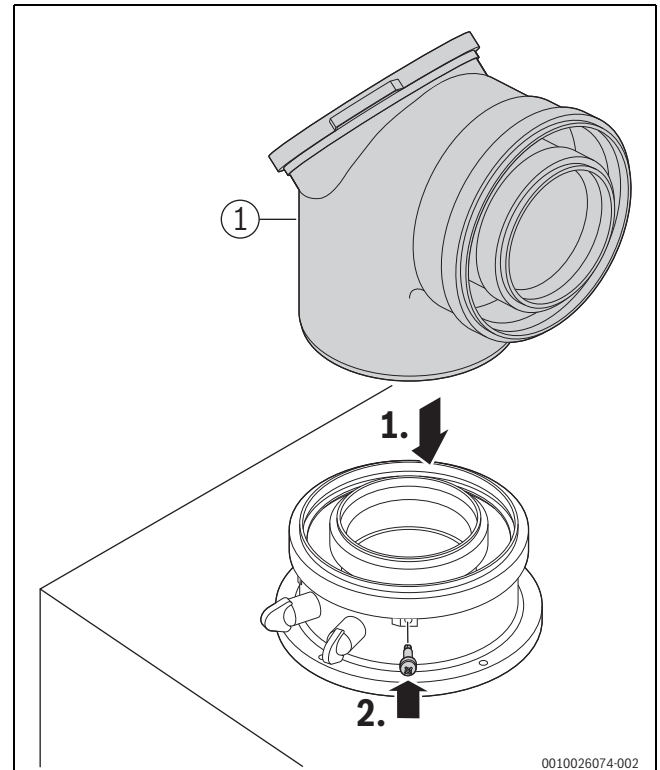
Afb. 30 Breng het rookgastoeberehen aan en borg met schroef
