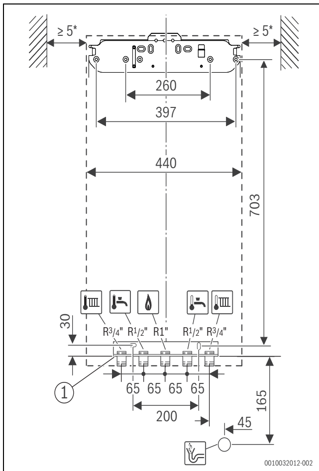
Afb. 3 Vooraanzicht (mm)
