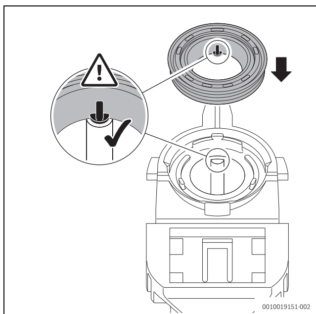
Afb. 58 Dichting correct op de condenssifon plaatsen
