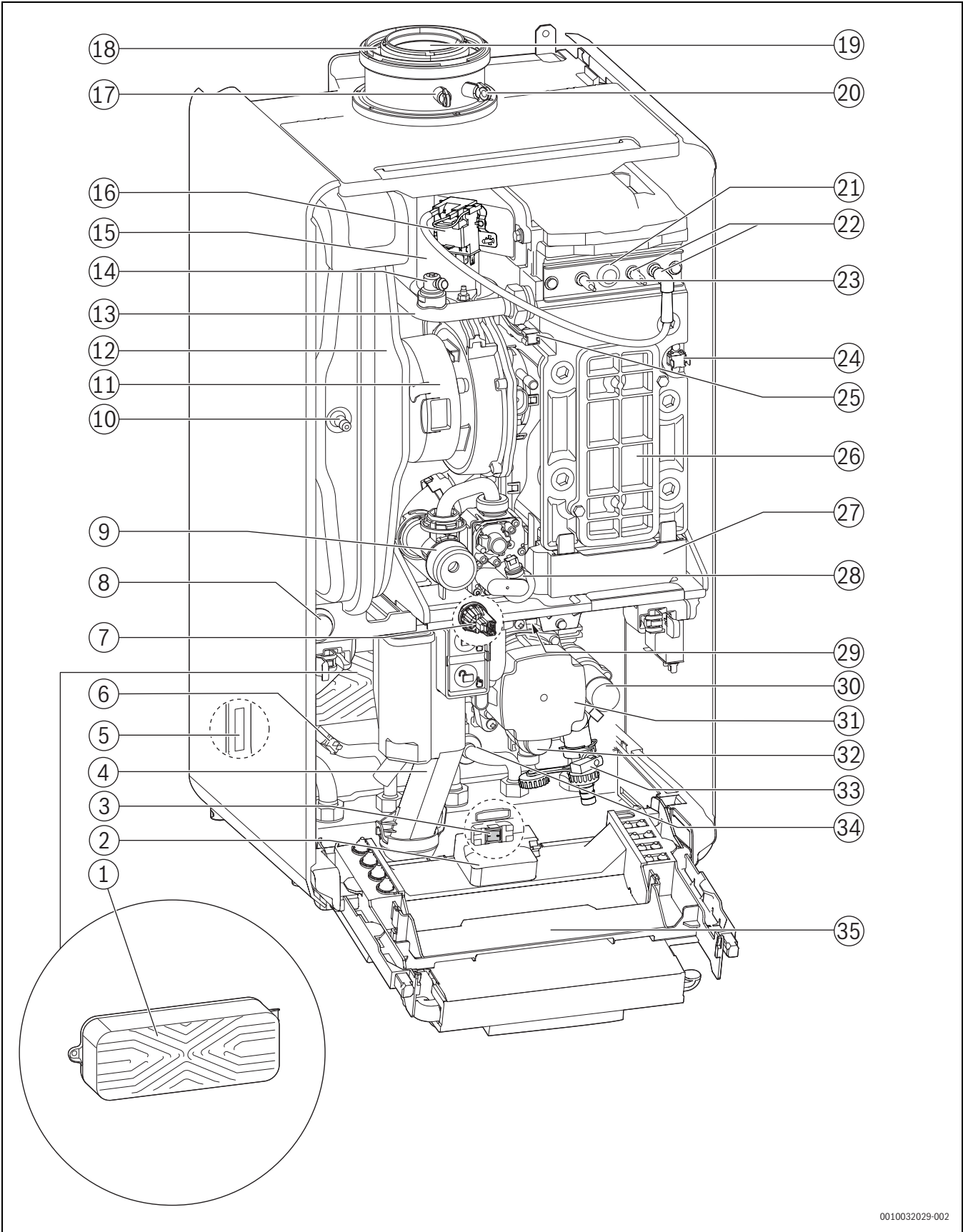
Afb. 4 Productoverzicht
