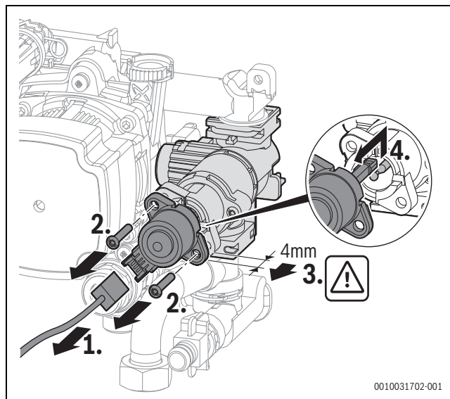
Afb. 66 Motor van de 3-wegklep uitbouwen (variant met schroeven)
