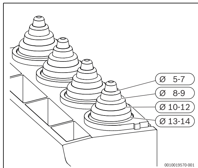
Afb. 33 Aanpassen trekcontlasting aan de kabeldiameter
