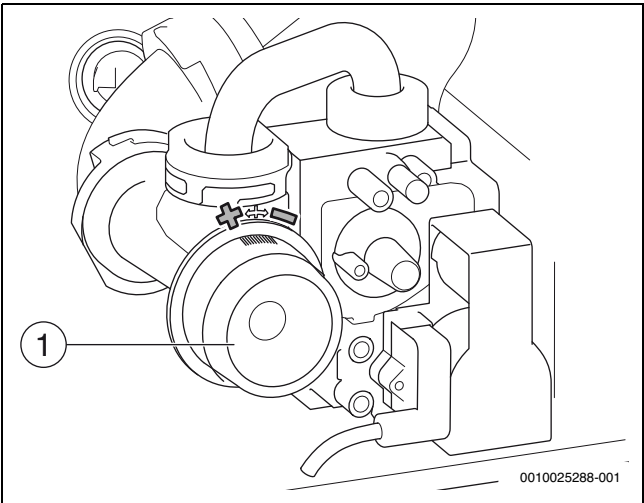
Afb. 38 Gas-/luchtverhouding instellen
