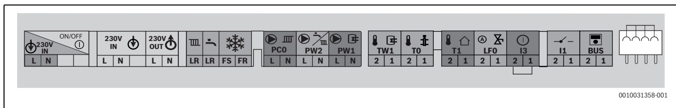
Afb. 34 Klemmenstrook voor extern toebehoren
