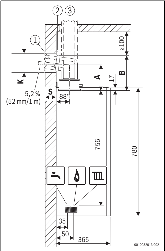
Afb. 2 Zijaanzicht (mm)
