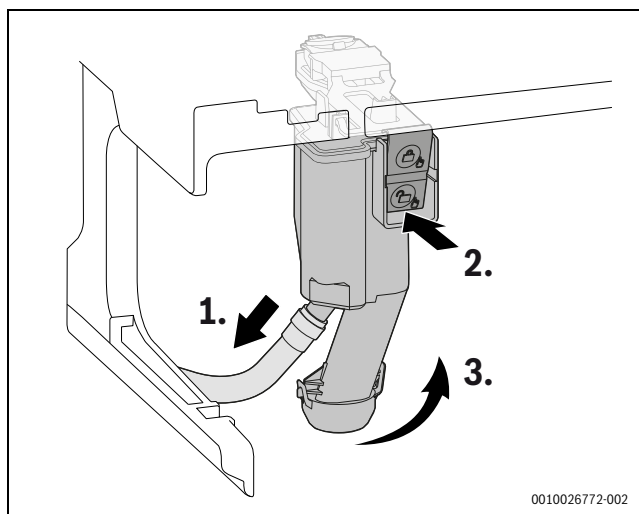
Afb. 57 Condenssifon demonteren
