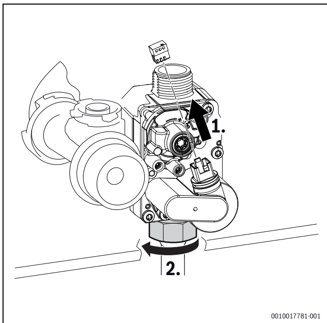
Afb. 62 Stekker lostrekken en wartelmoer losmaken
