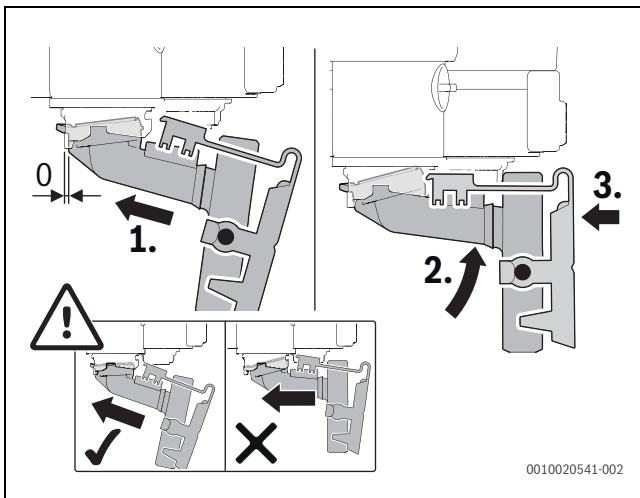
Afb. 60 Condenssifon inbouwen
