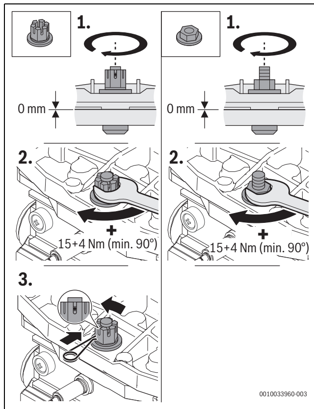
Afb. 46 Draai de moer op het branderdekseel vast
