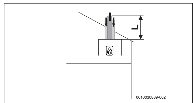
Afb. 10 Verticaal concentrisch luchttoevoer/rookgasafvoersysteem conform C 33x
