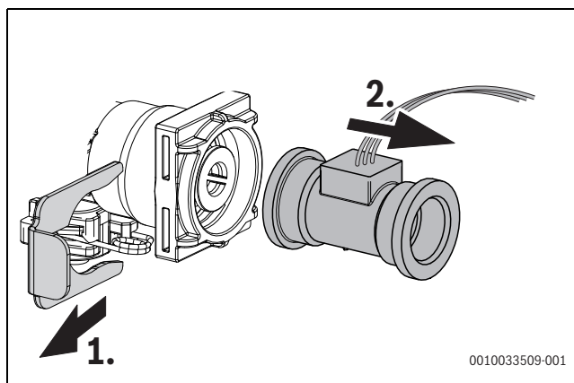
Afb. 50 Turbine op koudwaterbuis demonteren
