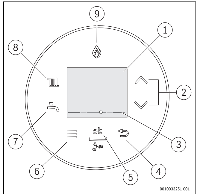
Afb. 36 Bedieningspaneel
