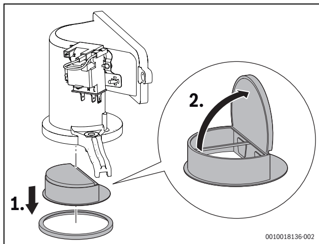
Afb. 48 Terugslagklep in de menginrichting
