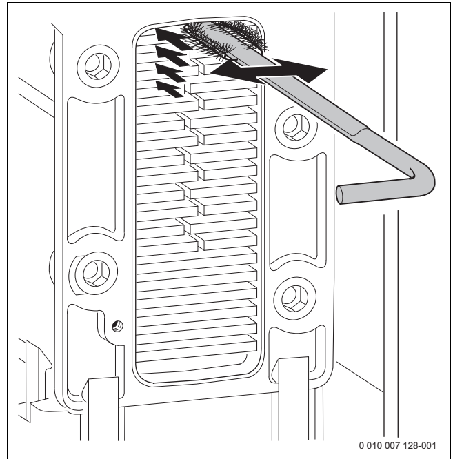
Afb. 54 Reinig het verwarmingslichaam met de borstel
