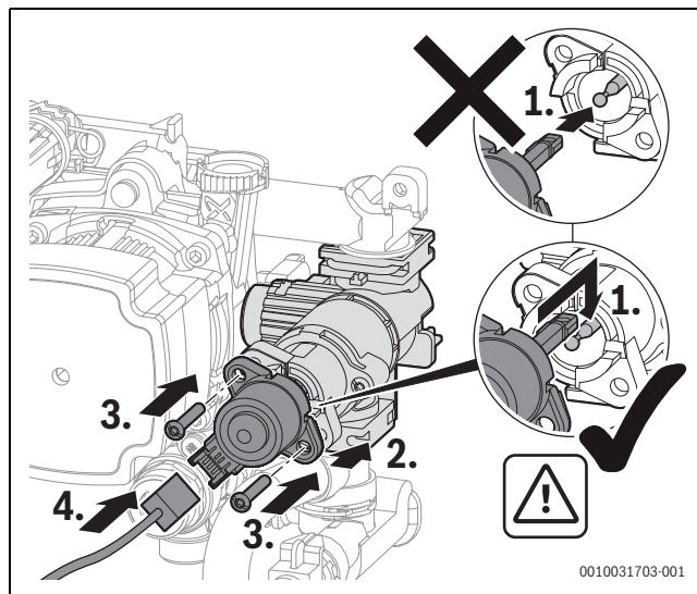
Afb. 67 Motor van de 3-wegklep inbouwen (variant met schroeven)
