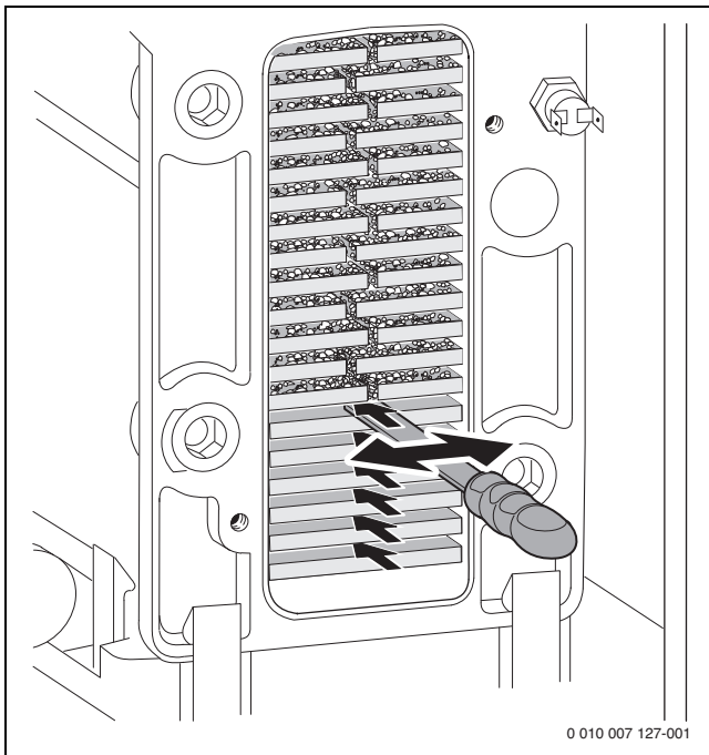
Afb. 53 Reinigingsgereedschap
