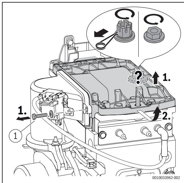
Afb. 44 Branderdekseel demonteren
