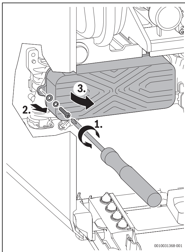
Afb. 51 Platenwarmtewisselaar demonteren
