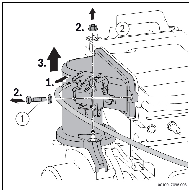
Afb. 47 Menginrichting demonteren
