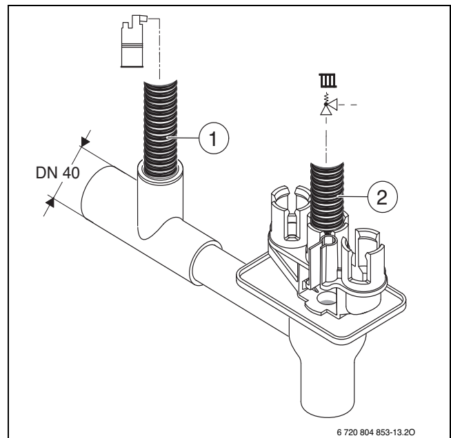
Afb. 27 Monteer de condensaat slang en de slang van het veiligheidsventiel op het sifon
