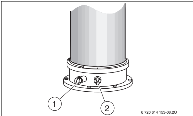
Afb. 41 Rookgasmeetpunt en verbrandingsluchtmeetpunt
