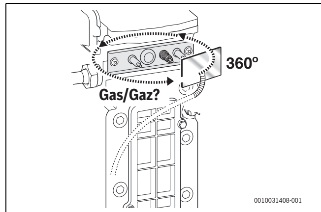
Afb. 43 Dichtheid controleren
