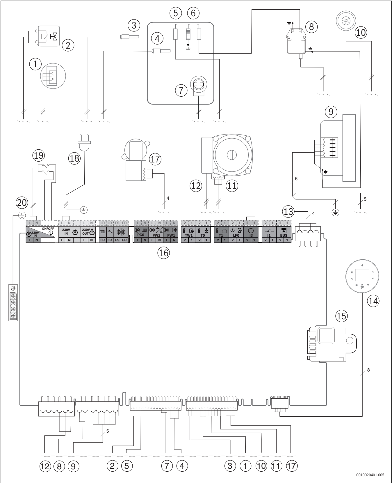
Afb. 69 Elektrische bedrading
