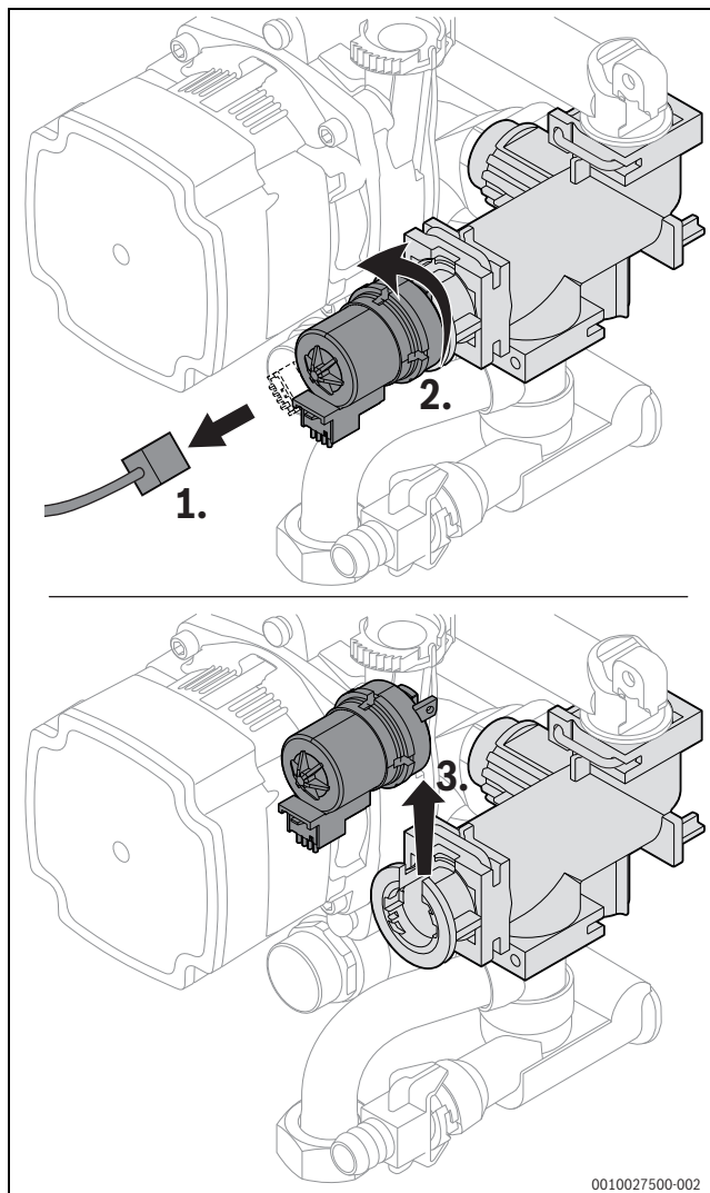
Afb. 64 Motor van de 3-wegklep uitbouwen (variant zonder schroeven)
