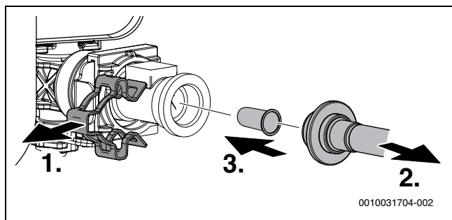
Afb. 49 Het filter uit de koudwaterbuis demonteren
