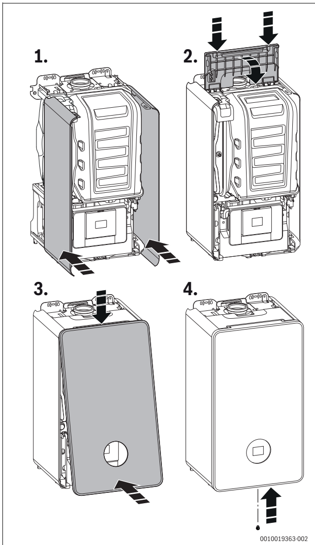
Afb. 35 Mantel monteren
