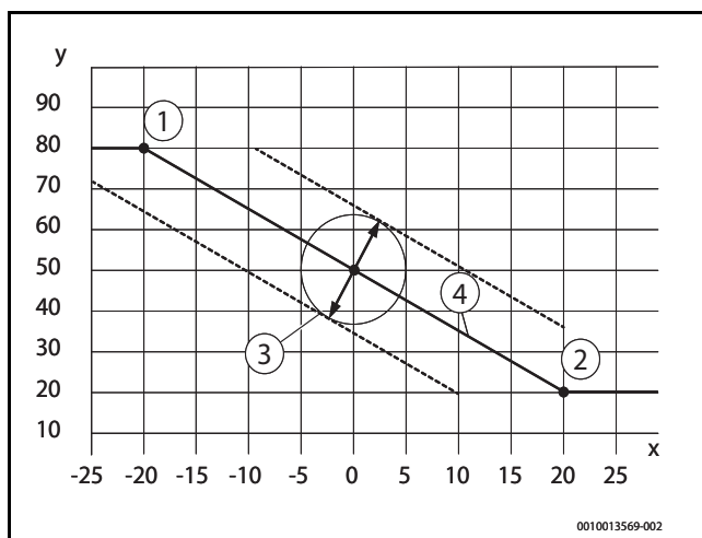
Bild 4 Außentemperaturgeführte Heizkurve
