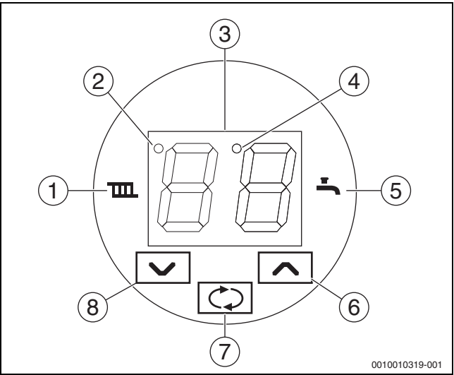
Bild 3 Bedienfeld
