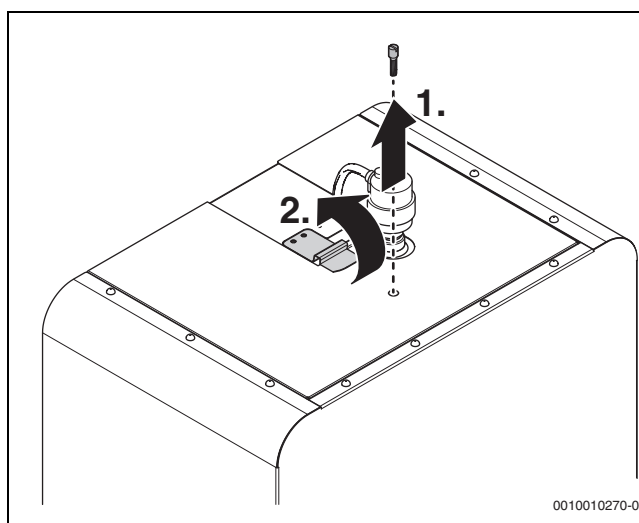
Bild 7 Lösen der Rastfeder
