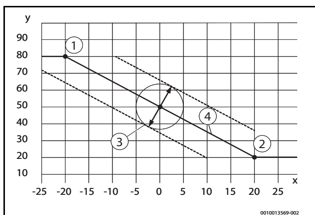
Bild 35 Außentemperaturgeführte Heizkurve
