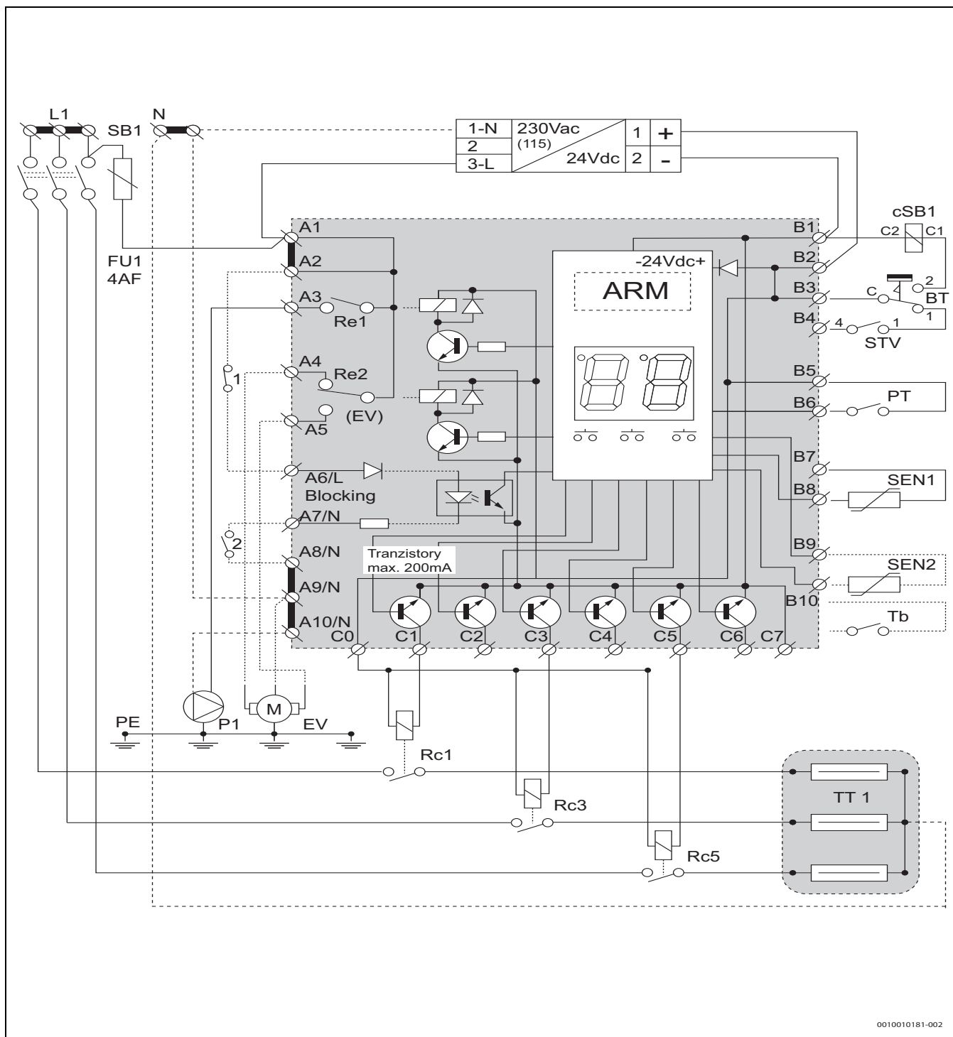
Bild 19 Anschlussplan des Heizgerätes Tronic Heat 3500 (4-12 kW), 1x 230 V AC
