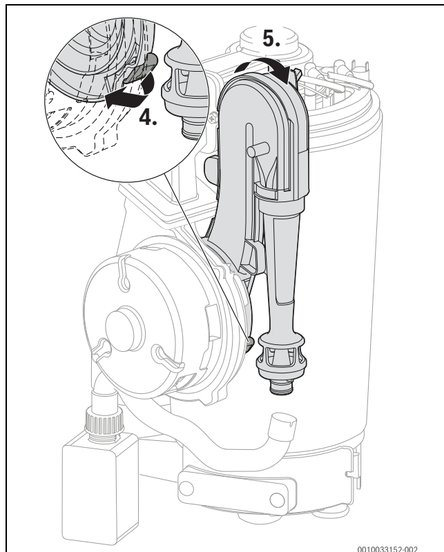
Afb. 115 Venturi afnemen
