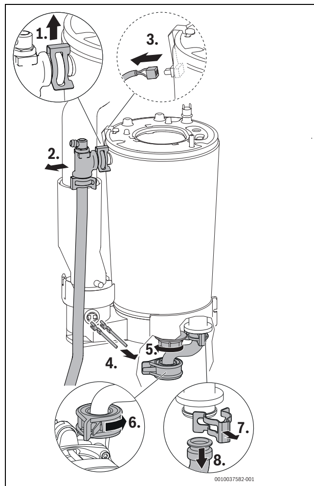
Afb. 129 Maak de aanvoerleiding los, trek de kabel los en maak de retourleiding los
