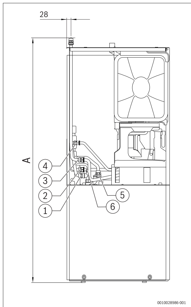
Afb. 13 Aanzicht van de linkerzijde (afmetingen in mm)
