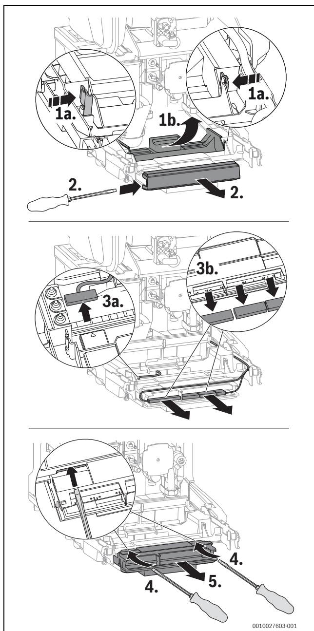
Afb. 143 Besturing uitnemen
