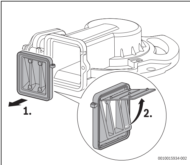
Afb. 119 Controleer de terugstroombeveiliging in de menginrichting
