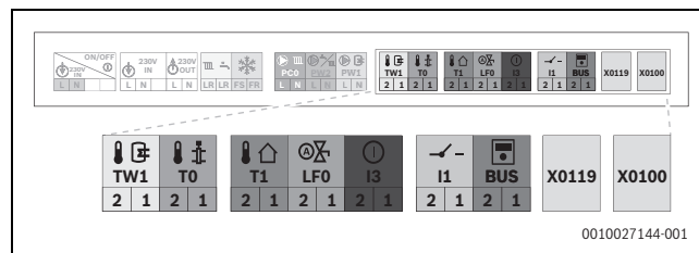
Afb. 85 Laagspanningsbereik: klemmenstrook
