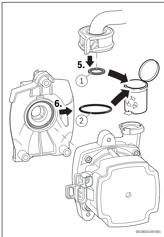
Afb. 134 Dichtingen afvoeren
