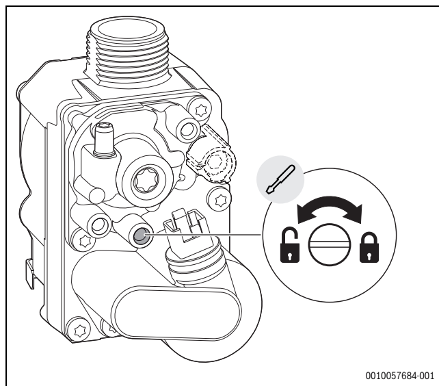
Afb. 103 Gasaansluitdruk meten
