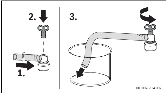
Afb. 76 Warmwatercircuit en cv-circuit ontluchten
