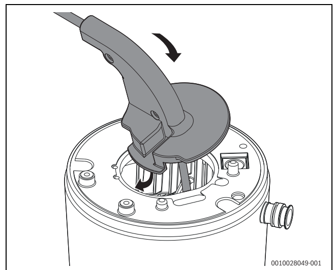
Afb. 123 Borstel in het verwarmingslichaam plaatsen
