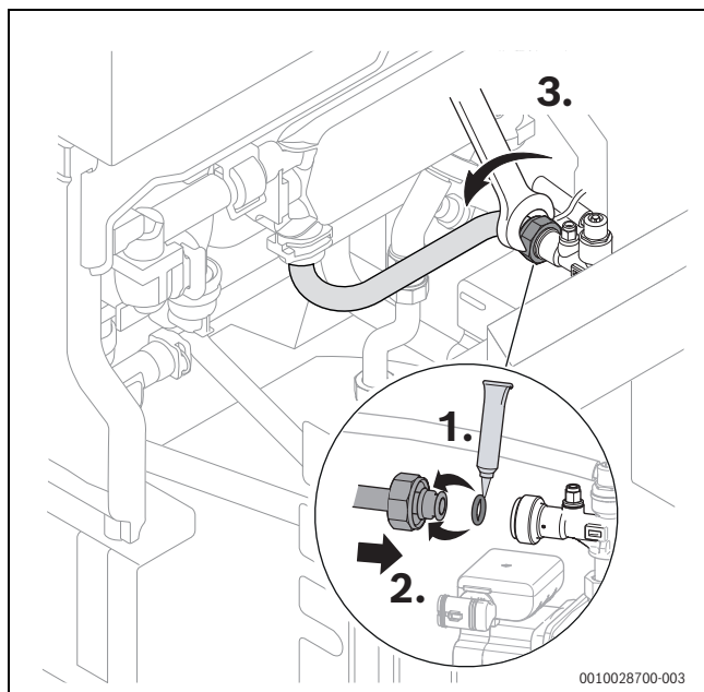
Afb. 61 Koudwaterbuis van het boilerlaadcircuit aansluiten
