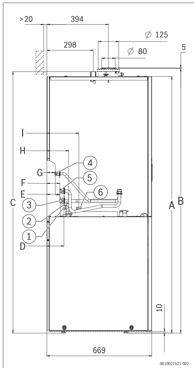
Afb. 8 Aanzicht van de linkerkzijde (afmetingen in mm)
