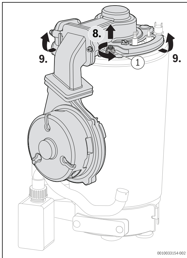
Afb. 117 Branderdekseel met ventilator en menginrichting afnemen
