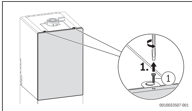
Afb. 108 Borgschroef losmaken
