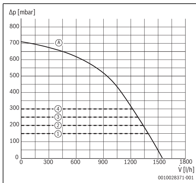
Afb. 153 Pompkarakteristiek en pompcurve (17/24 kW)
