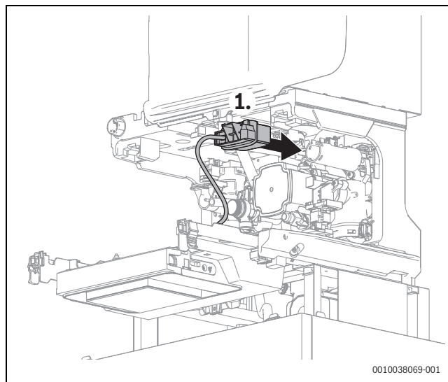
Afb. 64 Key-houder aan de achterkant van het toestel doorvoeren
