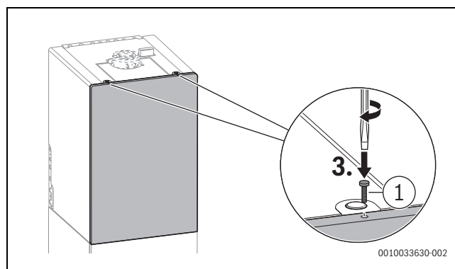
Afb. 92 Voorpaneel van de toestelmantel met schroef uit leveringsomvang borgen
