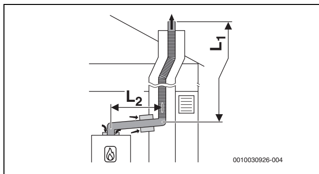
Afb. 32 Flexibele rookgasafvoer door de schacht conform B 53p met open luchttoevoer aan toestel en concentrisch verbindingstuk tussen opstellingsruimte en schacht
