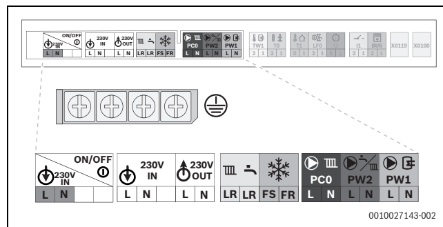
Afb. 84 Netspanningsbereik: klemmenstrook
