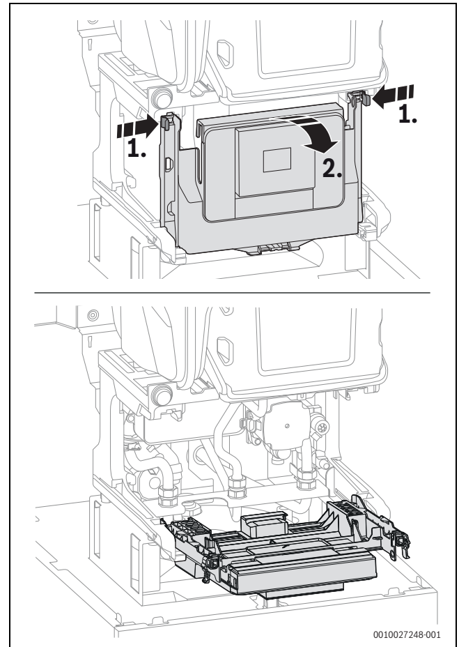
Afb. 111 Besturing naar beneden klappen
