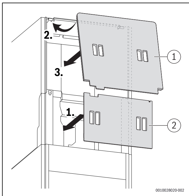
Afb. 94 Warmte-isolatie aan de achterzijde aanbrengen (toebehoren SF 13)
