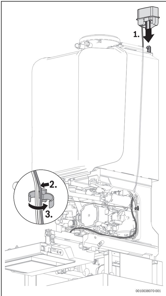
Afb. 65 Key-houder in de insteekplaats plaatsen en de kabel in de kabelhouder bevestigen
