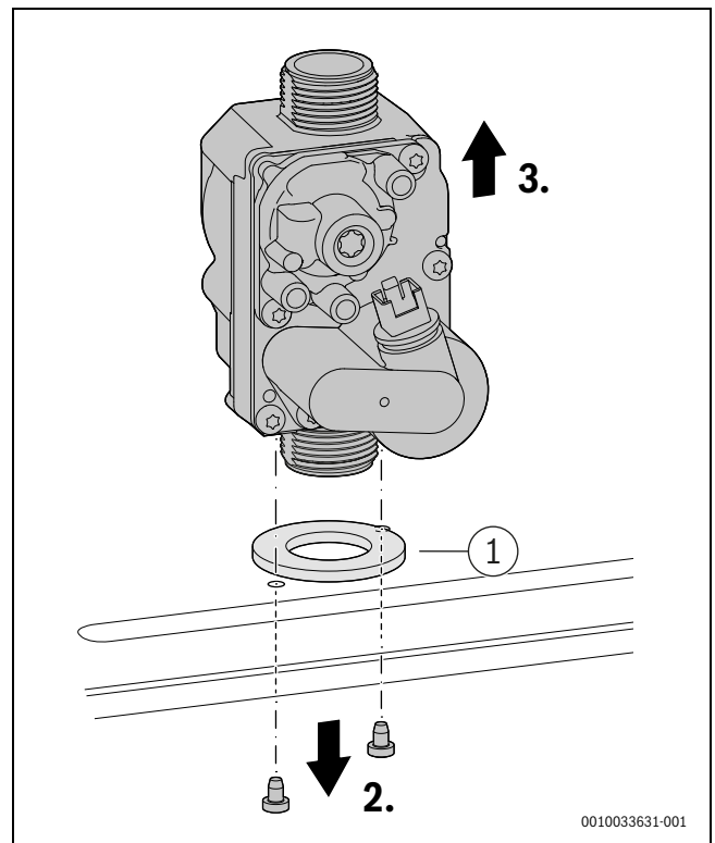
Afb. 138 Gasblok demonteren
