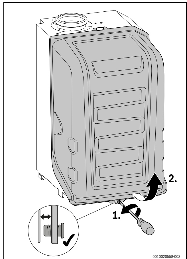
Afb. 102 Branderkap verwijderen
