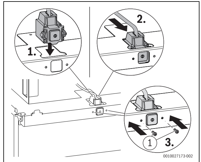
Afb. 78 Aan-uitschakelaar bevestigen
