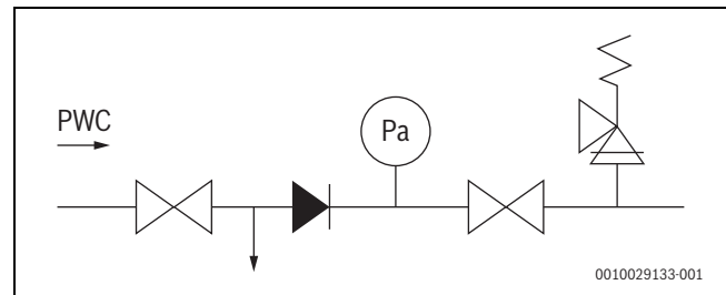
Afb. 67 Voorbeeld: veiligheidsgroep voor expansiewater conform EN 1488
