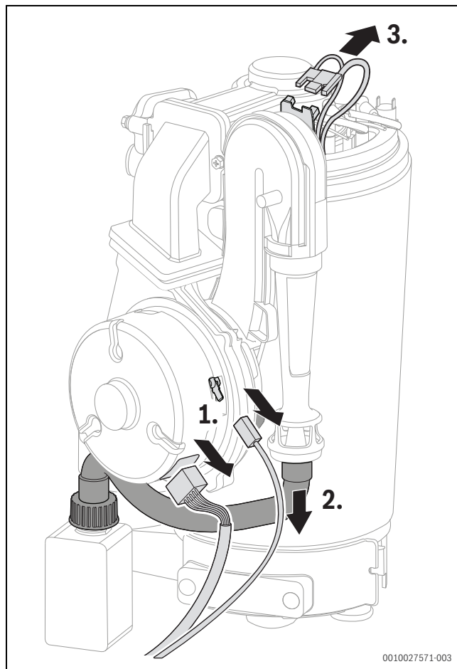
Afb. 114 Stekker en gasslang lostrekken
