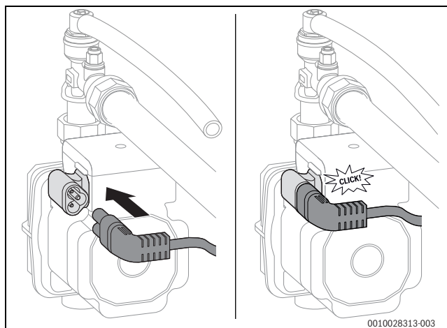
Afb. 86 Stratificatiepomp elektrisch aansluiten
