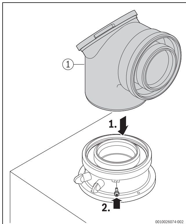
Afb. 72 Breng het rookgastoebehoren aan en borg met schroef
