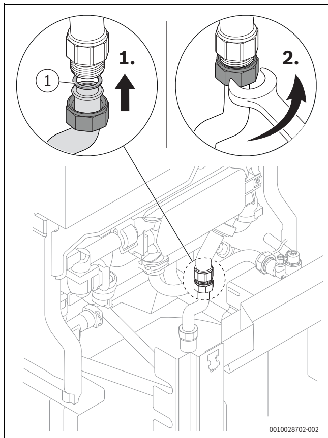
Afb. 62 Warmwaterbuis van het boilerlaadcircuit op de boiler aansluiten
