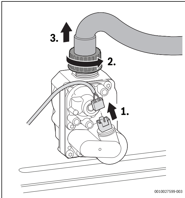
Afb. 135 Stekker op het gasblok lostrekken en wartelmoer met gasslang afnemen
