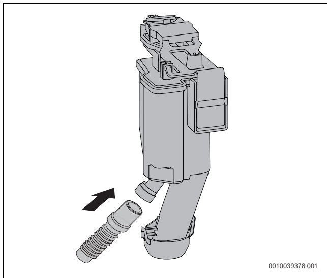
Afb. 69 Slang op condenssifon aansluiten
