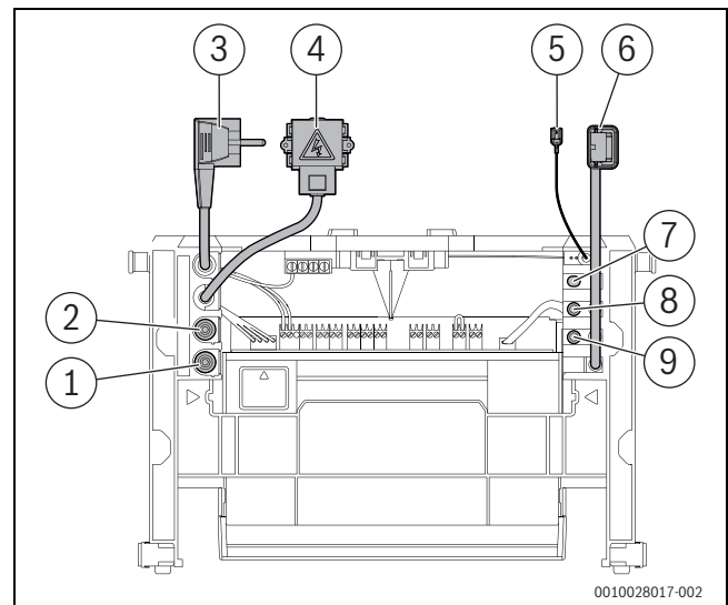
Afb. 81 Uitleveringstoestand van de besturing met aangesloten componenten
