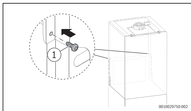
Afb. 93 Zijpanelen van de toestelmantel aan de linker- en rechterzijde vastschroeven
