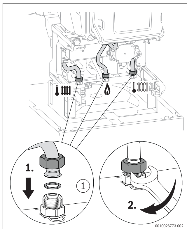
Afb. 60 CV-aanvoer, gas, cv-retour aansluiten
