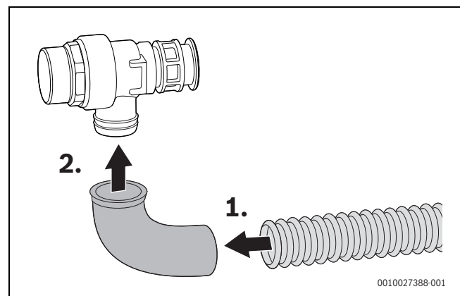
Afb. 68 Slang op veiligheidsventiel aansluiten
