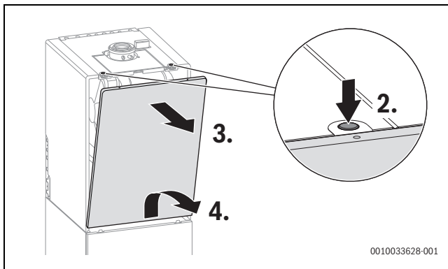
Afb. 109 Voorpaneel van de toestelmantel afnemen
