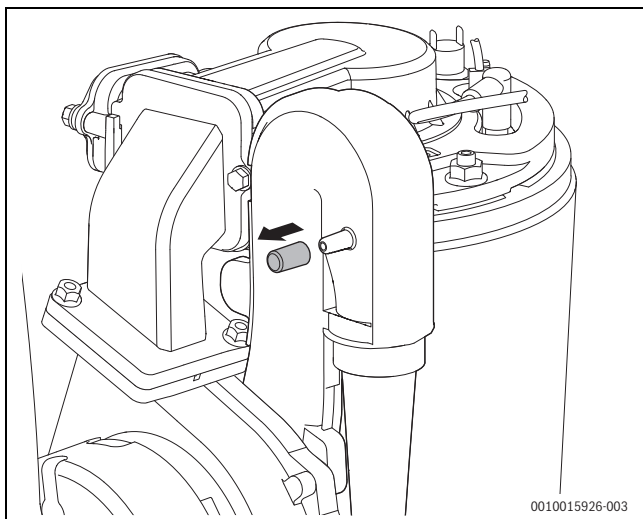
Afb. 112 Meetnippel op de menginrichting
