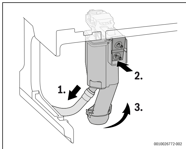
Afb. 144 Condenssifon demonteren
