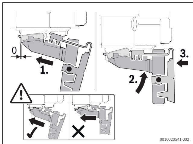
Afb. 63 Plaats de condenssifon weer terug en controleer deze op goede bevestiging
