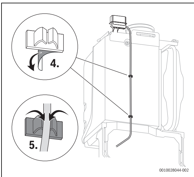
Afb. 66 Kabelhouder aan de achterzijde van het toestel aanbrengen en kabel bevestigen
