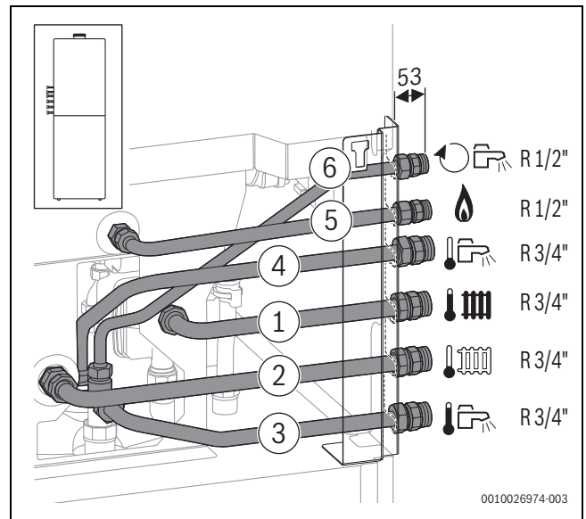
Afb. 11 Aanzicht van de achterzijde (afmetingen in mm): toebehoren CS 10 aan de linkerszijde gemonteerd
