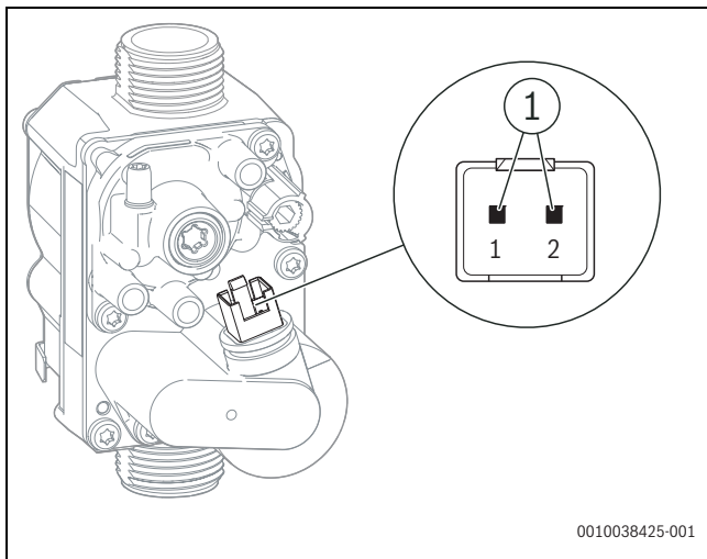
Afb. 113 Meetpunten op het gasblok
