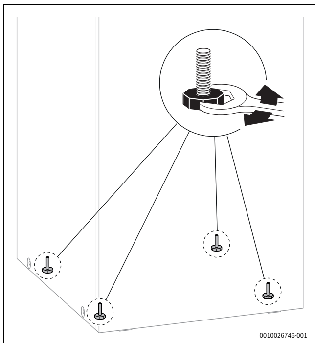
Afb. 95 Op de uiteindelijke opstellingsplaats oneffenheden in de vloer met de stelpoten opvangen
