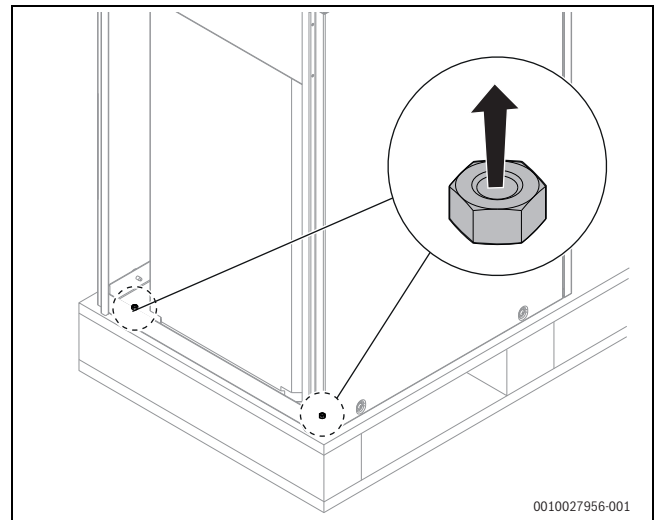
Afb. 49 Transportbeveiliging onder op de achterzijde van de boiler verwijderen
