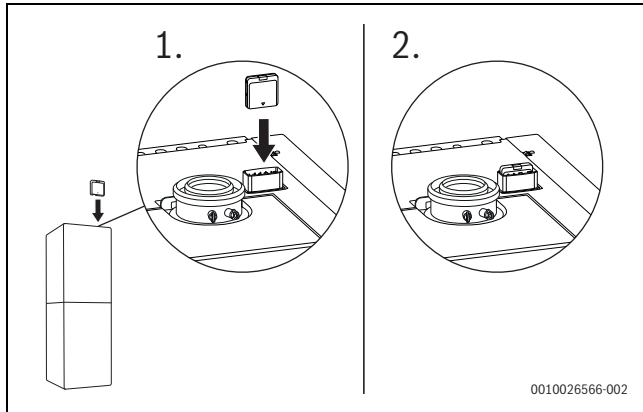
Afb. 73 Control Key in de Key-houder steken
