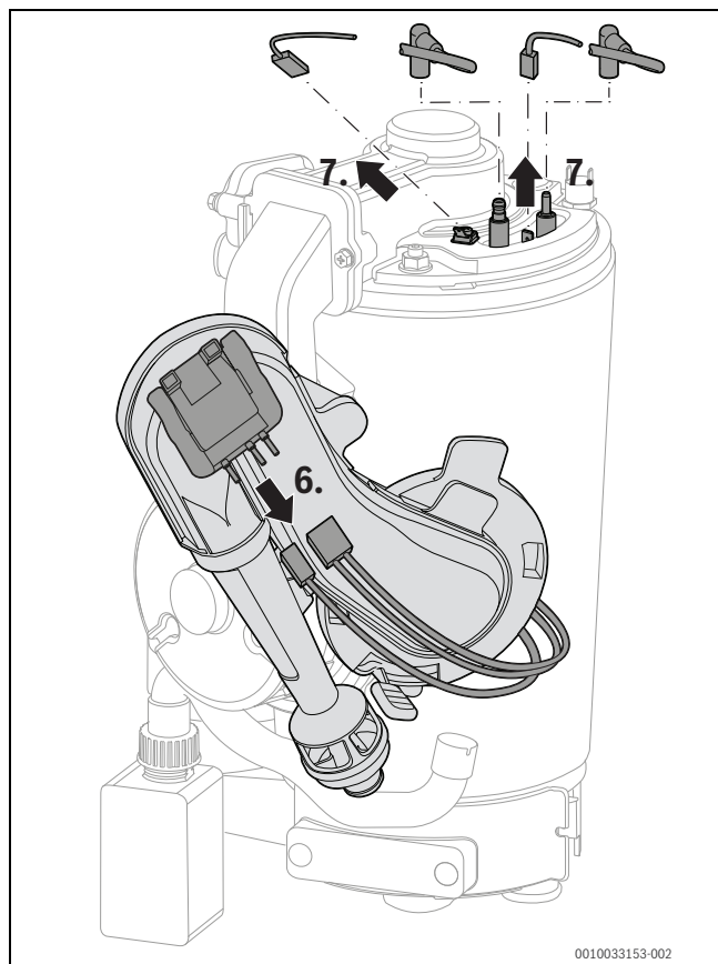
Afb. 116 Trek de kabel los
