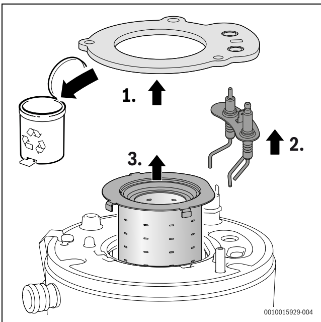
Afb. 120 Brander uitnemen
