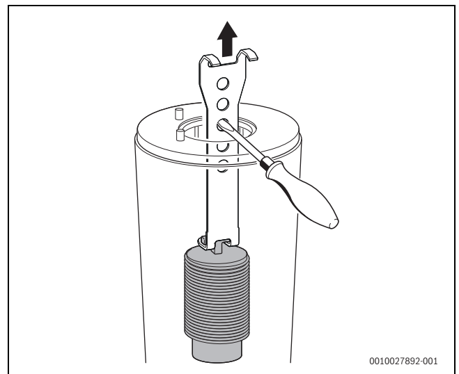
Afb. 122 Neem de onderste rookgasremmer uit
