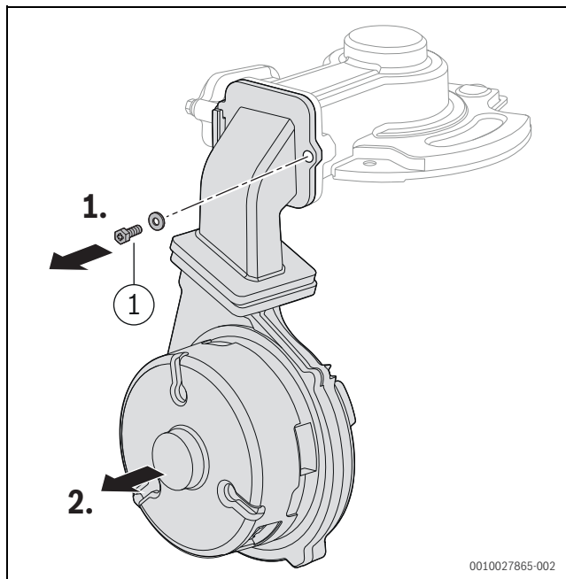
Afb. 118 Ventilator en menginrichting demonteren
