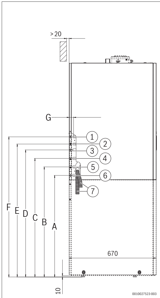
Afb. 10 Aanzicht van de linkerszijde (afmetingen in mm)
