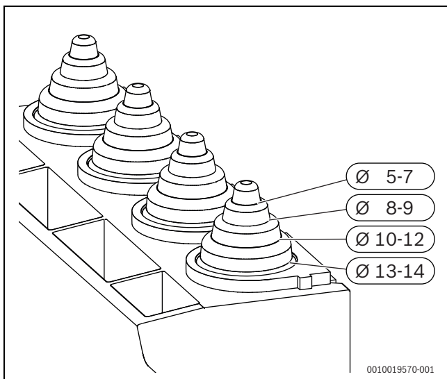
Afb. 83 Trekontlasting op kabeldiameter aanpassen
