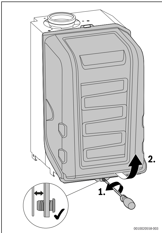
Afb. 110 Branderkap verwijderen
