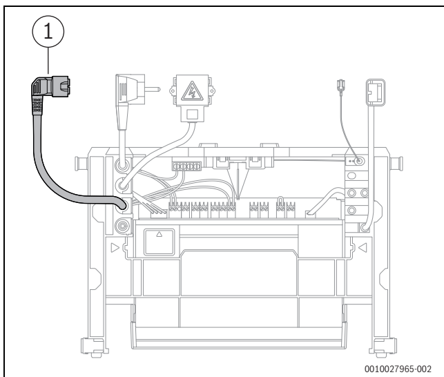
Afb. 82 Insteekplaats voor de aansluitkabel van de stratificatiepomp
