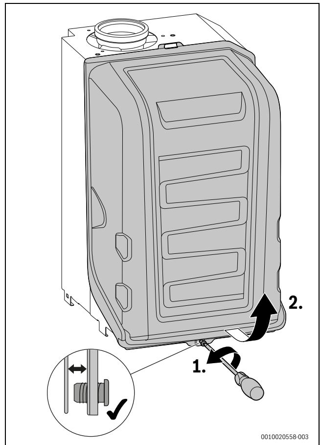
Afb. 75 Branderkap verwijderen
