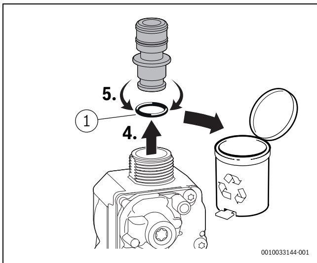
Afb. 136 Gassmoorklep afnemen
