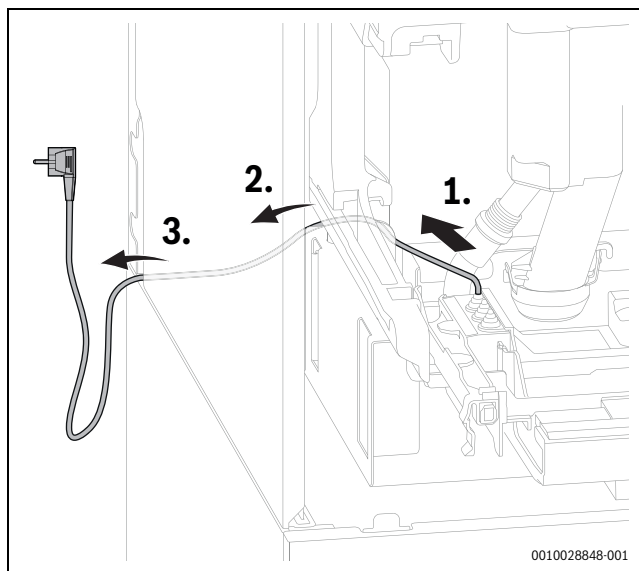
Afb. 87 Kabelinstallatie netkabel
