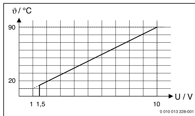
Fig. 2 Relation linéaire entre le signal 0-10 V (U en Volt) et la température de départ demandée \theta (en °C par rapport à la plage température de départ minimale à maximale [réglage de base 20 °C à 90 °C])
