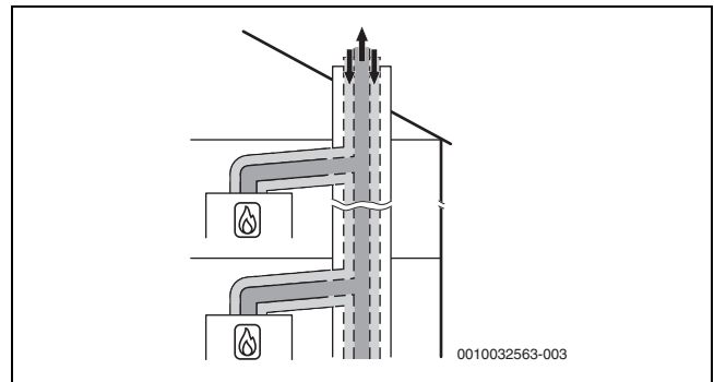
Afb. 19 Collectief systeem conform C (10)3x met concentrisch luchttoevoer/rookgasafvoersysteem in opstellingsruimte
