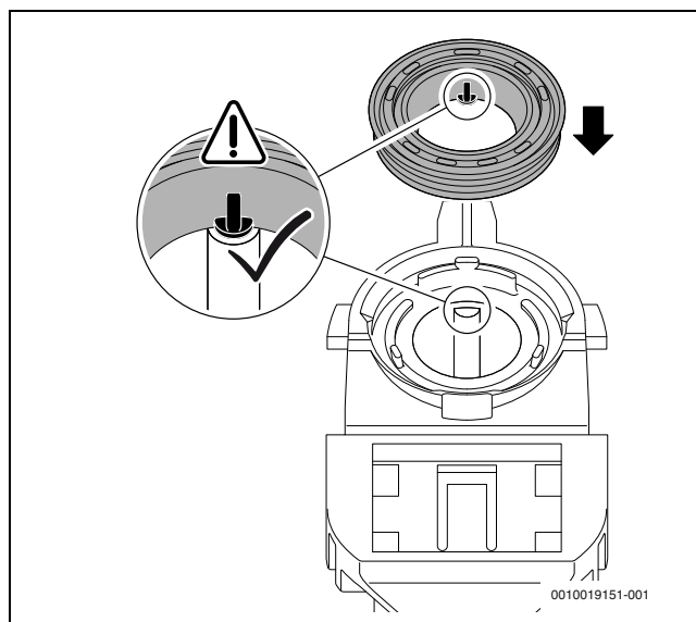
Afb. 62 Plaats de dichting correct op de condenssifon
