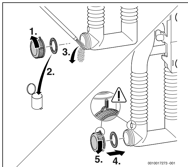
Afb. 60 Condenssifon reinigen
