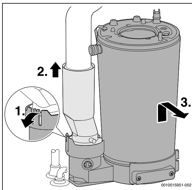
Afb. 74 Warmteblok demonteren
