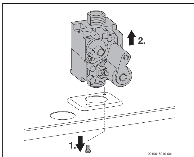
Afb. 69 Demonteren gasblok
