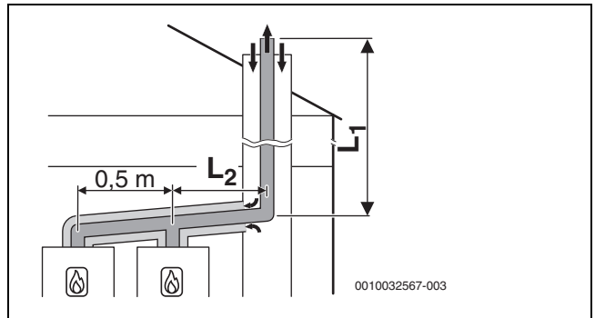
Afb. 28 Cascade met 2 toestellen:
