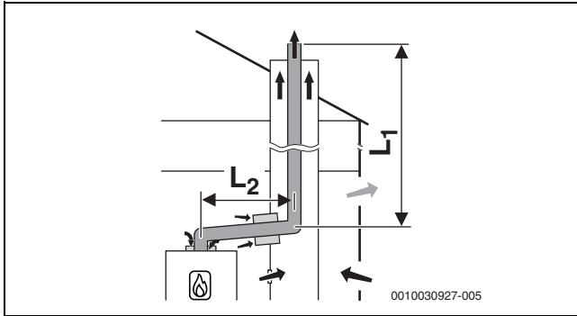
Afb. 17 Starre rookgasafvoer door de schacht conform B 53p met open luchttoevoer aan het toestel en enkelwandige rookgasafvoerbuys in de opstellingsruimte, beluchtingsopening in schacht
