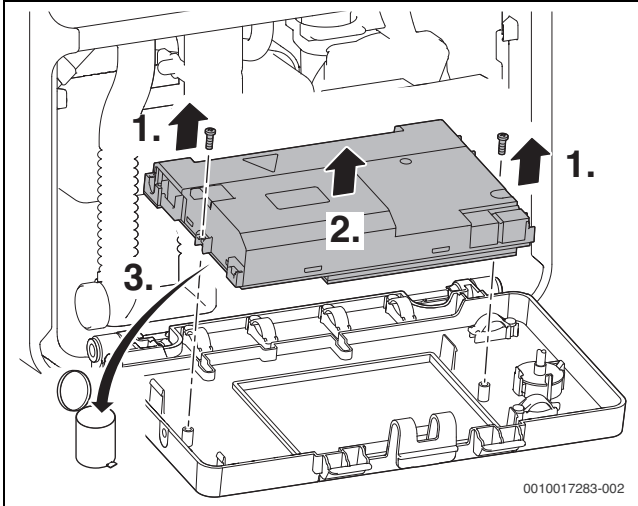
Afb. 75 Toestelelektronica vervangen
