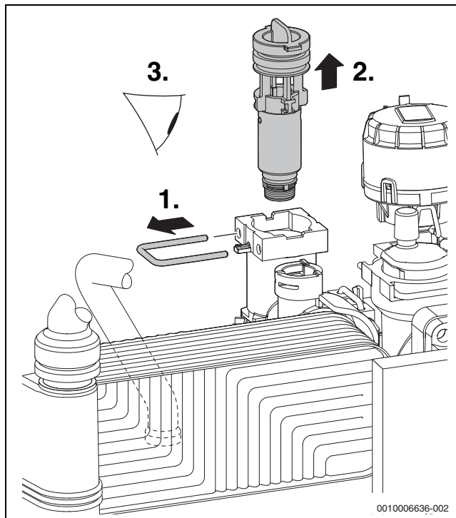
Afb. 66 Controleren filter in koudwaterleiding
