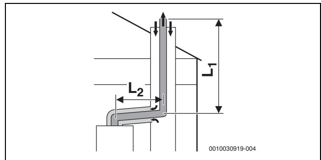
Afb. 13 Star rookgasafvoertraject conform C 93x in de schacht en concentrische verbindingsleiding in de opstellingsruimte
