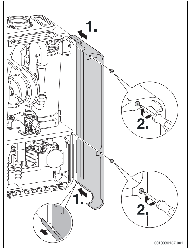
Afb. 77 Zijmantels aanbrengen
