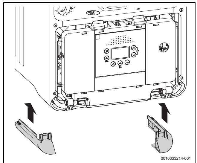
Afb. 78 Kunststof strips zijkant plaatsen
