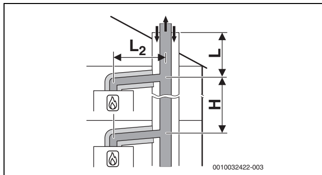
Afb. 25 Collectief systeem conform C_{(14)3x} met collectief star rookgasafvoersysteem en concentrisch luchttoevoer/rookgasafvoersysteem in opstellingsruimte
