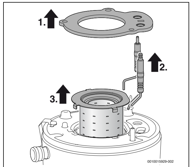
Afb. 53 Brander wegnemen
