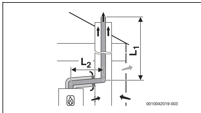
Afb. 15 Starre rookgasafvoer door de schacht conform B 53p met open luchttoevoer via concentrische verbindingsbuis in de opstellingsruimte, luchtrooster in schacht
