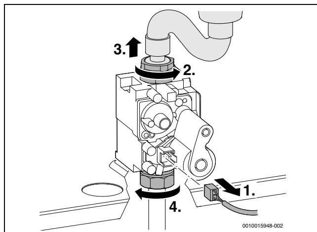
Afb. 68 Trek de stekker los en maak de wartelmoeren los
