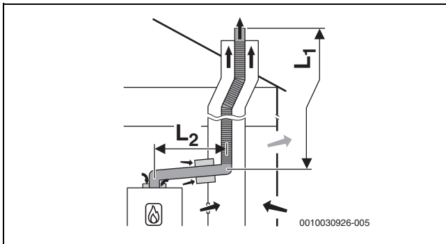
Afb. 18 Flexibele rookgasafvoer door de schacht conform B 53p met open luchttoevoer aan toestel en enkelwandige rookgasafvoerbuys in opstellingsruimte, beluchtingsopening in schacht
