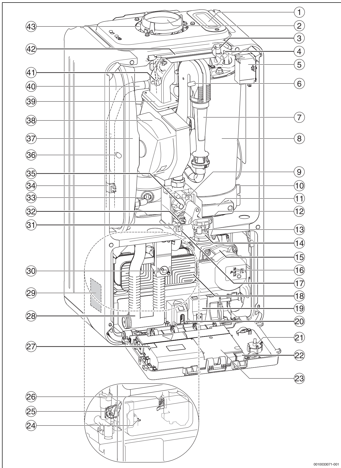
Afb. 3 Productoverzicht
