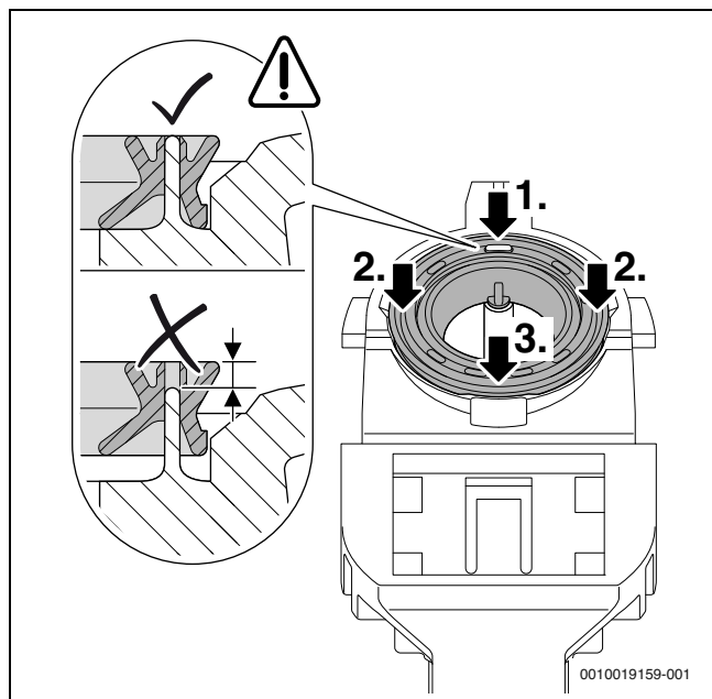
Afb. 63 Aandrukken dichting
