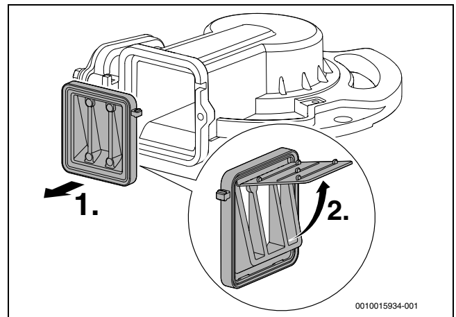
Afb. 52 Terugslagklep in de menginrichting
