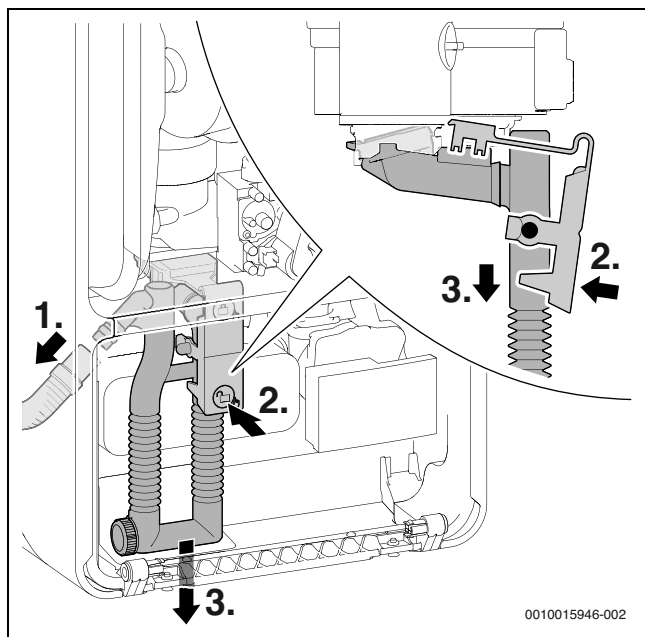
Afb. 59 Condenssifon demonteren
