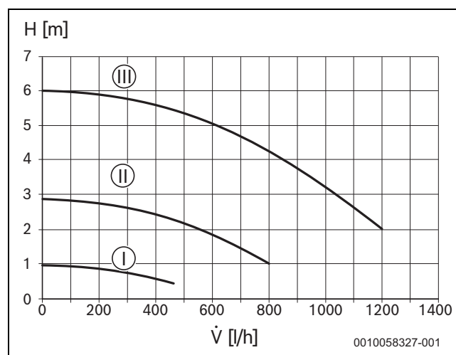
Afb. 44 Curve van de cv-pomp (constante druk)
