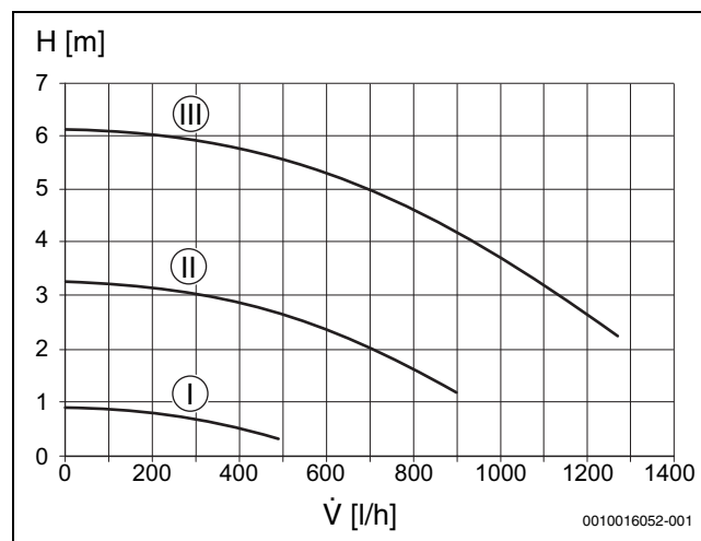
Afb. 43 Karakteristiek van de cv-pomp (constant toerental)
