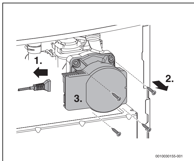
Afb. 70 CV-pomp demonteren
