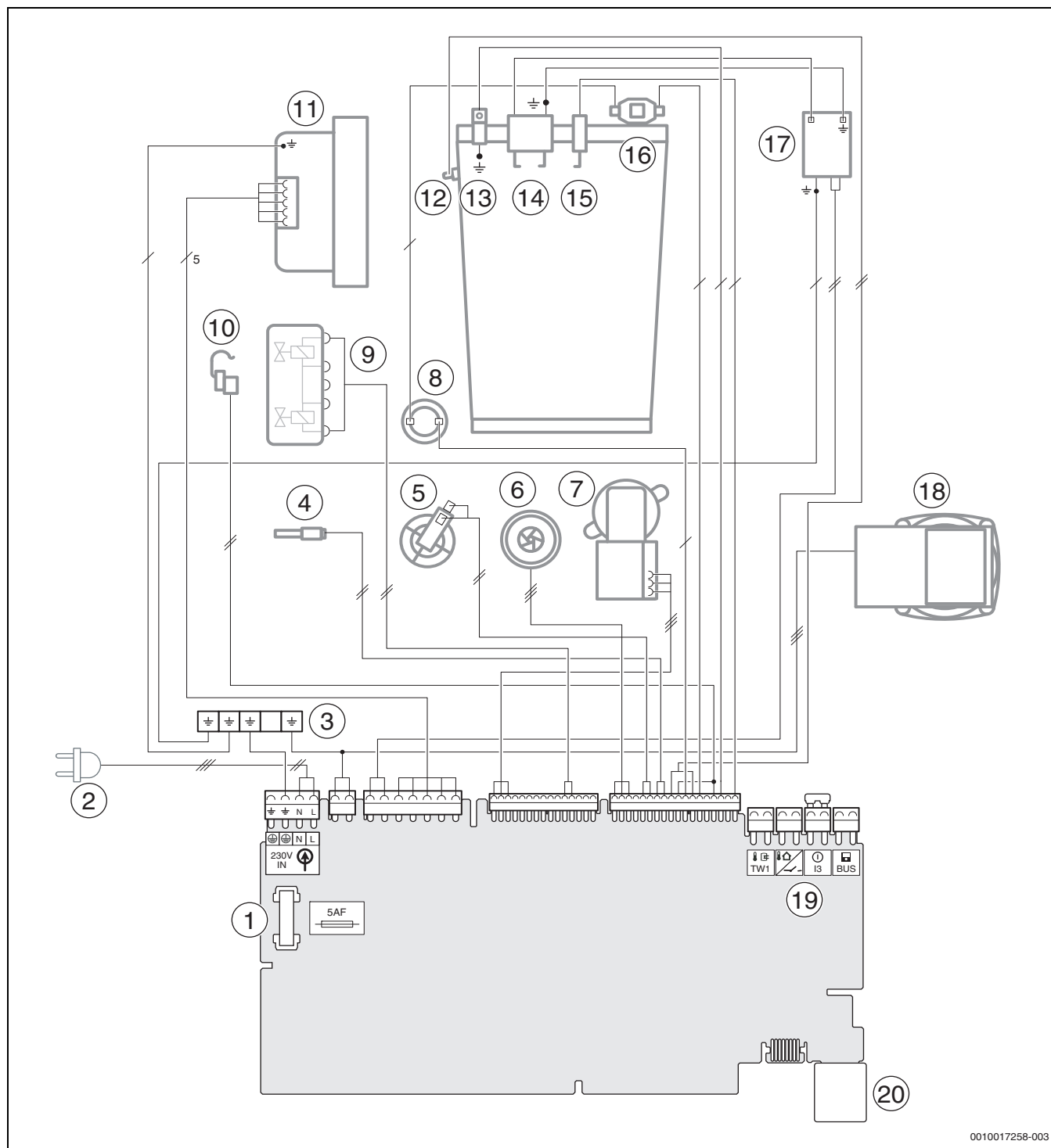
Afb. 80 Elektrische bedrading
