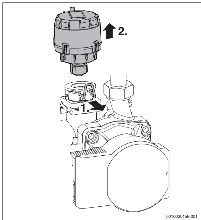
Afb. 72 Motor van de 3-wegklep demonteren
