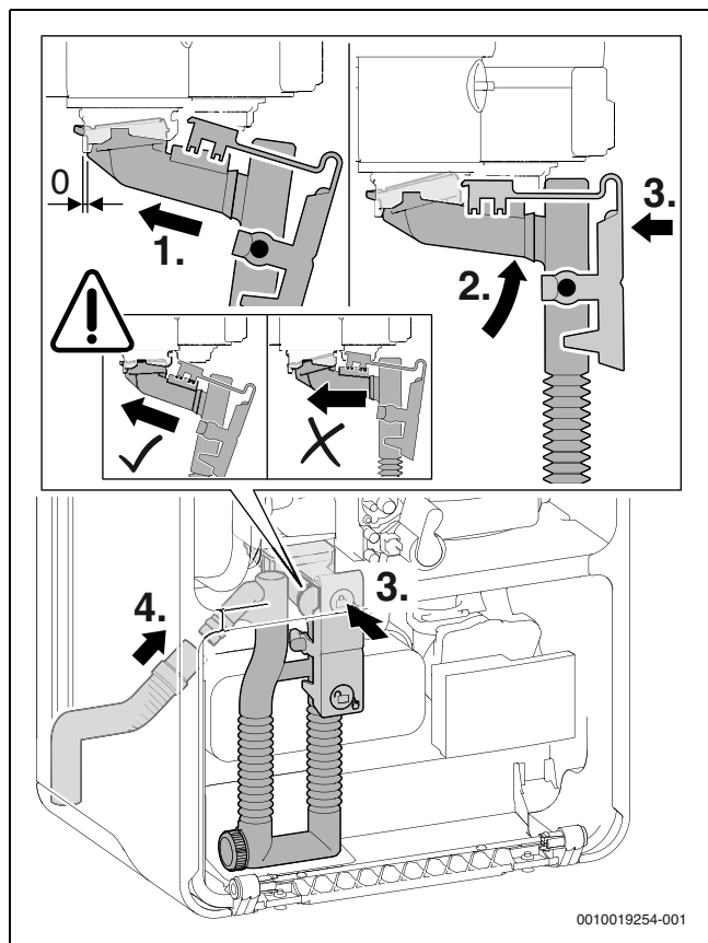
Afb. 64 Condenssifon plaatsen
