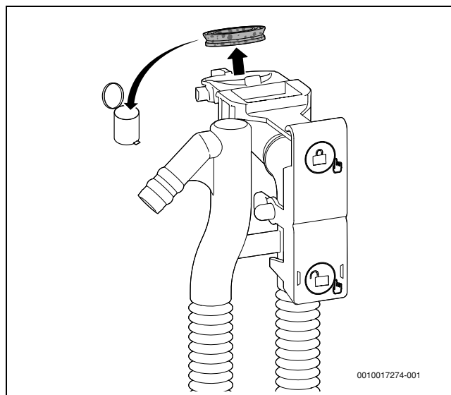
Afb. 61 Verwijder de dichting boven op de condenssifon
