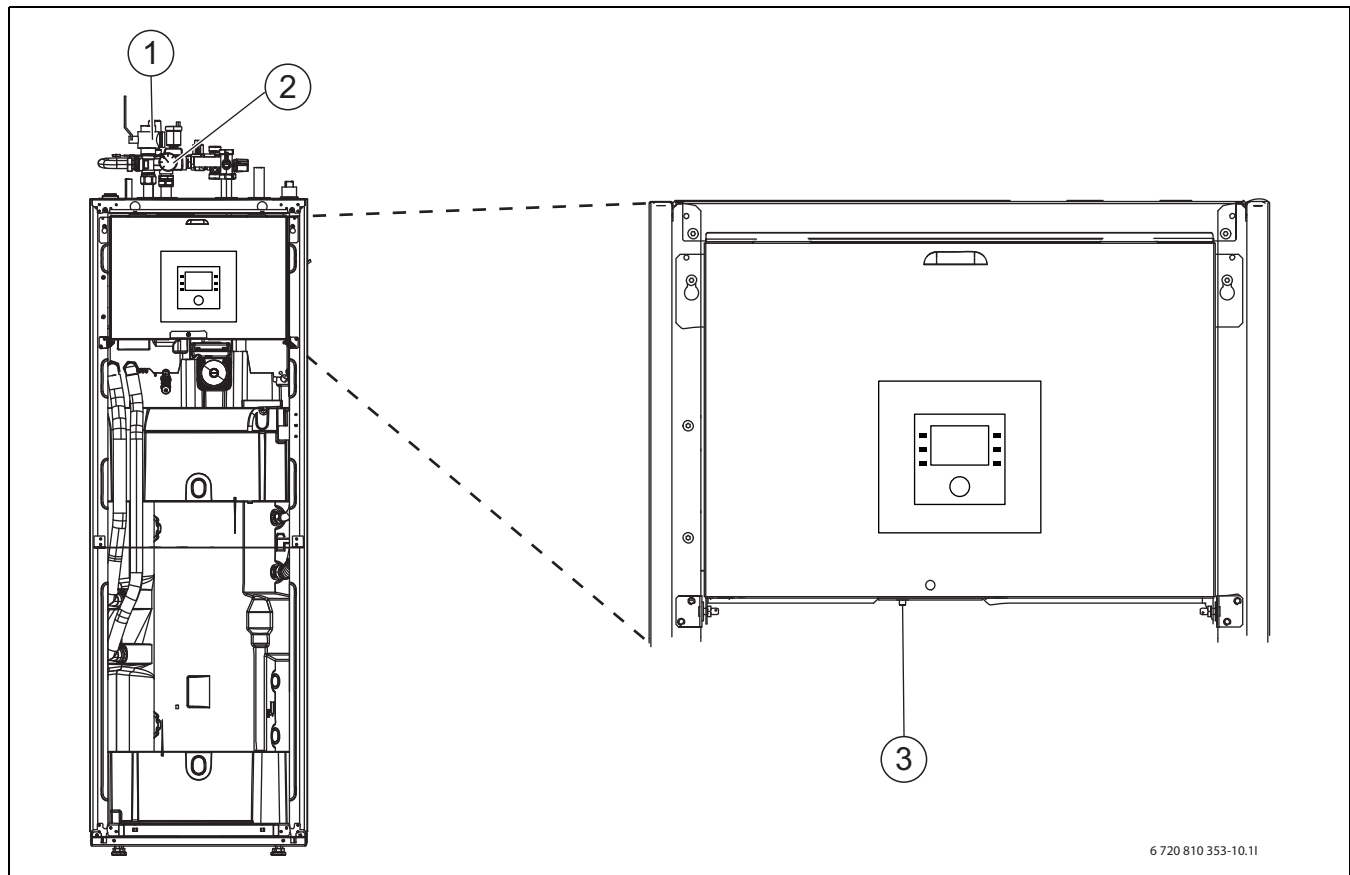
Afb. 6 Binneneenheid AWM/ AWMS
