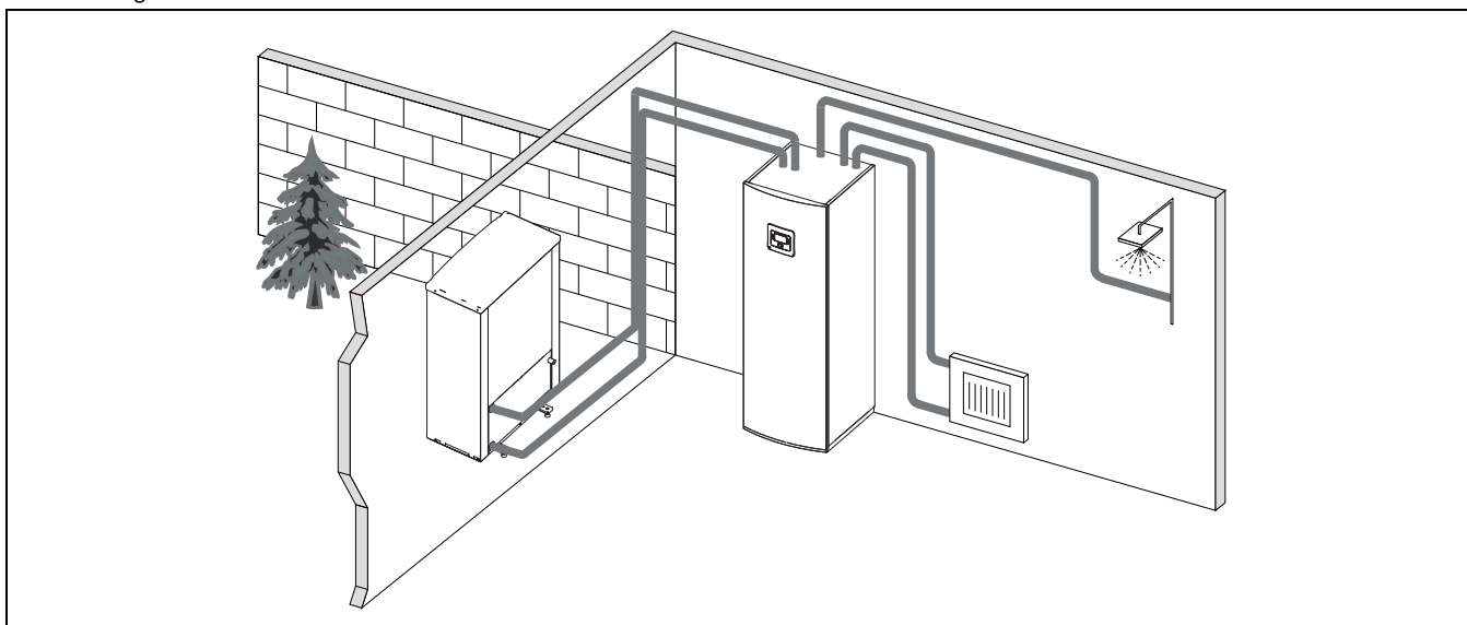
Afb. 3 Warmtepomp Compress 6000 AW, binneneenheid AWM/ AWMS met geïntegreerde warmwaterboiler en elektrische bijverwarming
