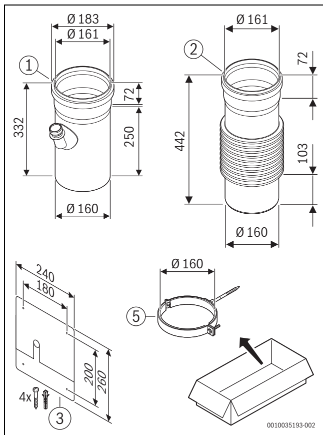
3 Ø 160: 7738113347
