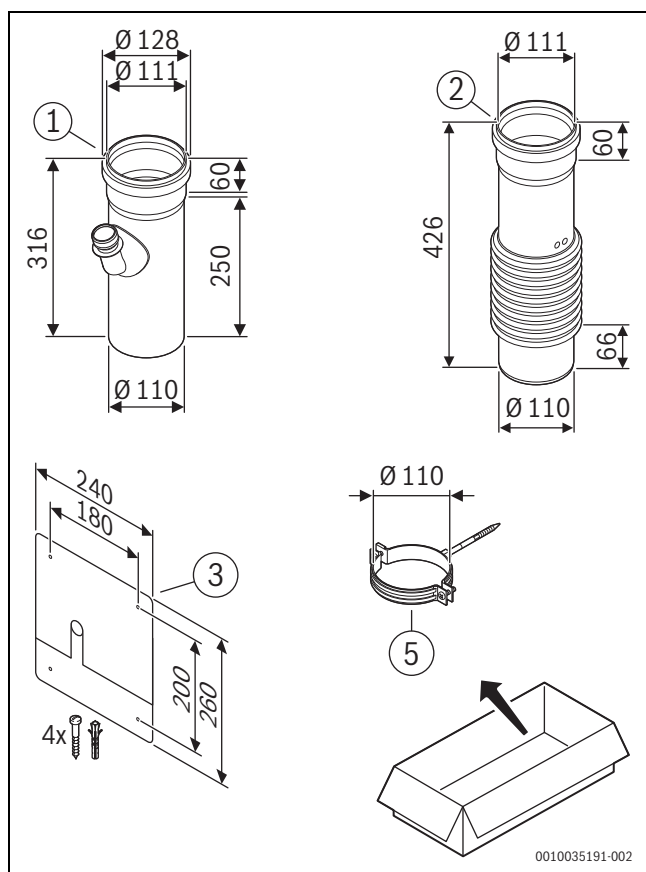
1 Ø 110: 7738113345
