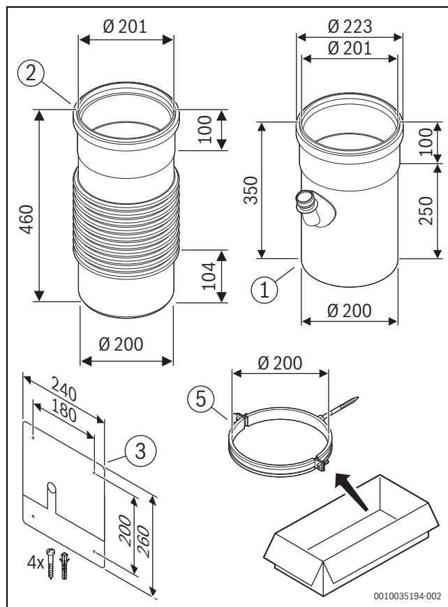
4 Ø 200: 7738113348
