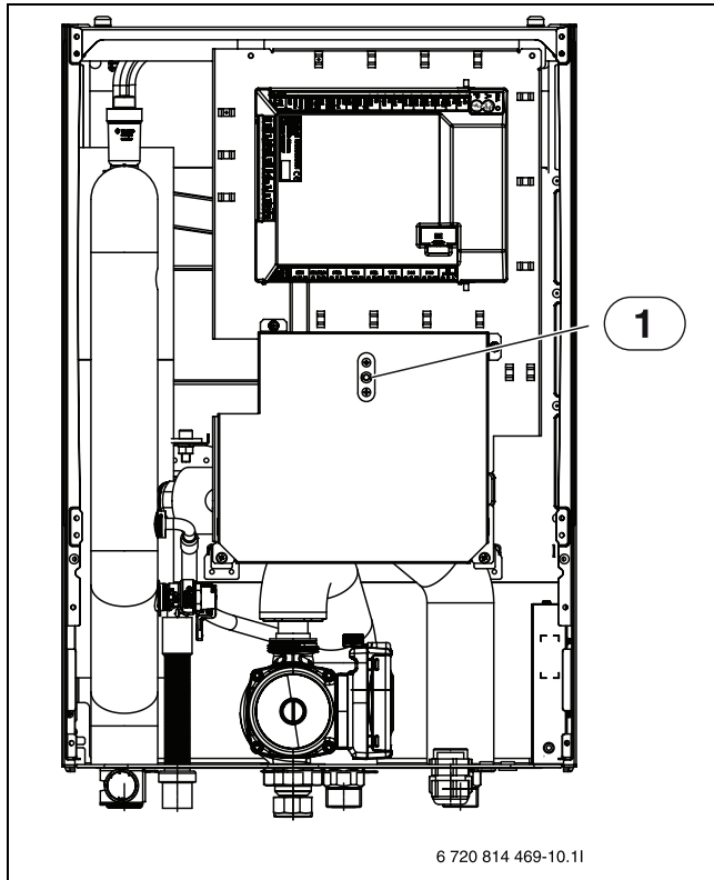
Afb. 6 Binneneenheid AWES
