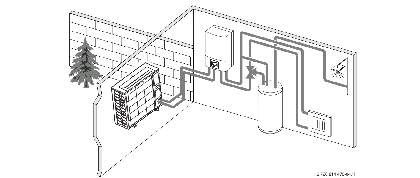
Afb. 2 Warmtepomp buiteneenheid, binneneenheid AWES met elektrische bijverwarming, externe boiler
