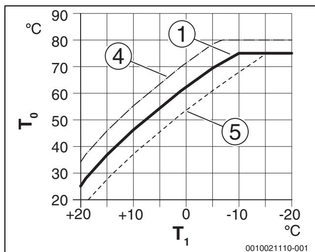
Afb. 5 Instelling van de stooklijn voor radiator Parallele verschuiving via Offset ruimtetemperatuur of gewenste kamertemperatuur
