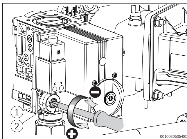
Afb. 13 O 2 -gehalte bij deellast instellen (keteltype 150 kW – 300 kW)
