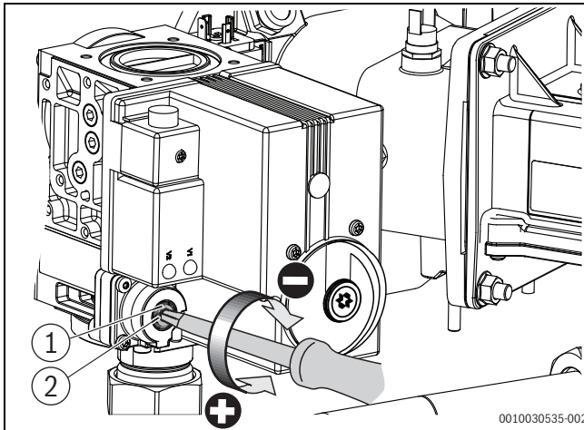
Afb. 6 O 2 -gehalte bij deellast instellen (keteltype 150 – 300 kW)
