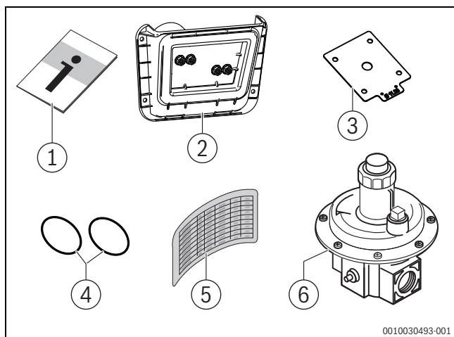
Afb. 3 Leveringsomvang ombouwset vloeibaar gas
