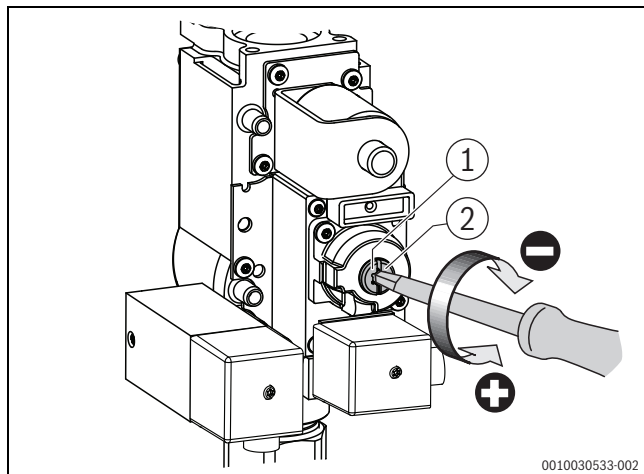
Afb. 12 O 2 -gehalte bij deellast instellen (keteltype 75 – 100 kW)
