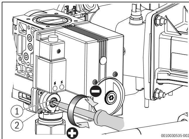
Afb. 10 O 2 -gehalte bij deellast instellen (keteltype 150 kW – 300 kW)
