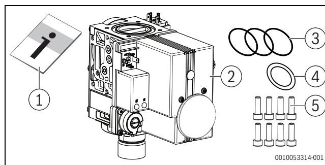
Afb. 2 Leveringsomvang reserve-gasblok 150 kW – 300 kW
