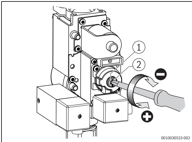
Afb. 5 O 2 -gehalte bij deellast instellen (keteltype 75 – 100 kW)
