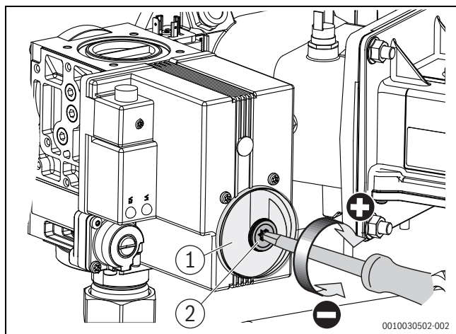
Afb. 8 O 2 -gehalte bij vollast instellen (keteltype 150 kW – 300 kW)
