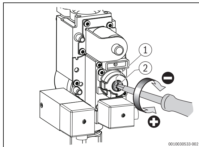
Afb. 9 O 2 -gehalte bij deellast instellen (keteltype 75 – 100 kW)
