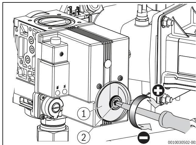
Afb. 4 O 2 -gehalte bij vollast instellen (keteltype 150 kW – 300 kW)
