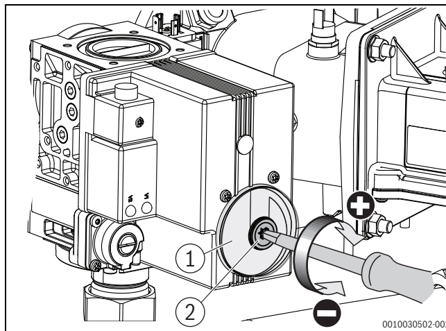
Afb. 11 O 2 -gehalte bij vollast instellen (keteltype 150 kW – 300 kW)
