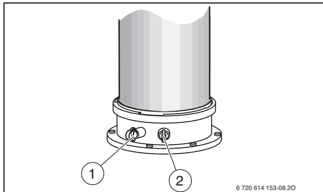
Afb. 39 Rookgasmeetpunt en verbrandingsluchtmeetpunt
