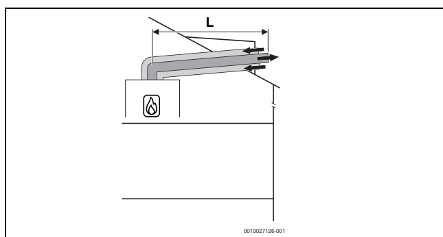
Afb. 5 Horizontaal concentrisch luchttoevoer-/rookgasafvoersysteem conform C 13x op het dak
