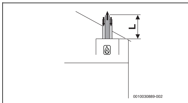
Afb. 8 Verticaal concentrisch luchttoevoer/rookgasafvoersysteem conform C 33x
