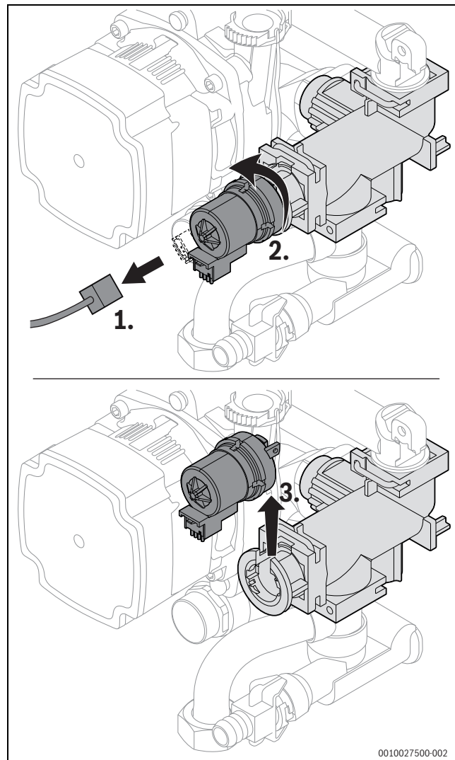
Afb. 62 Motor van de 3-wegklep uitbouwen (variant zonder schroeven)
