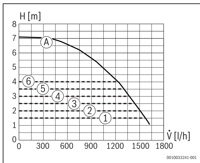
Afb. 66 Pompkarakteristieken en pompcurven
