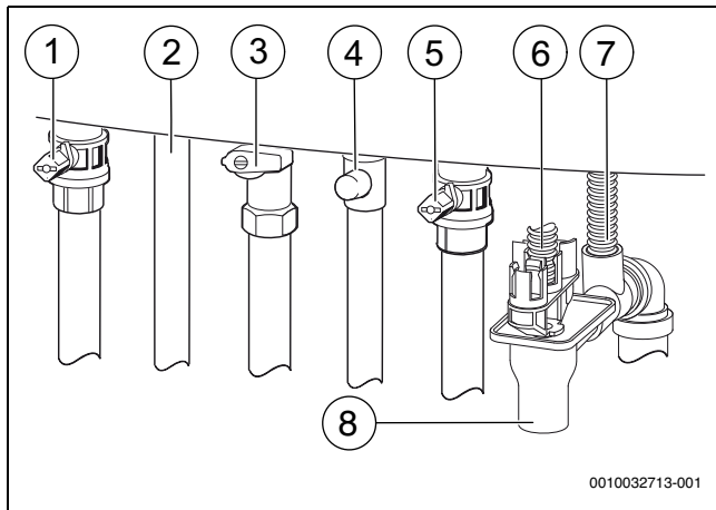
Afb. 30 Gas- en waterzijdige aansluitingen (toebehoren)
