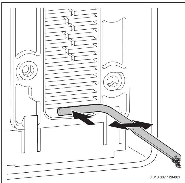
Afb. 54 Condensopvang reinigen
