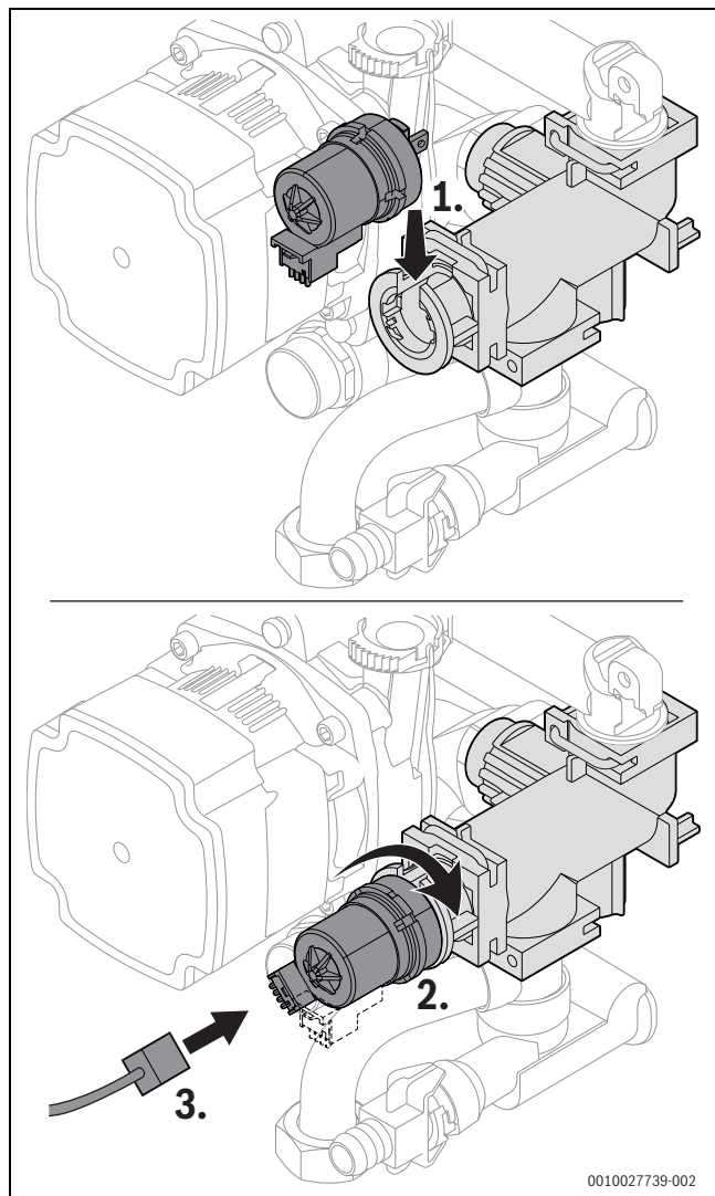
Afb. 63 Motor van de 3-wegklep inbouwen (variant zonder schroeven)
