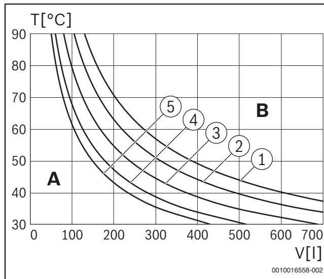
Afb. 21 Curve van het expansievat
