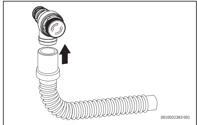
Afb. 24 Slang op veiligheidsventiel (verwarming) monteren
