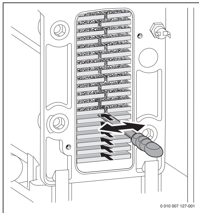
Afb. 51 Reinigingsgereedschap
