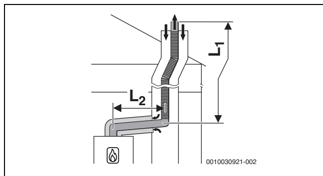
Afb. 14 Flexibel rookgasafvoertraject conform C 93x in een schacht en concentrisch luchttoevoer/rookgasafvoersysteem in opstellingsruimte
