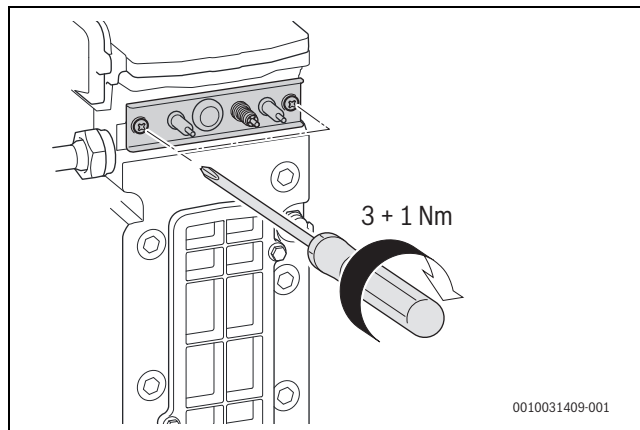
Afb. 40 Elektrodenset inbouwen
