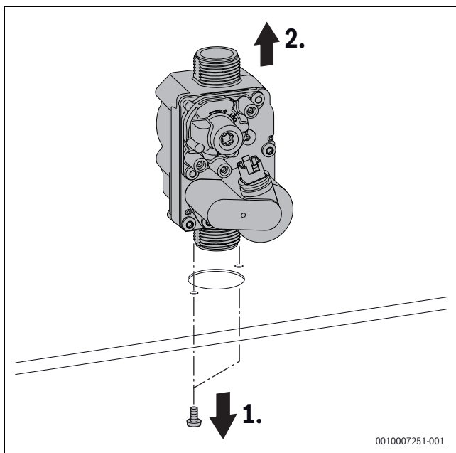
Afb. 61 Gasblok demonteren
