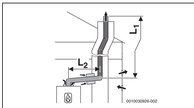
Afb. 16 Flexibele rookgasafvoer door de schacht conform B 23p /B 53p met open luchttoevoer aan toestel en concentrisch verbindingstuk tussen opstellingsruimte en schacht
