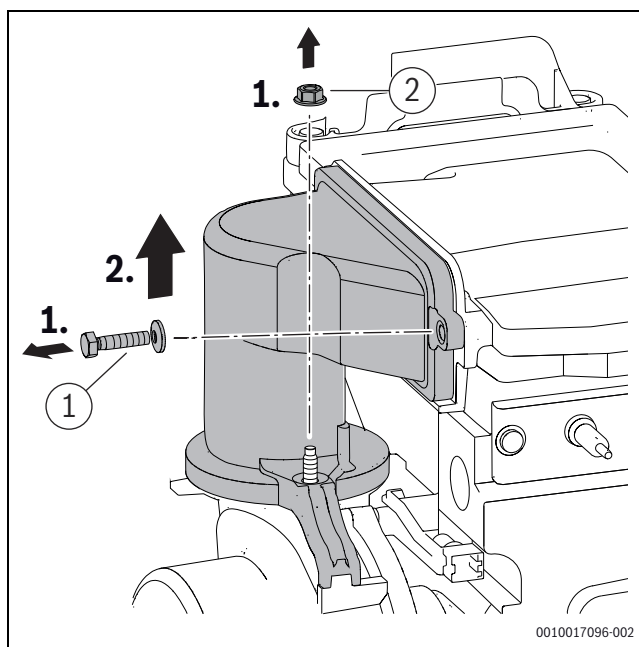
Afb. 45 Menginrichting demonteren
