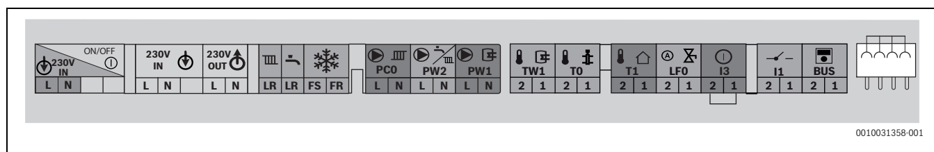
Afb. 33 Klemmenstrook voor extern toebehoren
