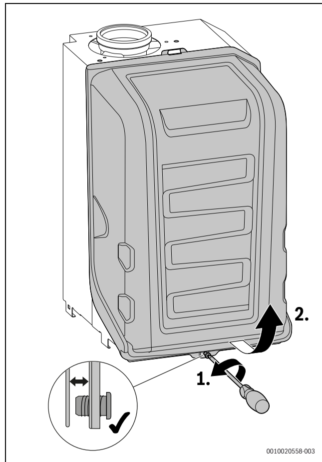
Afb. 36 Branderap verwijderen
