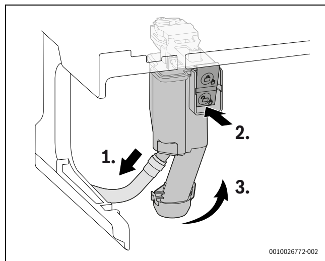
Afb. 55 Condenssifon demonteren
