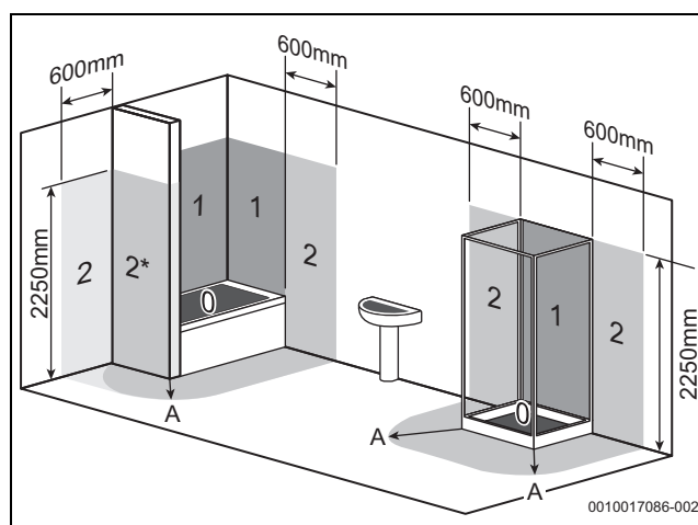
Afb. 18 Veiligheidszone (voorbeeldweergave)
