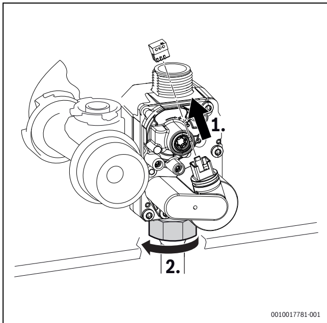
Afb. 60 Stekker lostrekken en wartelmoer losmaken
