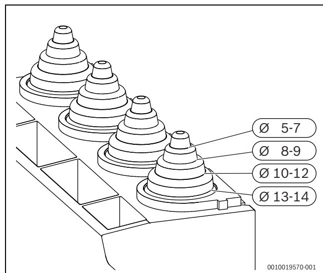
Afb. 32 Aanpassen trekontlasting aan de kabeldiameter
