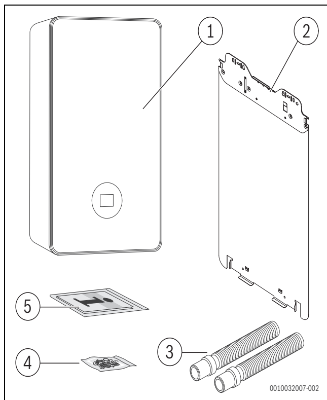
Afb. 1 Leveringsomvang
