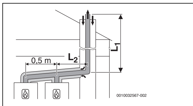
Afb. 17 Cascade met 2 toestellen: star rookgasafvoertraject conform C 93x in een schacht en concentrisch luchttoevoer/rookgasafvoersysteem in opstellingsruimte
