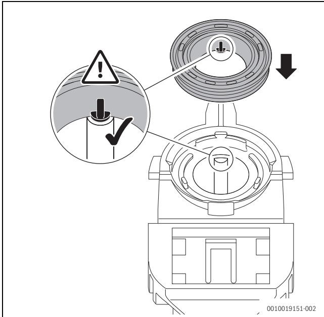
Afb. 56 Dichting correct op de condenssifon plaatsen
