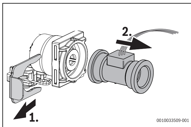
Afb. 48 Turbine op koudwaterbuis demonteren
