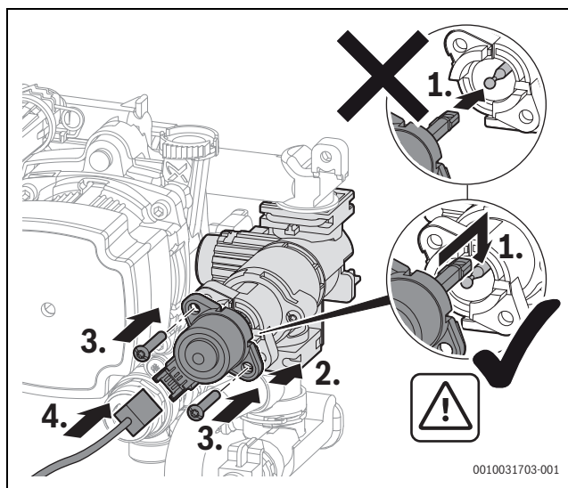
Afb. 65 Motor van de 3-wegklep inbouwen (variant met schroeven)
