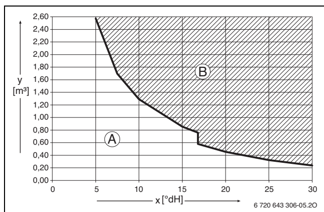
Afb. 19 Eisen aan het vul- en bijvulwater in °dH voor toestellen < 50 kW
