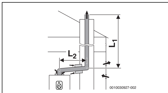
Afb. 15 Starre rookgasafvoer door de schacht conform B 23p /B 53p met open luchttoevoer aan toestel en concentrisch verbindingstuk tussen opstellingsruimte en schacht
