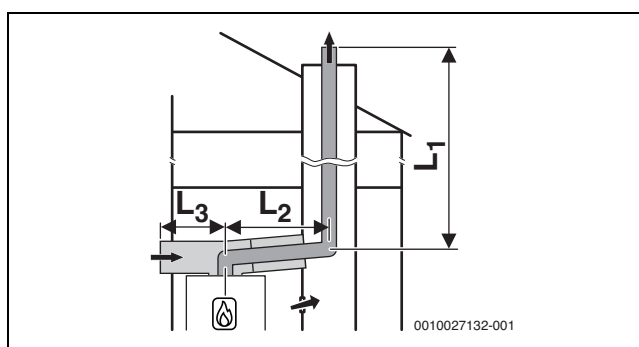
Afb. 10 Star rookgasafvoertraject conform C 53x in schacht en luchttoevoer/rookgasafvoersysteem met separate luchttoevoer en concentrische rookgasafvoer in opstellingsruimte
