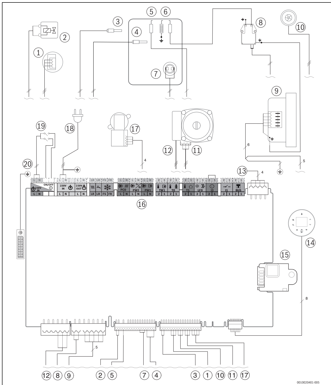
Afb. 67 Elektrische bedrading
