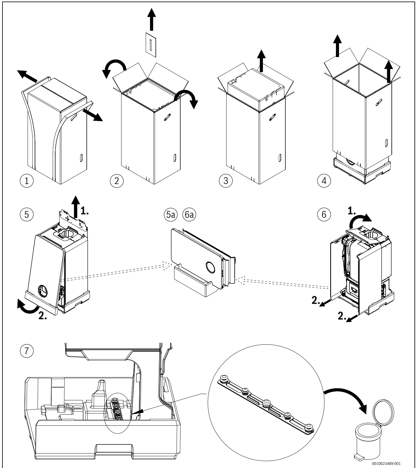
Afb. 22 Uitpakinstructies
