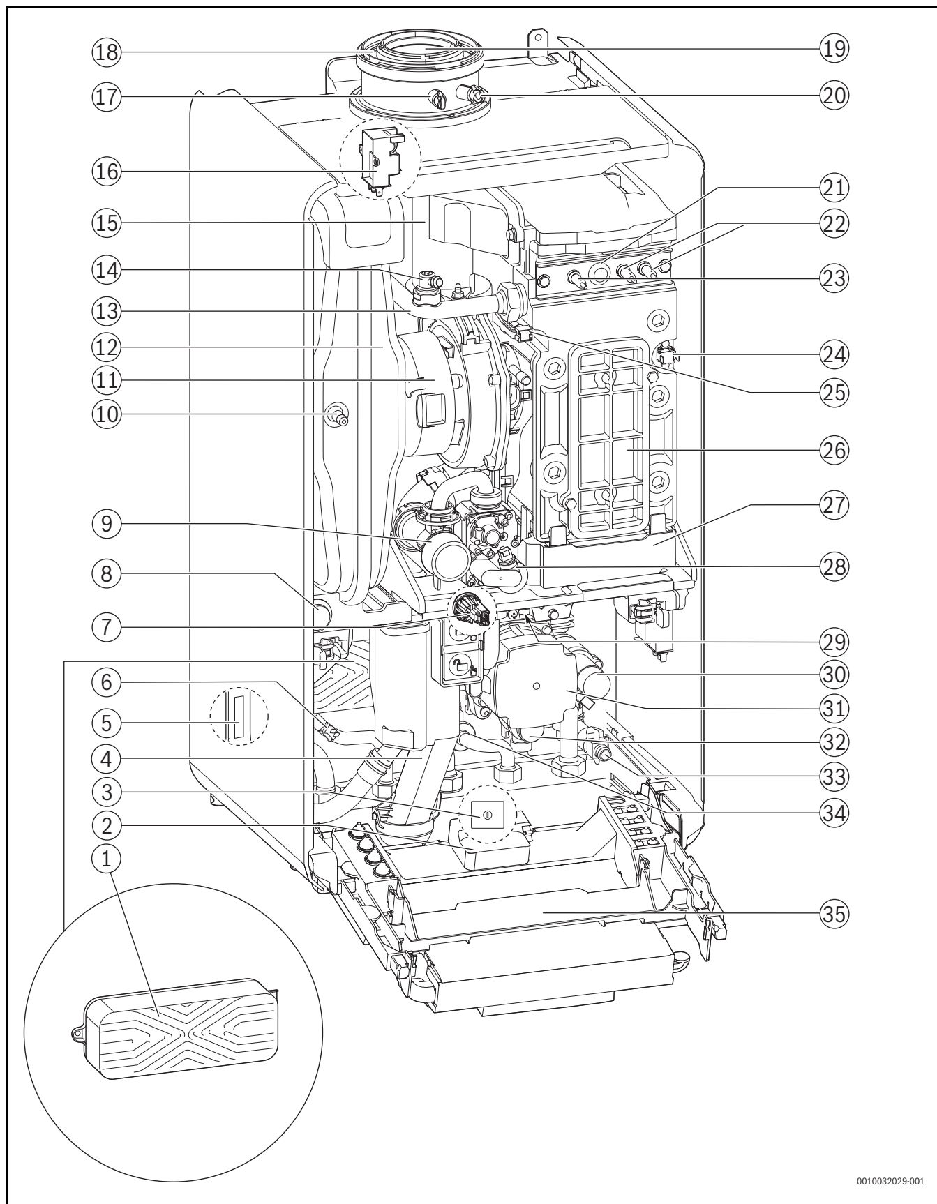
Afb. 2 Productoverzicht
