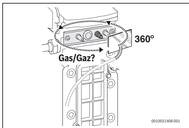
Afb. 41 Dichtheid controleren
