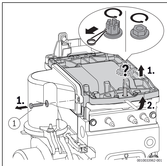
Afb. 42 Branderdekseel demonteren
