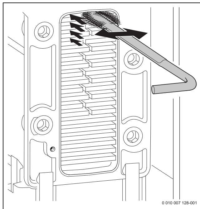
Afb. 52 Reinig het verwarmingslichaam met de borstel
