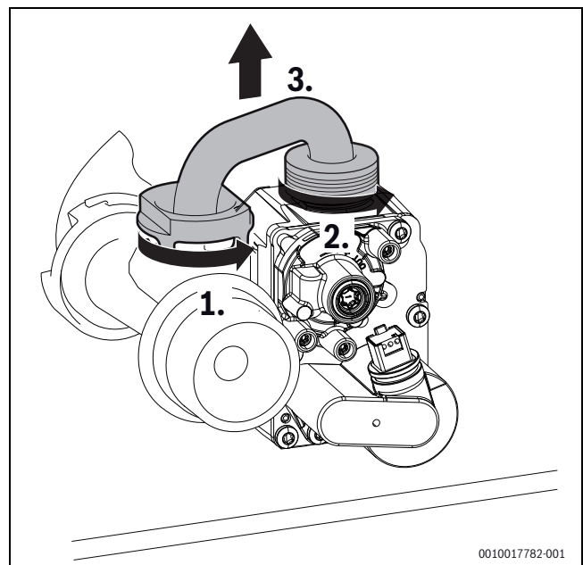
Afb. 59 Gasbuis demonteren
