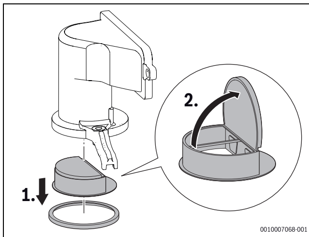
Afb. 46 Terugslagklep in de menginrichting
