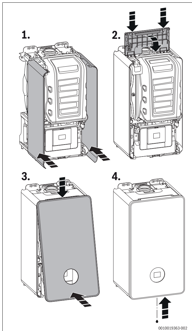
Afb. 34 Mantel monteren
