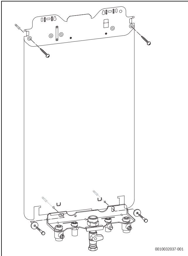
Afb. 23 Monteer de bevestigingsplaat en de montageplaat (toebehoren)
