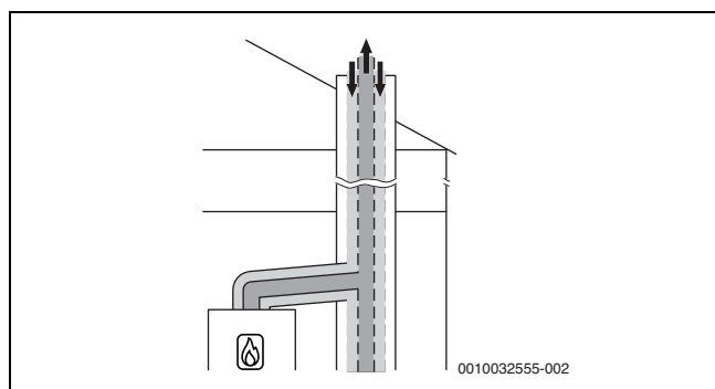
Afb. 9 Concentrisch luchttoevoer/rookgasafvoersysteem conform C 43x in opstellingsruimte
