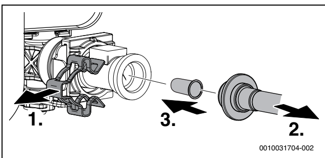
Afb. 47 Het filter uit de koudwaterbuis demonteren
