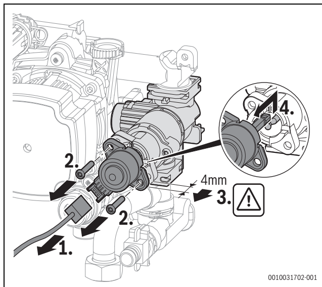
Afb. 64 Motor van de 3-wegklep uitbouwen (variant met schroeven)
