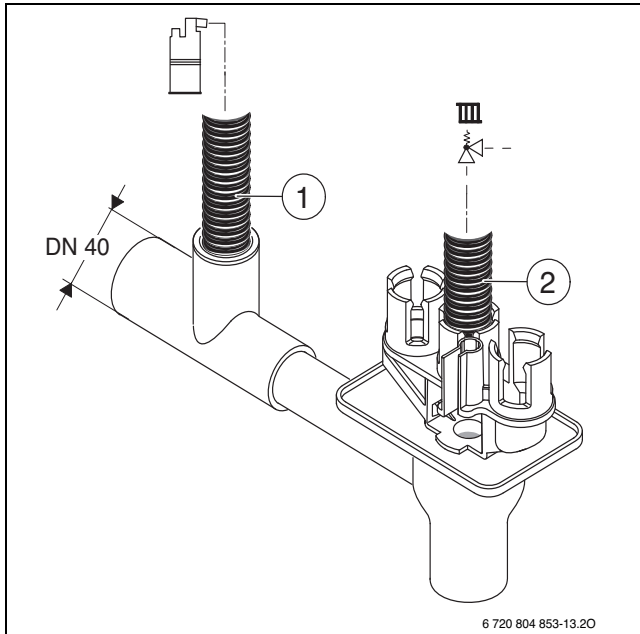
Afb. 26 Monteer de condensaat slang en de slang van het veiligheidsventiel op het sifon
