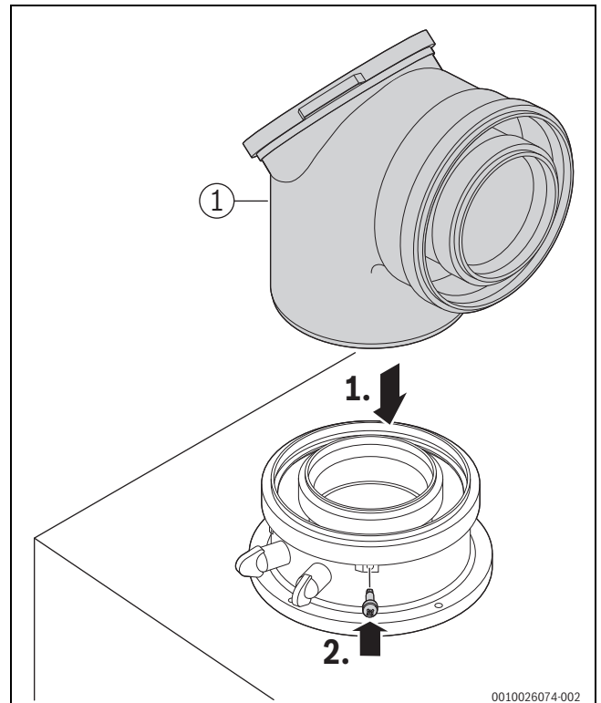
Afb. 29 Breng het rookgastoebehoren aan en borg met schroef
