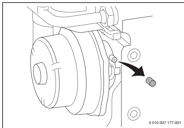
Afb. 49 Meetnippel op de menginrichting
