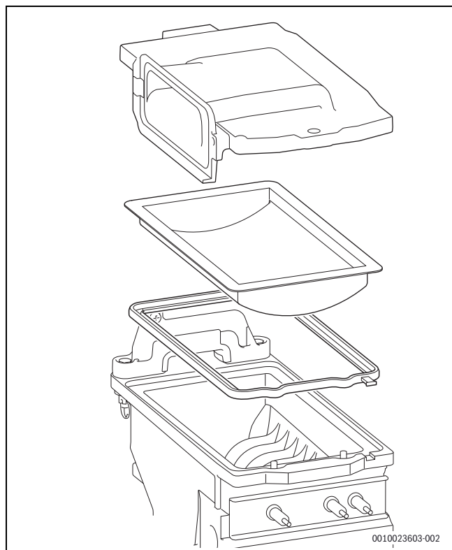
Afb. 43 Brander
