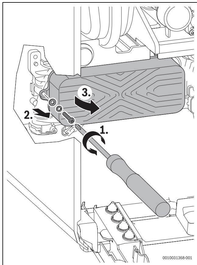
Afb. 50 Platenwarmtewisselaar demonteren
