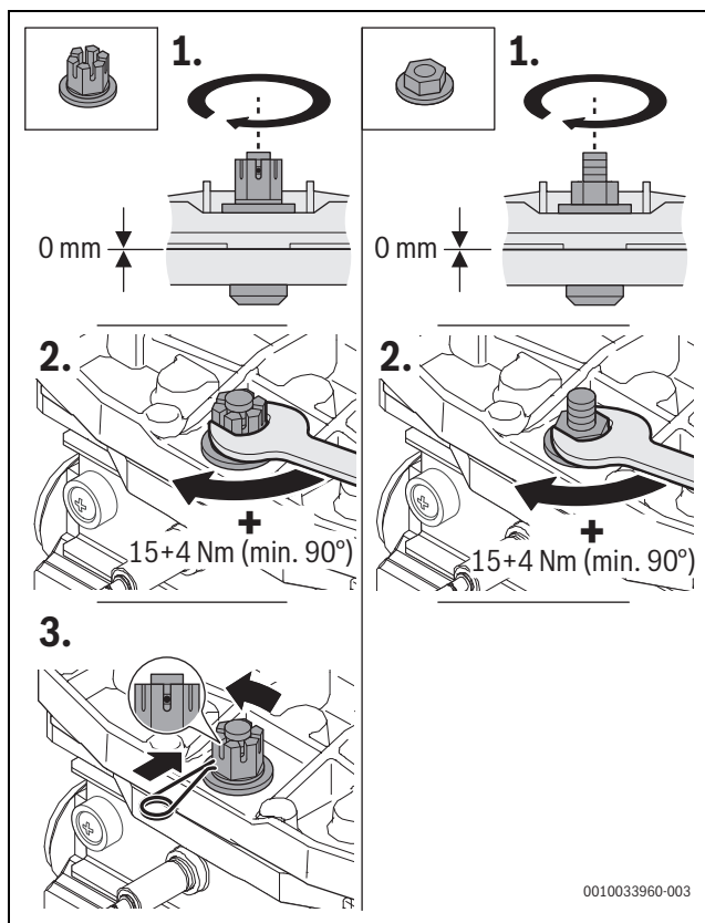
Afb. 44 Draai de moer op het branderdekseel vast
