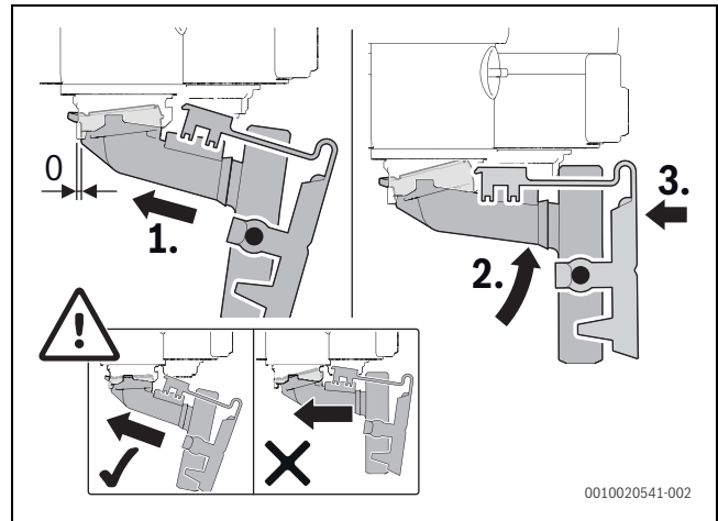
Afb. 58 Condenssifon inbouwen
