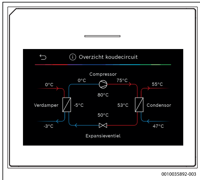
Afb. 10 Overzicht koelcircuit
