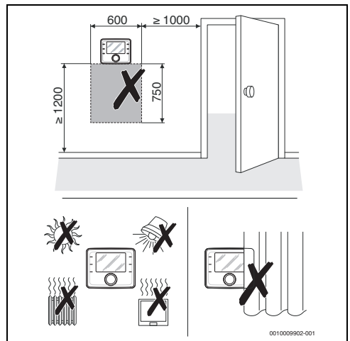
Afb. 5 Installatieplaats in de referentieruimte
