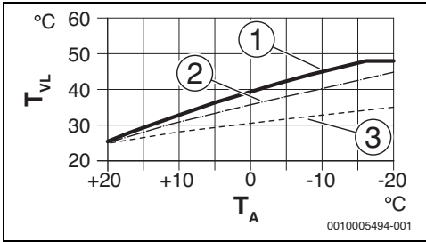
Afb. 16 Instelling van de stooklijn voor vloerverwarming Stijging via ontwerptemperatuur T_{AL} en minimale buitentemperatuur T_{A,min}
