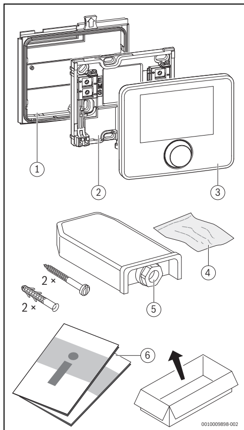
Afb. 3 Leveringsomvang
