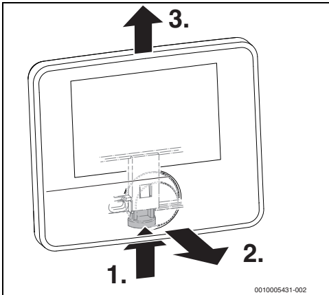
Afb. 9 Bedieningseenheid afnemen
