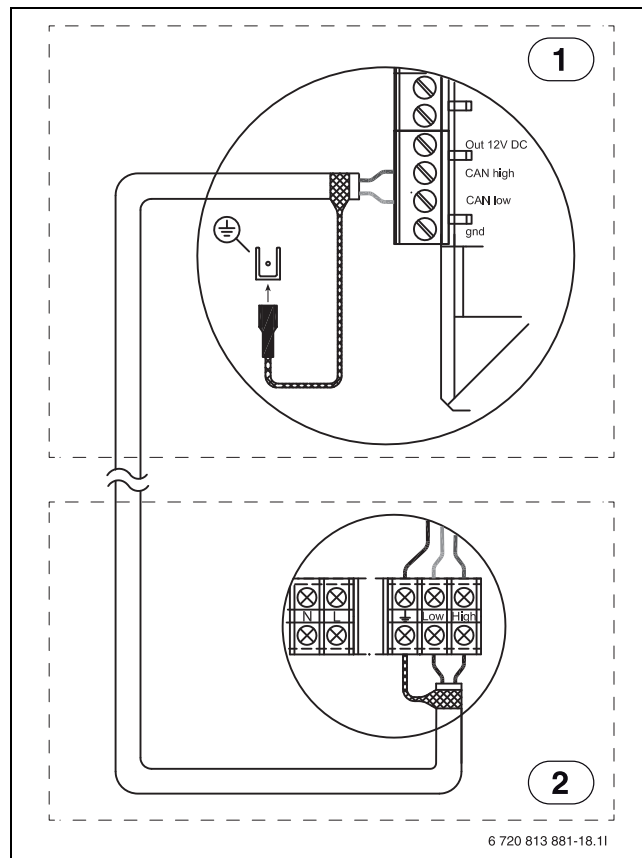
Afb. 11 CAN-BUS-verbinding
