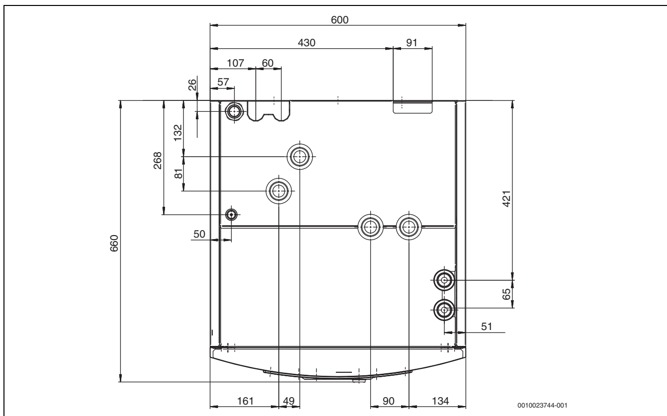
Afb. 5 Aansluitafmetingen, bovenaanzicht
