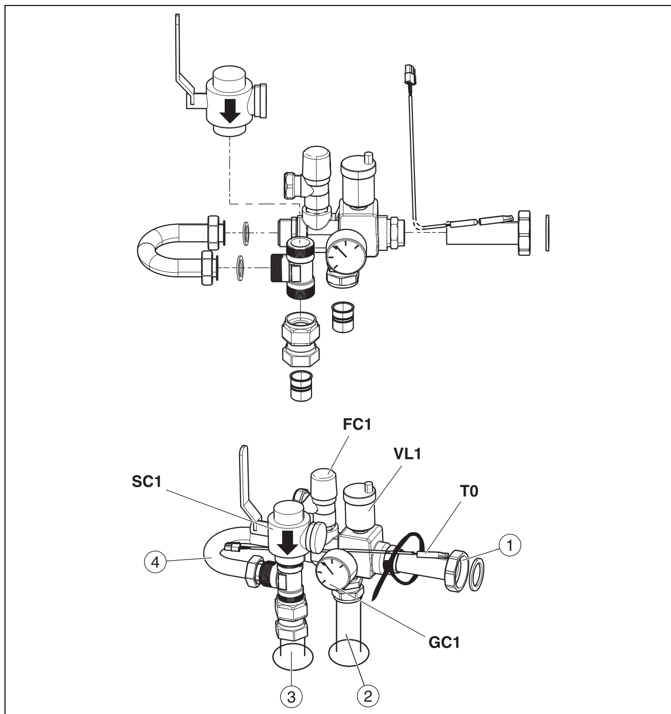
Afb. 8 Gemonteerde veiligheidsgroep, met bypass
