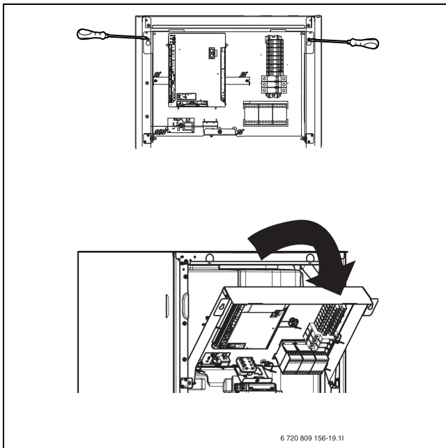
Afb. 20 Besturing
