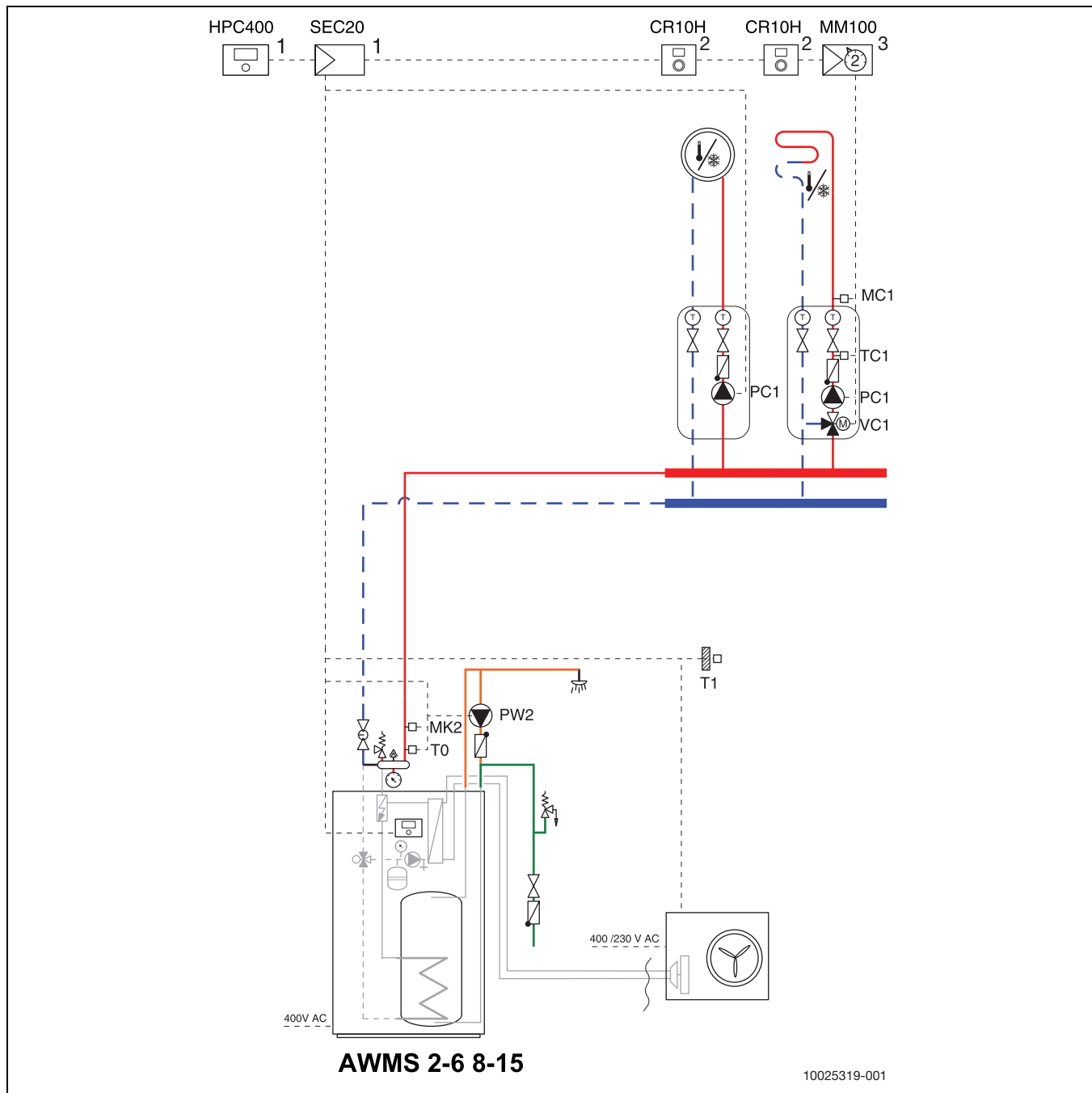
Afb. 27 Buiteneenheid met binneneenheid en twee verwarmingscircuits
