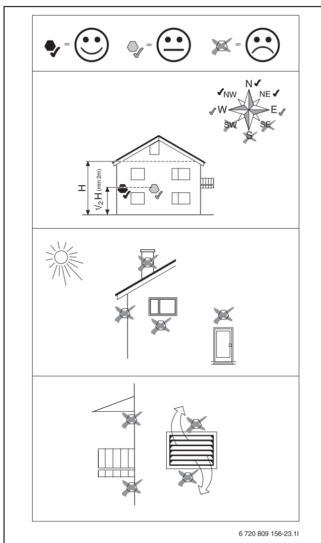
Afb. 13 Plaatsing van de buitentemperatuursensor
