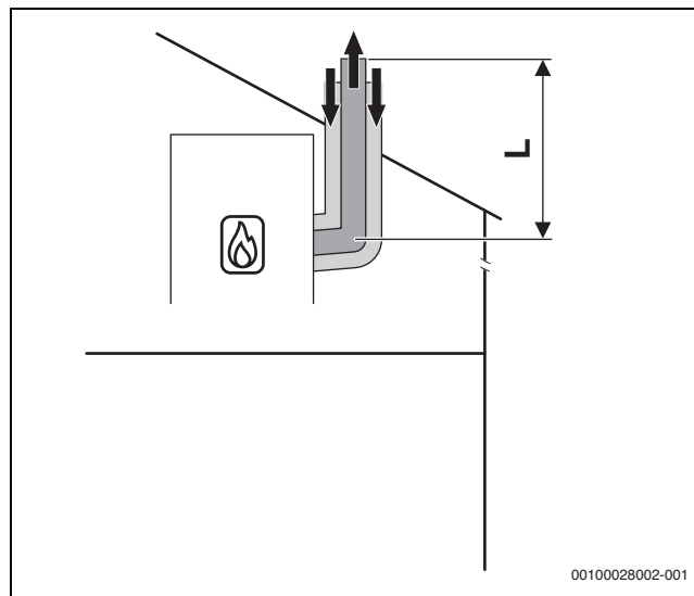
Afb. 8 Verticaal concentrisch luchttoevoer-/rookgasafvoersysteem conform C 33x
