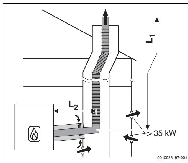
Afb. 20 Flexibel rookgasafvoer door de schacht B 33 met open luchttoevoer via het concentrisch luchttoevoer/rookgasafvoersysteem in opstellingsruimte
