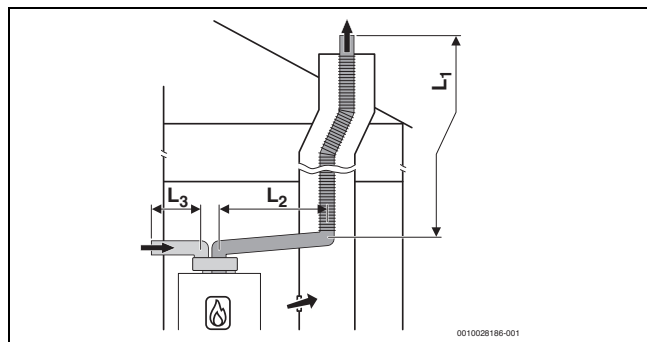
Afb. 12 Flexibel rookgasafvoertraject conform C 53 in schacht en luchttoevoer/rookgasafvoersysteem met gescheiden buizen voor luchttoevoer en rookgasafvoer in opstellingsruimte
