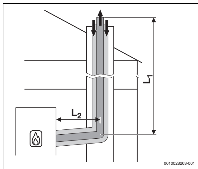
Afb. 7 Concentrisch luchttoevoer-/rookgasafvoersysteem conform C 33x in schacht
