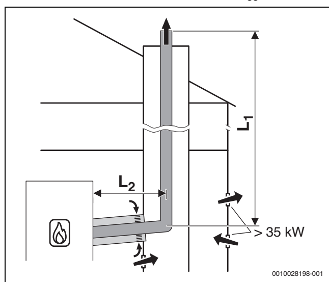
Afb. 19 Star rookgasafvoer door de schacht conform B 33 met open luchttoevoer via het concentrisch luchttoevoer/rookgasafvoersysteem in opstellingsruimte
