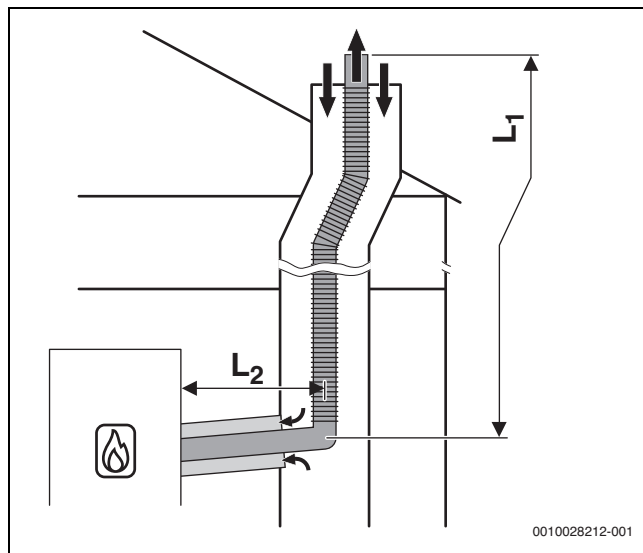
Afb. 15 Flexibel rookgasafvoertraject conform C 93x in een schacht en concentrisch luchttoevoer/rookgasafvoersysteem in opstellingsruimte
