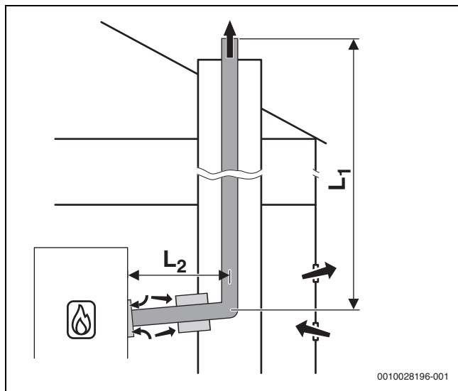
Afb. 17 Vaste rookgasafvoer door de schacht conform B 23p /B 53p met open systeem aan warmteproducent en concentrisch verbindingstuk tussen opstellingsruimte en schacht
