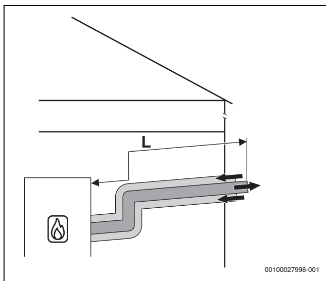
Afb. 4 Horizontaal concentrisch luchttoevoer-/rookgasafvoersysteem conform C 13x door de buitenwand
