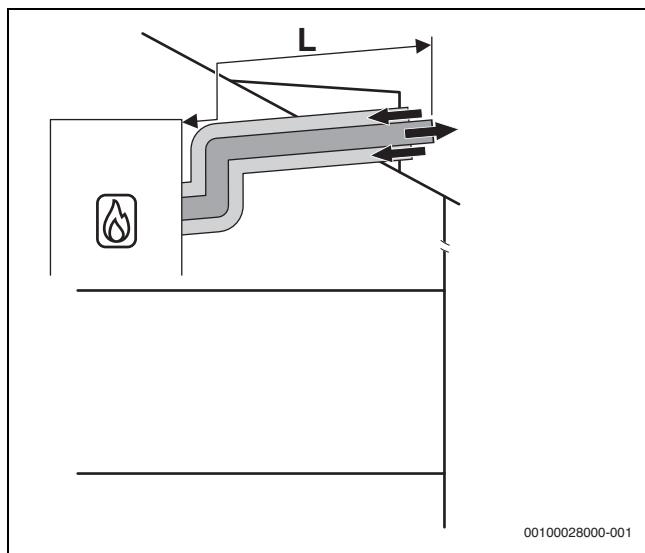
Afb. 3 Horizontaal concentrisch luchttoevoer-/rookgasafvoersysteem conform C 13x op het dak
