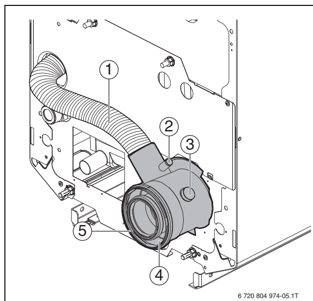
Afb. 16 Aansluitsteun voor luchttoevoer en rookgasafvoer monteren
