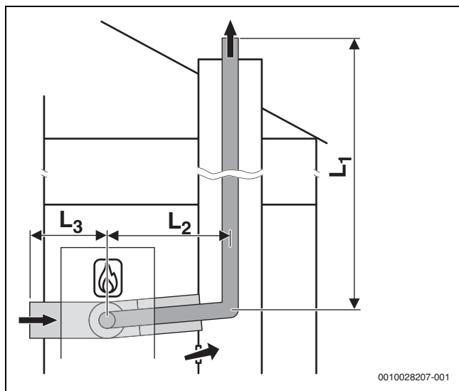
Afb. 9 Star rookgasafvoertraject conform C 53x in schacht en luchttoevoer/rookgasafvoersysteem met separate luchttoevoer en concentrische rookgasafvoer in opstellingsruimte
