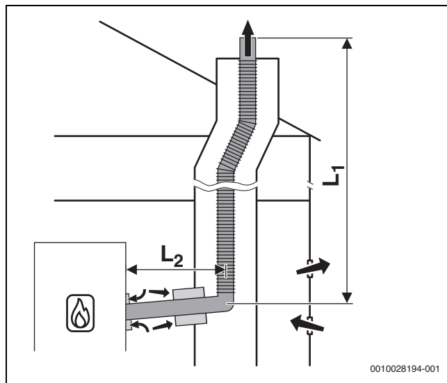
Afb. 18 Flexibele rookgasafvoer door de schacht conform B 23p /B 53p met open systeem aan warmteproducent en concentrisch verbindingstuk tussen opstellingsruimte en schacht
