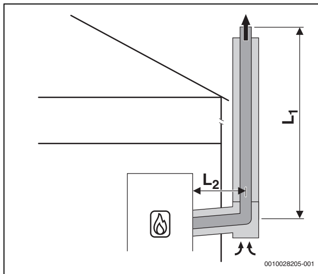
Afb. 13 Concentrisch luchttoevoer/rookgasafvoersysteem conform C 53x op de buitenmuur
