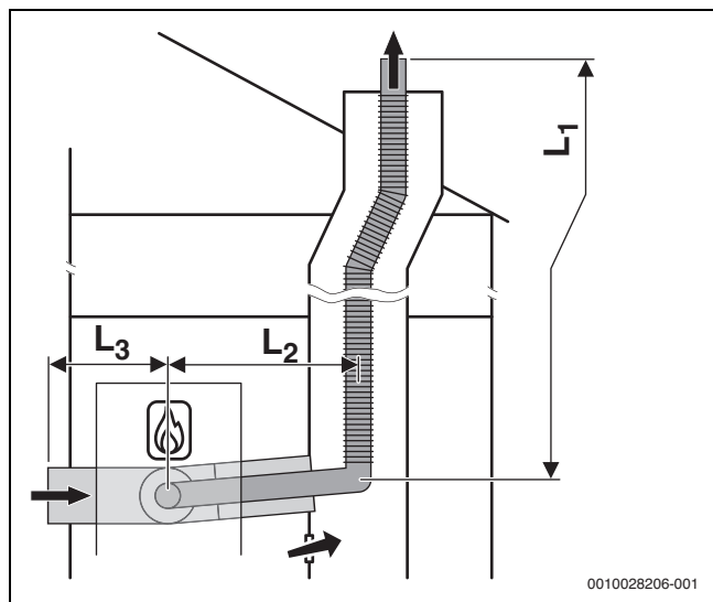
Afb. 11 Flexibel rookgasafvoertraject conform C 53x in schacht en luchttoevoer/rookgasafvoersysteem met separate luchttoevoer en concentrische rookgasafvoer in opstellingsruimte
