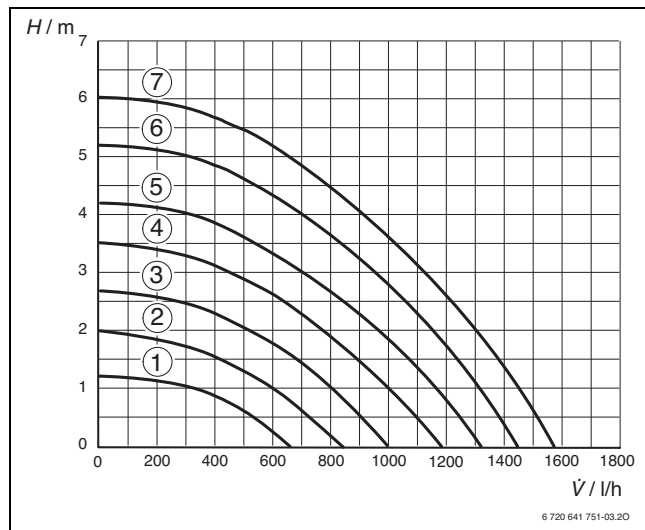
Afb. 32 Pompcurven
