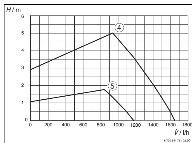
Afb. 31 Proportionele druk
