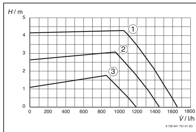
Afb. 30 Constante druk
