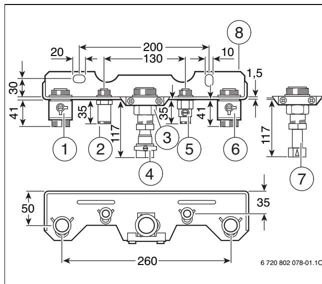
Afb. 6 Voorbeeld: montageaansluitplaat
