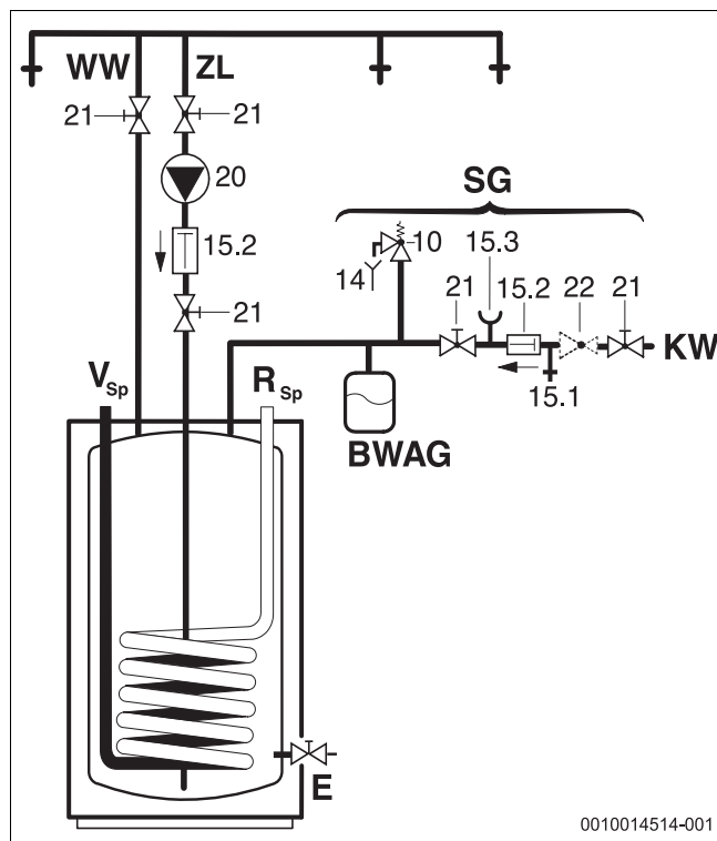
Afb. 9 Aansluitschema drinkwaterzijde
