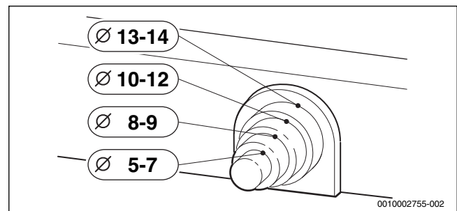
Afb. 29 Aanpassen trekontlasting aan de kabeldiameter
