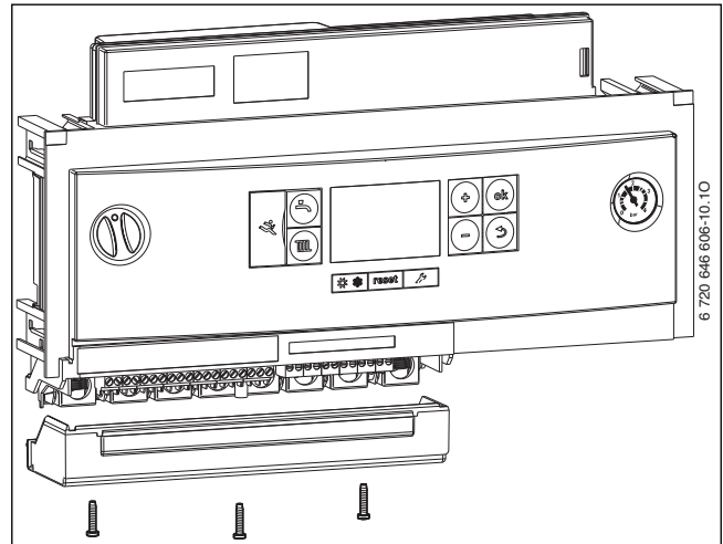
Afb. 28 Verwijderen afdekking
