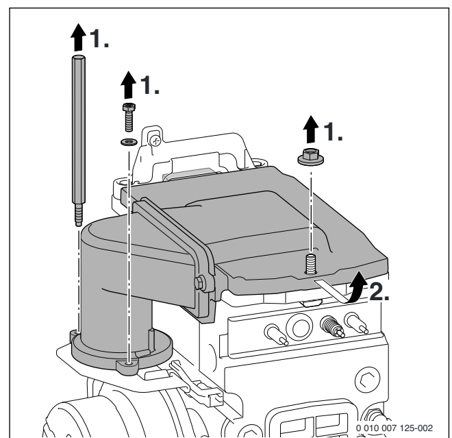
Afb. 49 Branderdeksel losmaken
