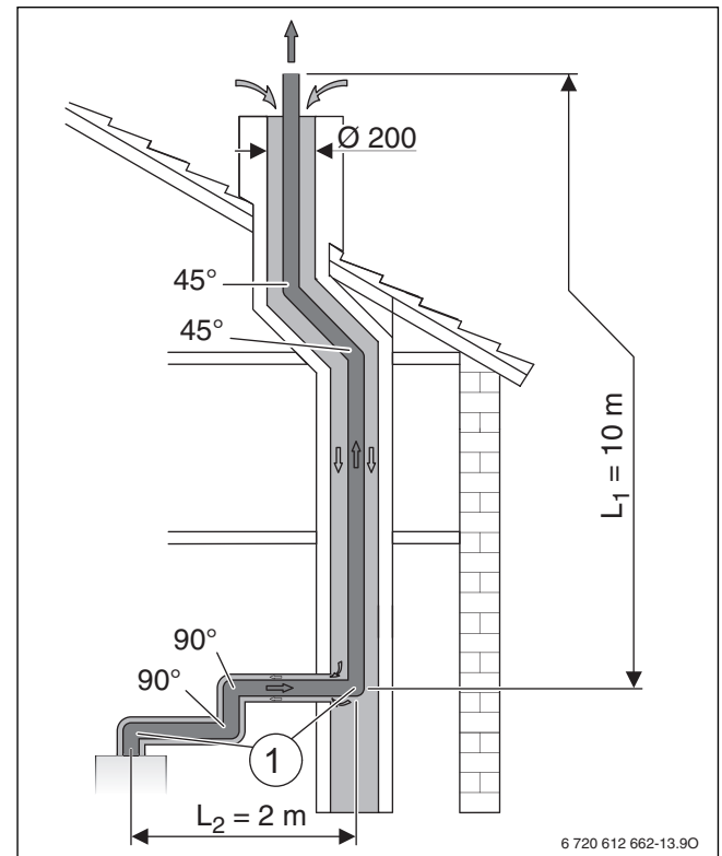
Afb. 17 Inbouwsituatie van een rookgasafvoersysteem in een schacht conform C_{93}
