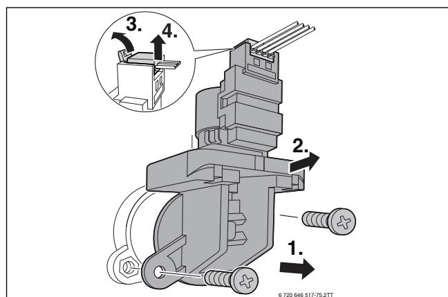
Afb. 65 3-wegklep demonteren
