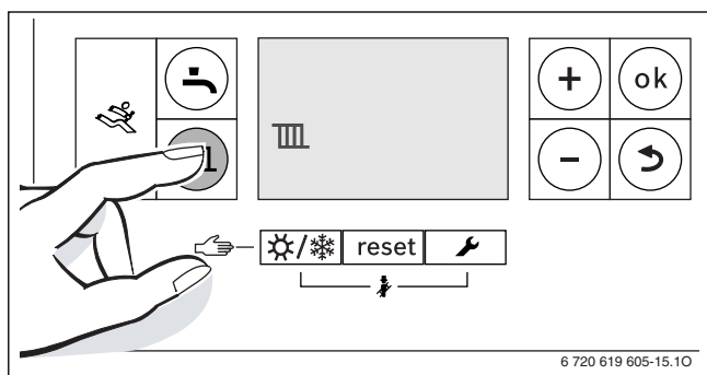
Afb. 31 Weergave cv-bedrijf
