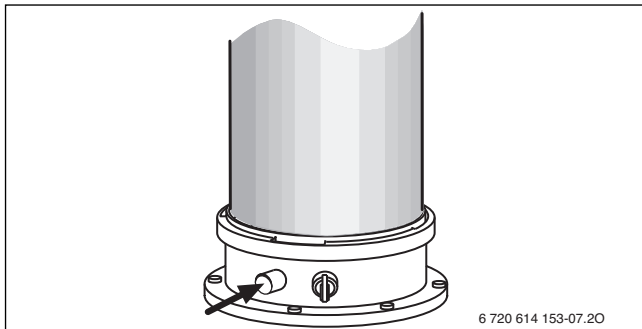
Afb. 43 Rookgasmeetpunt
