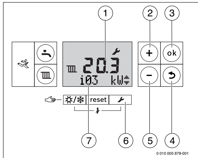
Afb. 42 Overzicht bedieningselementen
