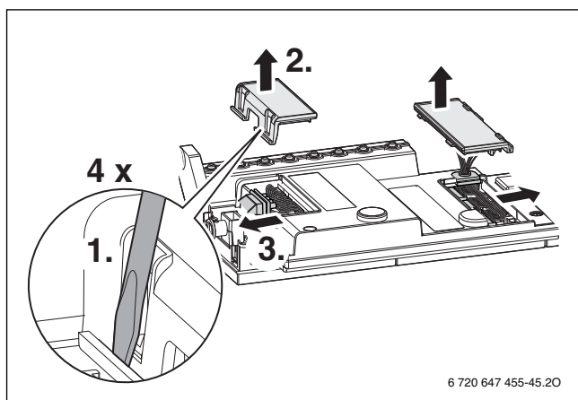
Afb. 73 Verwijderen afdekking
