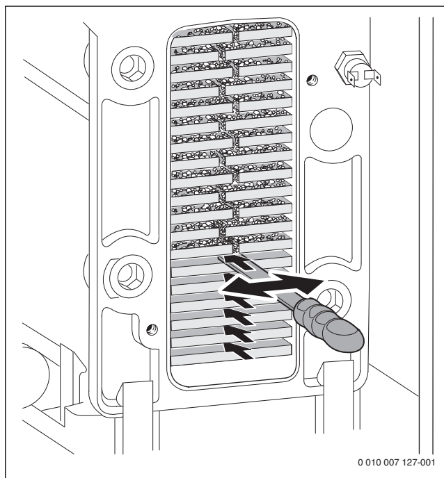
Afb. 53 Reinigingsgereedschap
