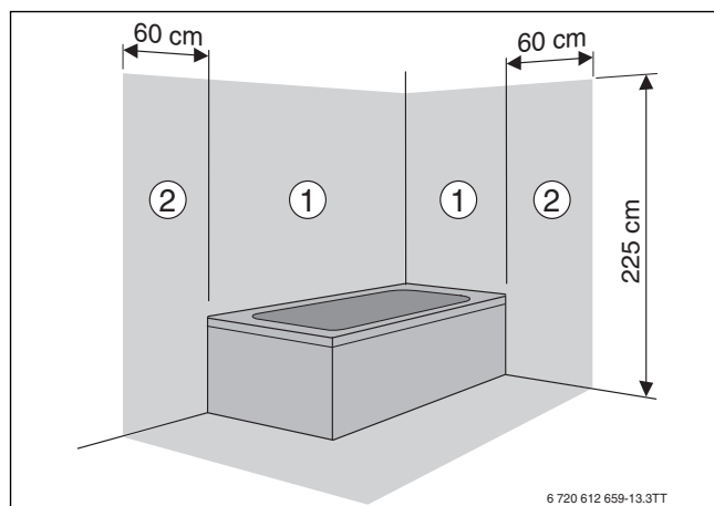
Afb. 27 Veiligheidszones
