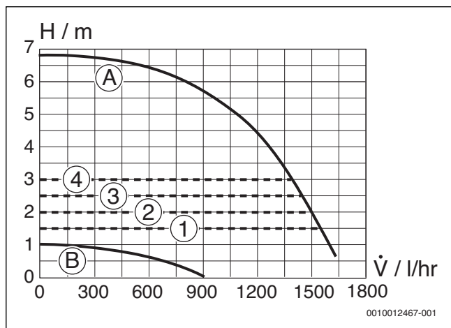
Afb. 79 Pompkarakteristieken en pompcurven
