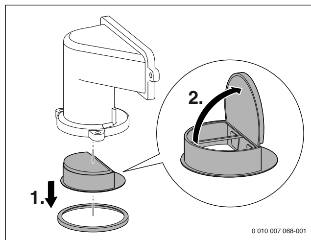
Afb. 59 Terugslagklep in de menginrichting
