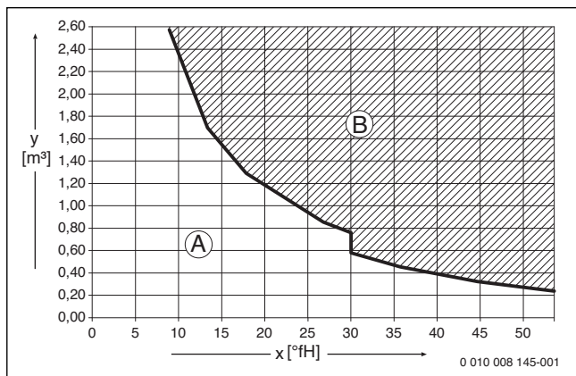
Afb. 19 Eisen aan het vul- en bijvulwater in °FH voor toestellen < 50 kW
