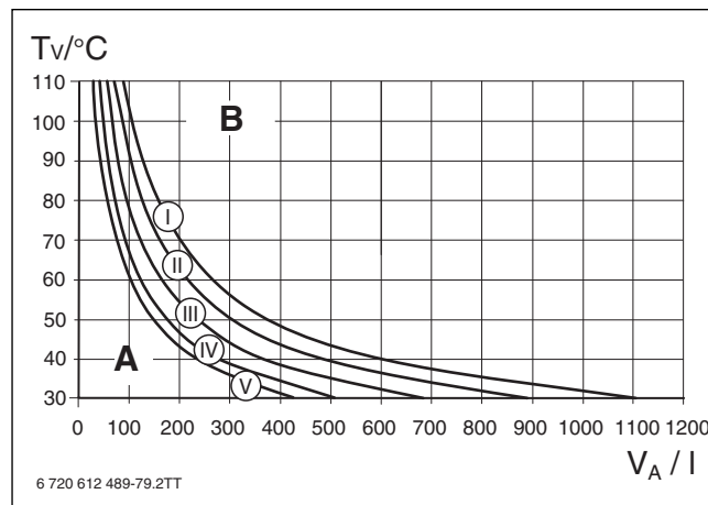
Afb. 20 Karakteristiek van het expansievat
