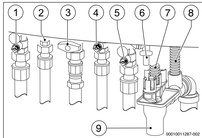
Afb. 26 Gas- en waterzijdige aansluitingen (toebehoren)
