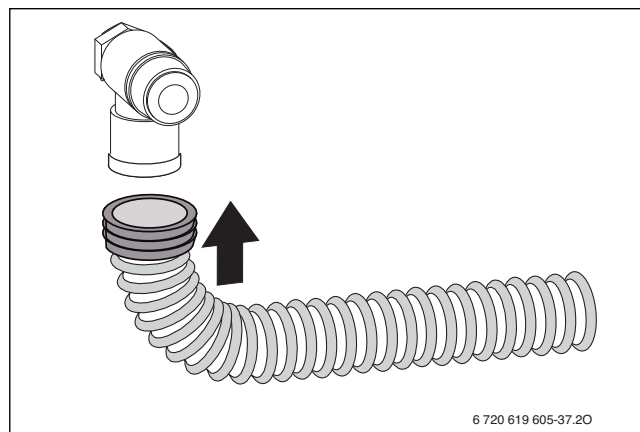
Afb. 22 Monteer de slang op het veiligheidsventiel
