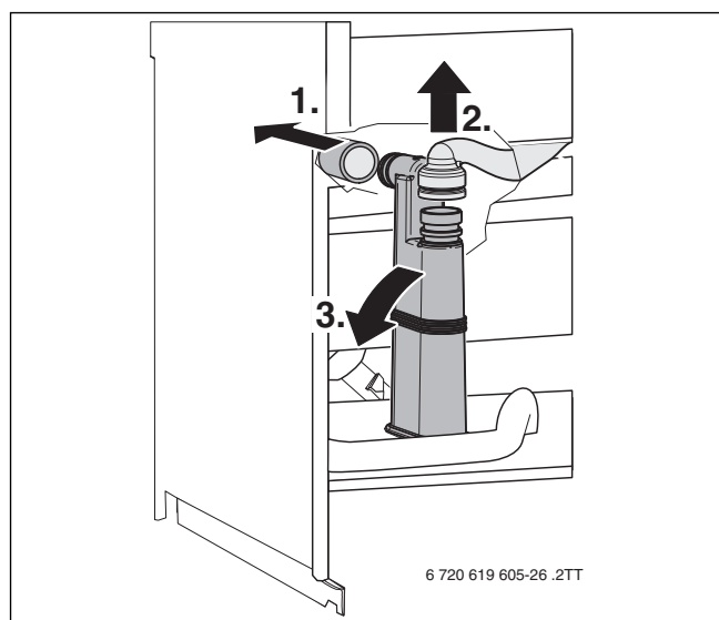
Afb. 57 Condenssifon demonteren
