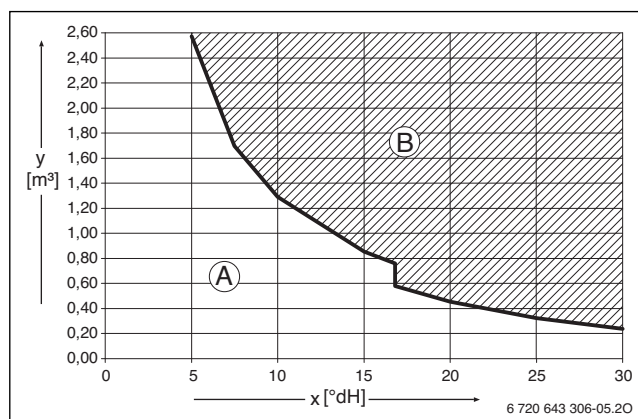
Afb. 18 Eisen aan het vul- en bijvulwater in °dH voor toestellen &lt; 50 kW
