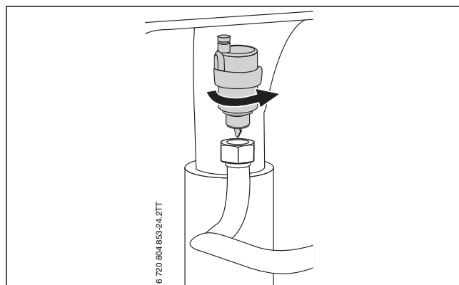
Afb. 63 Automatische ontluchter demonteren
