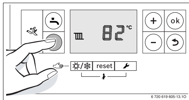
Afb. 33 Weergave aanvoertemperatuur
