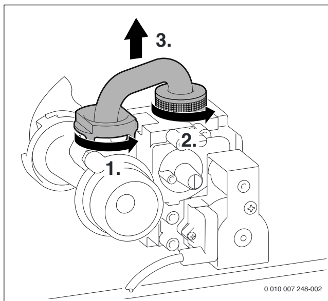
Afb. 67 Gasleiding demonteren
