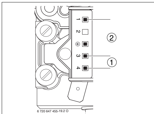
Afb. 66 Meetpunten op het gasblok
