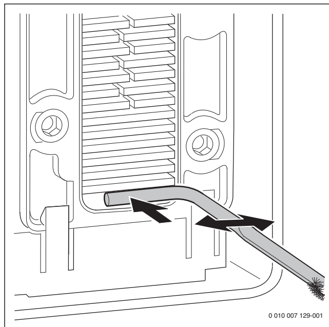
Afb. 56 Reinigen condensbak
