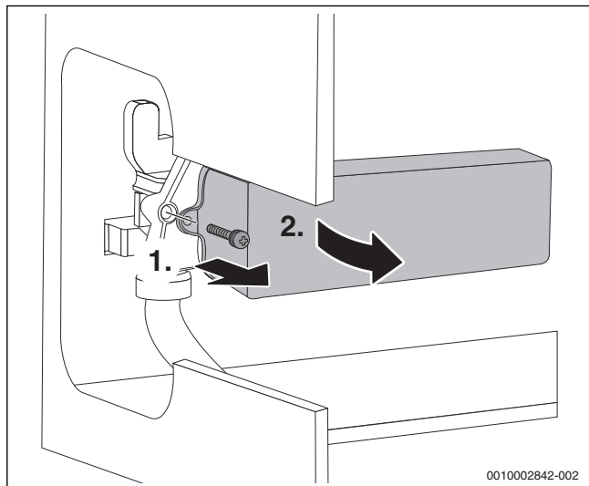
Afb. 60 Demonteren platenwarmtewisselaar
