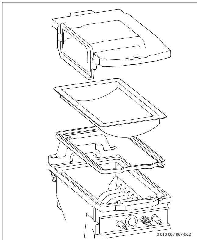
Afb. 50 Brander
