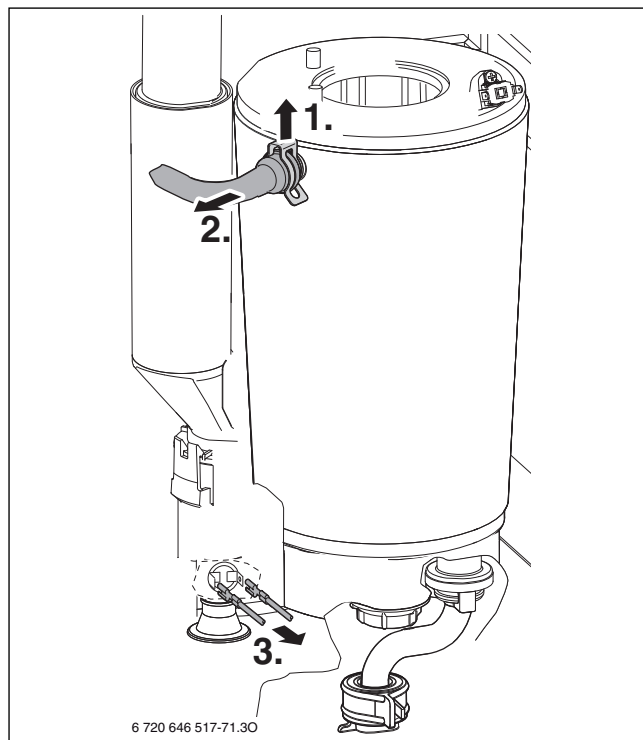
Afb. 74 Maak de aanvoerleiding los en trek de kabel los
