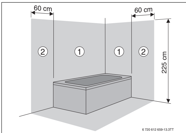
Afb. 30 Veiligheidszones
