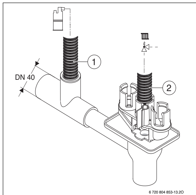
Afb. 28 Monteer de condensslang en de slang van het veiligheidsventiel op het sifon
