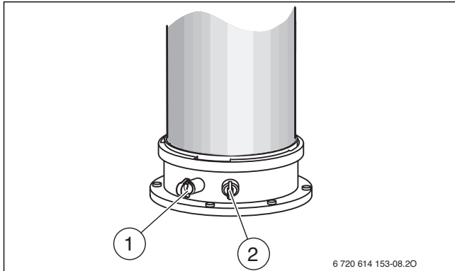
Afb. 49 Rookgasmeetpunt en verbrandingsluchtmeetpunt
