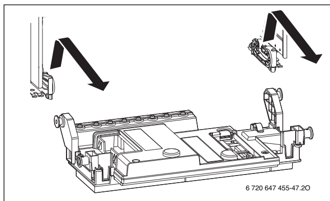
Afb. 73 Haak de besturing los
