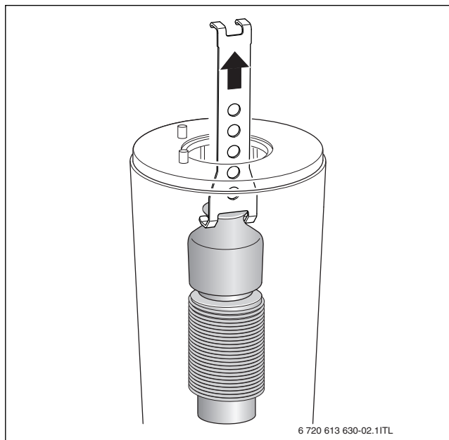
Afb. 54 Neem de bovenste warmteverspreider uit
