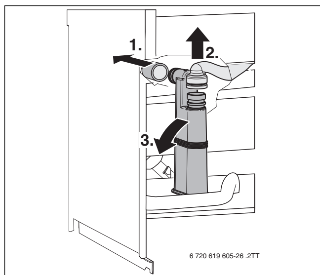
Afb. 59 Condenssifon demonteren
