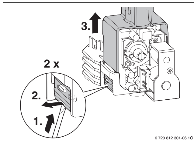
Afb. 69 Gasblok demonteren
