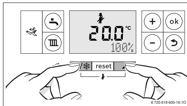
Afb. 48 100 % (maximaal nominaal warmtevermogen warm water)
