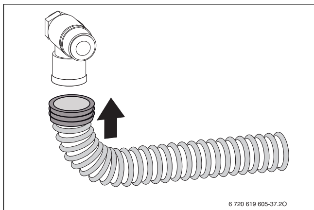
Afb. 25 Monteer de slang op het veiligheidsventiel
