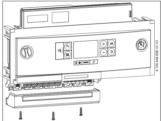
Afb. 31 Verwijderen afdekking
