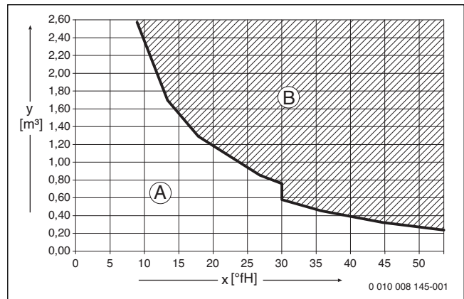
Afb. 22 Eisen aan het vul- en bijvulwater in °fH voor toestellen < 50 kW
