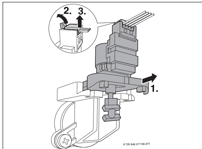
Afb. 65 Motor van de 3-wegklep demonteren
