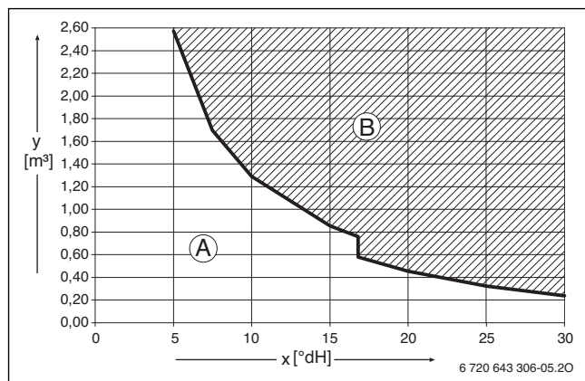
Afb. 21 Eisen aan het vul- en bijvulwater in °dH voor toestellen < 50 kW
