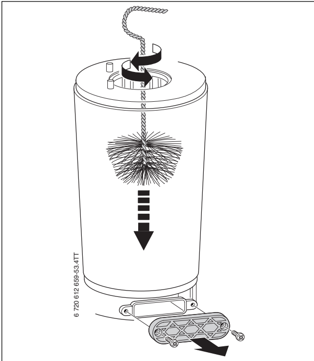
Afb. 56 Verwarmingslichaam reinigen
