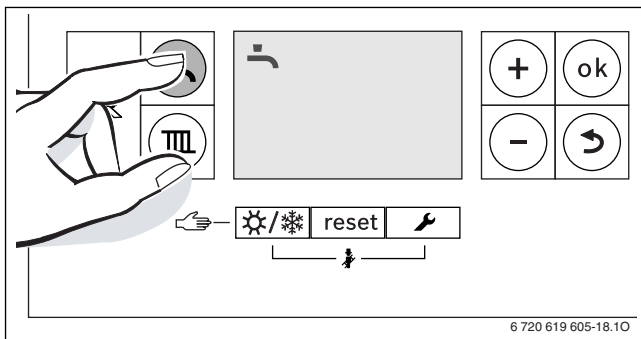
Afb. 38 Weergave warmwaterbedrijf
