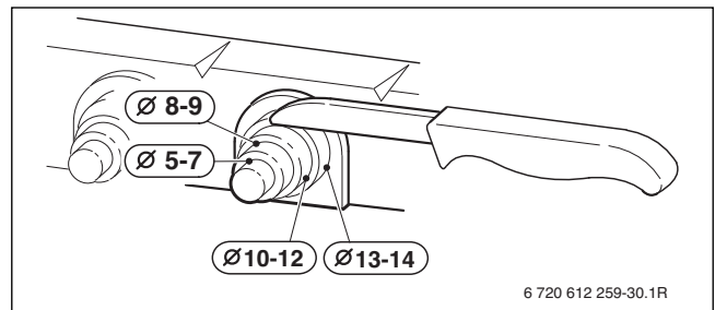
Afb. 32 Aanpassen trekontlasting aan de kabeldiameter
