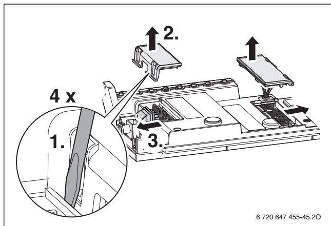
Afb. 72 Verwijderen afdekking
