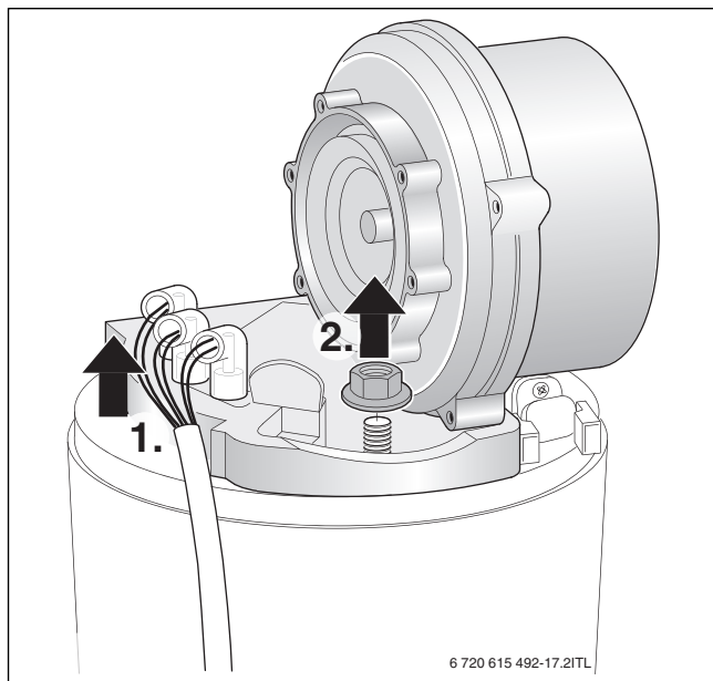
Afb. 52 Ventilator uitnemen
