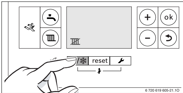
Afb. 42 Inschakelen handmatig zomerbedrijf
