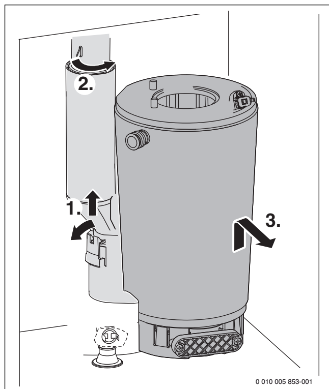
Afb. 76 Verwarmingslichaam demonteren
