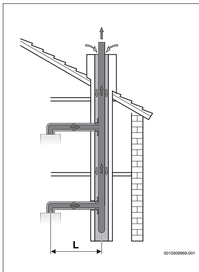
Afb. 18 Collectieve rookgasafvoer met concentrische buis conform C 43
