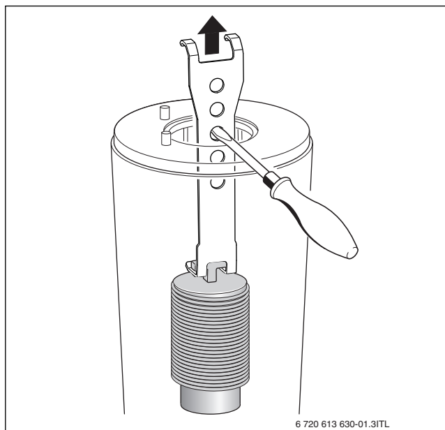
Afb. 55 Neem de onderste warmteverspreider uit
