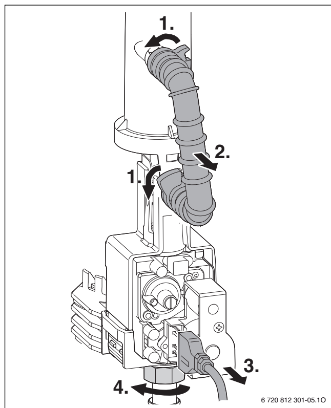
Afb. 68 Gasblok demonteren
