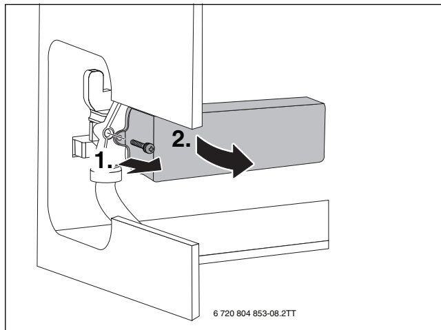
Afb. 61 Platenwarmtewisselaar demonteren
