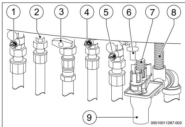
Afb. 29 Gas- en waterzijdige aansluitingen (toebehoren)
