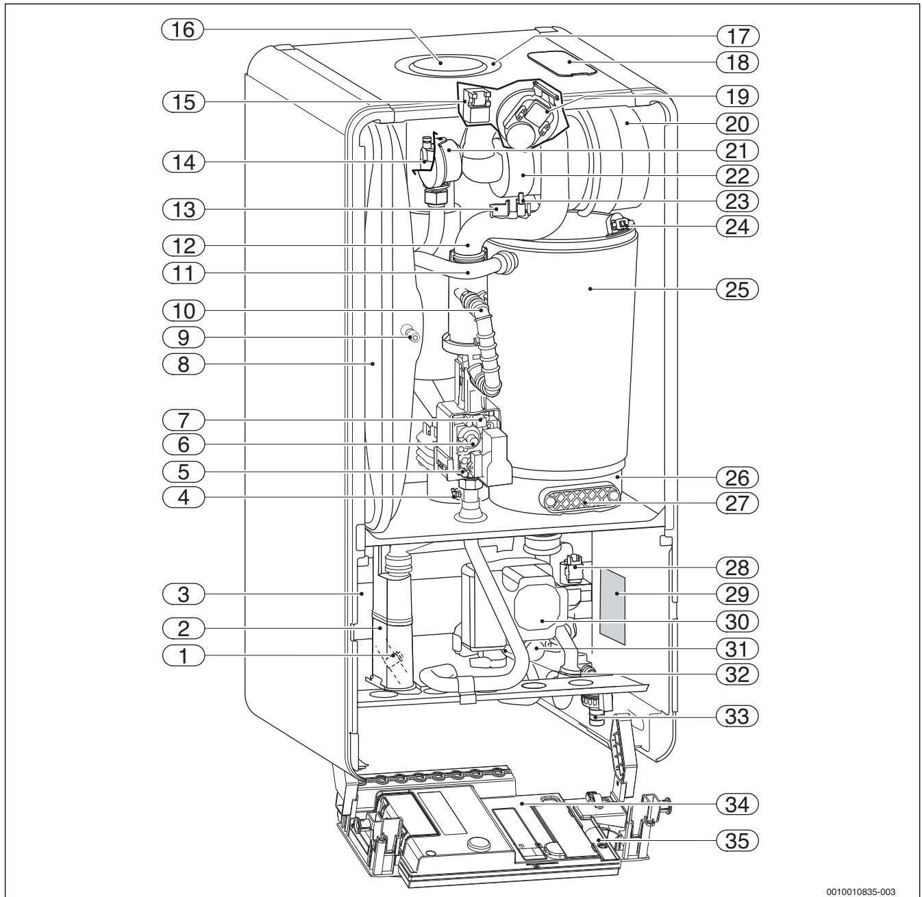
Afb. 3 Productoverzicht
