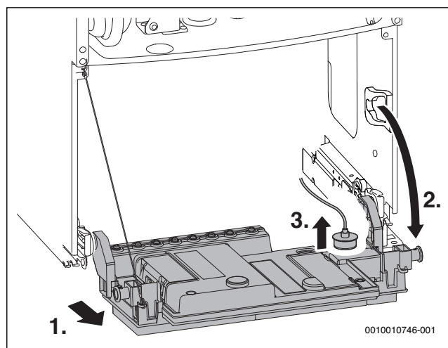
Afb. 71 Klap de besturing naar beneden
