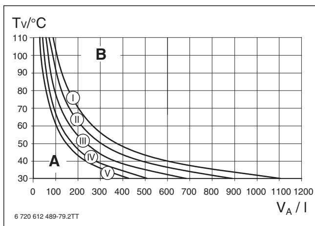
Afb. 23 Karakteristiek van het expansievat
