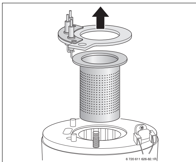
Afb. 53 Brander wegnemen
