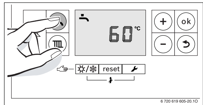
Afb. 40 Weergave warmwatertemperatuur
