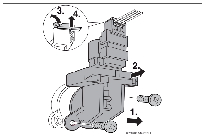
Afb. 66 3-wegklep demonteren
