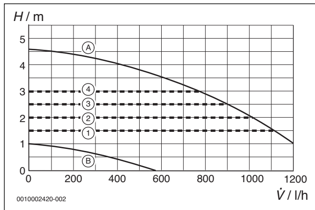
Afb. 81 Pompkarakteristieken en pompcurven
