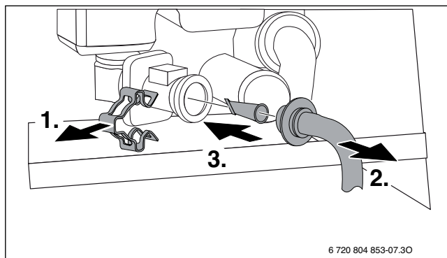
Afb. 62 Demonteer het filter uit de koudwaterleiding
