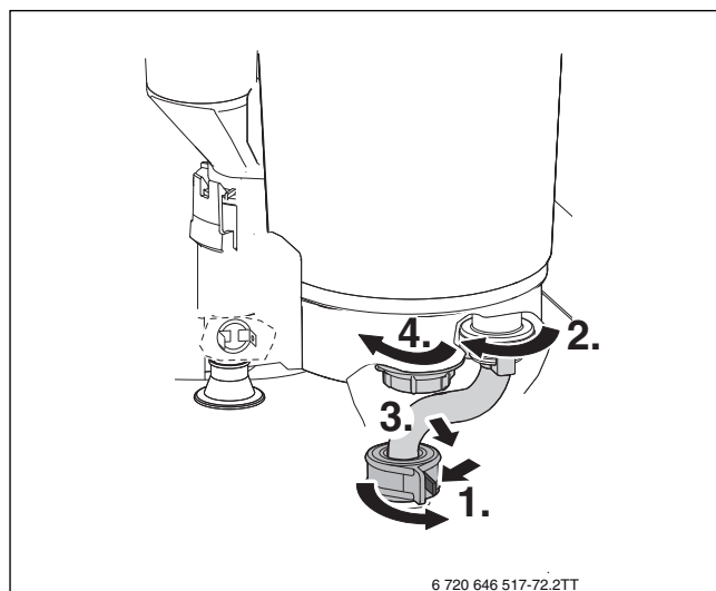
Afb. 75 Verwijder de moer en maak de retourleiding los
