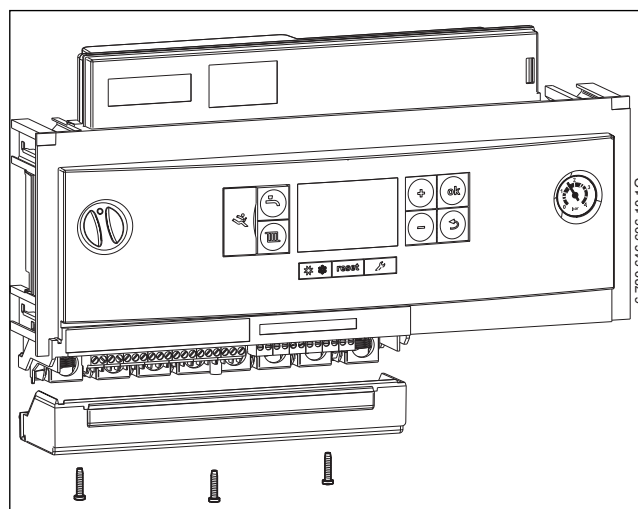
Afb. 70 Verwijderen afdekking
