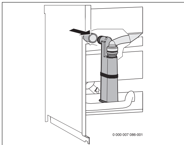
Afb. 26 Slang op condensatsifon monteren
