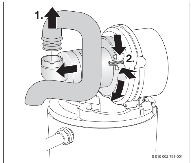
Afb. 51 Demonteer de aanzuigbuis en de menginrichting
