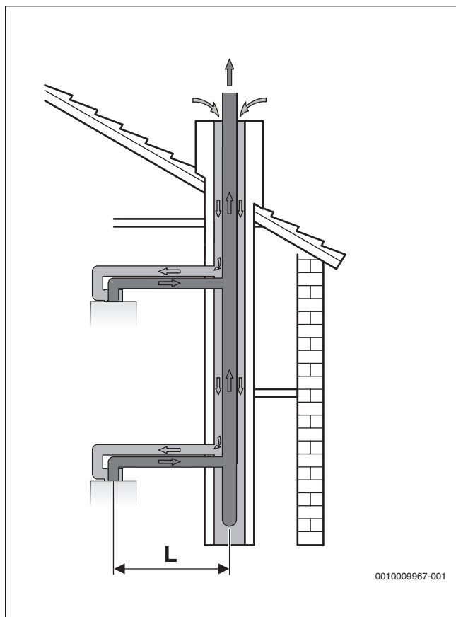
Afb. 19 Collectieve rookgasafvoer met parallelbuis conform C 43
