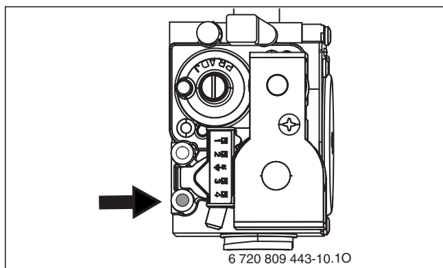
Afb. 47 Meetpunt voor gasaansluitdruk
