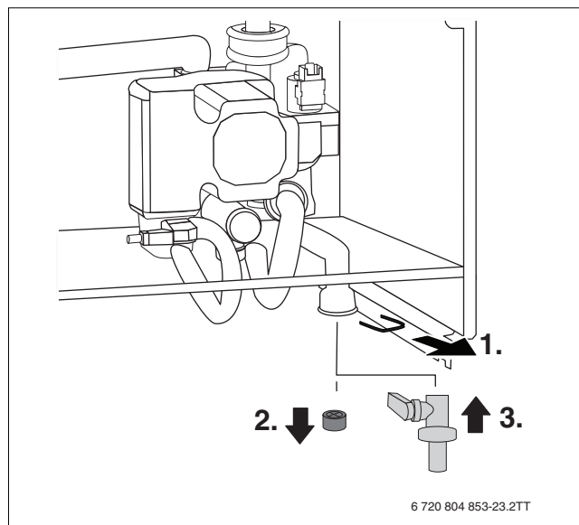
Afb. 27 Monteer de vul- en aftapkraan
