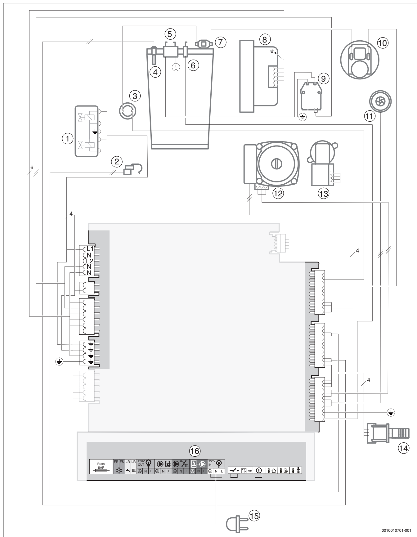
Afb. 79 Elektrische bedrading
