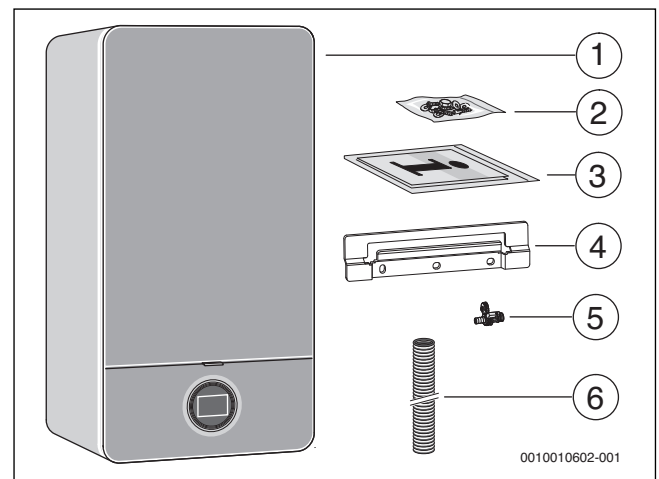
Afb. 1 Leveringsomvang
