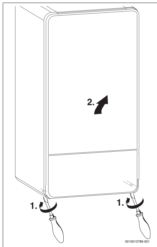
Afb. 24 Verwijderen mantel
