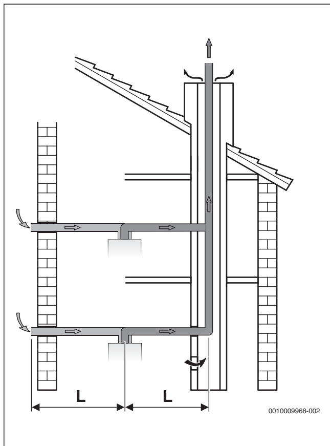
Afb. 20 Collectieve rookgasafvoer met parallelbuis conform C 83
