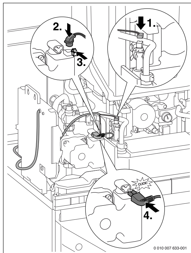
Afb. 50 Boilerlaadpomp en warmwatertemperatuursensor aansluiten
