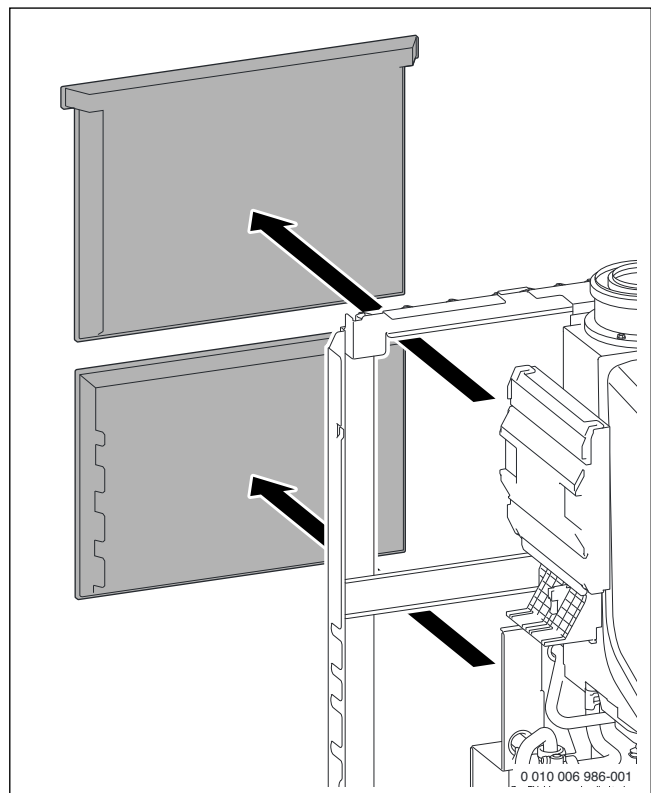
Afb. 56 Warmte-isolatie aan de achterzijde afnemen
