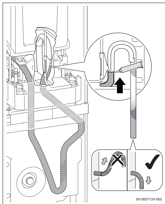
Afb. 43 Sifonslang op eindstuk steken
