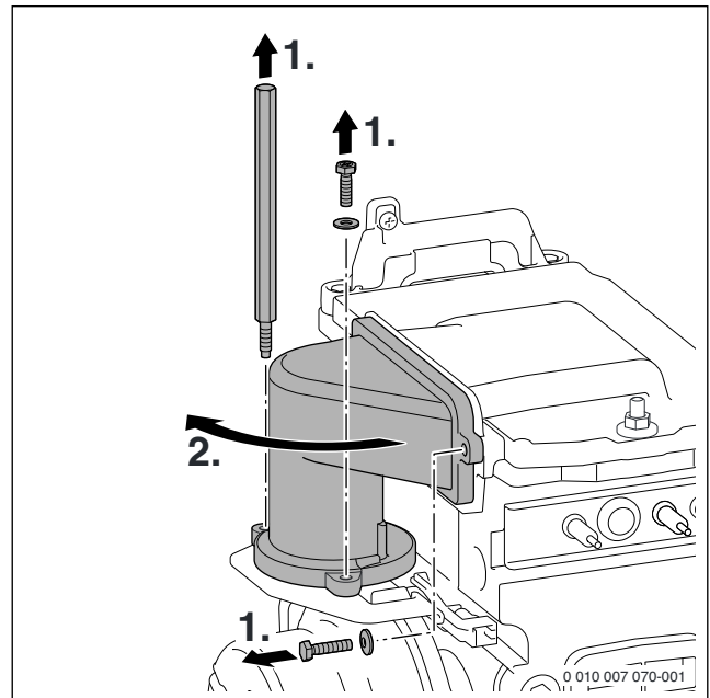
Afb. 103 Demonteer de menginrichting
