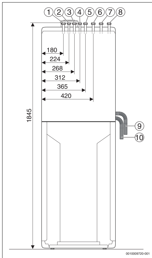
Afb. 5 Aansluitmaten van de toebehoren CS 11 - Verticale aansluitset (maten in mm)
