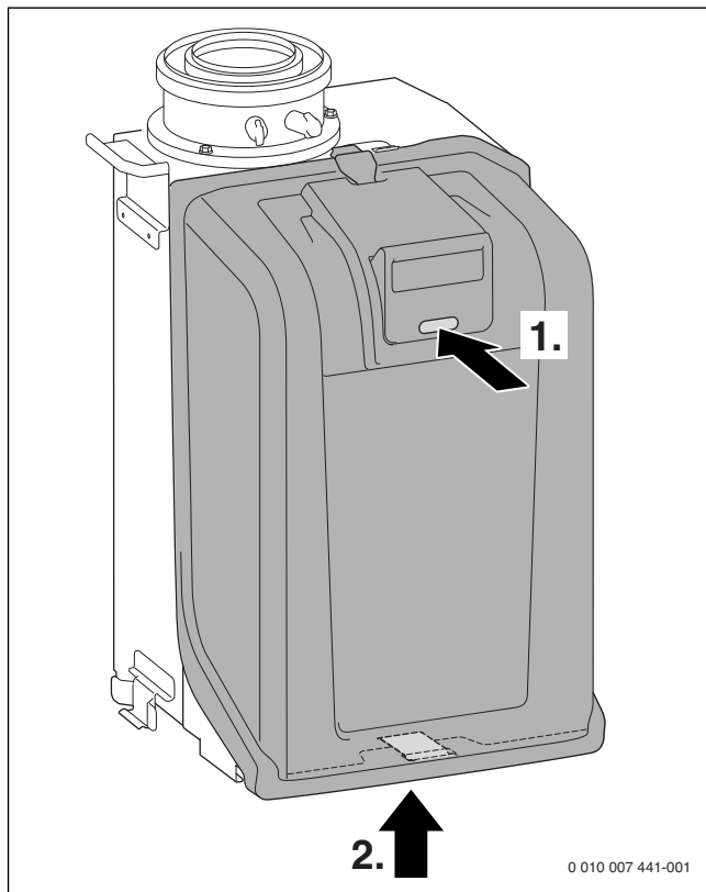
Afb. 87 Branderkap verwijderen
