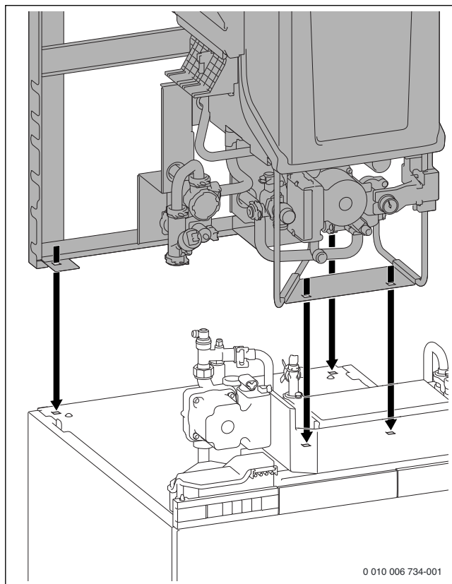
Afb. 39 Ketel op de boiler plaatsen
