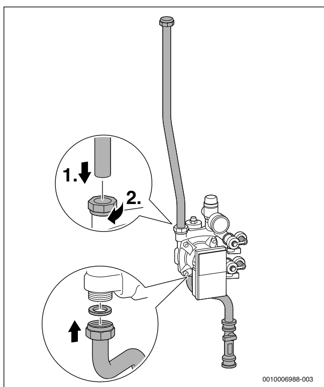
Afb. 58 Solar-retourleiding en debietbegrenzer op de solargroep monteren
