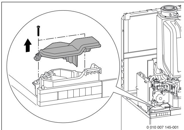
Afb. 52 Afdekking van de aansluitbox verwijderen
