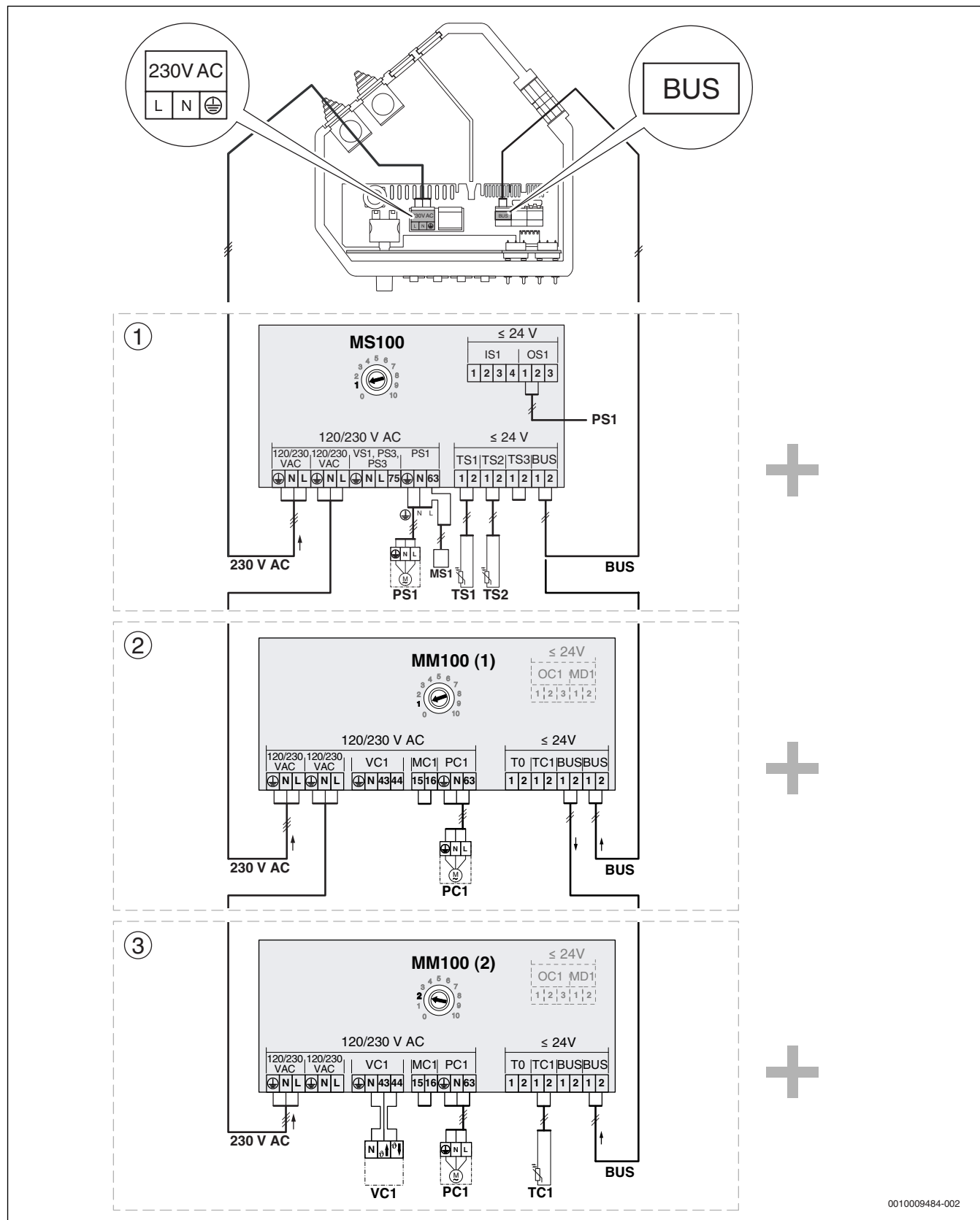
Afb. 69 Aansluiting van de module MS 100 en MM 100, indien aanwezig
