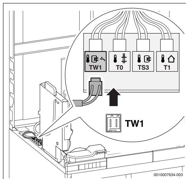
Afb. 51 Boilertemperatuursensor aansluiten
