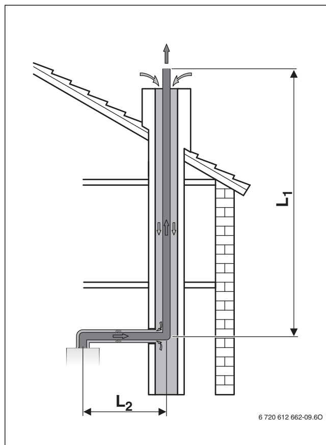
Afb. 20 Rookgasafvoer in schacht conform C 93
