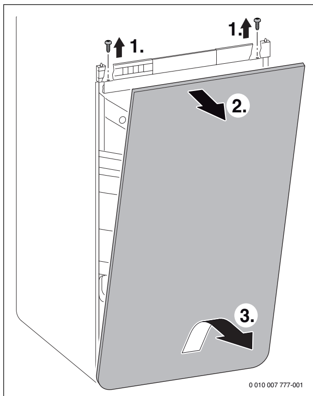
Afb. 37 Voorste mantel van de boiler afnemen
