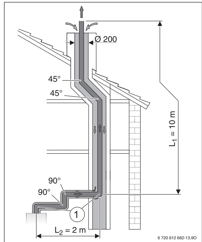
Afb. 26 Inbouwsituatie van een rookgasafvoersysteem in een schacht conform C 93
