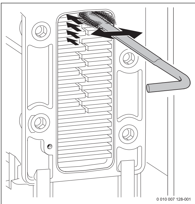
Afb. 98 Warmtewisselaar met borstel reinigen
