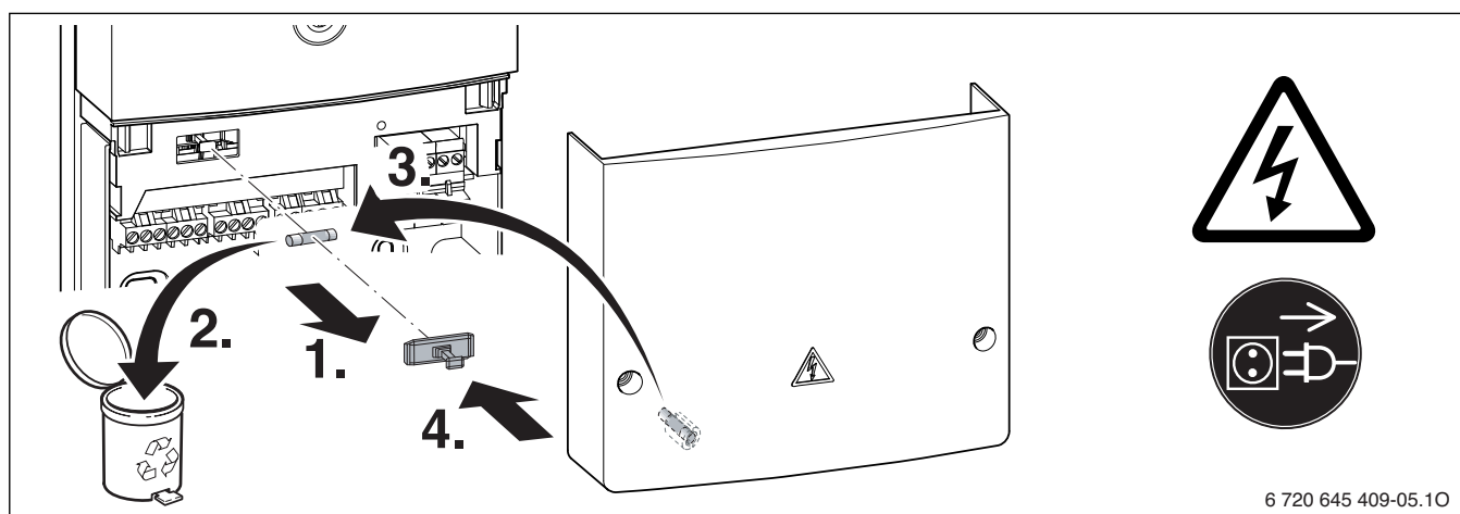
Afb. 113 Zekering van module vervangen
