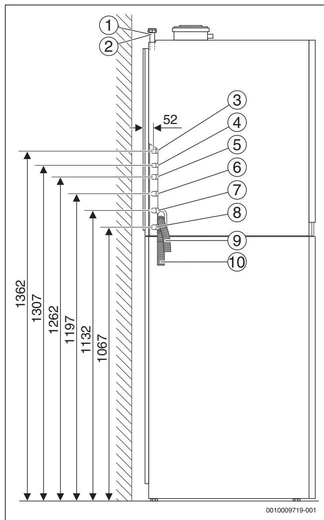
Afb. 4 Aansluitmaten van de toebehoren CS 10 - Horizontale aansluitset (maten in mm)
