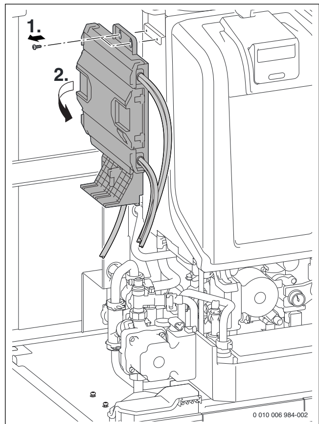
Afb. 47 Besturing afnemen
