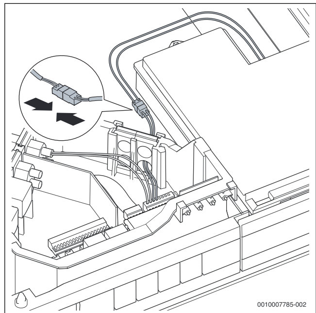
Afb. 55 Schuiflade voor de regelaar op de aansluitbox aansluiten
