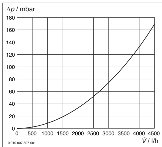
Afb. 117 Drukverliesdiagram gemengd cv-circuit (HK2)
