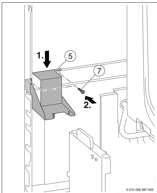
Afb. 57 Houder voor het solarstation met schroef fixeren
