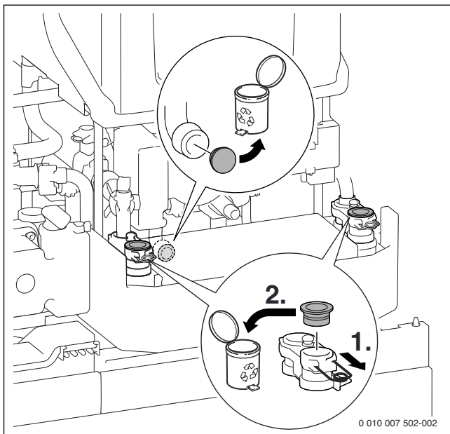
Afb. 44 Stop op verwarmingslichaam en op de platenwarmtewisselaar verwijderen
