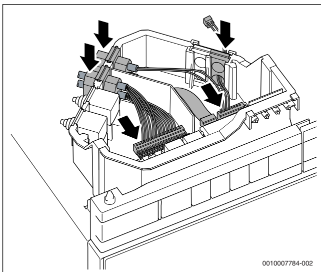
Afb. 53 Besturing op de aansluitbox aansluiten
