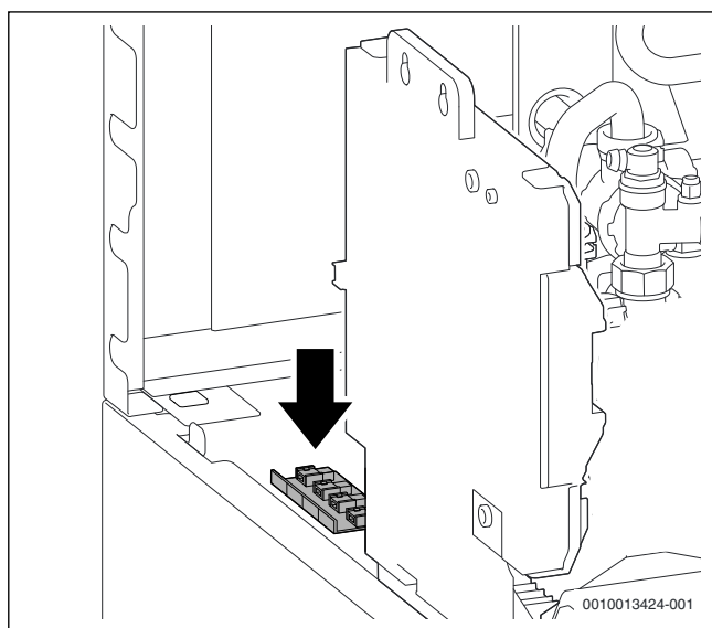
Afb. 49 Stekkerstrook op de boiler bevestigen
