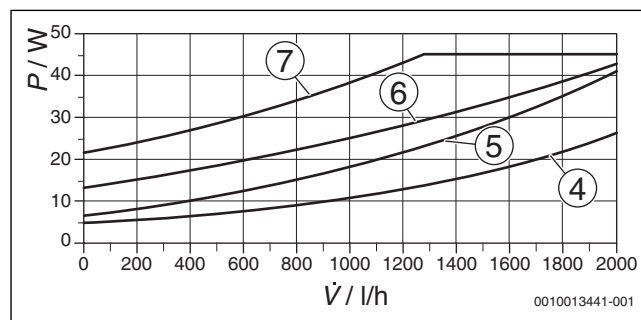
Afb. 123 Opgenomen vermogen voor proportionele druk en constante druk
