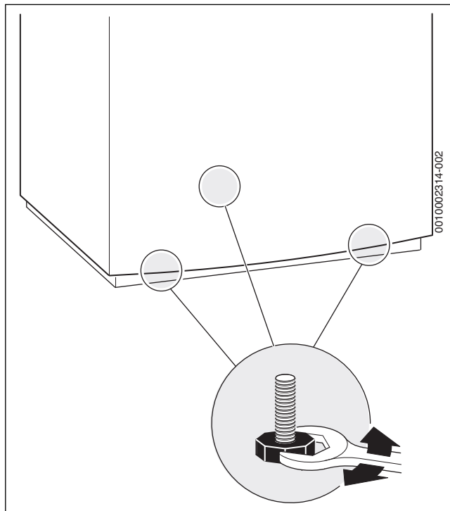
Afb. 38 Boiler uitlijnen
