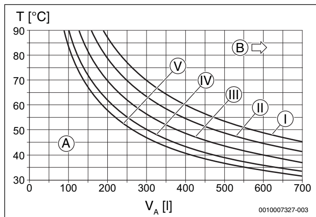
Afb. 32 Karakteristiek van het expansievat 17 l
