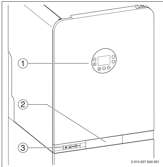
Afb. 82 Overzicht bedieningselementen
