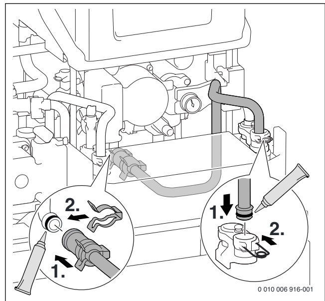
Afb. 46 Leidingverbinding tussen platenwarmtewisselaar en verwarmingslichaam uitvoeren (retour)
