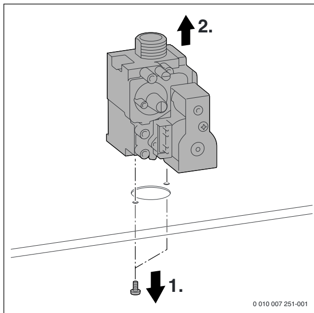
Afb. 109 Gasblok demonteren
