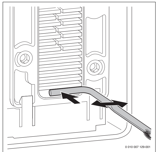
Afb. 100 Condensbak reinigen
