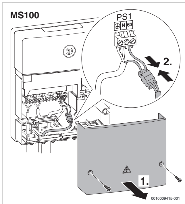
Afb. 62 Stekker van de temperatuurbegrenzer solar MS1 in module MS 100 verbinden
