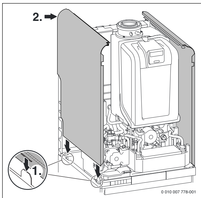
Afb. 79 Rechter- en linkermantel monteren
