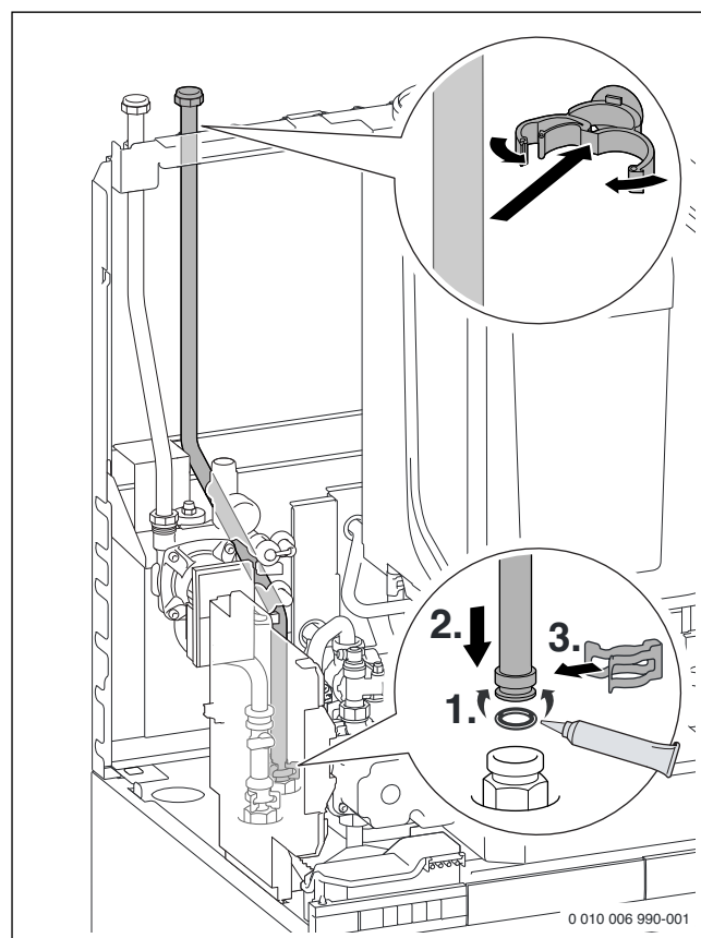
Afb. 60 Solaraanvoerleiding monteren en de leidingen boven bevestigen
