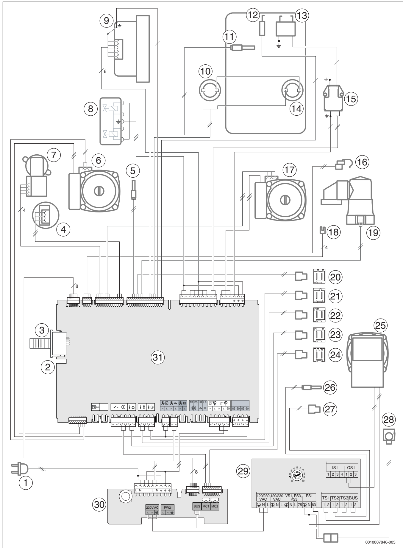
Afb. 114 Elektrische bedrading
