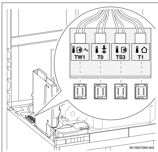
Afb. 70 Stekker op besturing
