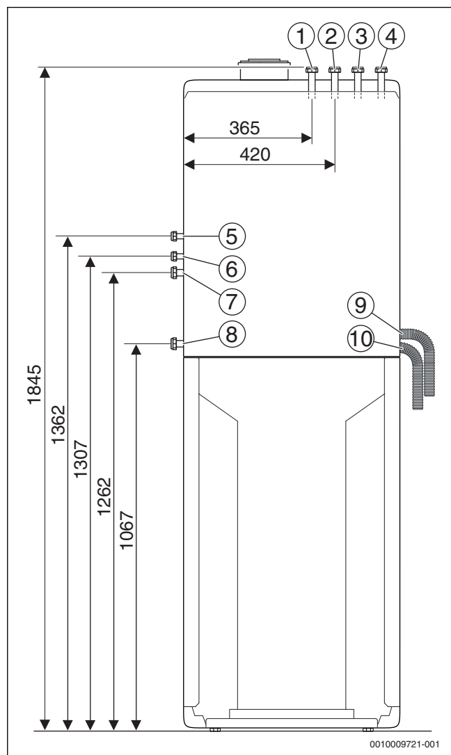
Afb. 7 Aansluitmaten van de toebehoren CS 12 - CV-circuituitbreiding 1 (maten in mm)
