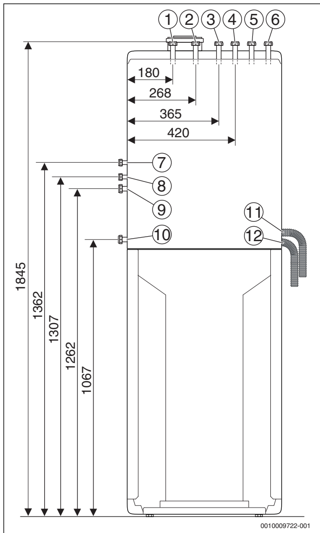
Afb. 9 Aansluitmaten van de toebehoren CS 13 - CV-circuituitbreiding 2 (maten in mm)
