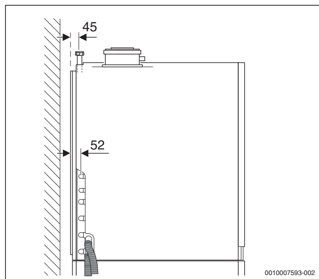
Afb. 8 Aansluitmaten van de toebehoren CS 12 - CV-circuituitbreiding 1 (maten in mm)
