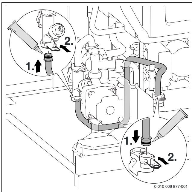
Afb. 45 Leidingverbinding tussen 3-wegklep en platenwarmtewisselaar uitvoeren (aanvoer)
