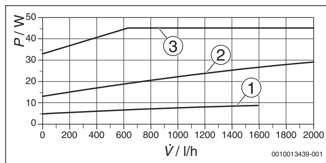
Afb. 122 Opgenomen vermogen voor de pompstanden I tot III
