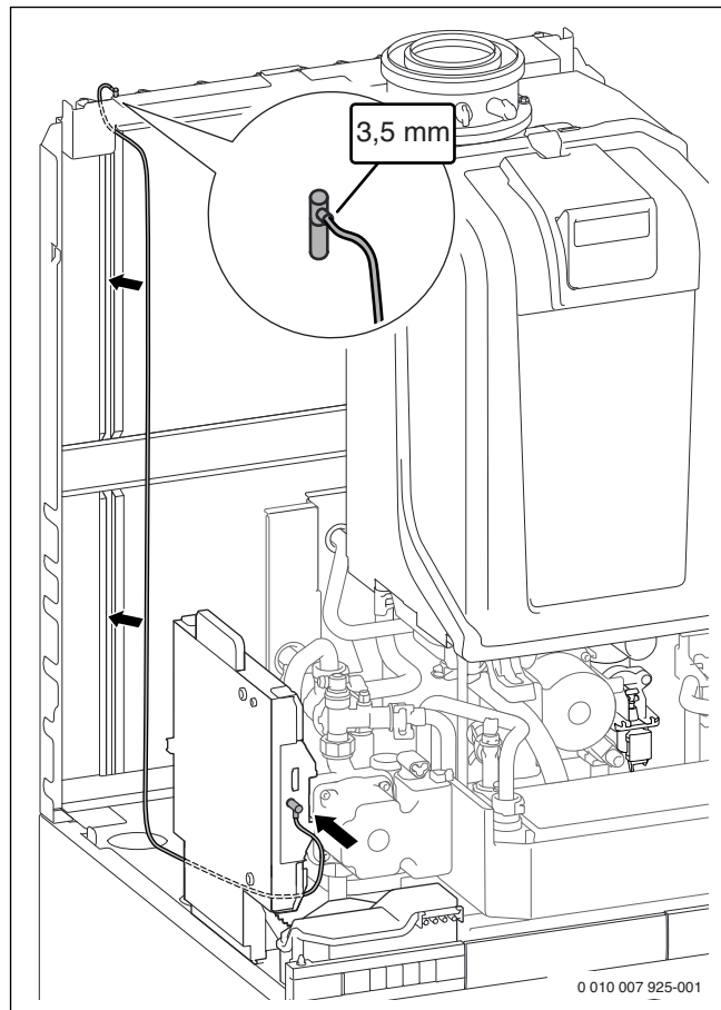
Afb. 71 Aansluiting en installatie van de kabel op Bosch MB LANi
