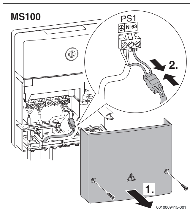
Afb. 72 Stekker van de temperatuurbegrenzer solar MS1 in module MS 100 verbinden
