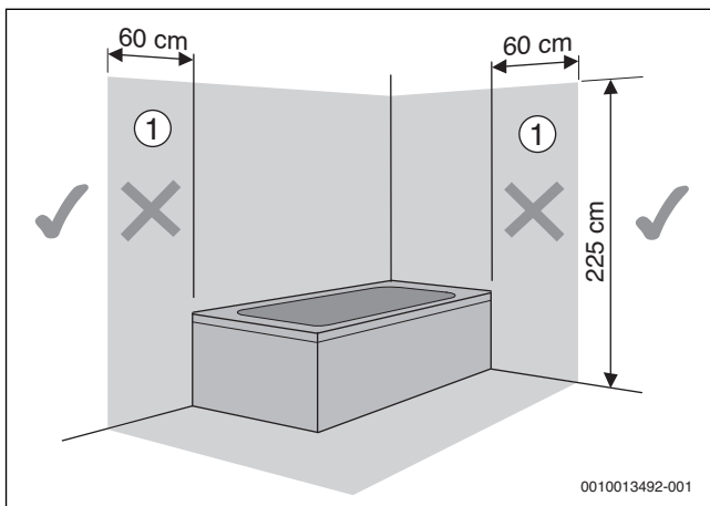
Afb. 65 Veiligheidszones
