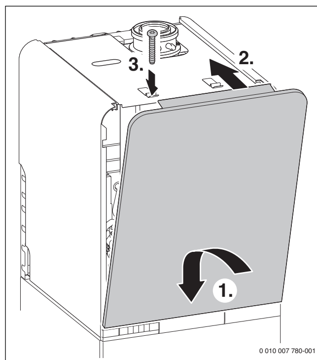
Afb. 81 Voorste mantel inhangen en met de schroef uit de leveringsomvang borgen
