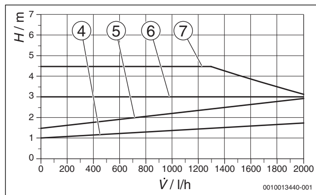
Afb. 121 Pompkarakteristiek voor proportionele druk en constante druk
