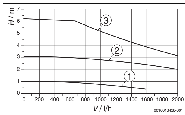
Afb. 120 Pompcurve voor de pompstanden I tot III
