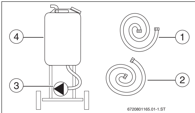
Afb. 76 Onderdelen van een vulinrichting
