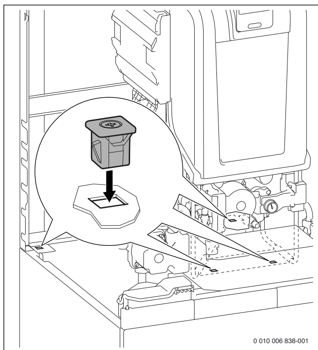
Afb. 40 Ketel met de 4 meegeleverde clips op de boiler fixeren
