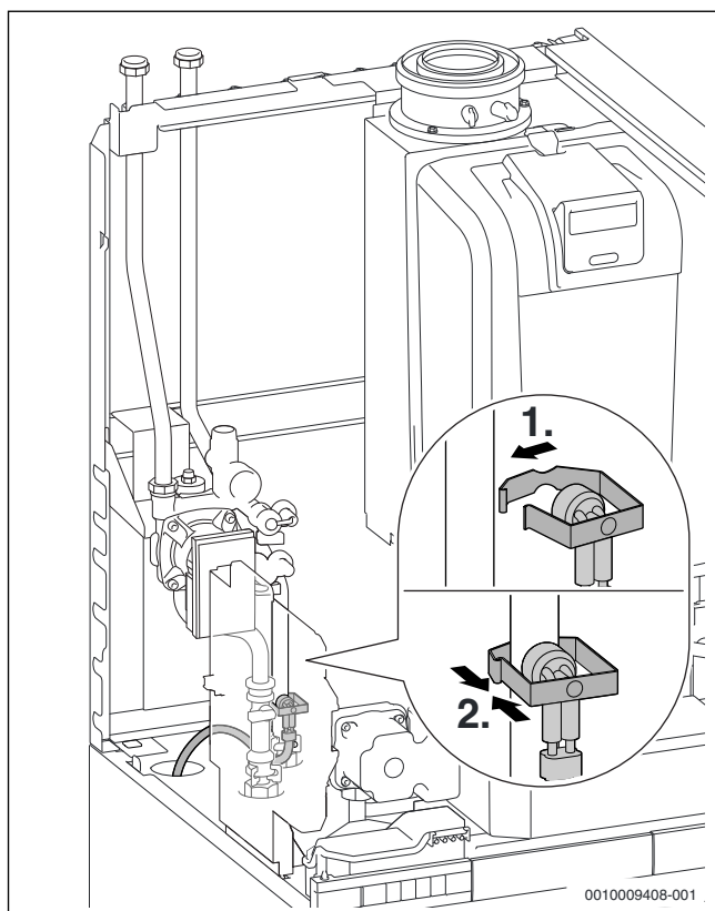
Afb. 61 Temperatuurbegrenzer solar MS1 op de solar-aanvoerleiding monteren
