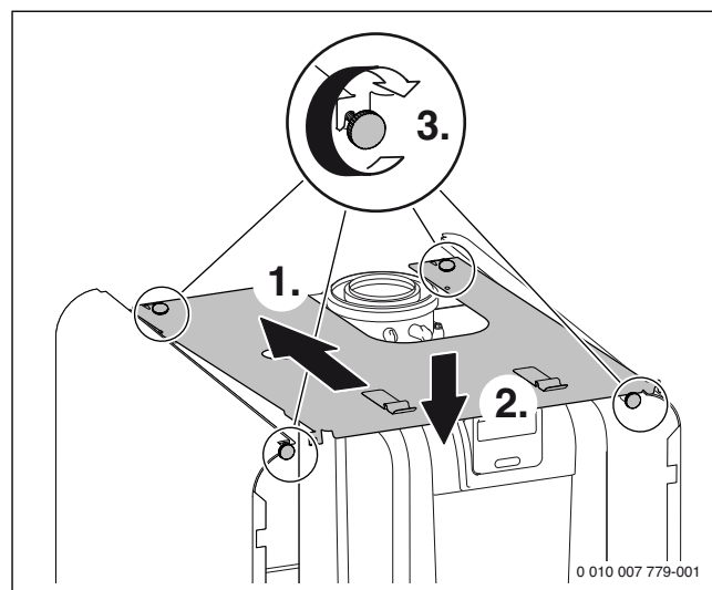
Afb. 80 Bovenste mantel naar achteren schuiven en met de 4 schroeven voor en achter bevestigen
