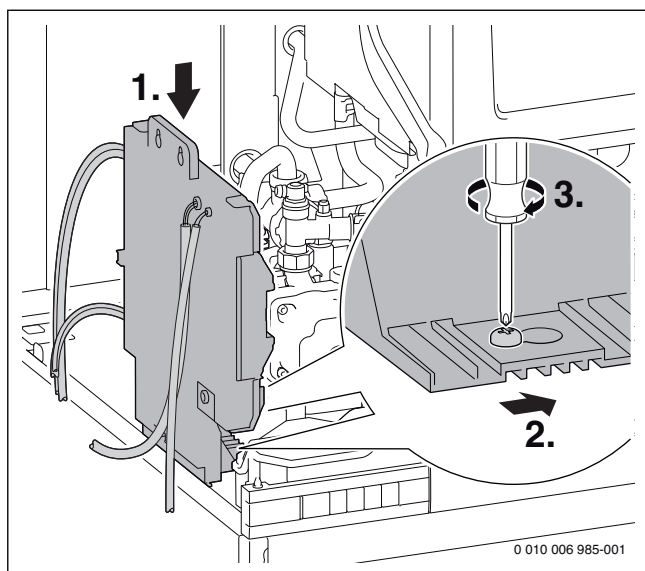
Afb. 48 Besturing op de boiler bevestigen
