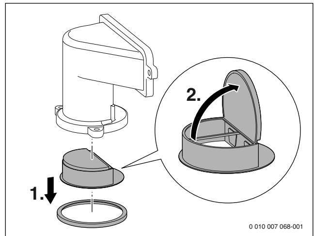
Afb. 104 Terugslagklep in de menginrichting
