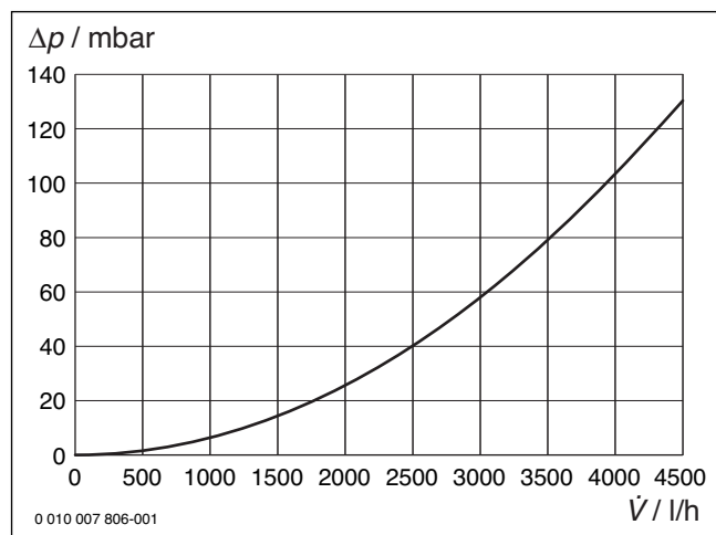
Afb. 116 Drukverliesdiagram ongemengd cv-circuit (HK1)
