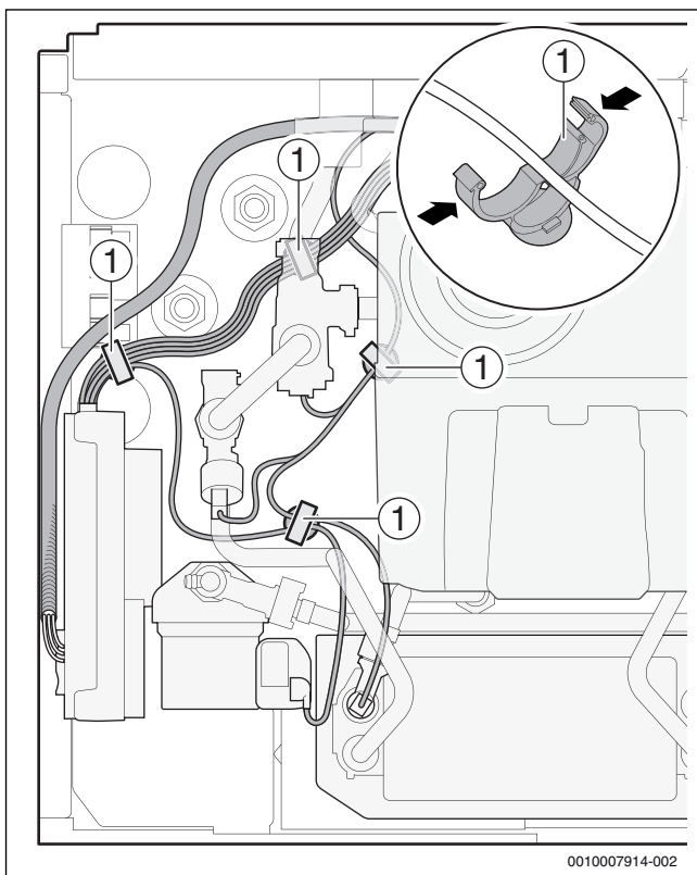
Afb. 54 Kabel met 4 clips bevestigen
