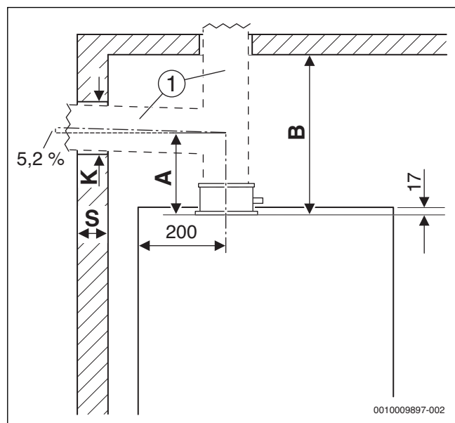
Afb. 11 Afmetingen
