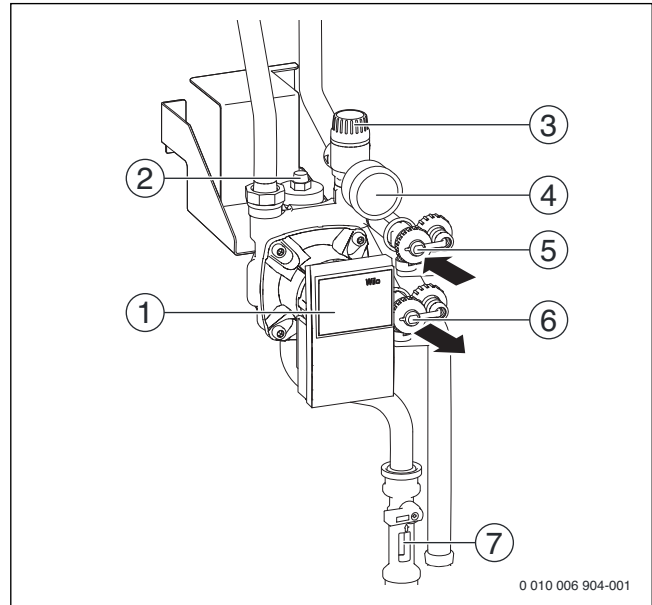
Afb. 77 Overzicht solargroep
