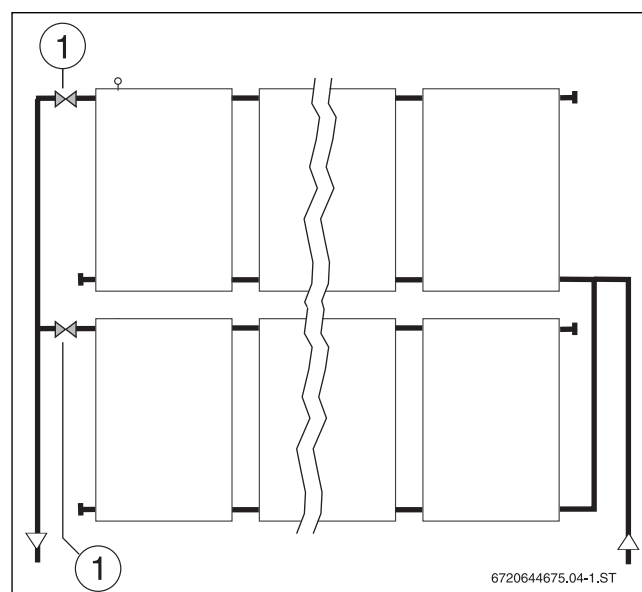
Afb. 75 Spoelen van parallel geschakelde collectorvelden
