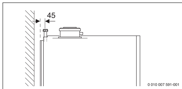
Afb. 6 Aansluitmaten van de toebehoren CS 11 - Verticale aansluitset (maten in mm)
