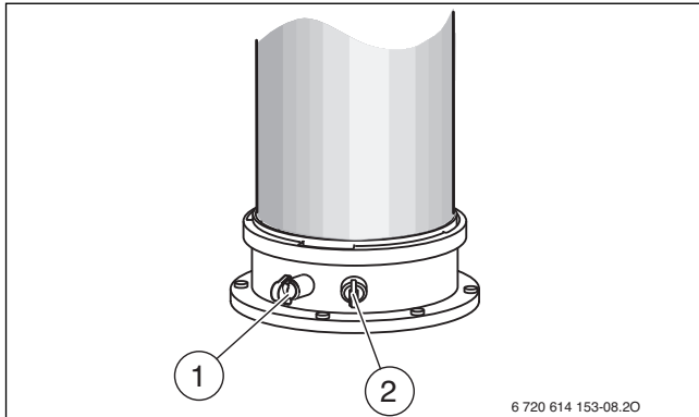
Afb. 90 Rookgasmeetpunt en verbrandingsluchtmeetpunt
