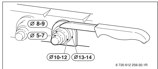
Afb. 67 Aanpassen trekcontlasting aan de kabeldiameter
