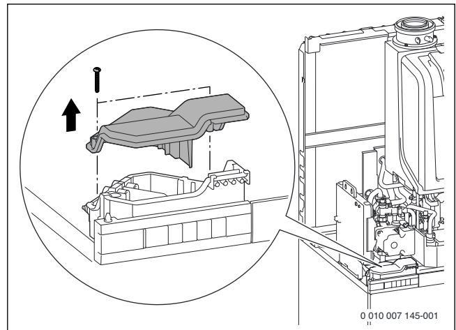
Afb. 66 Afdekking van de aansluitbox verwijderen
