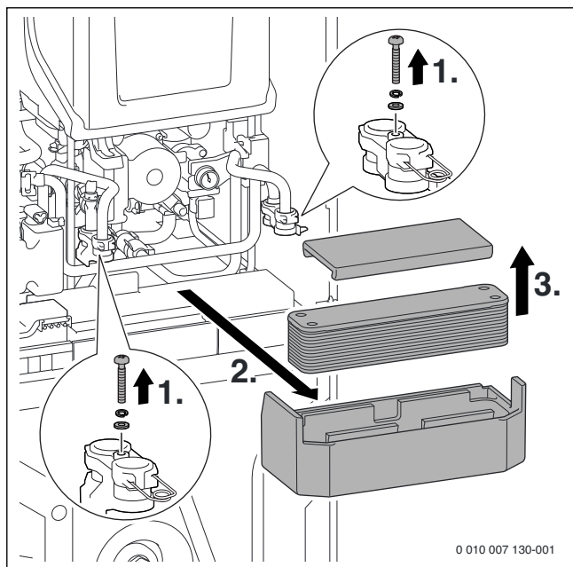
Afb. 105 Platenwarmtewisselaar demonteren
