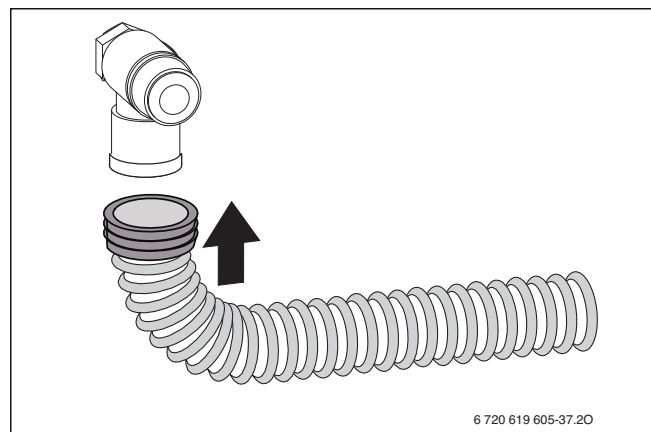
Afb. 33 Monteer de slang op het overstortventiel
