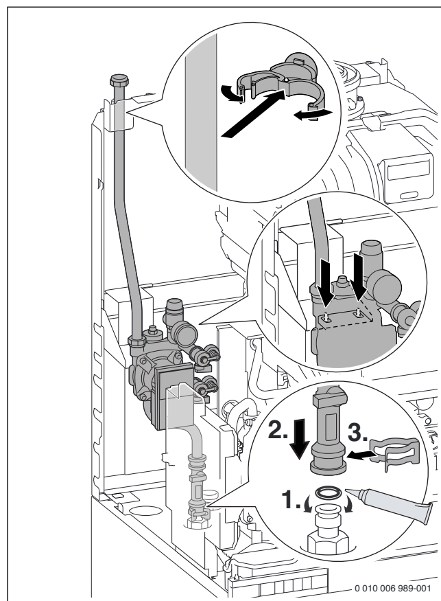
Afb. 59 Solarstation in de houder hangen en debietmeter op de boiler aansluiten
