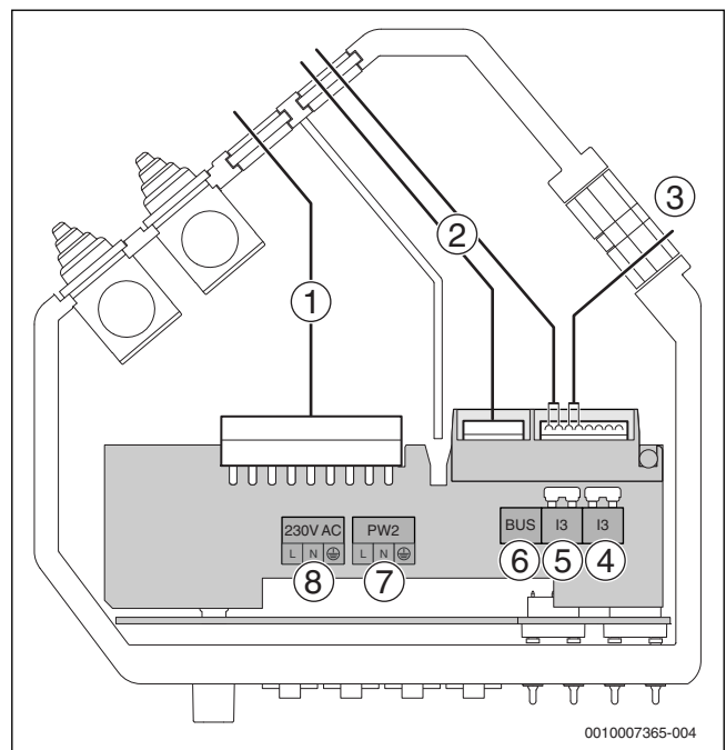
Afb. 68 Aansluitbox
