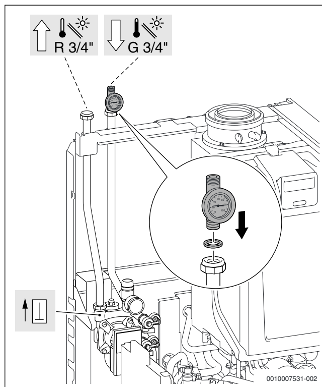
Afb. 63 Servicekraan met thermometer op de solaraanvoerleiding monteren
