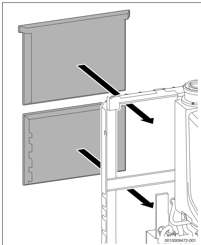
Afb. 78 Warmte-isolatie aan de achterzijde monteren
