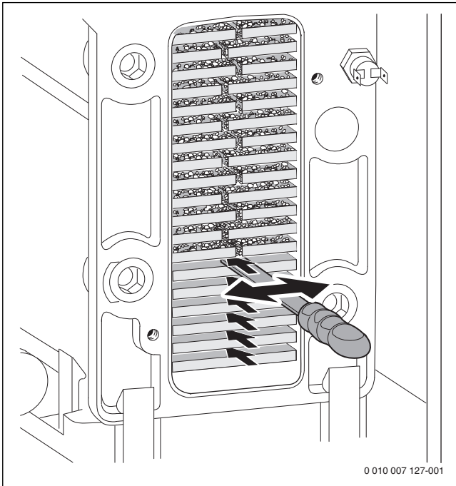
Afb. 97 Reinigingsgereedschap
