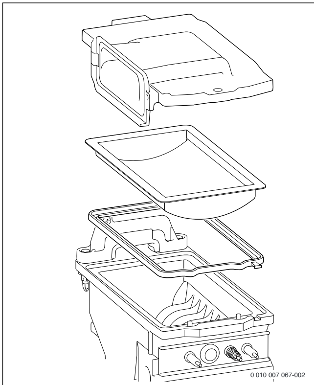
Afb. 94 Brander
