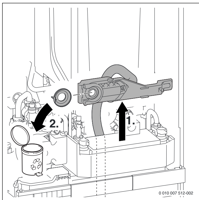
Afb. 41 Vuilfilter uit de onderhoudspositie nemen en beschermdeksel afnemen
