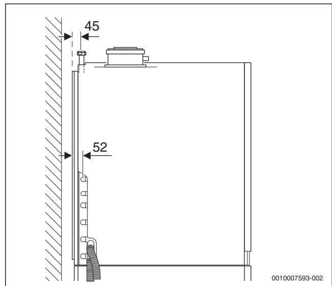
Afb. 10 Aansluitmaten van de toebehoren CS 13 - CV-circuituitbreiding 2 (maten in mm)
