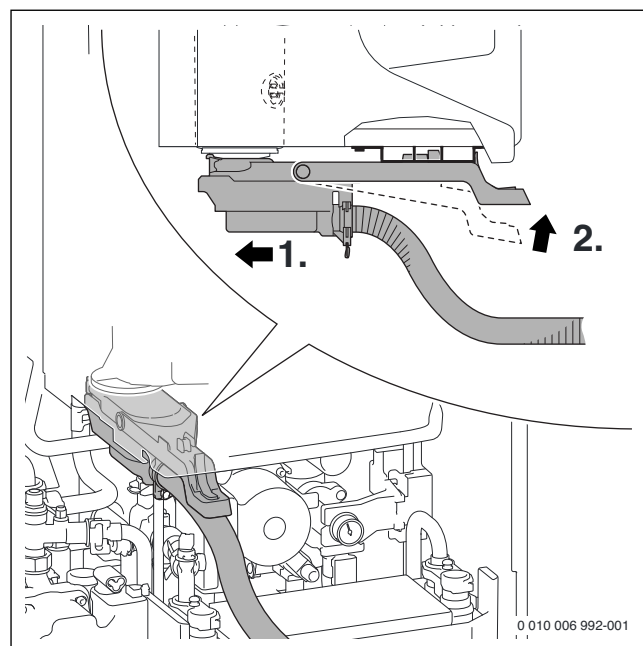
Afb. 42 Vuilfilter monteren
