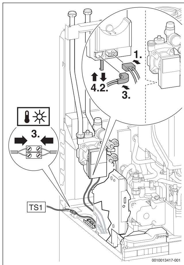
Afb. 64 Sluit solarpomp en collectortemperatuursensor TS1 aan
