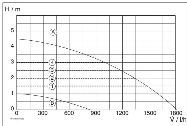
Afb. 105 Pompkarakteristieken en pompcurven
