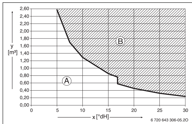
Afb. 35 Eisen aan het vul- en bijvulwater voor ketels < 50 kW
