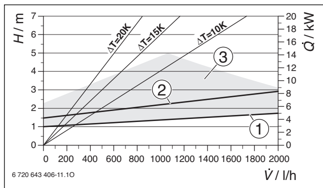
Afb. 112 Pompcurven
