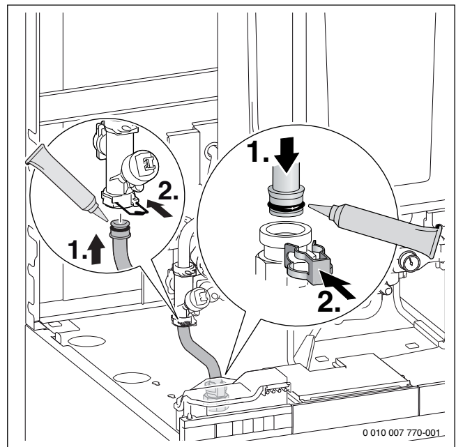
Afb. 48 Buisverbinding tussen 3-wegklep en boileraanvoer maken
