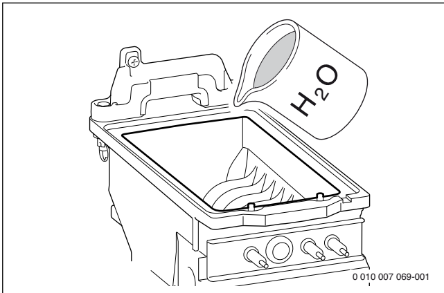
Afb. 91 Spoelen
