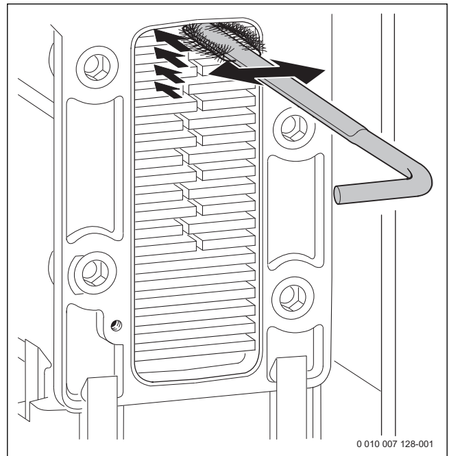
Afb. 90 Warmtewisselaar met borstel reinigen
