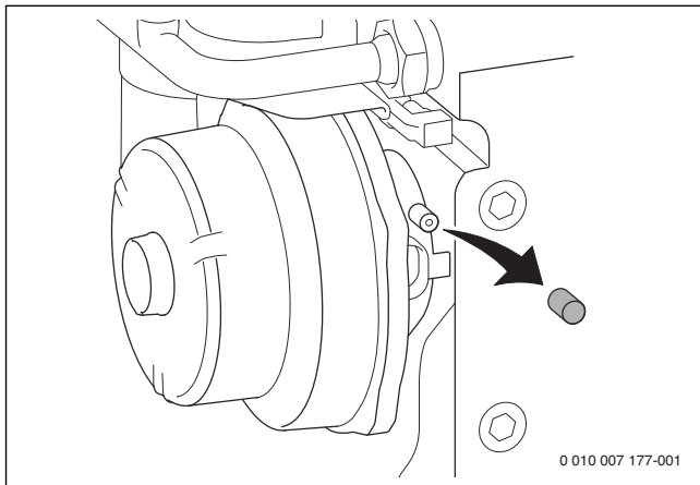
Afb. 88 Meetpunt op de menginrichting
