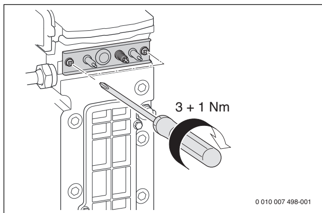
Afb. 83 Elektrodenset weer inbouwen
