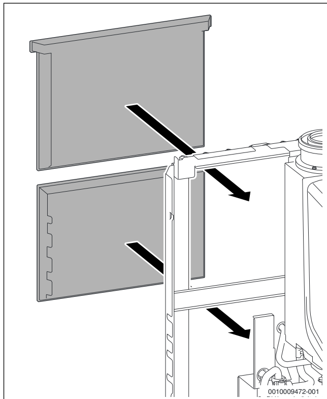
Afb. 70 Warmte-isolatie aan de achterzijde monteren
