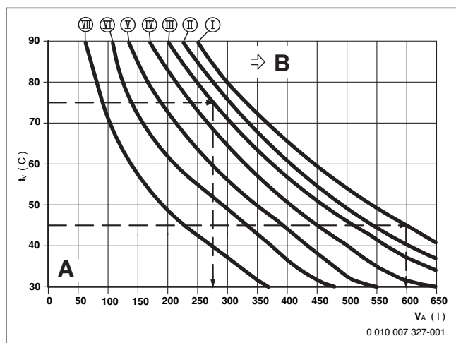
Afb. 36 Karakteristiek van het expansievat 18 l
