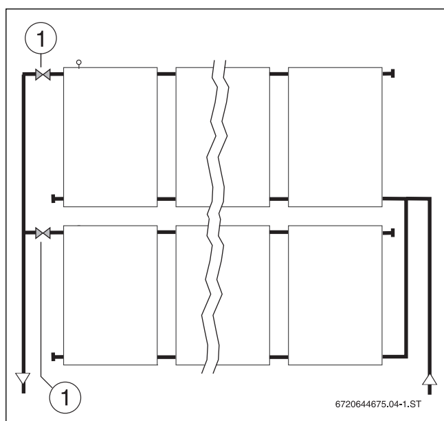
Afb. 67 Spoelen van parallel geschakelde collectorvelden
