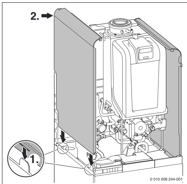
Afb. 71 Rechter- en linkermantel monteren
