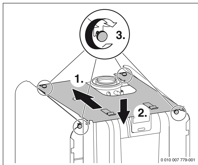
Afb. 72 Bovenste mantel naar achteren schuiven en met de 4 schroeven voor en achter bevestigen
