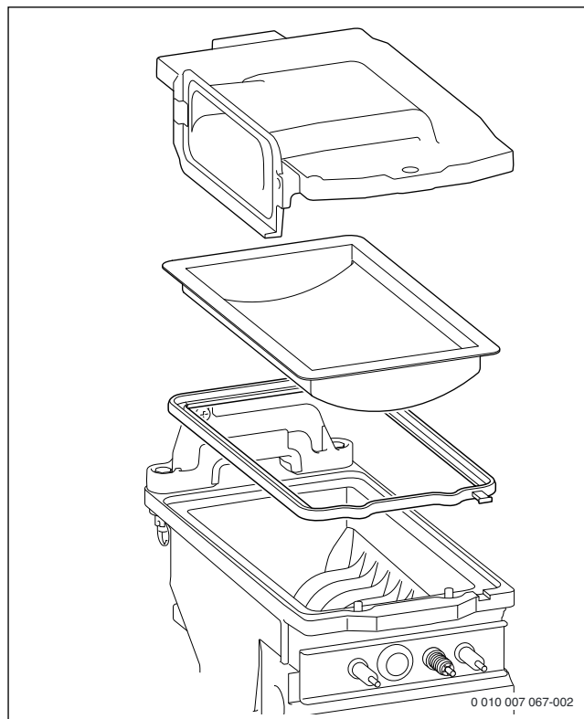
Afb. 86 Brander
