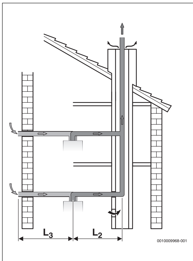
Afb. 34 Collectieve rookgasafvoer met parallelbuis conform C 83
