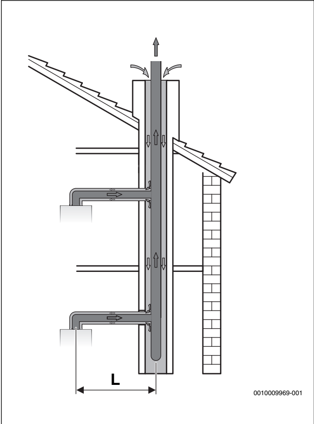
Afb. 32 Collectieve rookgasafvoer met concentrische buis conform C 43
