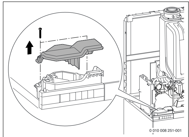
Afb. 60 Afdekking van de aansluitbox verwijderen
