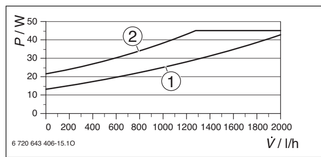
Afb. 115 Opgenomen vermogen
