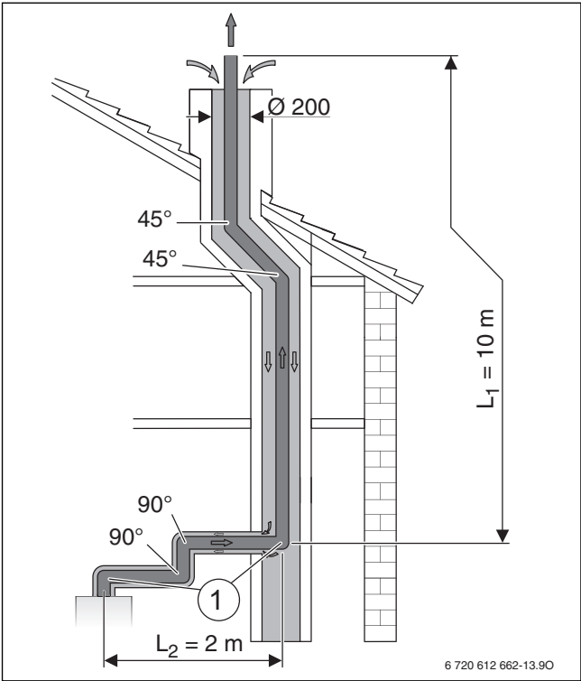
Afb. 31 Inbouwsituatie van een rookgasafvoersysteem conform C 93
