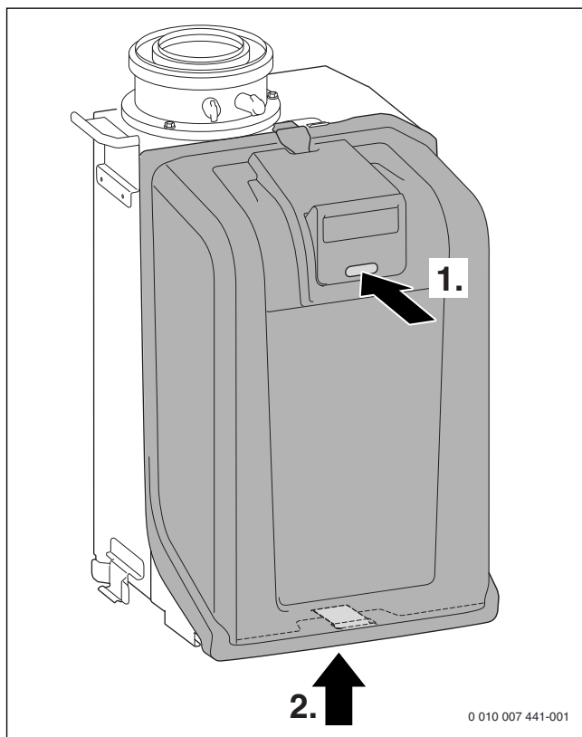
Afb. 79 Branderkap verwijderen
