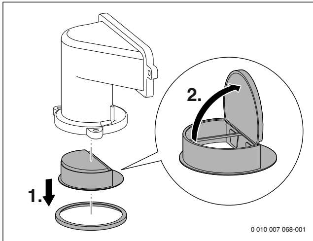
Afb. 87 Terugslagklep in de menginrichting
