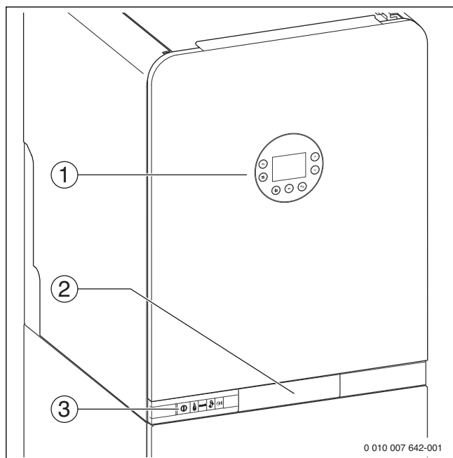
Afb. 74 Overzicht bedieningselementen
