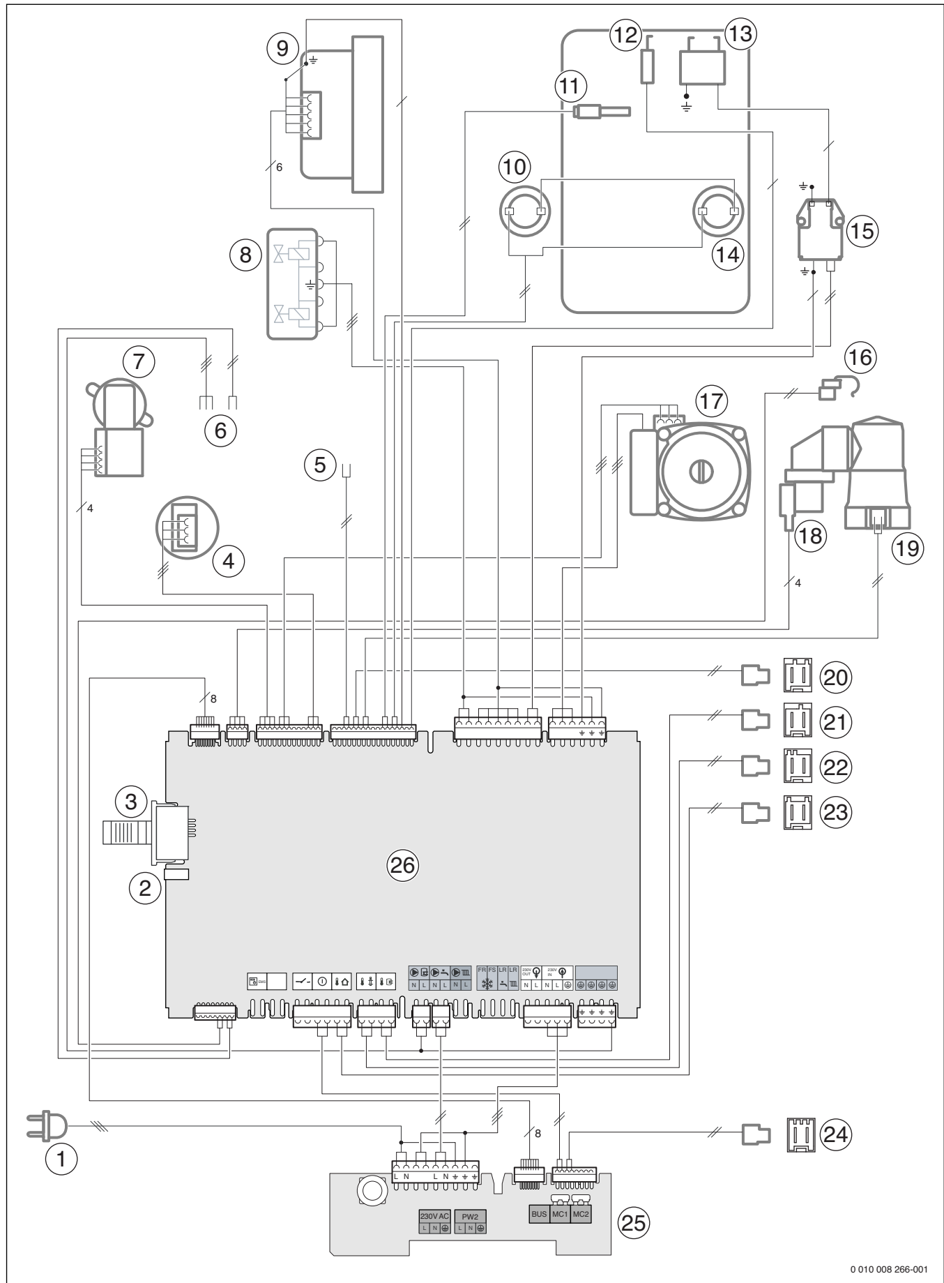
Afb. 104 Elektrische bedrading
