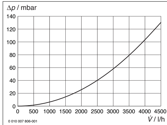
Afb. 106 Drukverliesdiagram ongemengd cv-circuit (HK1)
