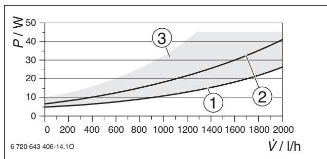
Afb. 113 Opgenomen vermogen
