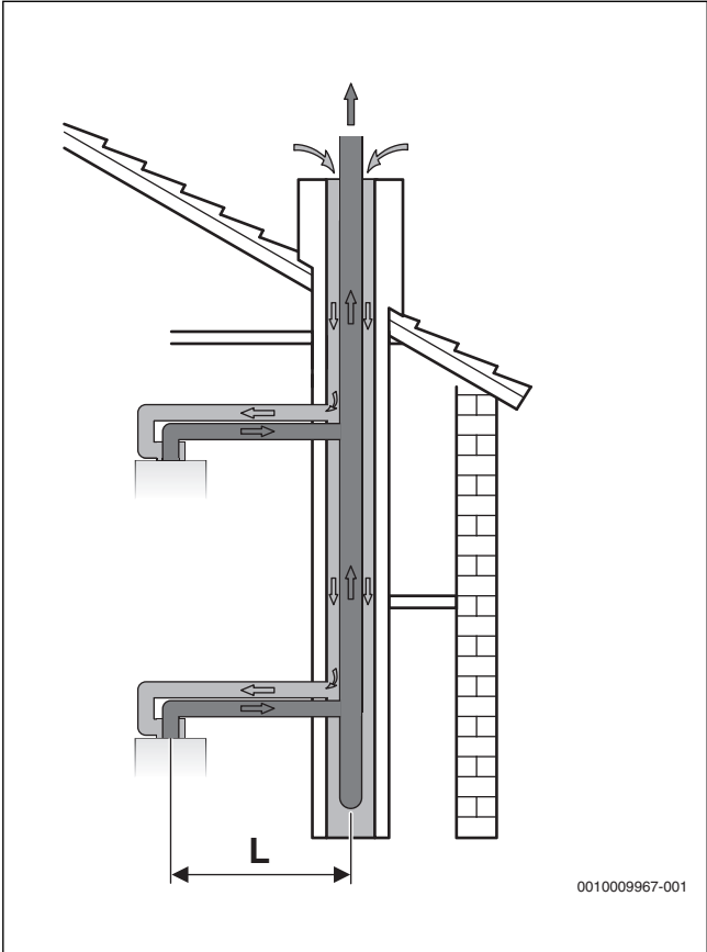
Afb. 33 Collectieve rookgasafvoer met parallelbuis conform C 43
