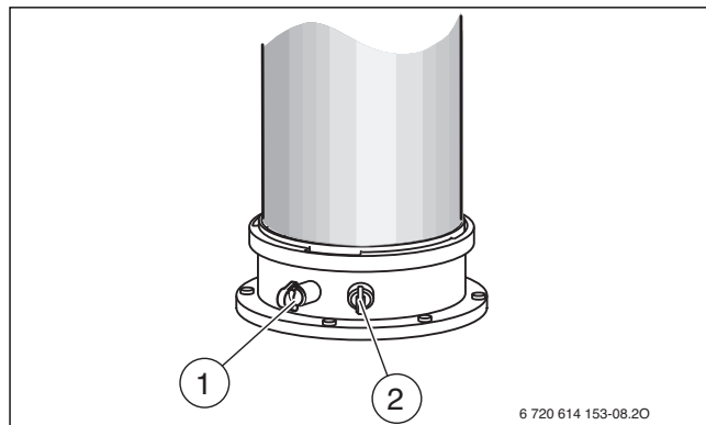
Afb. 82 Rookgasmeetpunt en verbrandingsluchtmeetpunt
