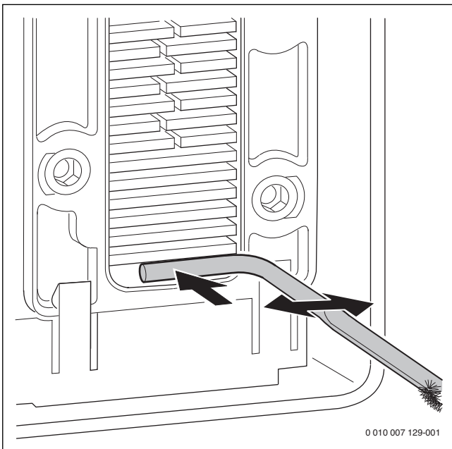
Afb. 92 Condensbak reinigen
