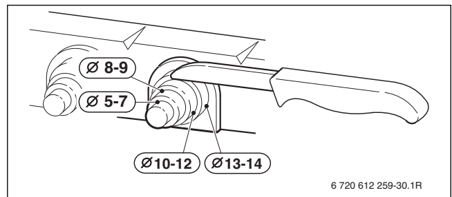
Afb. 61 Aanpassen trekcontasting aan de kabeldiameter
