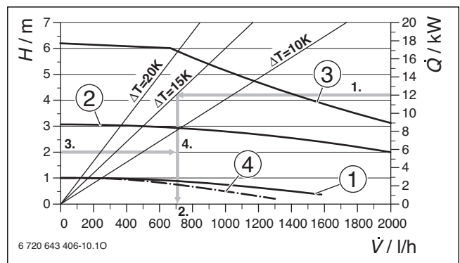
Afb. 110 Pompcurven
