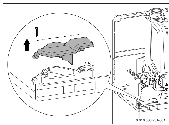
Afb. 53 Afdekking van de aansluitbox verwijderen
