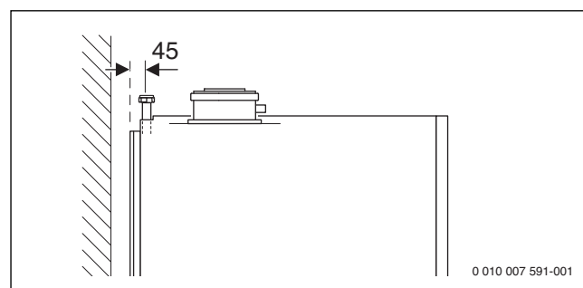
Afb. 7 Aansluitmaten van het toebehoren CS 11 - Aansluitset verticaal (maten in mm)
