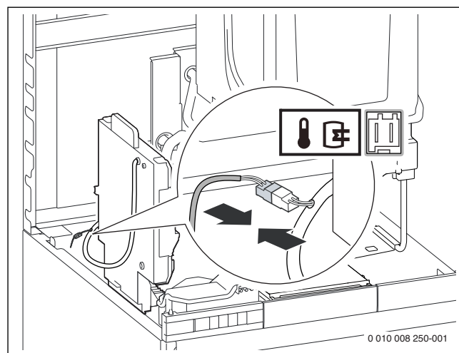
Afb. 52 Boilertemperatuursensor aansluiten
