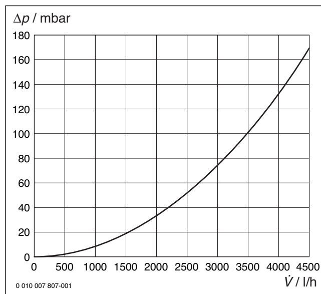
Afb. 107 Drukverliesdiagram gemengd cv-circuit (HK2)
