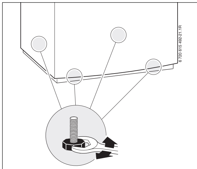
Afb. 41 Boiler uitlijnen
