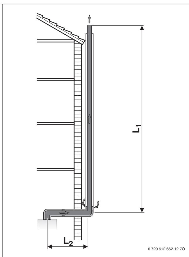
Afb. 30 Rookgasafvoersysteem op de gevel conform C 53
