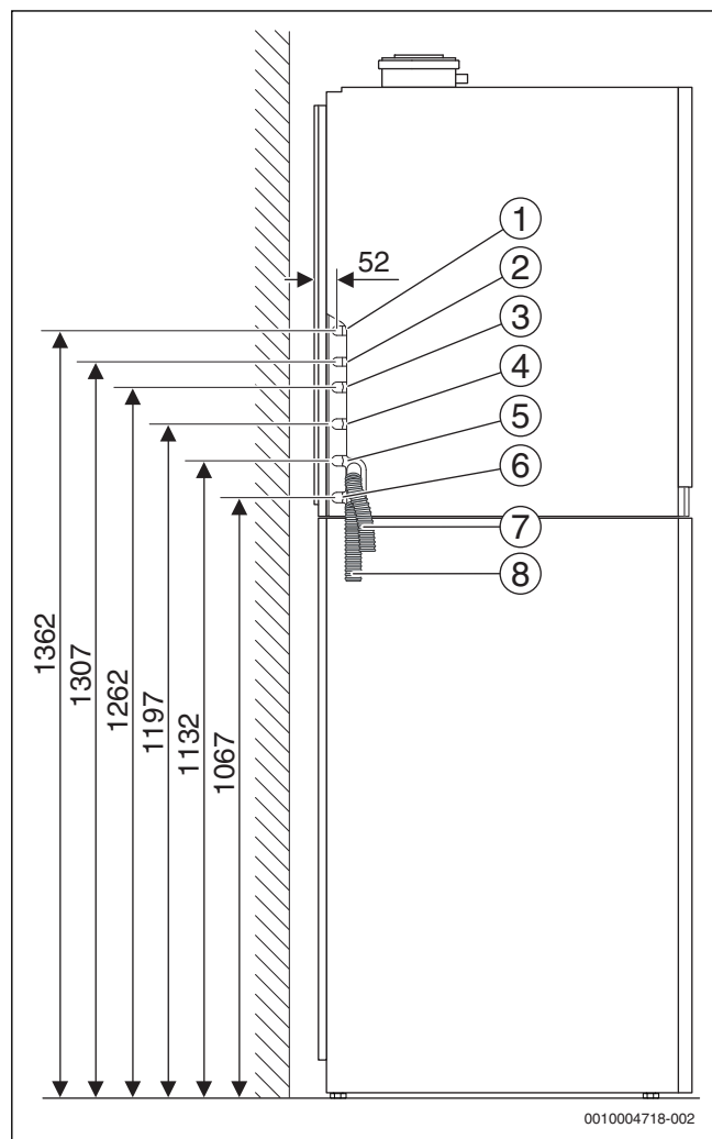
Afb. 5 Aansluitmaten van het toebehoren CS 10 - Aansluitset horizontaal (maten in mm)
