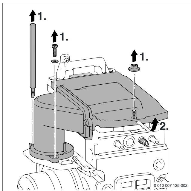
Afb. 85 Branderdeksel losmaken
