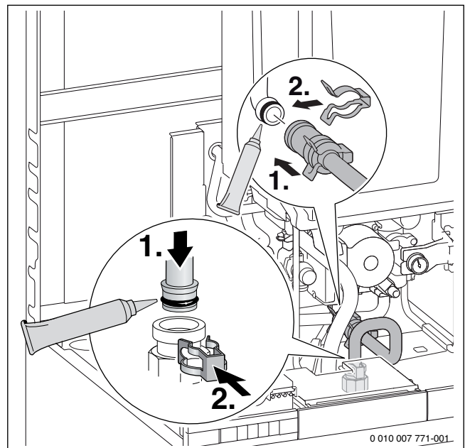
Afb. 49 Buisverbinding tussen boilerretour en ketelblok maken
