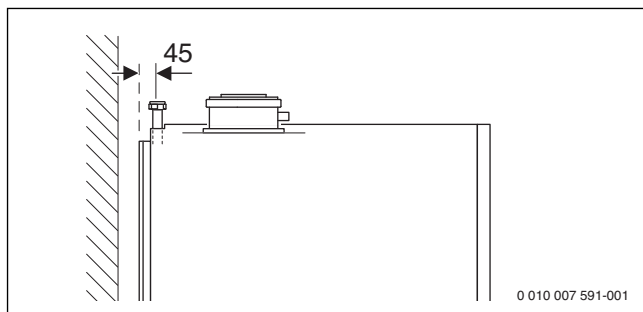
Afb. 13 Aansluitmaten van het toebehoren CS 14 - Aansluitset verwarmingsondersteuning (maten in mm)
