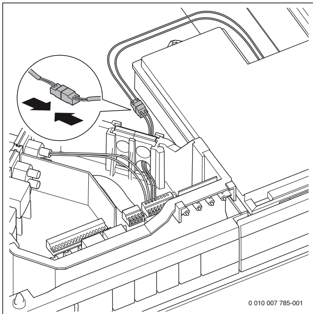
Afb. 56 Schuiflade voor de regelaar op de aansluitbox aansluiten
