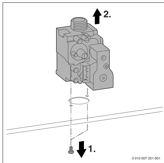
Afb. 100 Gasblok demonteren
