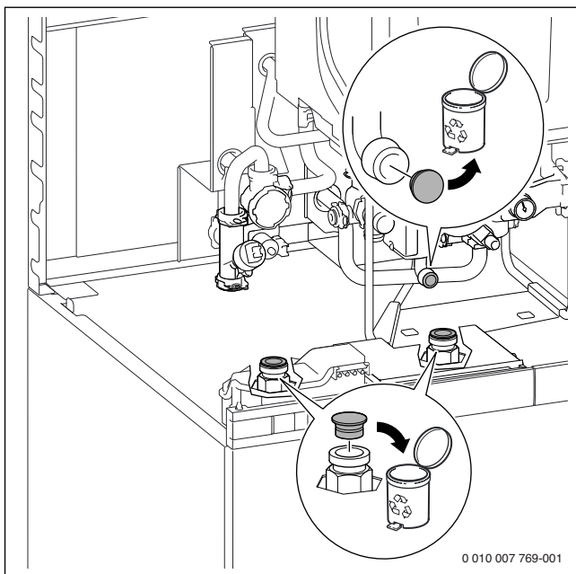
Afb. 47 Stop op ketelblok en op de boileraanvoer en -retour verwijderen
