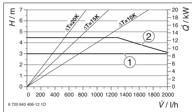
Afb. 114 Pompcurven
