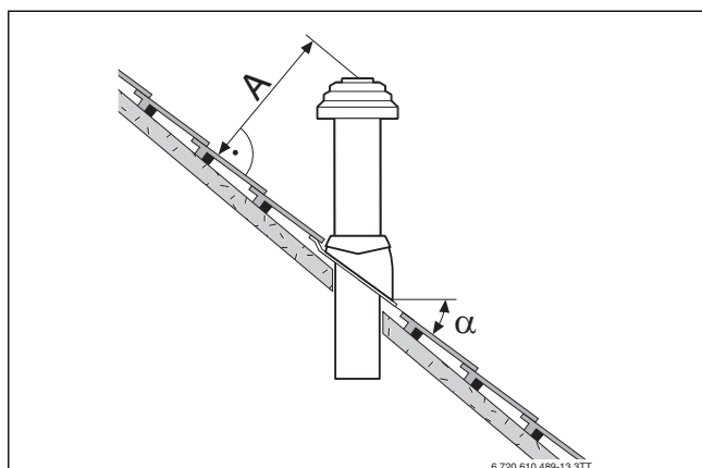
Afb. 21 Afstandsmaten en dakhellingen bij schuin dak
