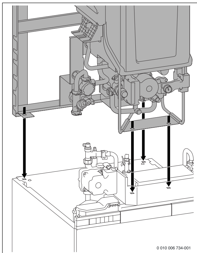
Afb. 44 Ketel op de boiler plaatsen
