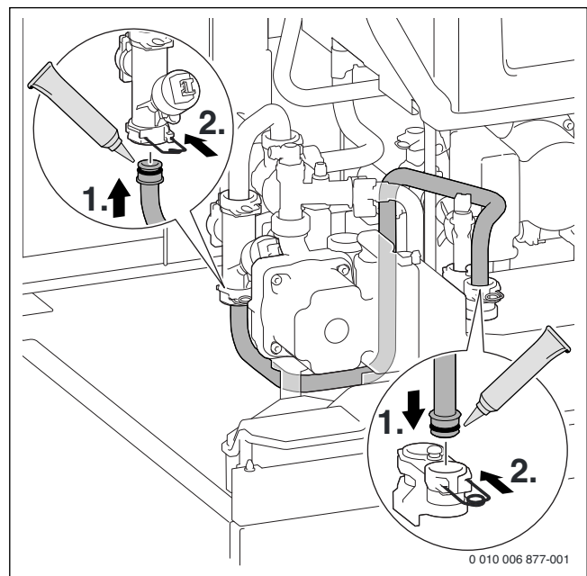
Afb. 50 Leidingverbinding tussen 3-wegklep en platenwarmtewisselaar uitvoeren (aanvoer)
