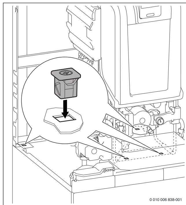
Afb. 45 Ketel met de 4 meegeleverde clips op de boiler fixeren
