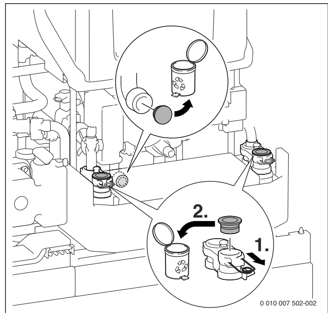
Afb. 49 Stop op verwarmingslichaam en op de platenwarmtewisselaar verwijderen
