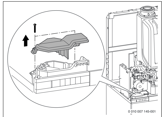
Afb. 62 Afdekking van de aansluitbox verwijderen
