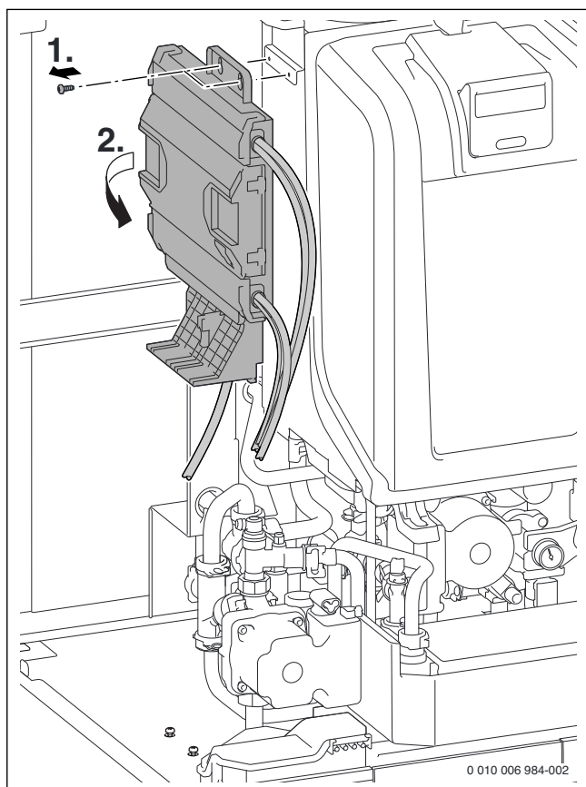
Afb. 52 Besturing afnemen
