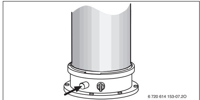
Afb. 82 Rookgasmeetpunt
