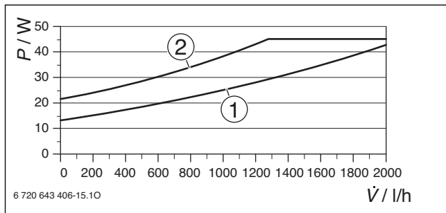
Afb. 118 Opgenomen vermogen
