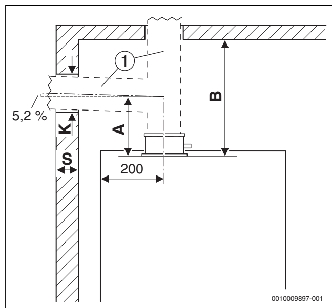
Afb. 16 Afmetingen
