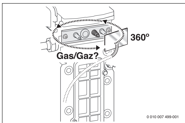
Afb. 86 Op lekken controleren
