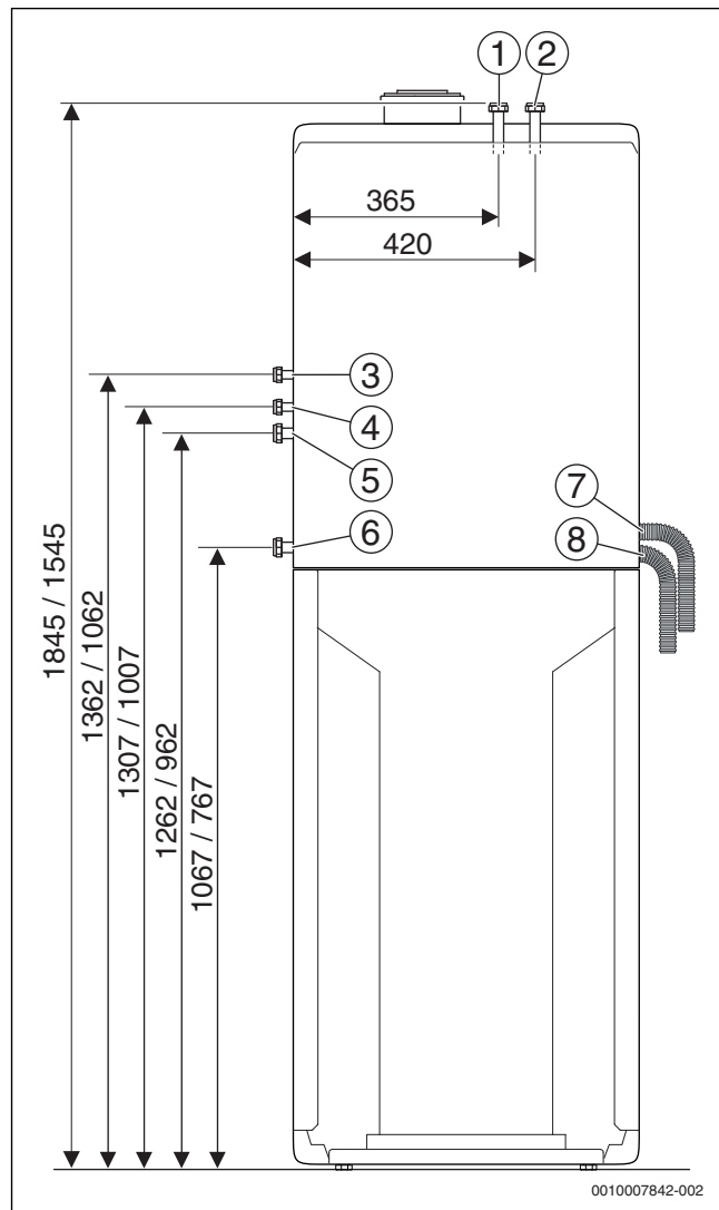
Afb. 8 Aansluitmaten van het toebehoren CS 12 - Uitbreidingset 1 cv-kring (maten in mm)
