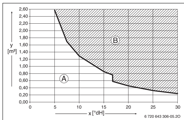
Afb. 36 Eisen aan het vul- en bijvulwater voor ketels < 50 kW
