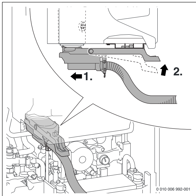
Afb. 47 Vuilfilter monteren
