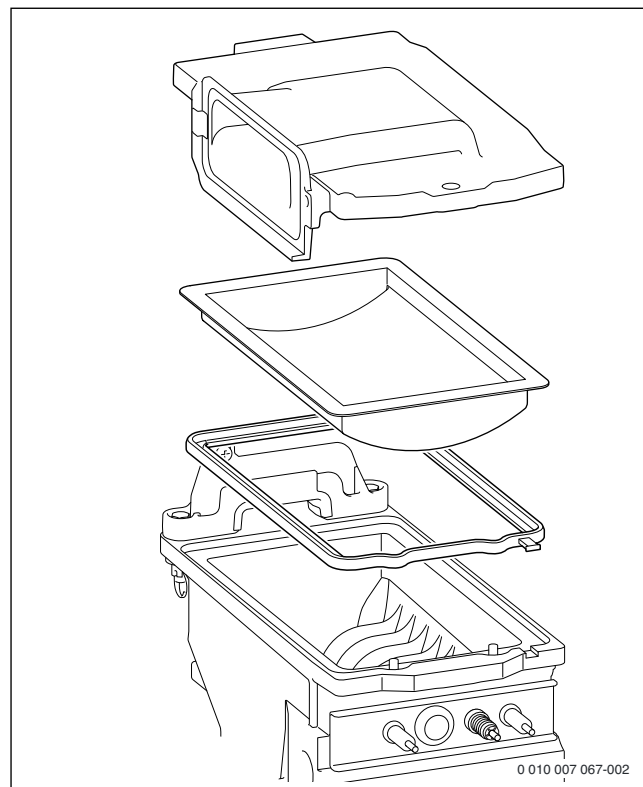
Afb. 88 Brander
