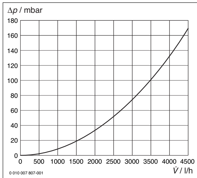
Afb. 110 Drukverliesdiagram gemengd cv-circuit (HK2)
