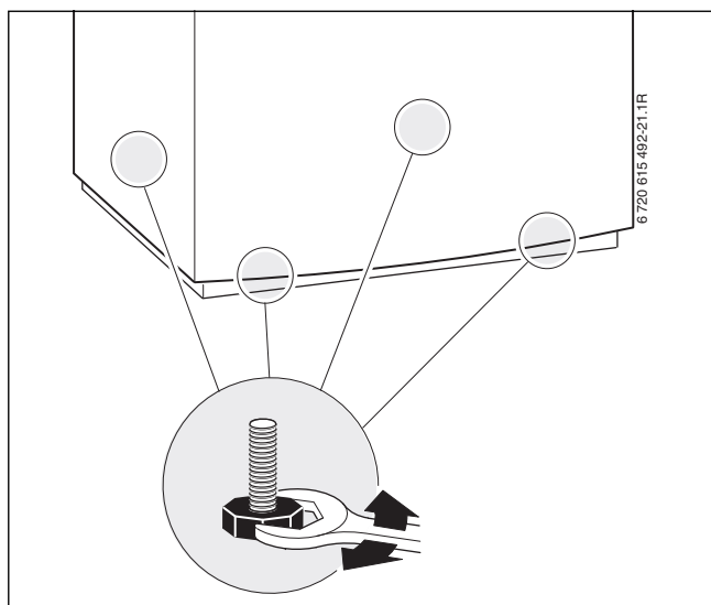
Afb. 43 Boiler uitlijnen
