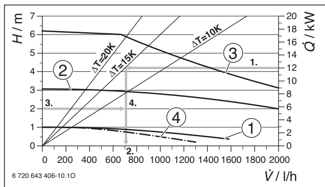
Afb. 113 Pompcurven
