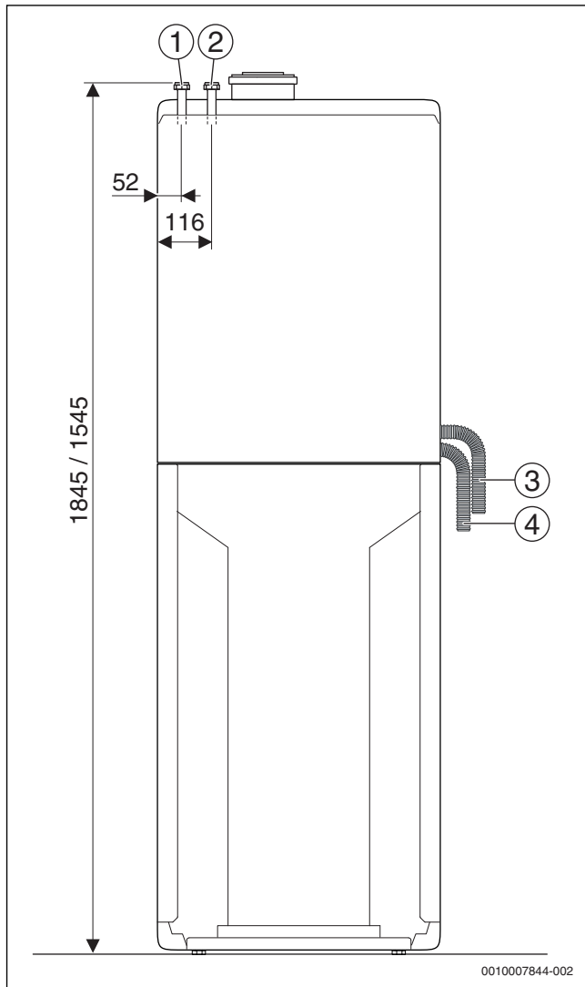
Afb. 12 Aansluitmaten van het toebehoren CS 14 - Aansluitset verwarmingsondersteuning (maten in mm)
