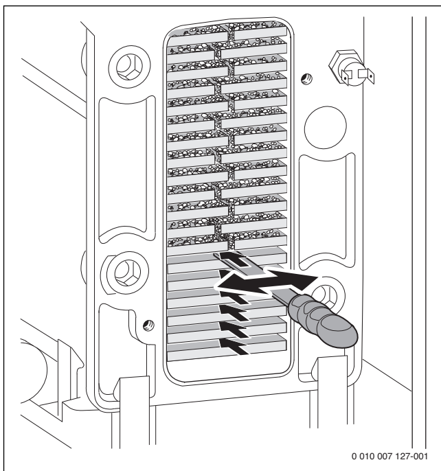
Afb. 91 Reinigingsgereedschap
