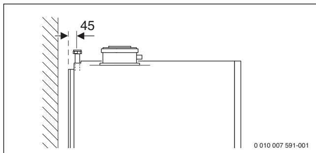
Afb. 13 Aansluitmaten van het toebehoren CS 14 - Aansluitset verwarmingsondersteuning (maten in mm)
