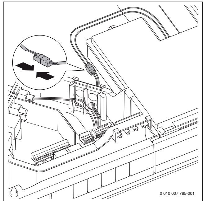
Afb. 59 Schuiflade voor de regelaar op de aansluitbox aansluiten
