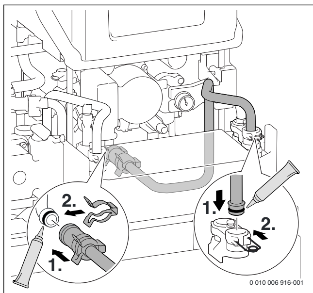
Afb. 51 Leidingverbinding tussen platenwarmtewisselaar en verwarmingslichaam uitvoeren (retour)
