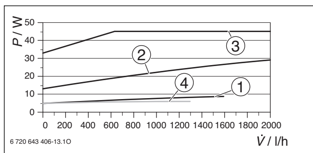
Afb. 114 Opgenomen vermogen
