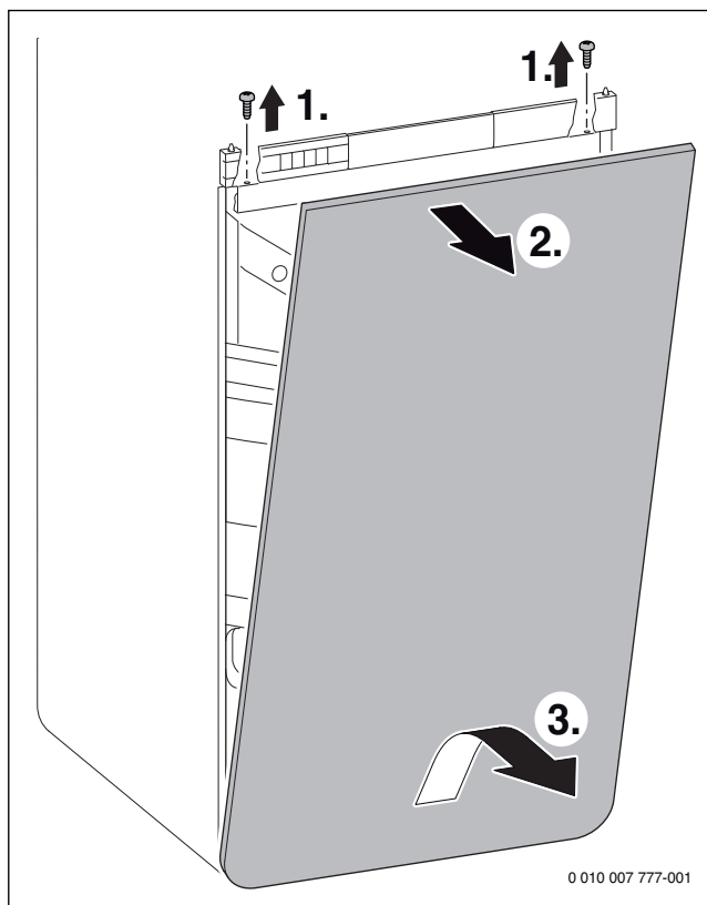
Afb. 42 Voorste mantel van de boiler afnemen
