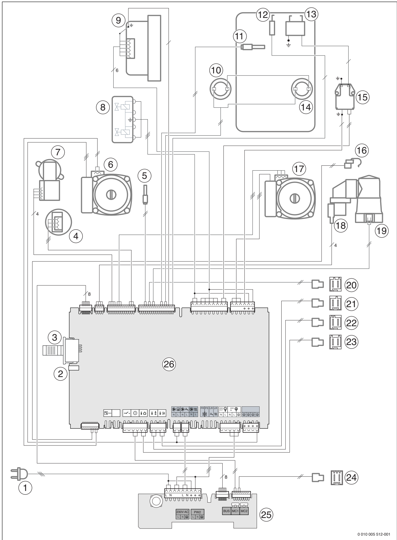
Afb. 107 Elektrische bedrading
