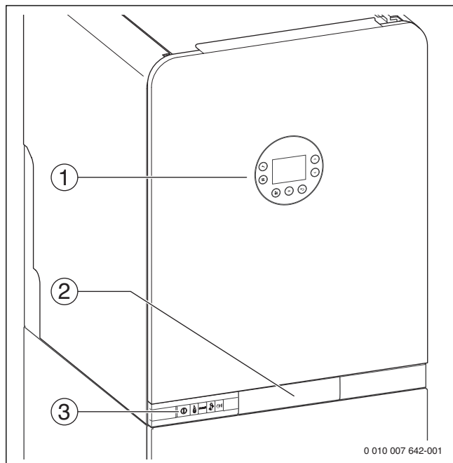
Afb. 76 Overzicht bedieningselementen
