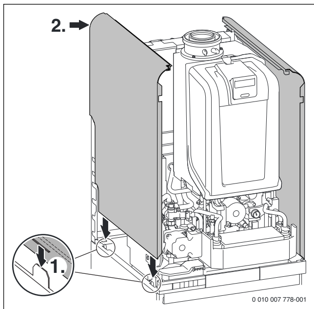
Afb. 73 Rechter- en linkermantel monteren
