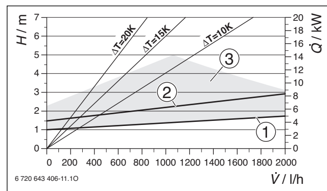
Afb. 115 Pompcurven
