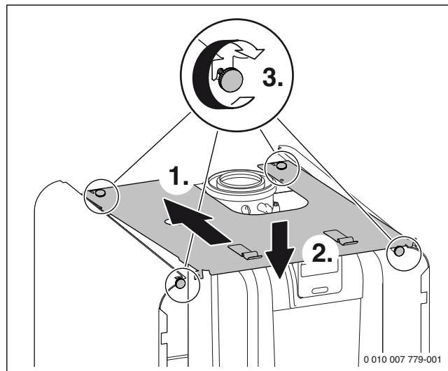
Afb. 74 Bovenste mantel naar achteren schuiven en met de 4 schroeven voor en achter bevestigen
