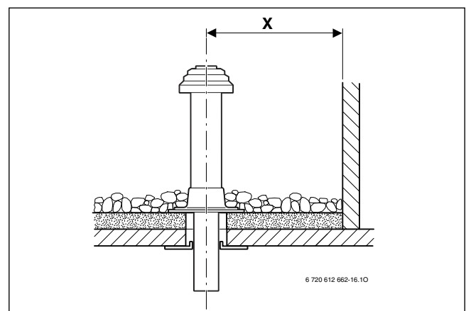
Afb. 20 Afstandsmaten bij plat dak
