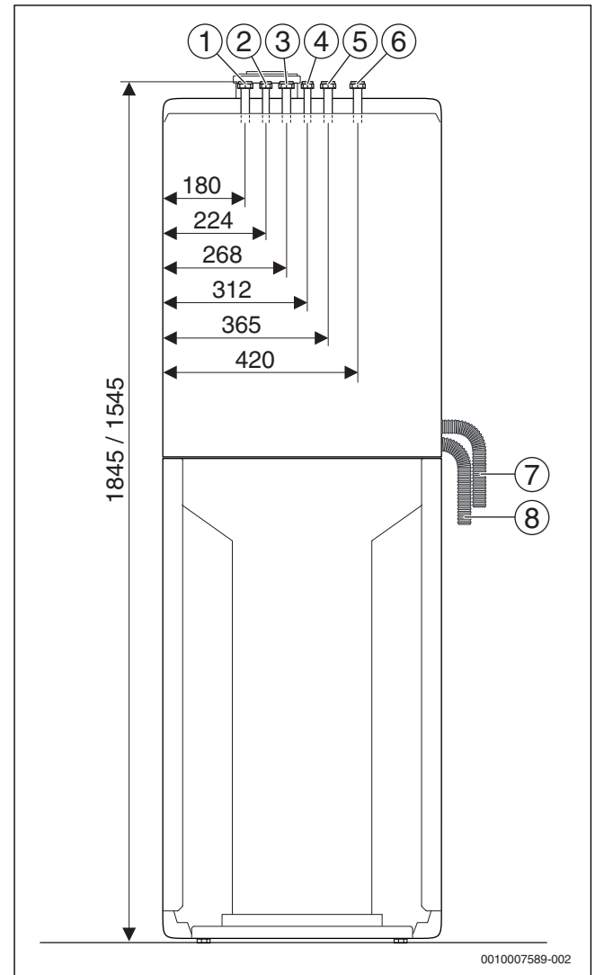
Afb. 6 Aansluitmaten van het toebehoren CS 11 - Aansluitset verticaal (maten in mm)
