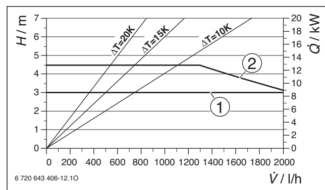
Afb. 117 Pompcurven
