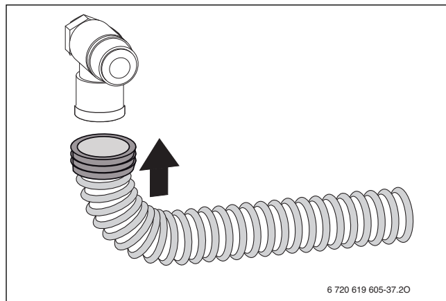
Afb. 38 Monteer de slang op het overstortventiel
