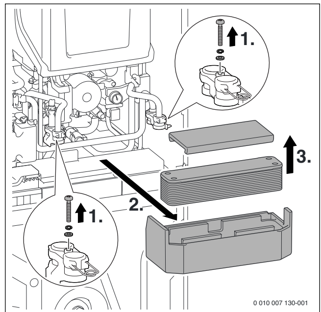
Afb. 99 Platenwarmtewisselaar demonteren
