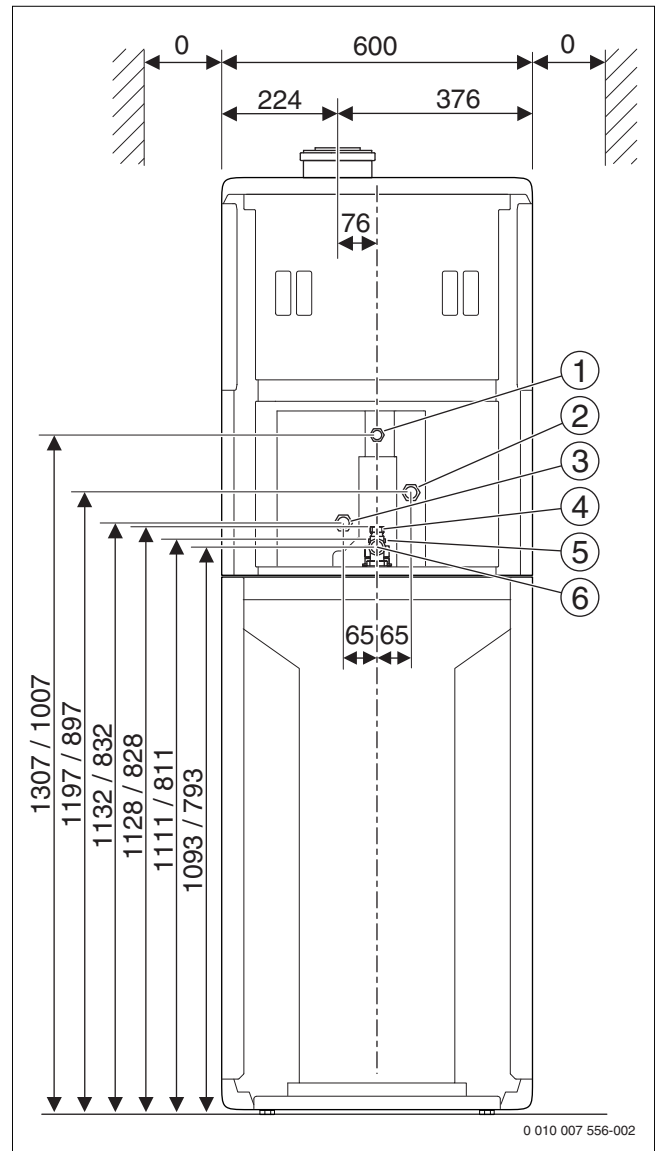
Afb. 3 Afmetingen en aansluitingen zonder toebehoren (afmetingen in mm) (aanbevolen wandafstand ≥ 50 mm)
