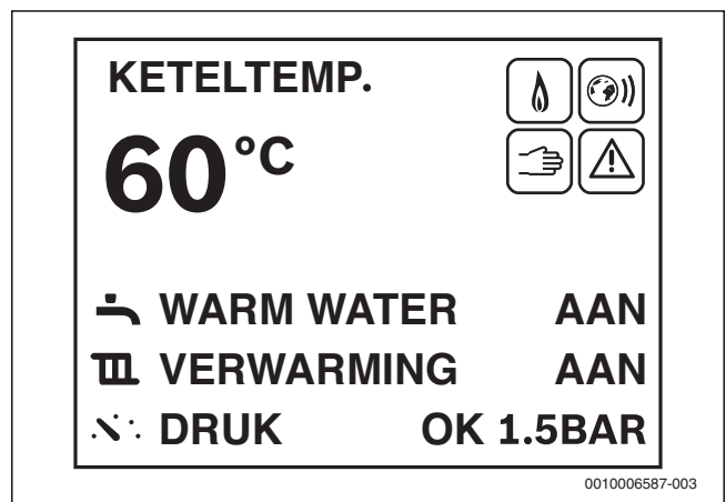
Afb. 79 standaardweergave
