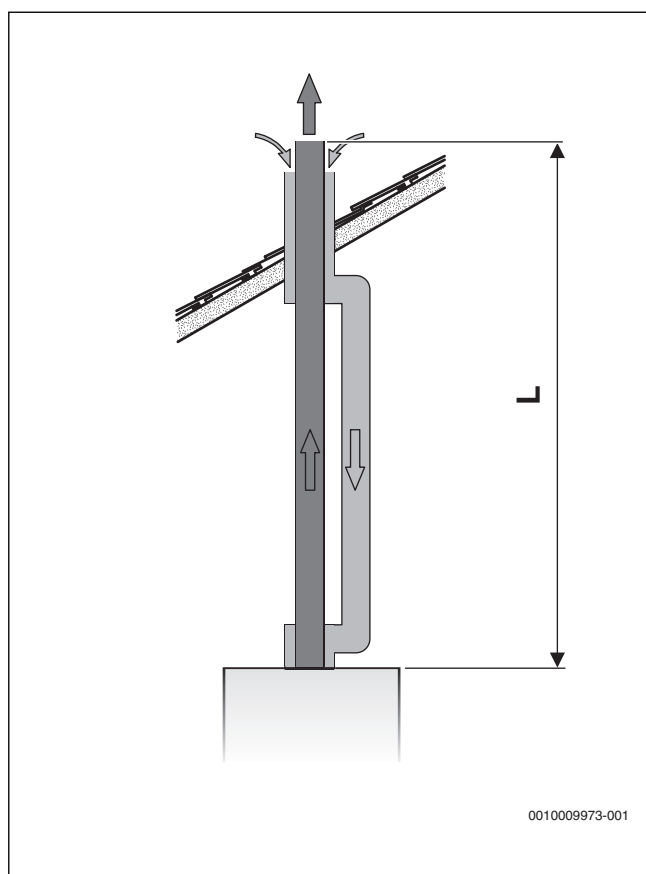
Afb. 30 Rookgasafvoer verticaal conform C 33
