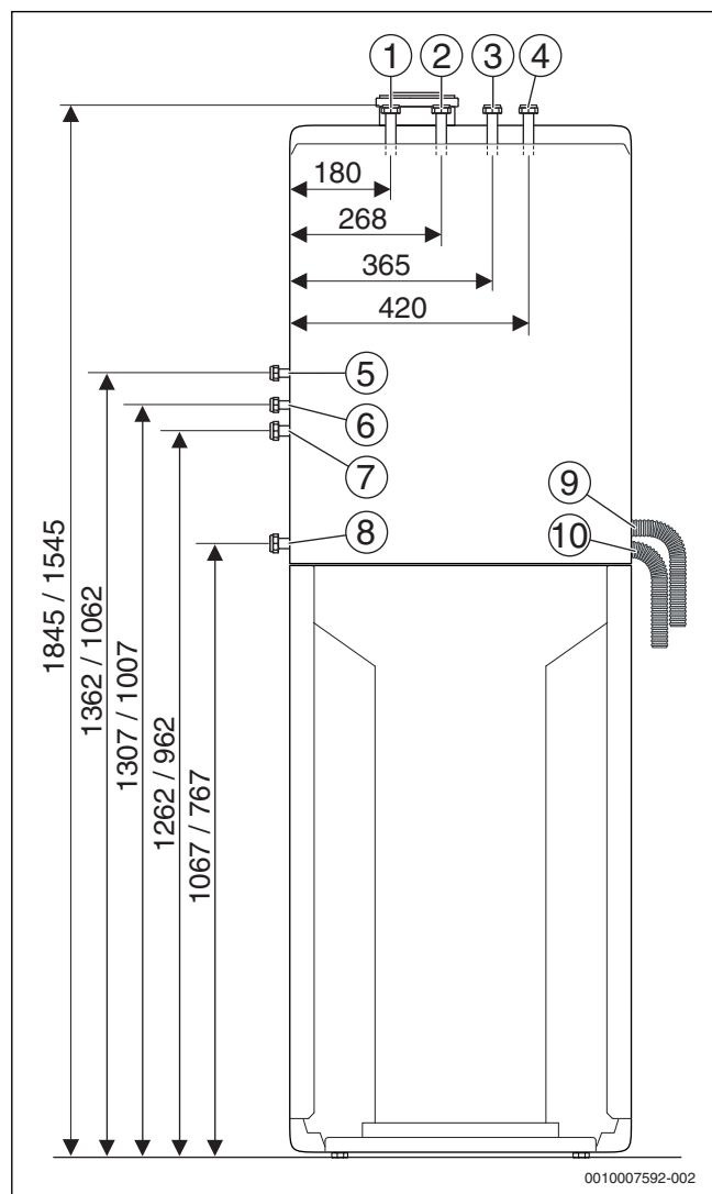
Afb. 10 Aansluitmaten van het toebehoren CS 13 - Uitbreidingset 2 cv-kringen (maten in mm)
