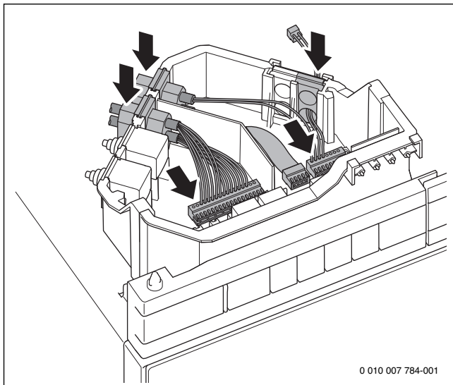
Afb. 57 Besturing op de aansluitbox aansluiten
