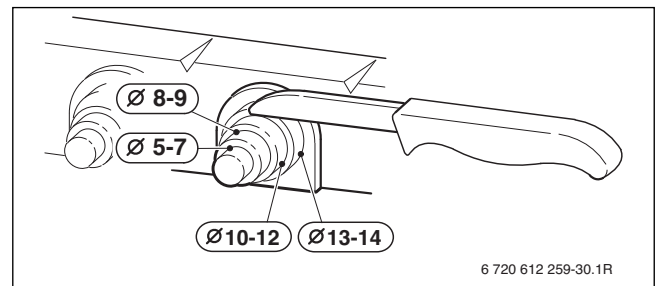
Afb. 63 Aanpassen trekcontasting aan de kabeldiameter
