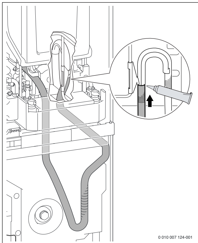
Afb. 48 Sifonslang op eindstuk steken
