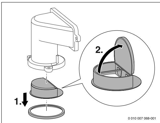
Afb. 98 Terugslagklep in de menginrichting
