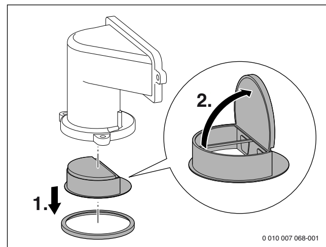
Afb. 89 Terugslagklep in de menginrichting
