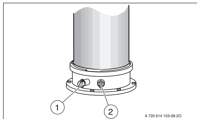
Afb. 84 Rookgasmeetpunt en verbrandingsluchtmeetpunt
