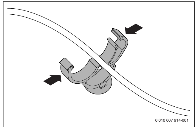
Afb. 58 Kabel met de clips bevestigen
