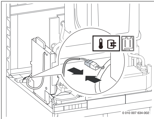
Afb. 55 Boilertemperatuursensor aansluiten
