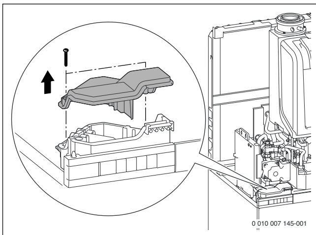
Afb. 56 Afdekking van de aansluitbox verwijderen
