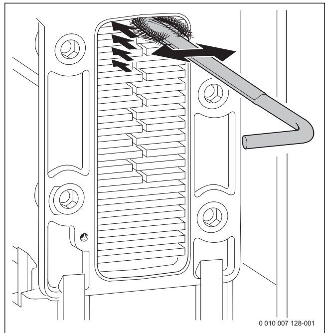
Afb. 92 Warmtewisselaar met borstel reinigen
