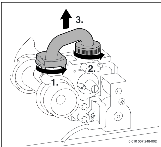
Afb. 101 Gasleiding demonteren
