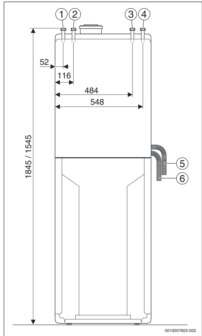
Afb. 14 Aansluitmaten van het toebehoren CS 15 - Aansluitset verwarmingsondersteuning door solarsysteem (maten in mm)
