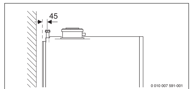
Afb. 7 Aansluitmaten van het toebehoren CS 11 - Aansluitset verticaal (maten in mm)
