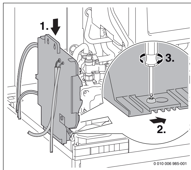
Afb. 53 Besturing op de boiler bevestigen
