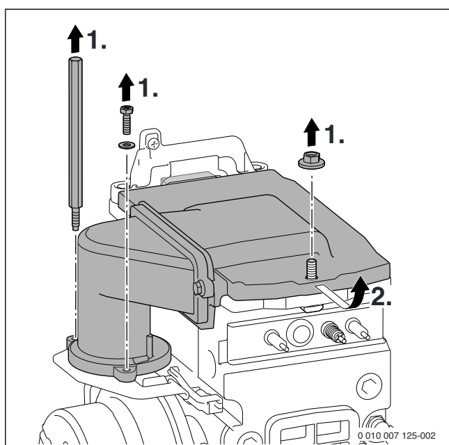
Afb. 87 Branderdeksel losmaken
