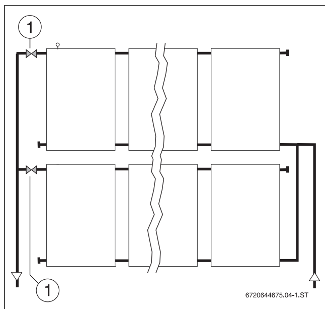
Afb. 69 Spoelen van parallel geschakelde collectorvelden
