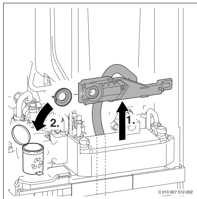
Afb. 46 Vuilfilter uit de onderhoudspositie nemen en beschermdeksel afnemen
