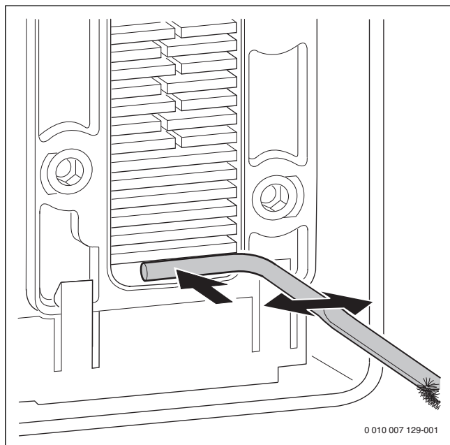
Afb. 94 Condensbak reinigen
