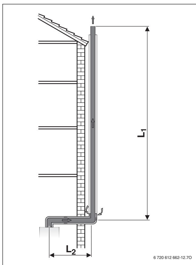
Afb. 31 Rookgasafvoersysteem op de gevel conform C 53
