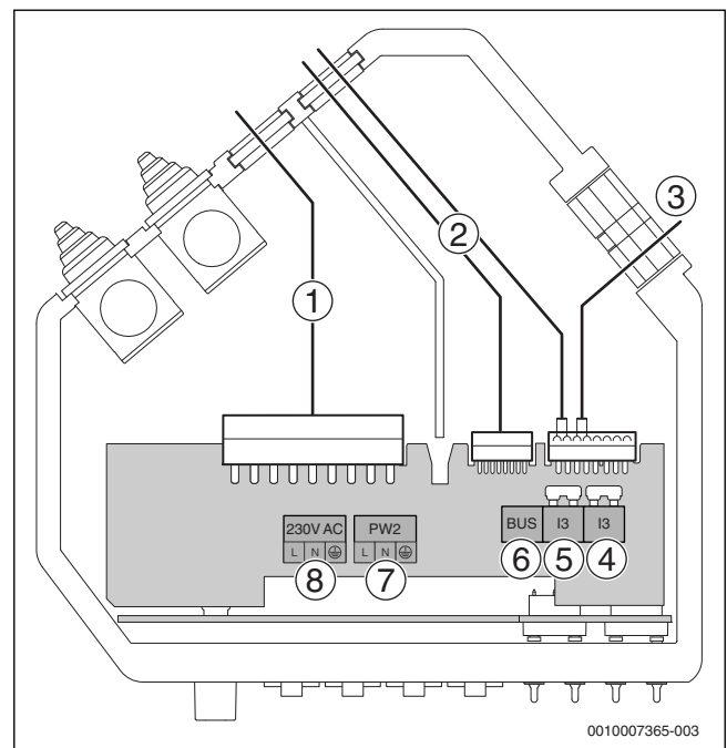
Afb. 64 Aansluitbox
