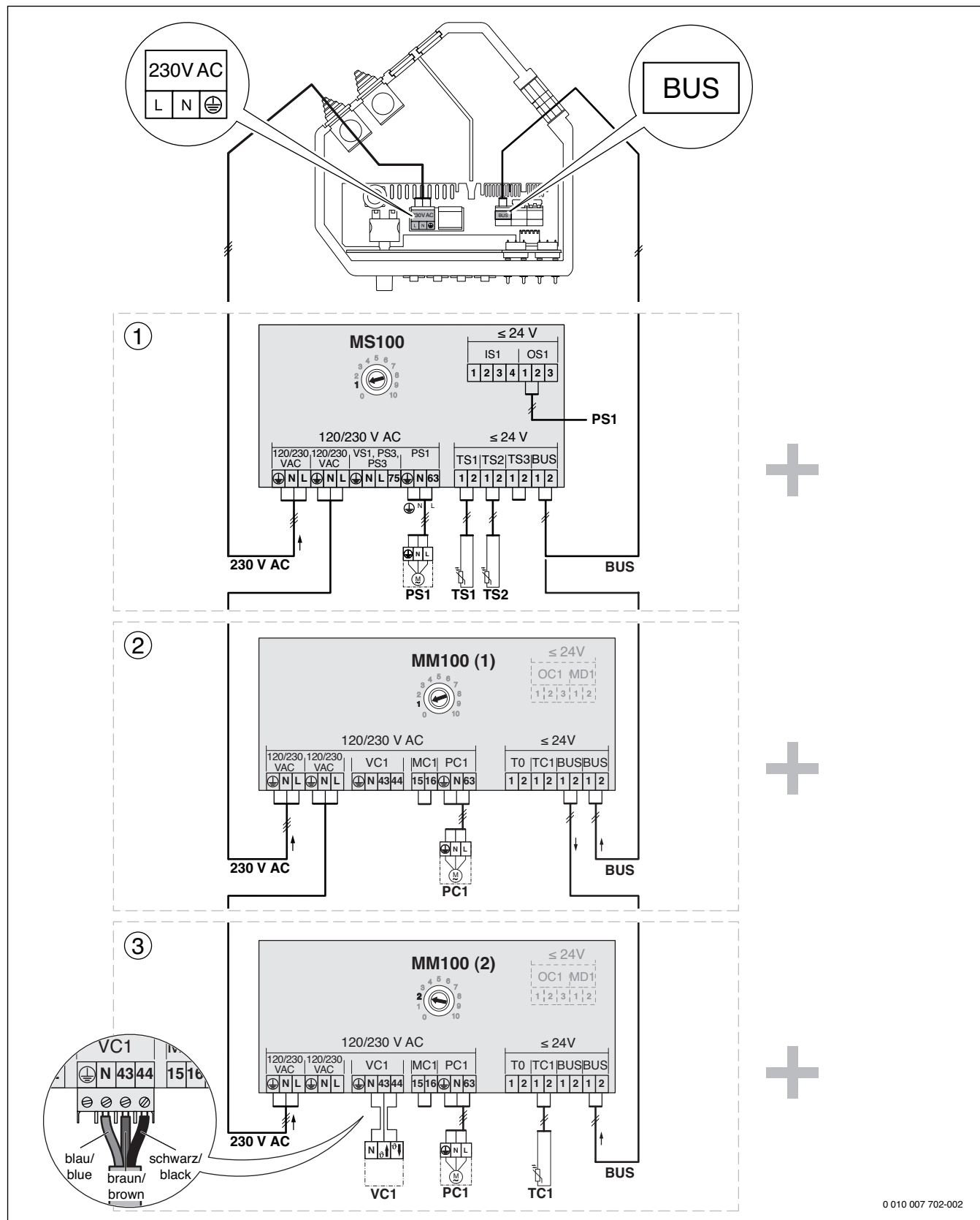
Afb. 65 Aansluiting van de module MS 100 en MM 100, indien aanwezig
