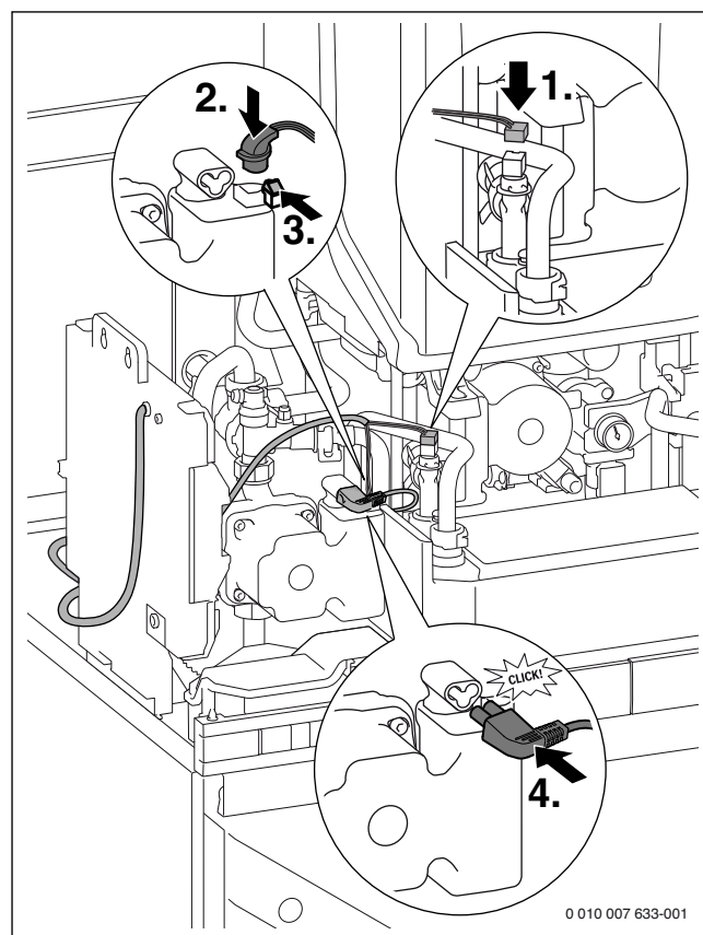
Afb. 54 Boilerlaadpomp en warmwatertemperatuursensor aansluiten
