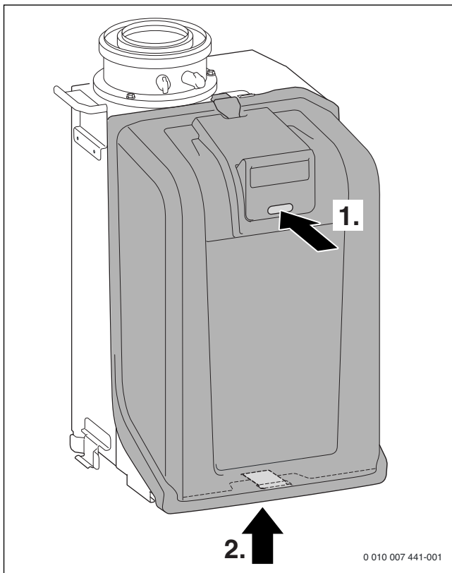
Afb. 81 Branderkap verwijderen
