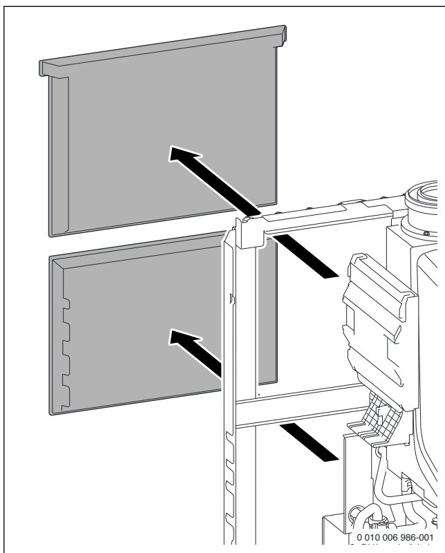
Afb. 60 Warmte-isolatie aan de achterzijde afnemen
