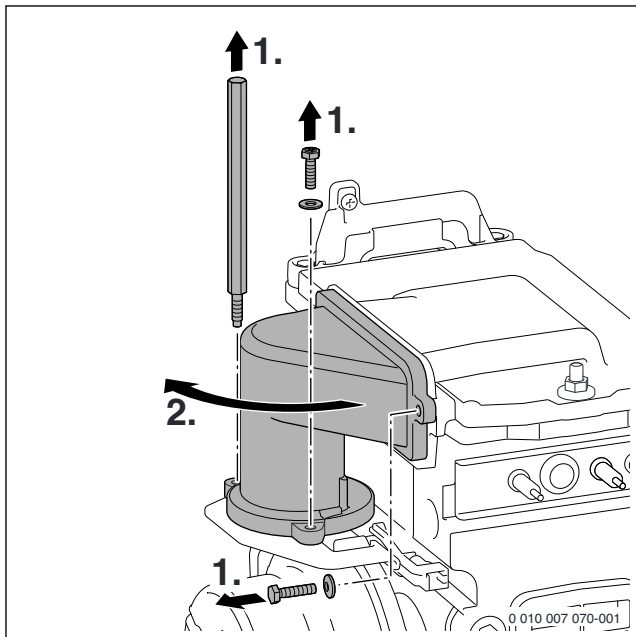
Afb. 97 Demonteer de menginrichting
