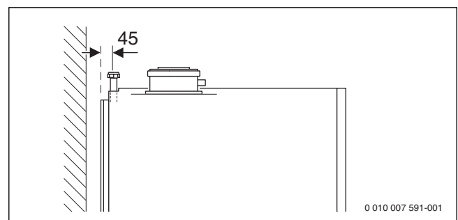
Afb. 15 Aansluitmaten van het toebehoren CS 15 - Aansluitset verwarmingsondersteuning door solarsysteem (maten in mm)
