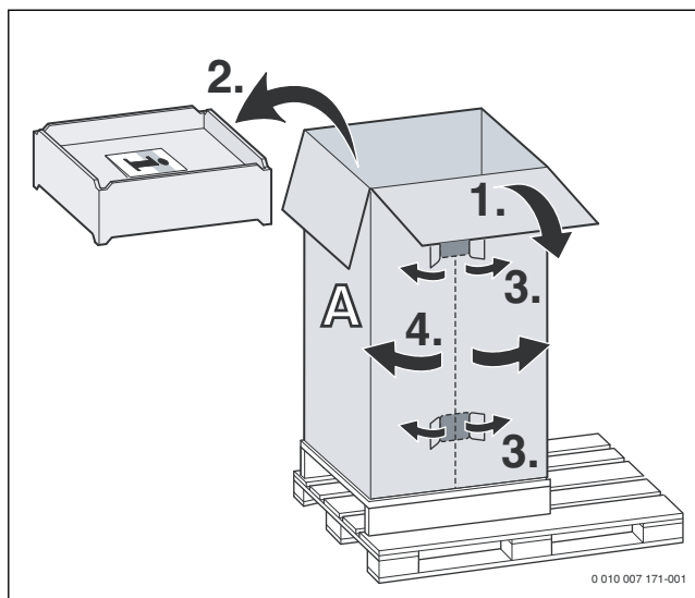
Afb. 41 Boiler uitpakken
