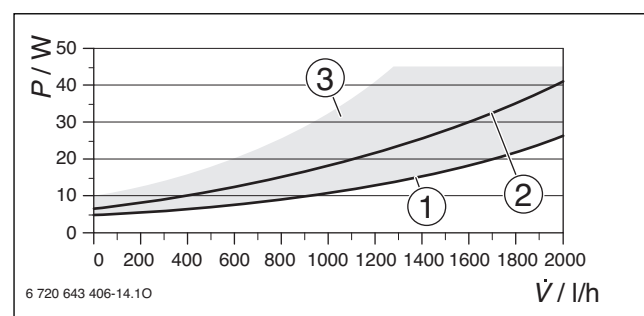
Afb. 116 Opgenomen vermogen
