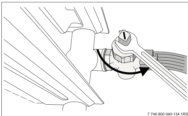
Afb. 38 Installatie bij vorstgevaar aftappen
