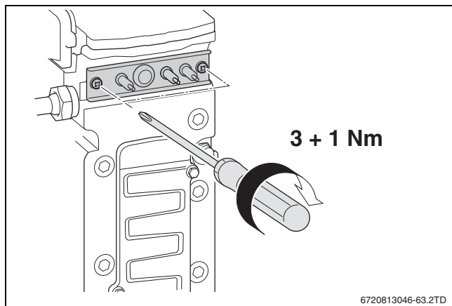
Afb. 39 Elektrodenset inbouwen
