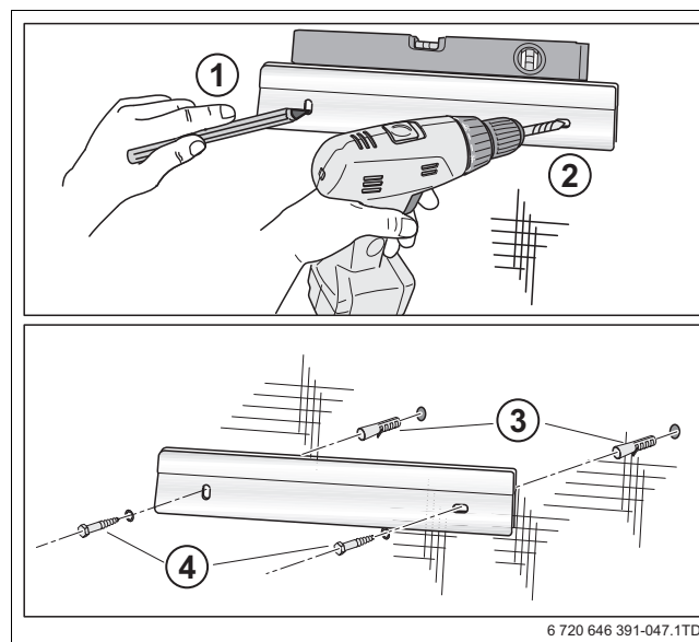
Afb. 13 Steun monteren
