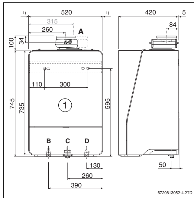
Afb. 5 Afmetingen en aansluitingen [mm] 1) servicematen, ingebouwd in kast, kan 0 mm zijn.
