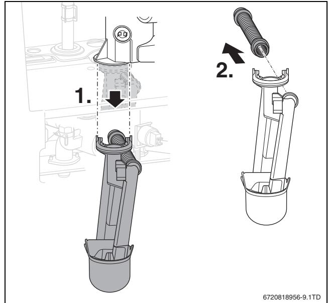
Afb. 44 Condenssifon
