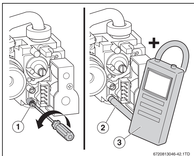
Afb. 29 Gasaansluitdruk meten
