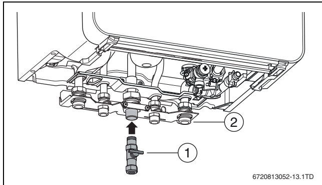
Afb. 16 Gasaansluiting uitvoeren
