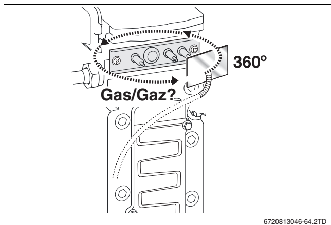
Afb. 40 Dichtheidscontrole
