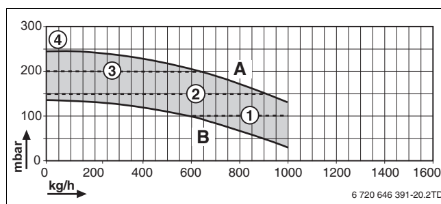
Afb. 7 Restopvoerhoogte bij GC9000iW 20 E
