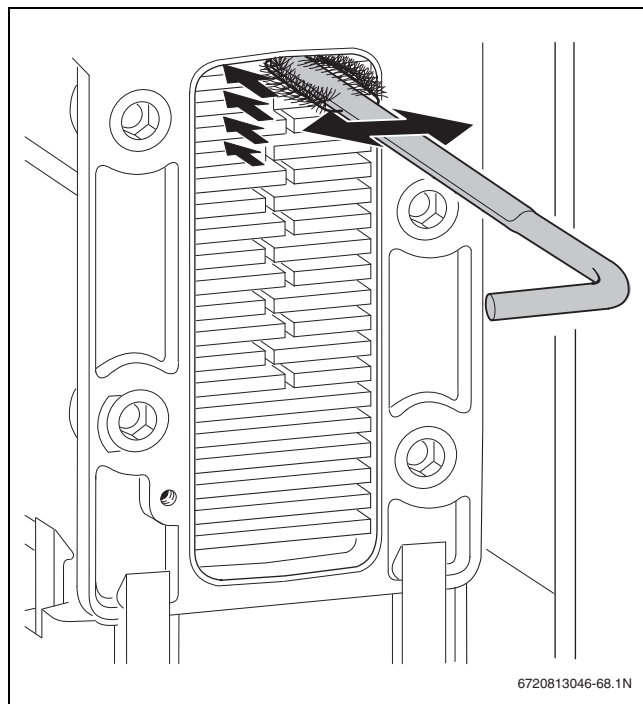
Afb. 47 Warmtewisselaar met borstel reinigen
