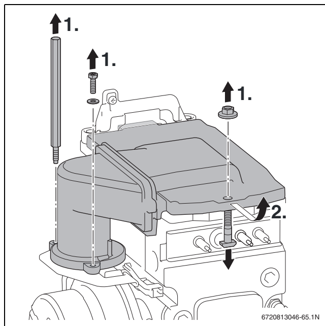
Afb. 41 Branderdeksel demonteren
