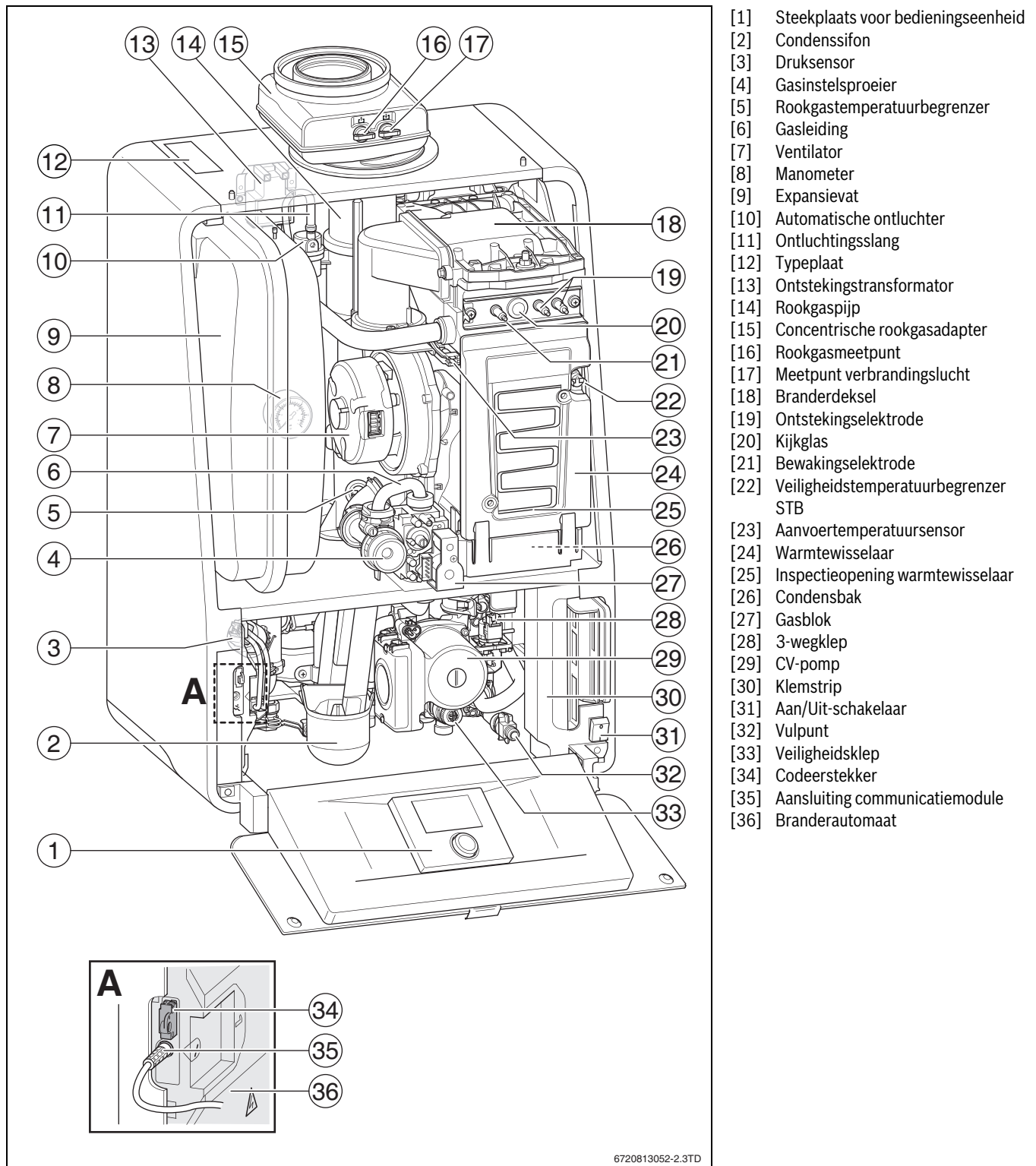
Afb. 2 GC9000iW 20 E/30 E(B)
