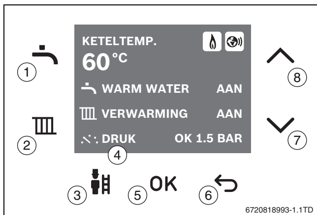
Afb. 31 Bedieningspaneel
