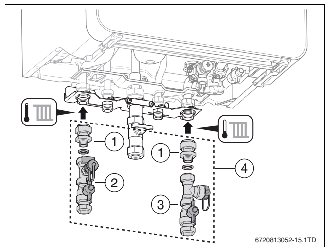
Afb. 18 Aansluiten cv-leidingen op de ketel
