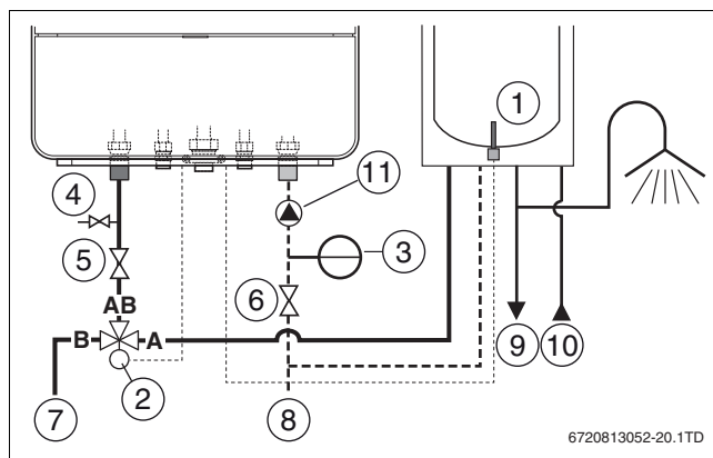
Afb. 21 Externe 3-wegklep monteren (230 V)
