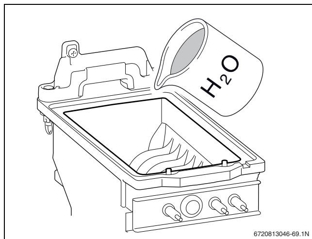
Afb. 48 Spoelen
