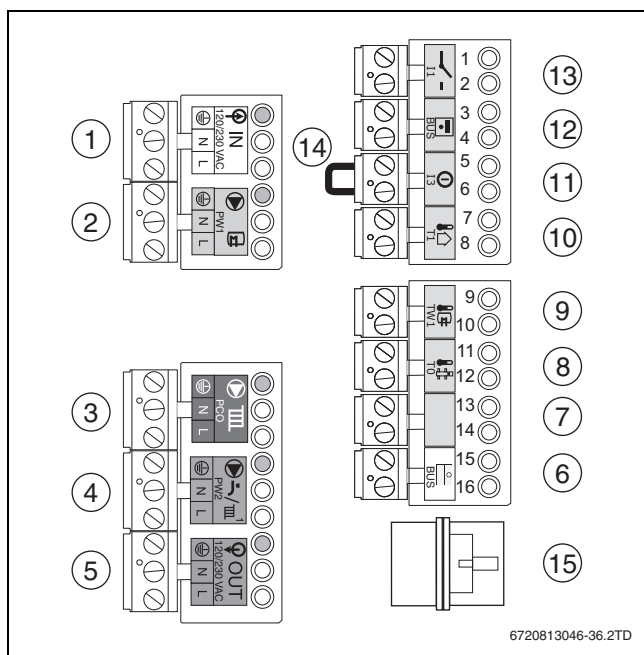
Afb. 26 Klemmenstroken
