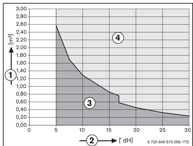
Afb. 12 Eisen aan het vul- en bijvulwater voor ketels < 50 kW
