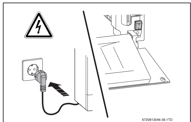
Afb. 28 Inschakelen netspanning
