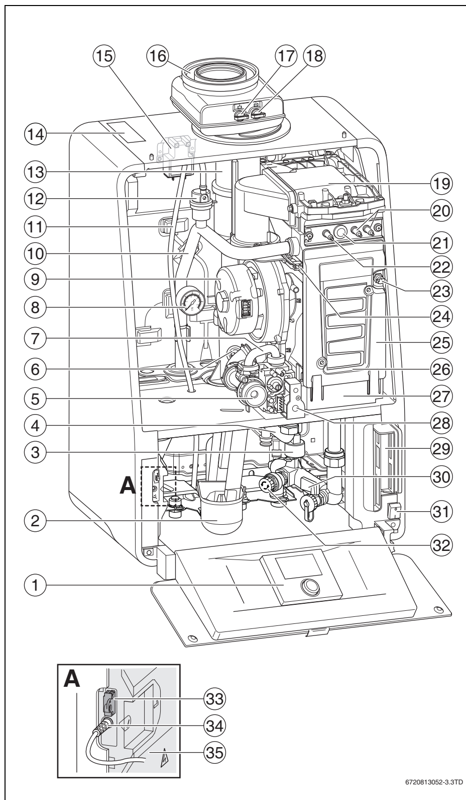
Afb. 3 GC9000iW 45
