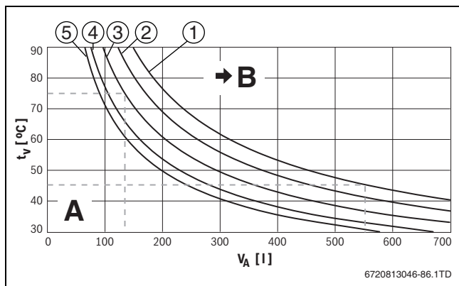
Afb. 19 Diagram van het expansievat, expansievat 14 l
