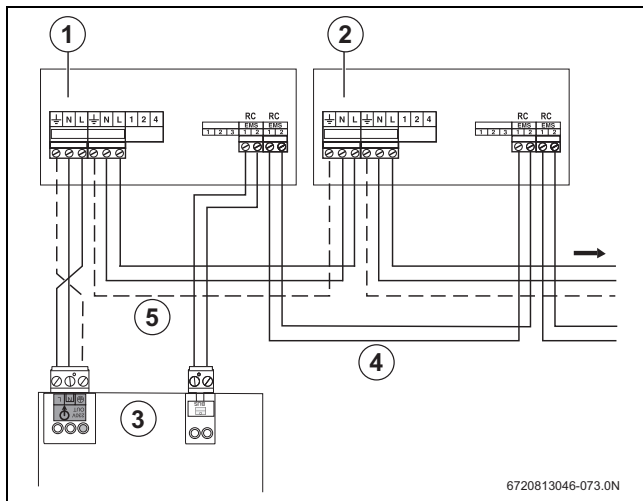
Afb. 27 Aansluiten meerdere functiemodules
