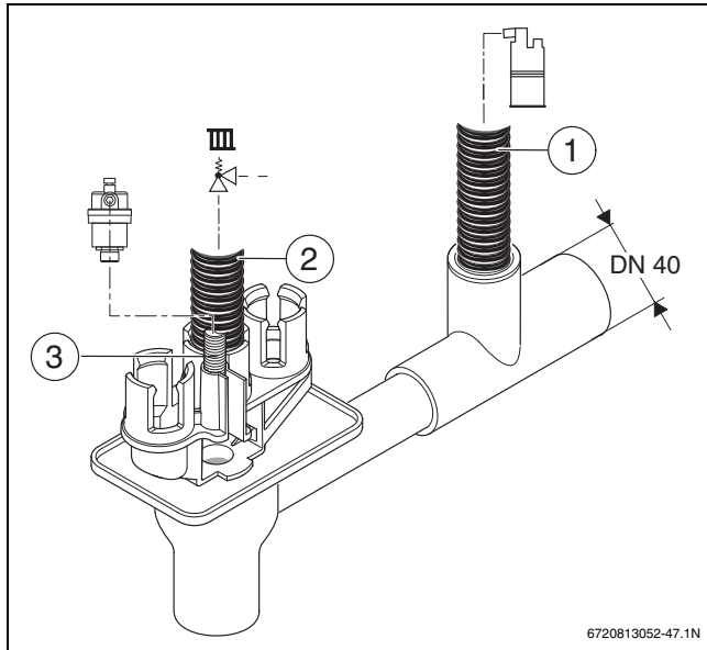
Afb. 22 Monteer de condensslang en de slang van het overstortventiel en ontlufter
