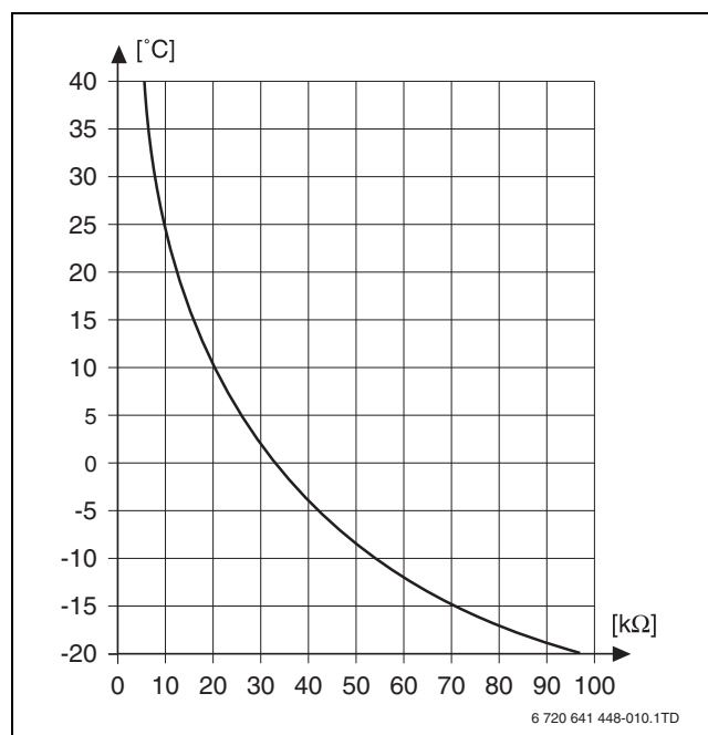
Afb. 10 Weerstandsgrafiek buitentemperatuursensor
