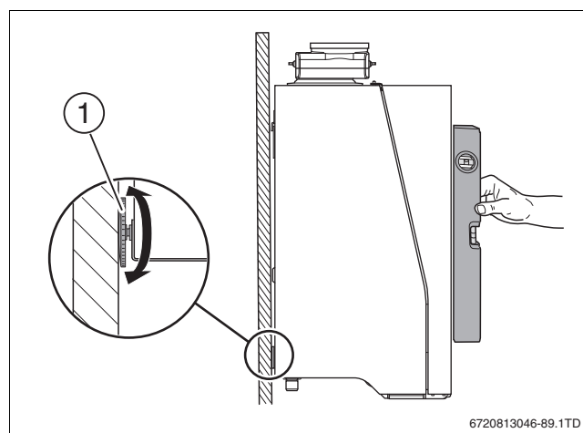
Afb. 14 Ketel uitrichten
