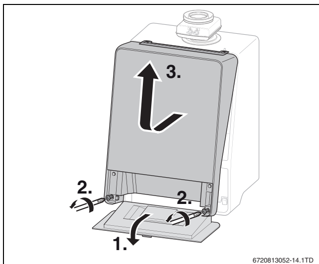
Afb. 17 Demonteer de mantel van de ketel
