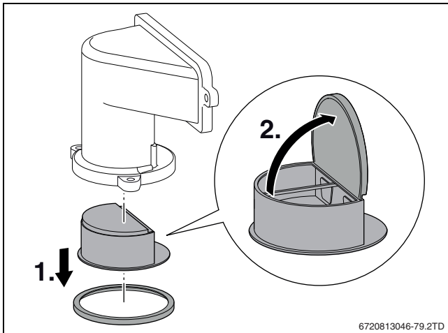
Afb. 43 Terugslagklep in de menginrichting
