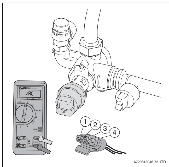
Afb. 50 3-wegklep
