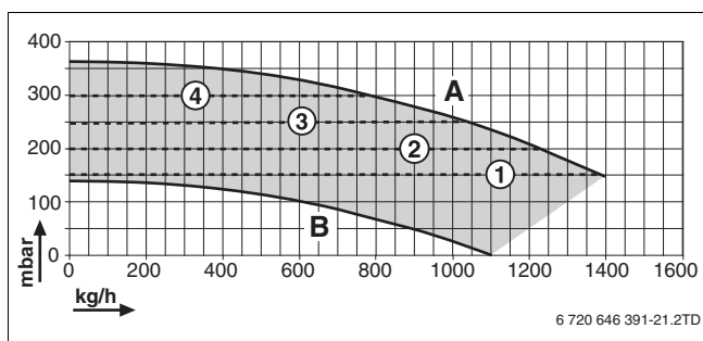
Afb. 8 Restopvoerhoogte bij GC9000iW 30 E(B)
