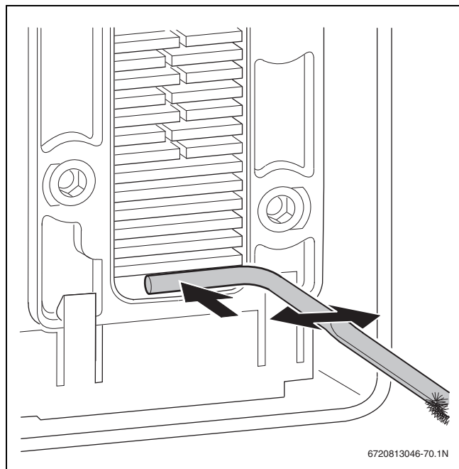
Afb. 49 Condensbak reinigen
