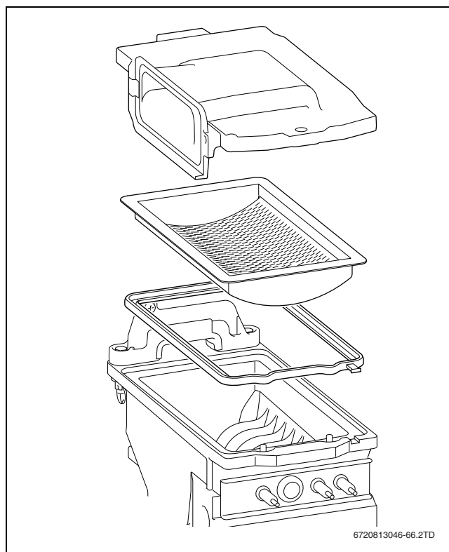
Afb. 42 Brander wegnemen
