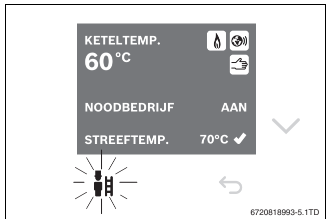
Afb. 35 Menu noodbedrijf
