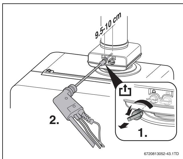
Afb. 30 CO/CO 2 -gehalte meten
