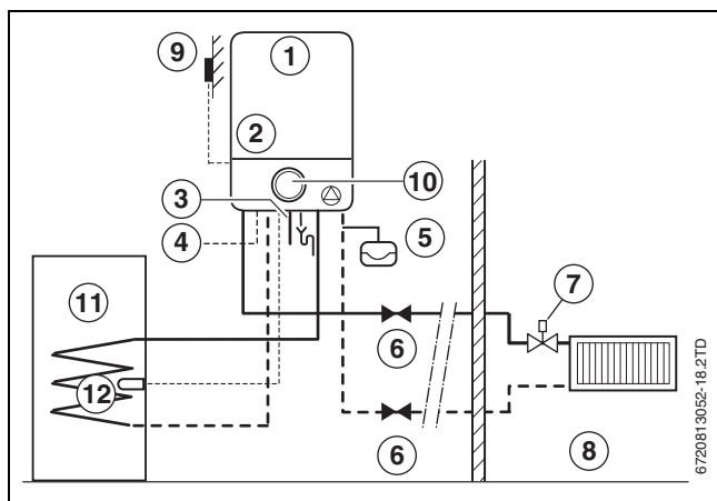
Afb. 20 Toepassingsvoorbeeld met weersafhankelijke regeling en boiler
