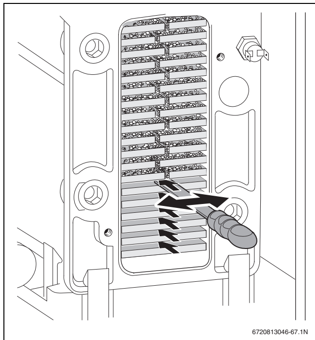
Afb. 46 Reinigingsgereedschap
