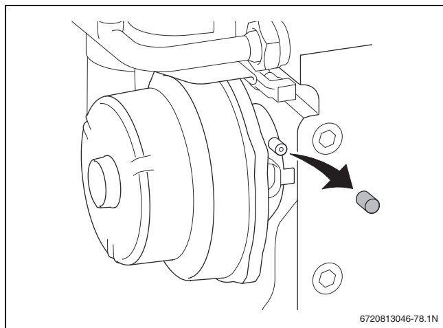
Afb. 45 Meetpunt op de menginrichting
