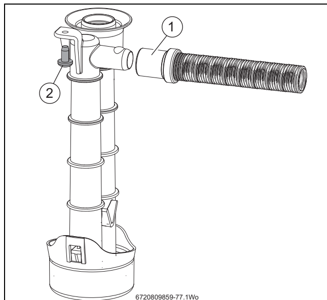
Afb. 12 Condenssifon
