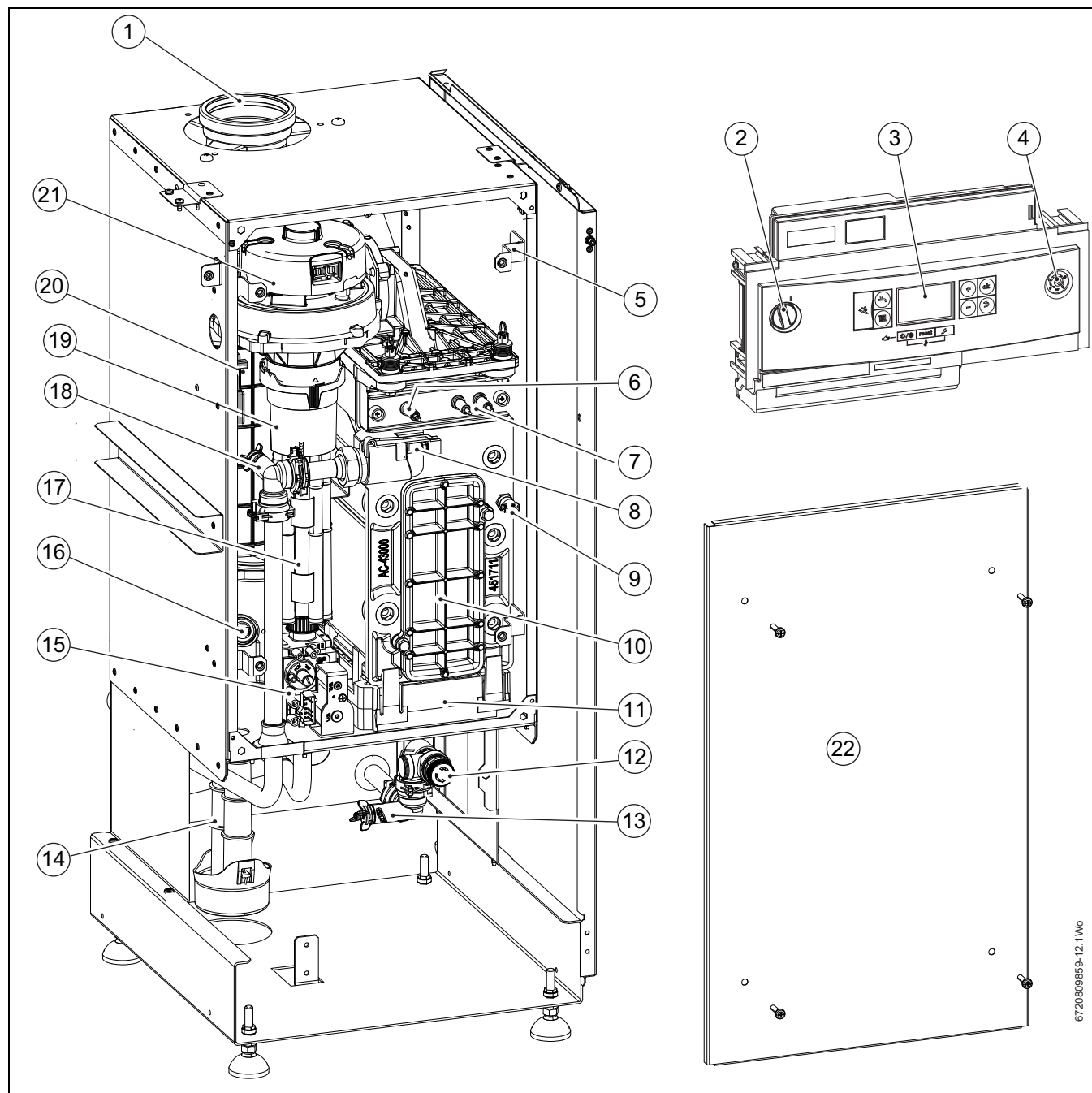
Afb. 3 Suprapur KBR - hoofdcomponenten
