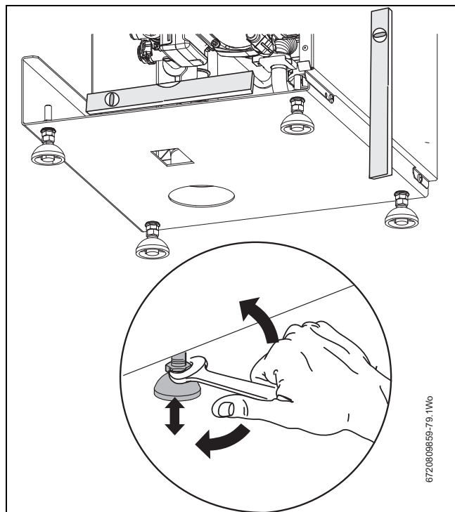
Afb. 15 Ketel uitlijnen
