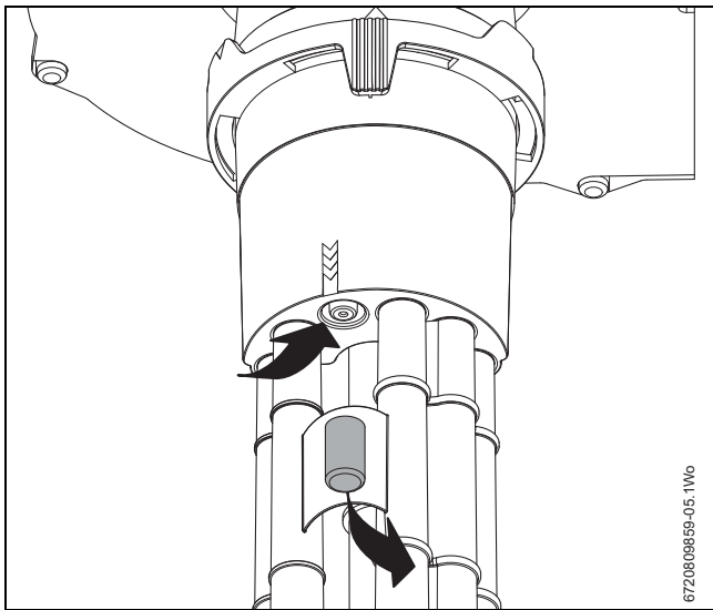
Afb. 49 Ventilator drukmeetpunt en deksel
