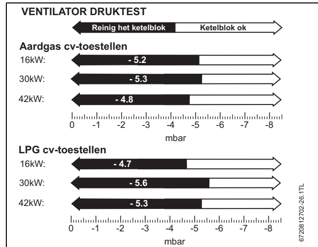
Afb. 51 Ventilatorregeling drukmeetwaarden
