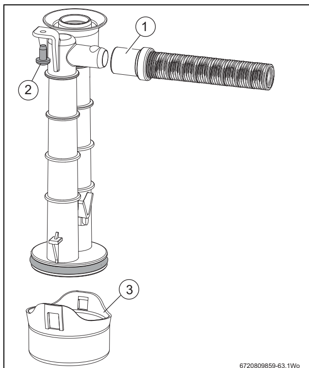
Afb. 65 Condenssifon
