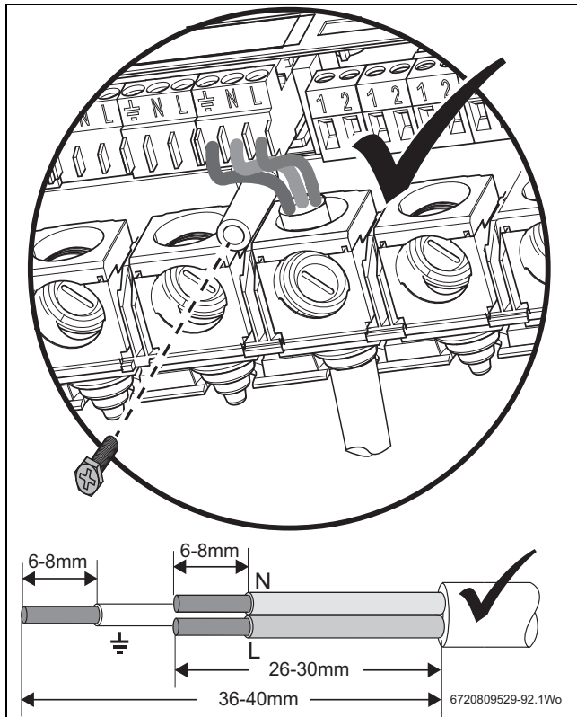
Afb. 23 Kabelhouders
