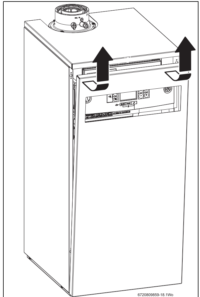
Afb. 47 Toegang tot component
