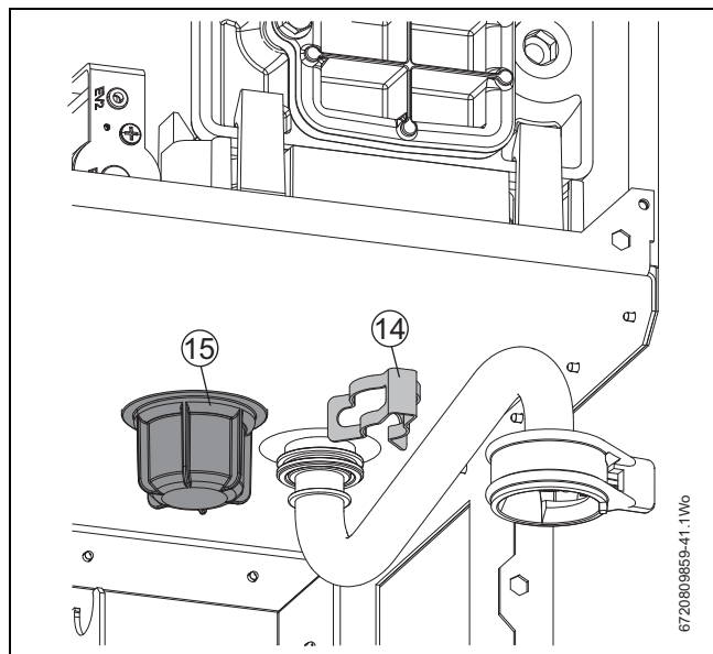
Afb. 68 Primaire warmtewisselaar verwijderen
