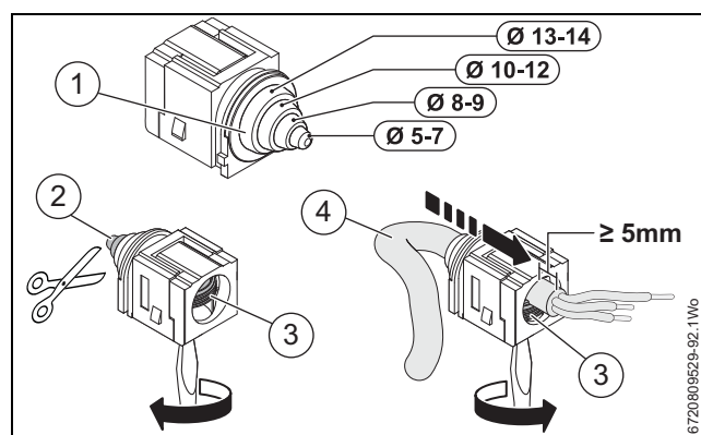
Afb. 22 Kabeldoorvoer
