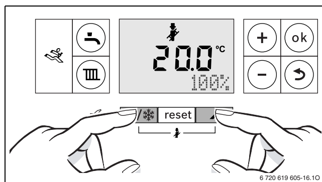
Afb. 44 Gebruik van het cv-toestel
