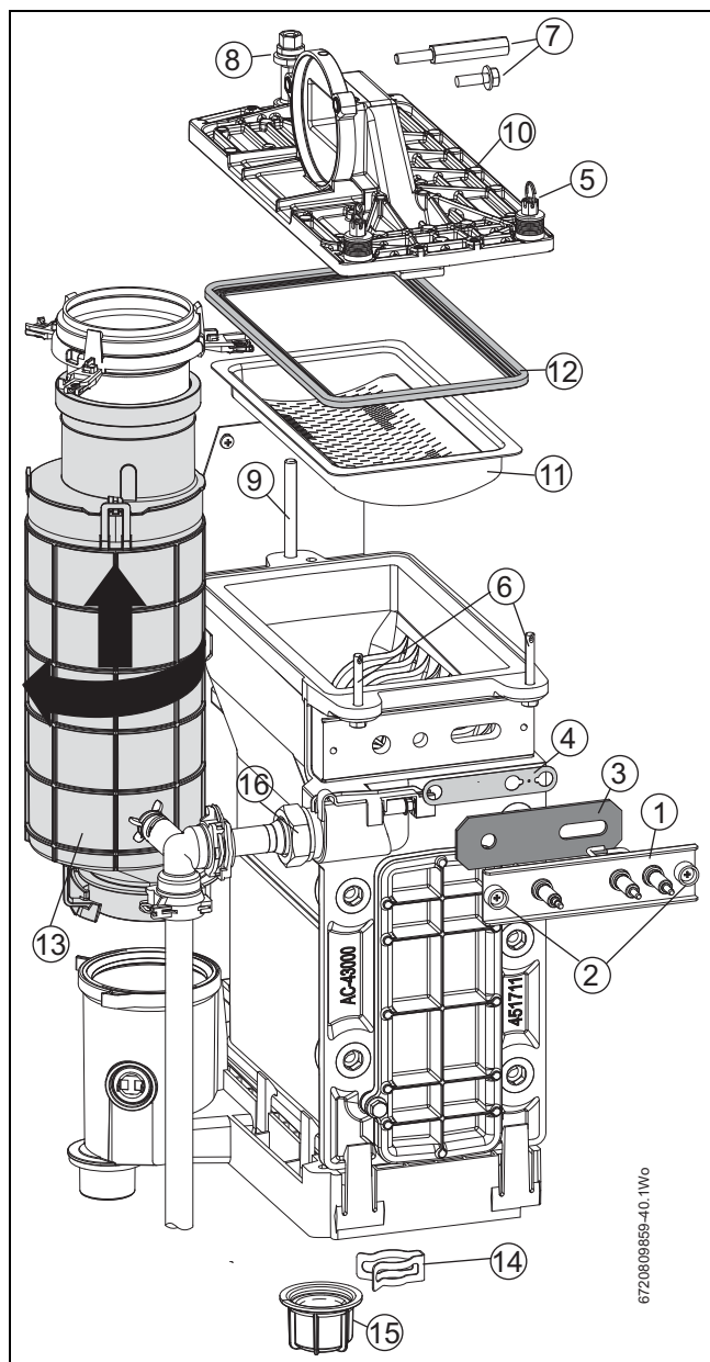
Afb. 67 Primaire warmtewisselaar
