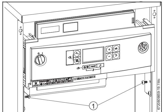
Afb. 48 Bedieningspaneel in de servicepositie
