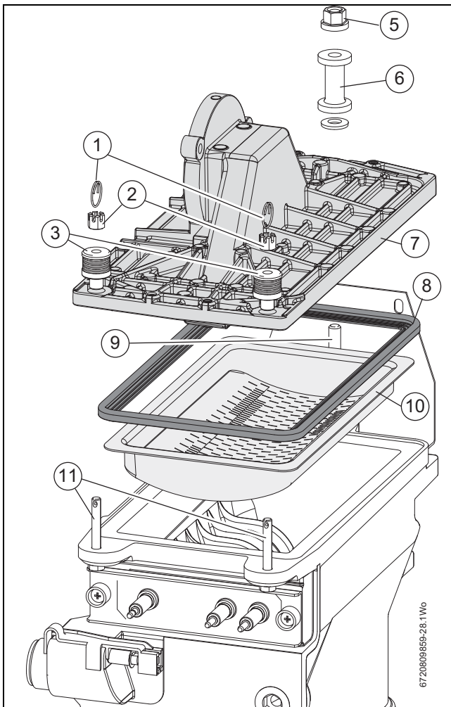
Afb. 57 Brander verwijderen
