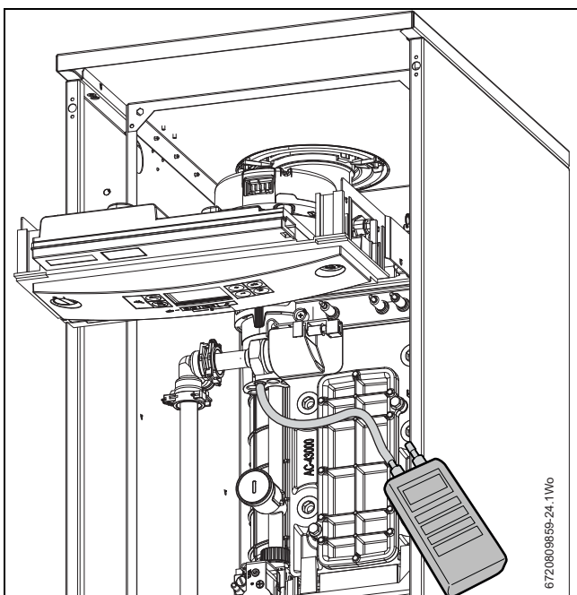
Afb. 50 Ventilatorregeling druktest
