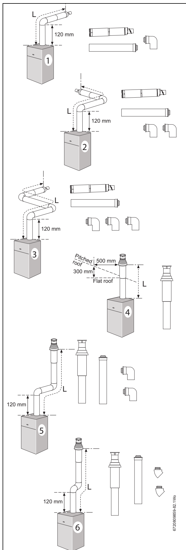
Fig. 17 Rookgasafvoerbuison-opties
