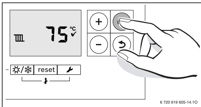
Afb. 36 Maximale aanvoertemperatuur instellen
