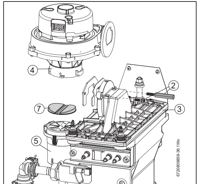
Afb. 62 Ventilator verwijderen - 42 kW versie weergegeven
