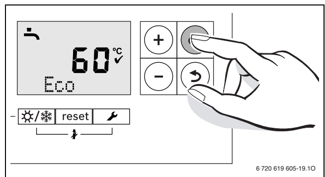
Afb. 38 Eco-bedrijf instelling
