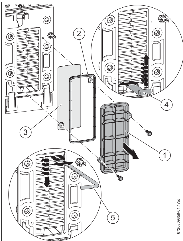
Afb. 55 Warmtewisselaar reinigen
