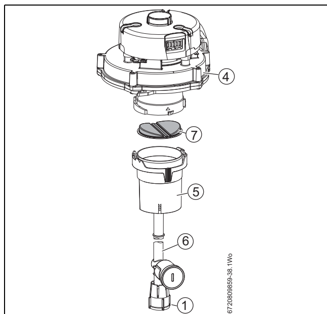
Afb. 63 Klepventiel verwijderen
