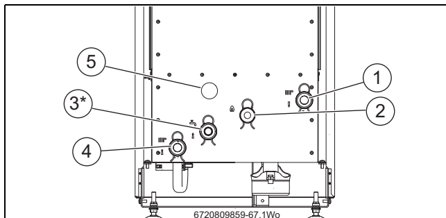
Afb. 24 Controles voorafgaande aan de inbedrijfstelling
