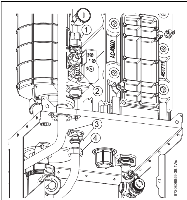
Afb. 66 Gasarmatuur
