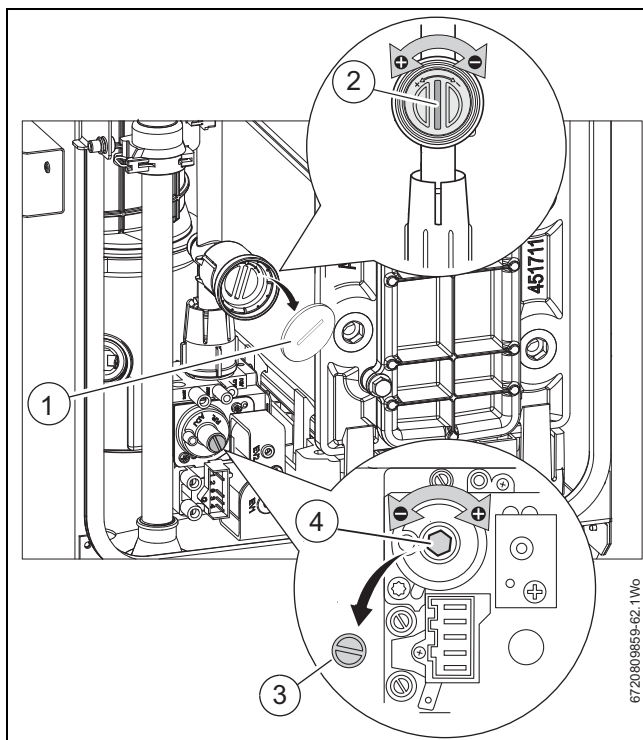
Afb. 54 CO 2 inregeling
