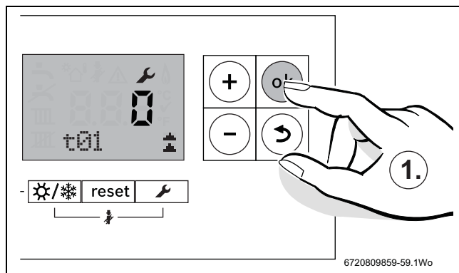
Afb. 76 Blader door de testopties
