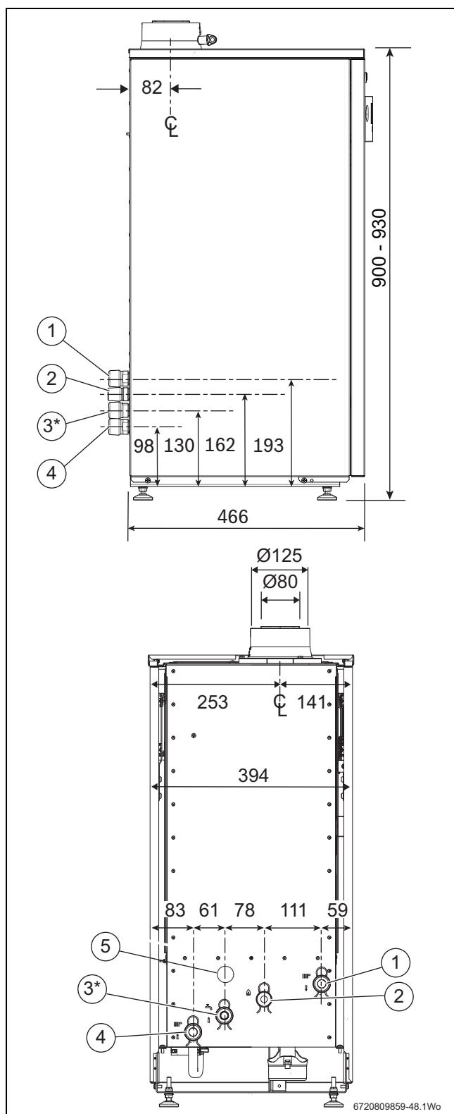
Afb. 16 Afmetingen en aansluitingen (maten in mm)
