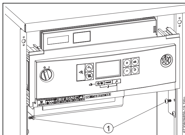
Afb. 59 Bedieningspaneel in de servicepositie
