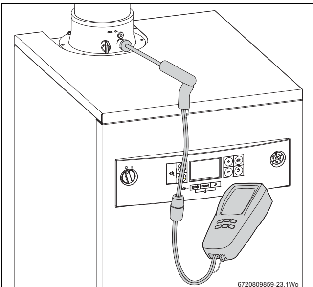
Afb. 46 Rookgasafvoer adapter test
