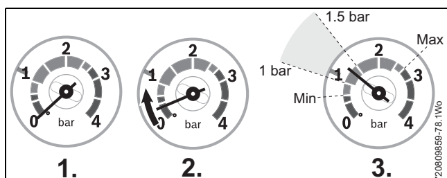
Afb. 25 Installatiedruk bepalen
