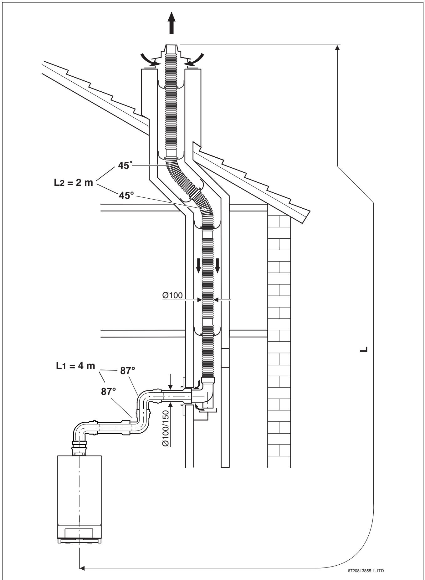
Afb. 10 Voorbeeld lengten rookgasafvoerbuïs
