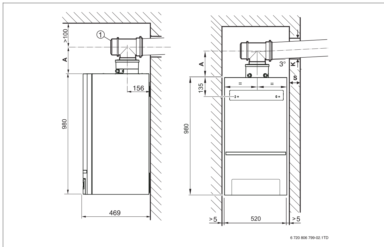
Afb. 9 Inbouwmaten (maten in mm)
