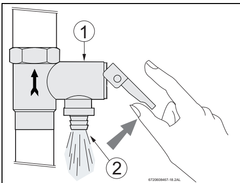
Afb. 56 Overstortventiel
