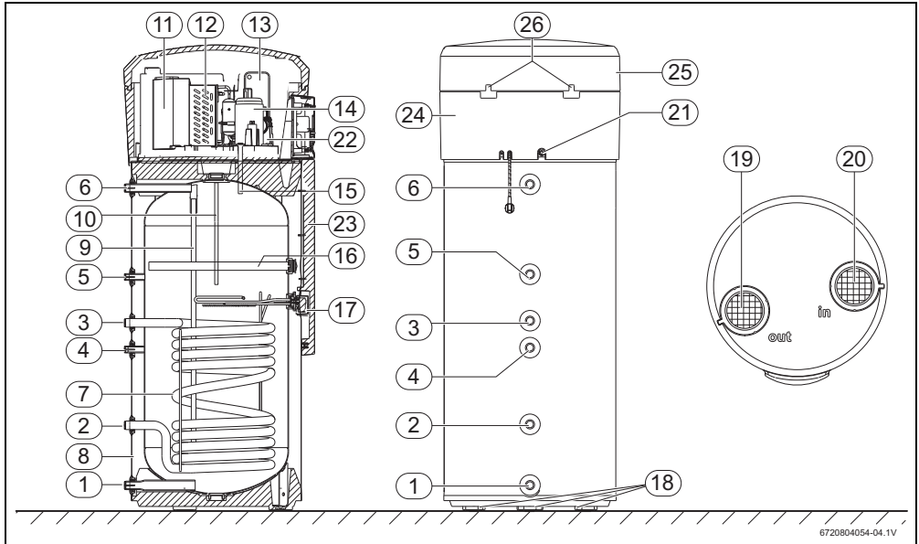
Afb. 3 Warmtepomp
