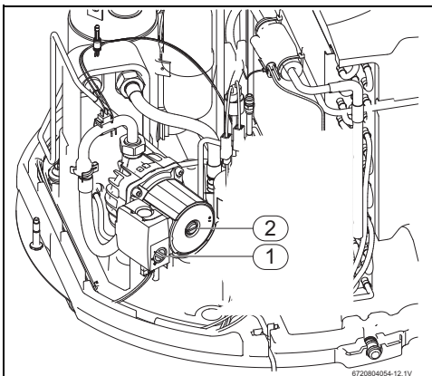
Afb. 13 Circulatiepomp
