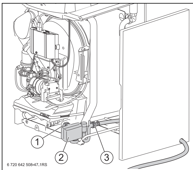
Afb. 71 Sifon demonteren
