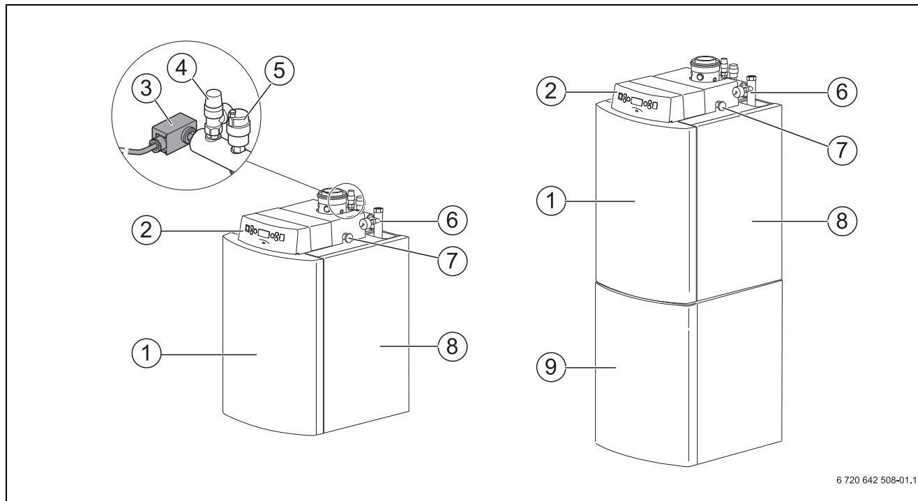
Afb. 1 CV-ketel (links cv-ketel, rechts cv-ketel met boiler)
