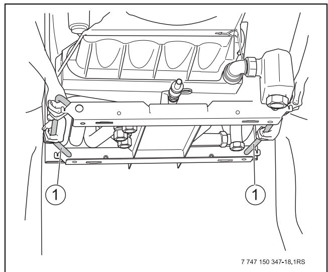
Afb. 11 CV-ketel optillen en dragen
