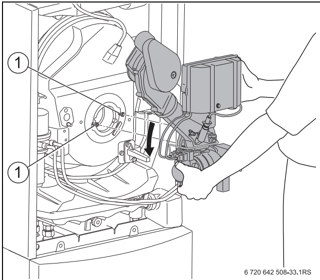
Afb. 74 Brander wegnemen
