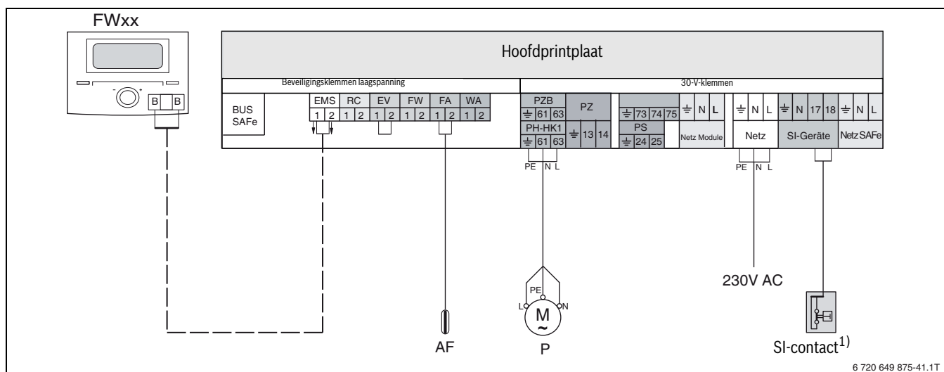
Afb. 13 Aansluitschema ongemengd cv-circuit
