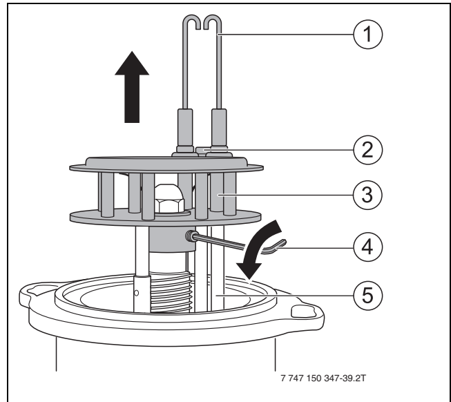
Afb. 76 Demonteer het mengsysteem
