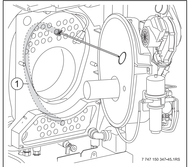
Afb. 70 Rookgaskanalen reinigen
