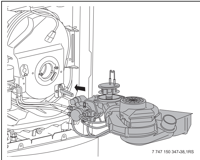
Afb. 75 Brander in servicepositie plaatsen.
