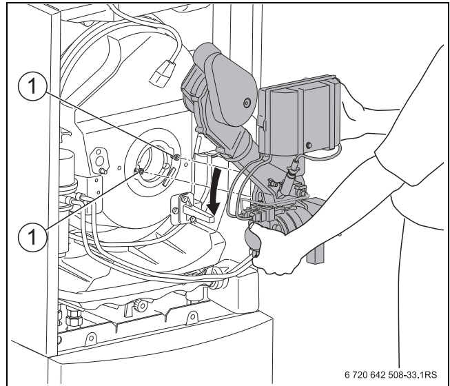
Afb. 54 Brander wegnemen
