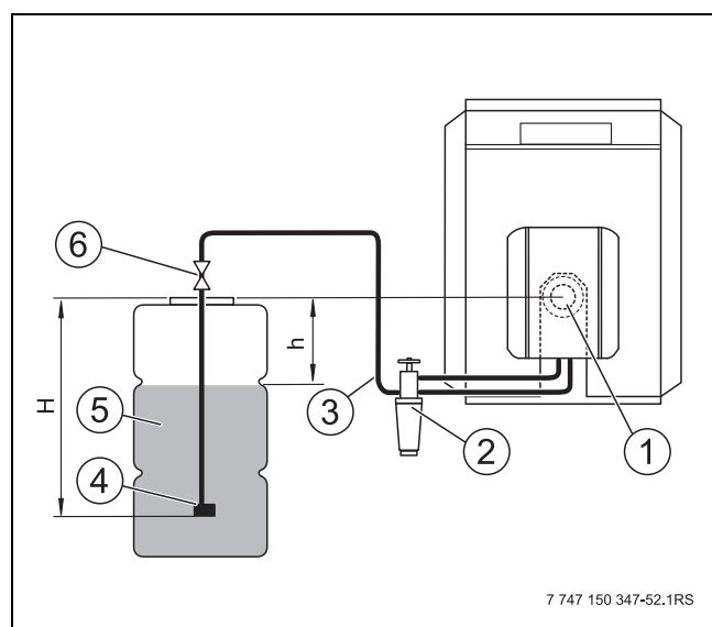
Afb. 30 Dimensionering van de olietoevoerinstallatie, olietank onder de oliepomp
