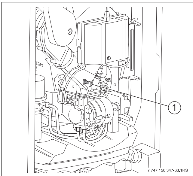
Afb. 47 Statische ventilatordruk meten
