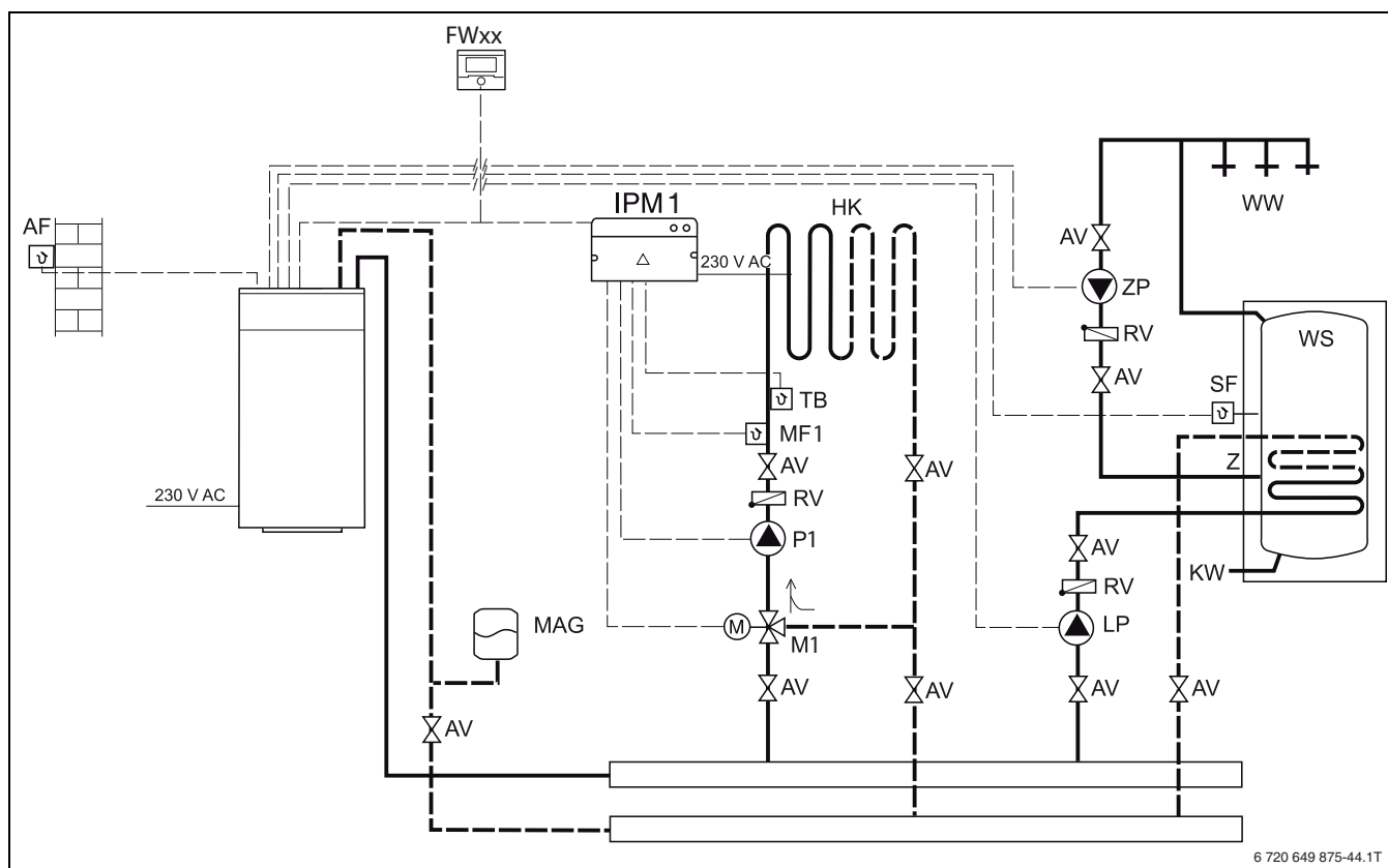
Afb. 16 Vereenvoudigd installatievoorbeeld: een gemengd cv-circuit met warmwaterbereiding via ketelregeling
