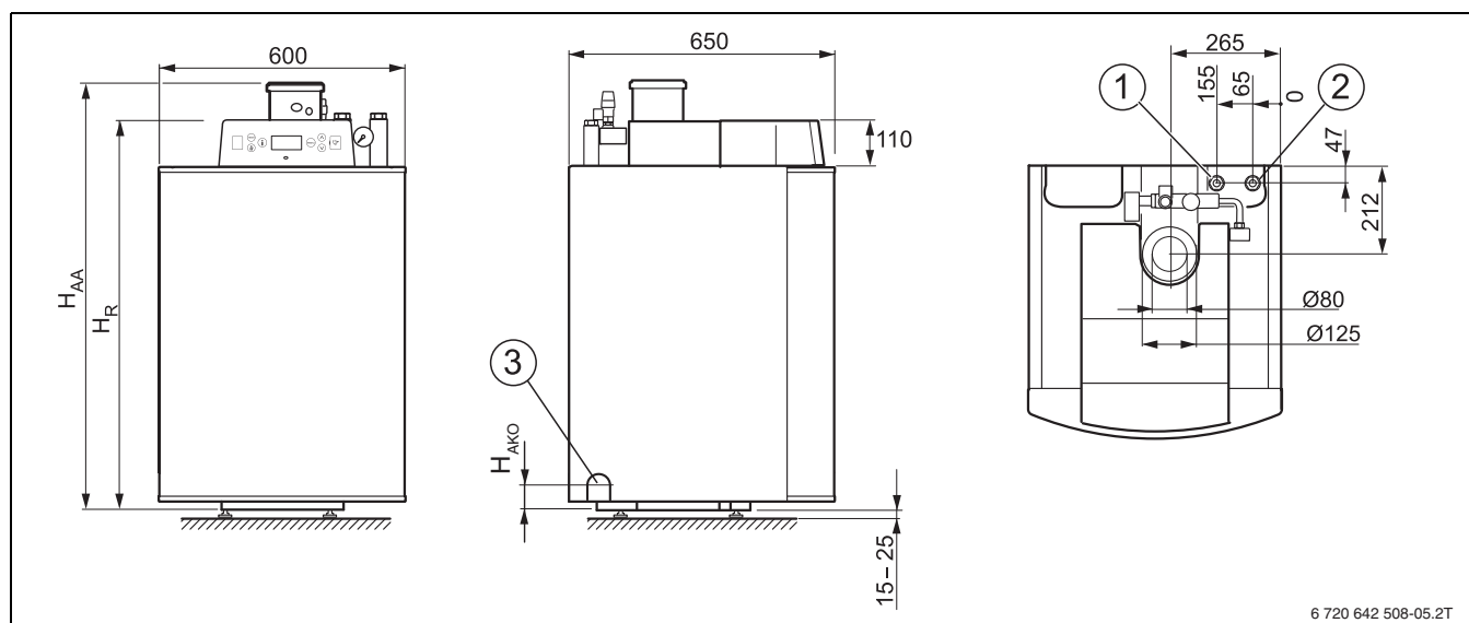
Afb. 4 Aansluitingen en afmetingen van de cv-ketel (maten in mm)
