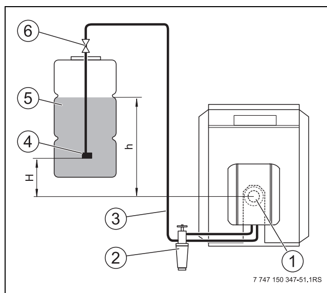
Afb. 29 Dimensionering van de olietoevoerinstallatie, olietank boven de oliepomp
