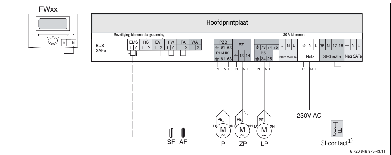
Afb. 15 Aansluiting ongemengd cv-circuit met warmwaterbereiding via ketelregeling
