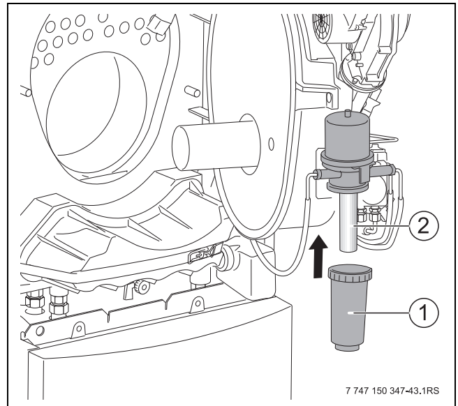
Afb. 66 Filterelement vervangen
