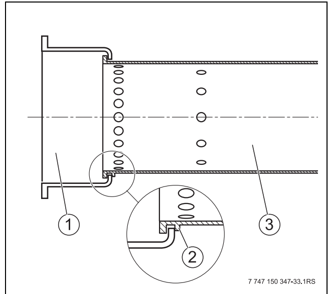
Afb. 61 Branderbuis plaatsen
