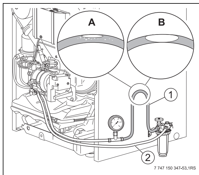
Afb. 42 Transparante slang omhoogbinden
