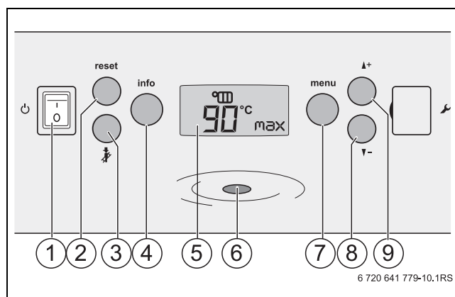
Afb. 38 Bedieningselementen
