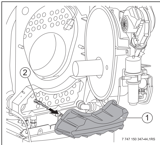
Afb. 67 Turbulatoren uittrekken
