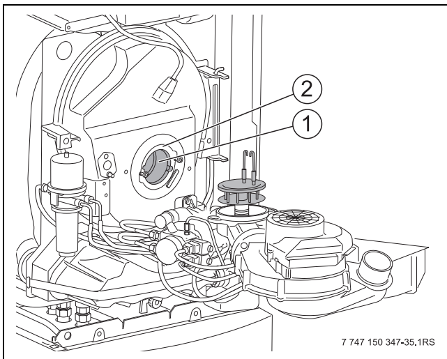
Afb. 60 Branderbuis vervangen
