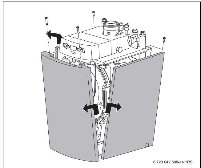
Afb. 10 Zijwanden afnemen
