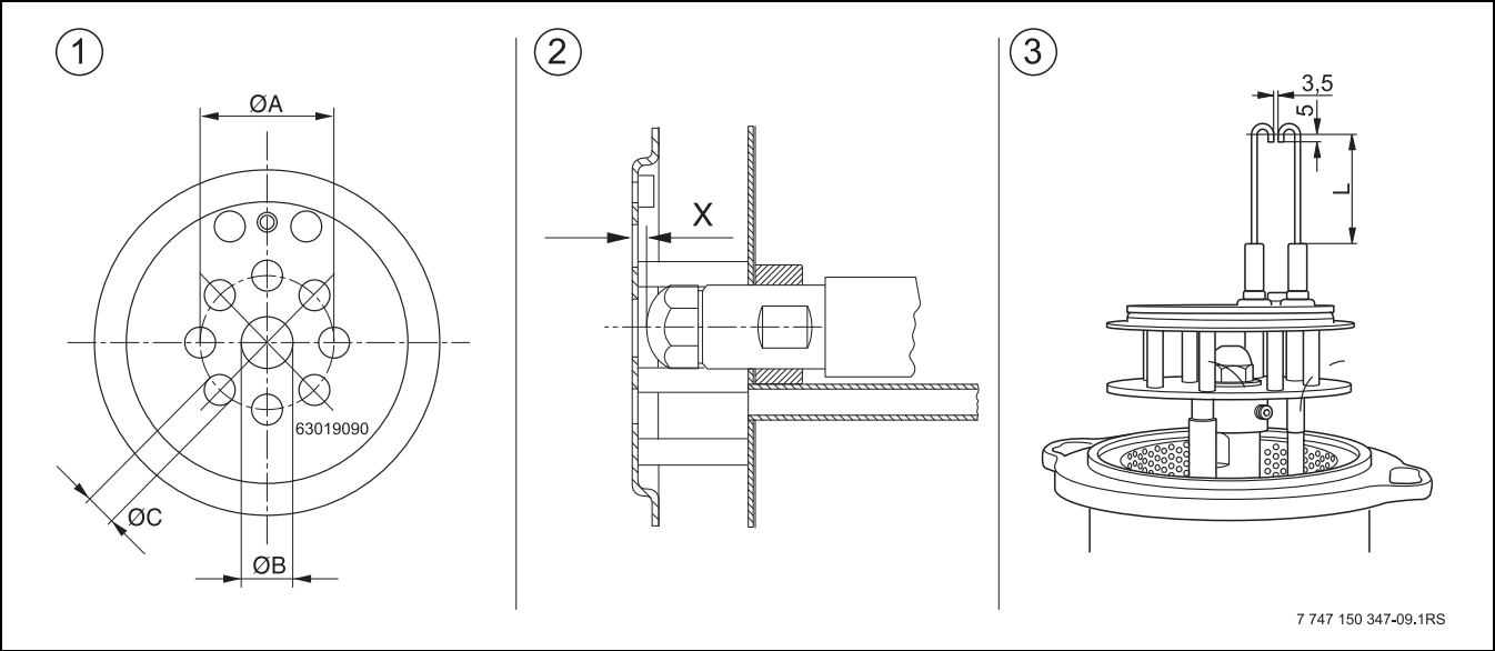
Afb. 6 Mengsysteem brander en ontstekingselektrode
