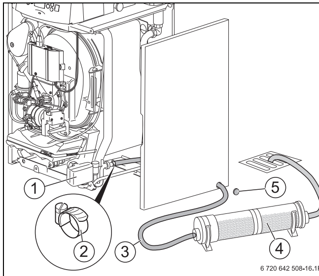
Afb. 25 Condenswaterafvoer met neutralisatie
