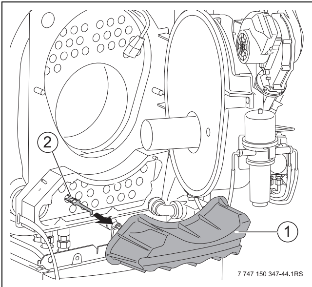
Afb. 69 Turbulatoren uittrekken
