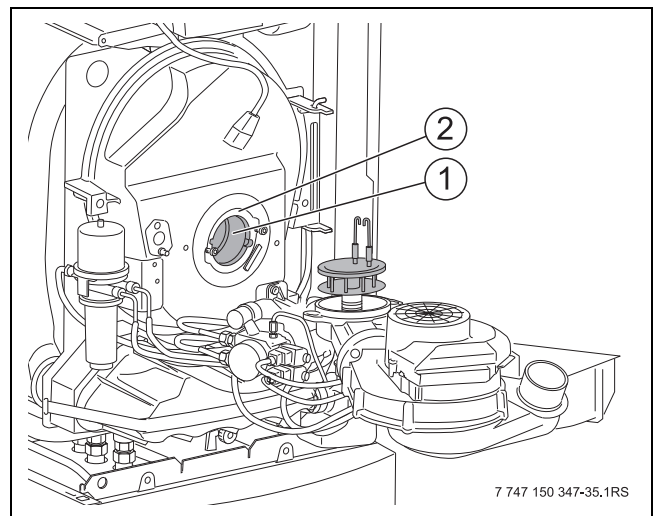
Afb. 62 Dichting controleren
