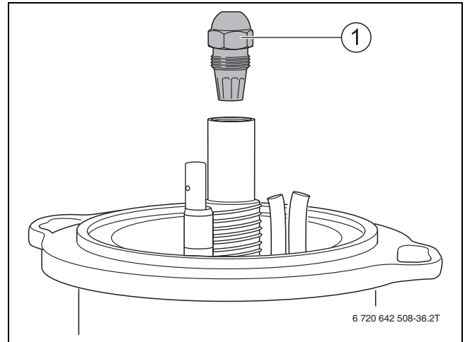
Afb. 57 Sproeier afschroeven
