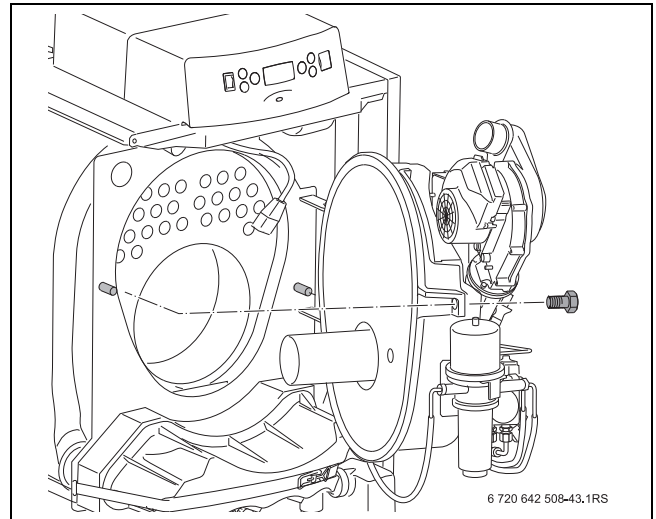
Afb. 65 Brander deur openen
