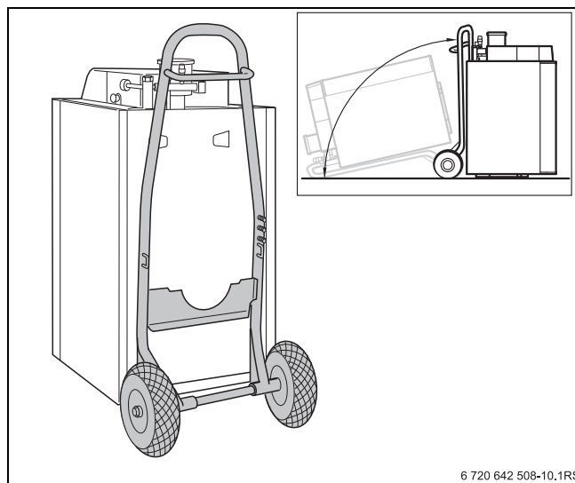
Afb. 21 Stelvoetjes met transportmiddel monteren
