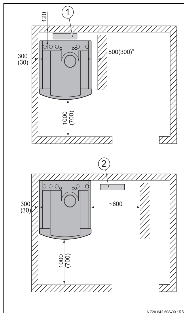
Afb. 20 Aanbevolen wandafstanden, tussen haakjes minimale wandafstanden (in mm)
