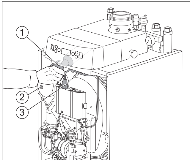
Afb. 52 Venturi afnemen
