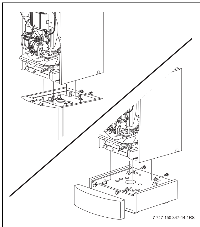
Afb. 23 CV-ketel op een tapwaterboiler of ketelsokkel heffen en monteren
