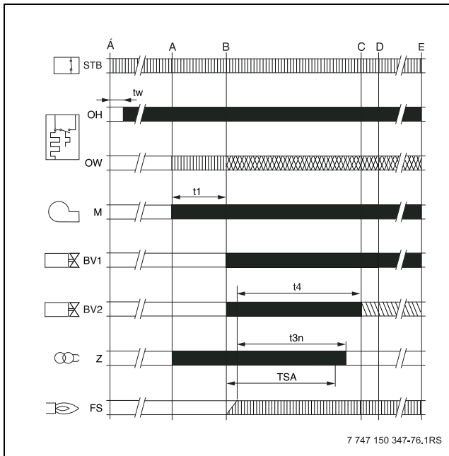
Afb. 78 Programmaprocedure bij branderautomaten
