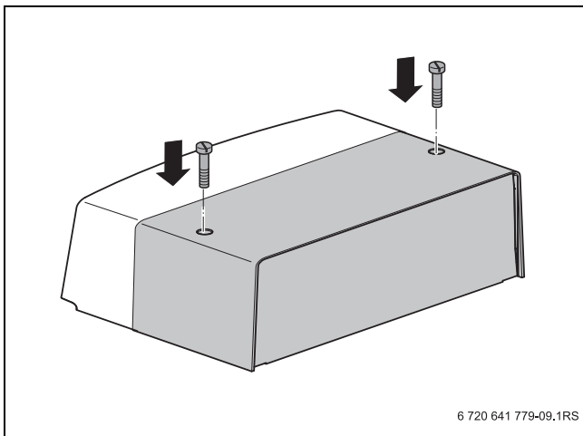
Afb. 37 Afdekkap monteren
