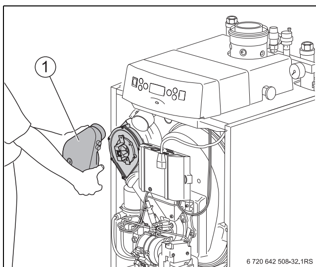
Afb. 53 Aansluiting voor de verbrandingslucht wegnemen
