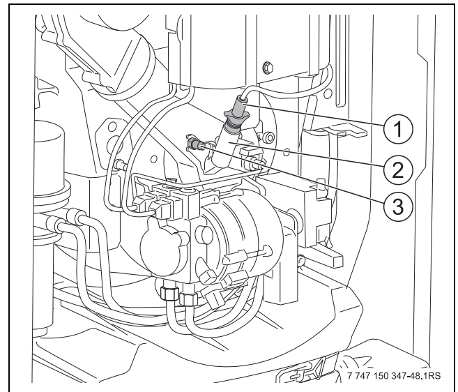
Afb. 73 Fotocel demonteren
