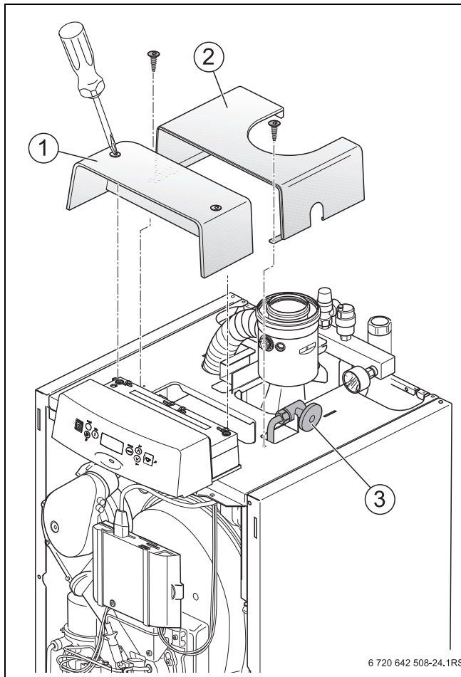
Afb. 32 Olieleiding aansluiten
