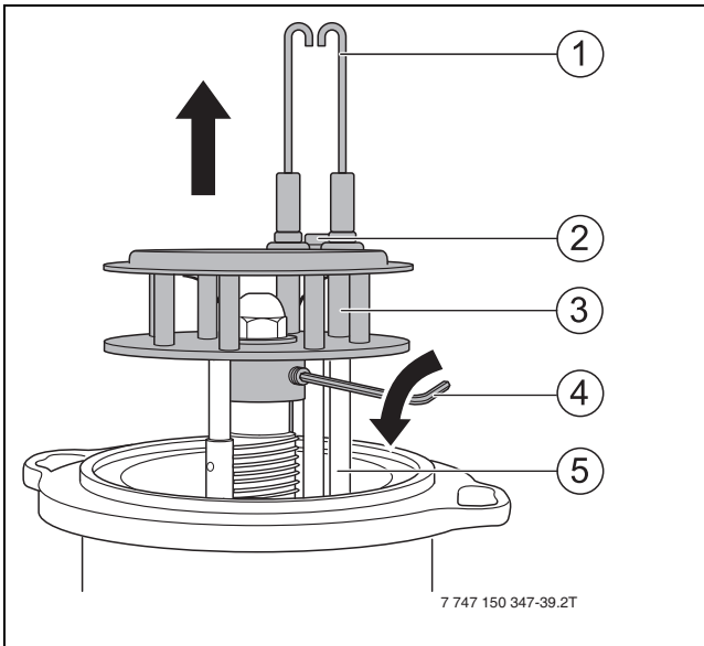
Afb. 56 Demonteer het mengsysteem
