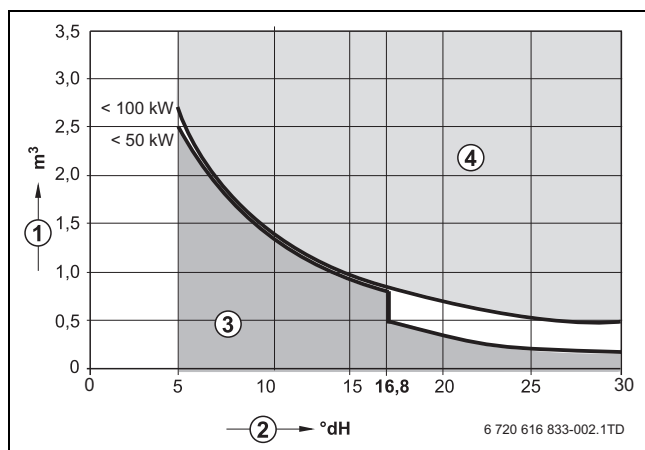
Afb. 8 Eisen aan het ketelwater voor losse ketels tot 100 kW
