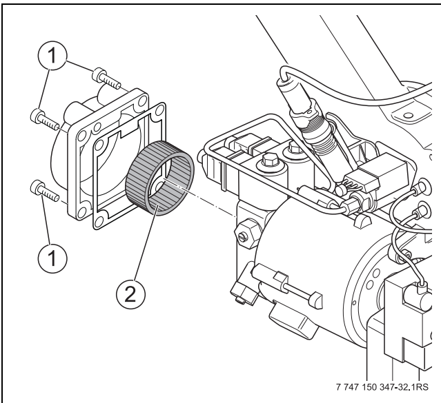
Afb. 64 Oliepompfilter controleren
