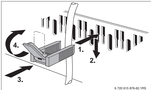
Afb. 36 Kabels met trekontlasting vastzetten
