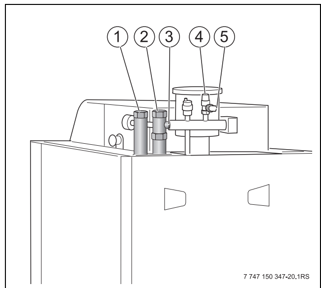
Afb. 26 Achteraanzicht van de cv-ketel
