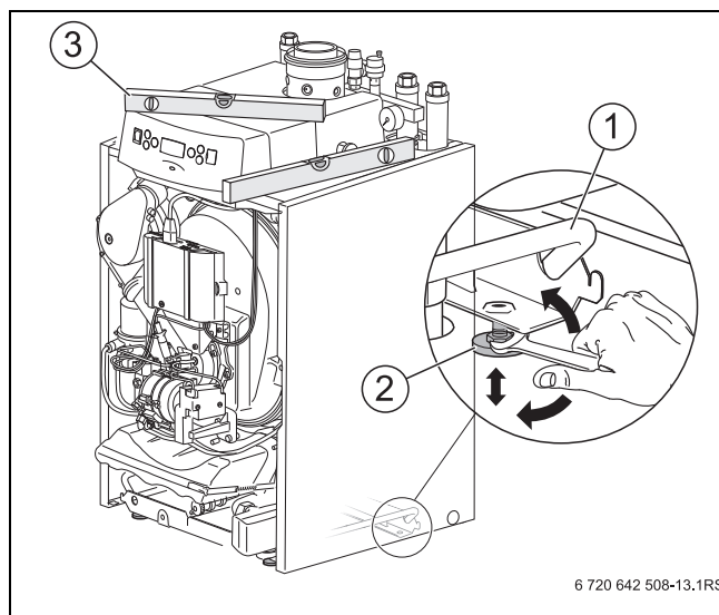
Afb. 24 Ketel uitlijnen
