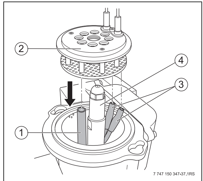
Afb. 58 Mengsysteem monteren
