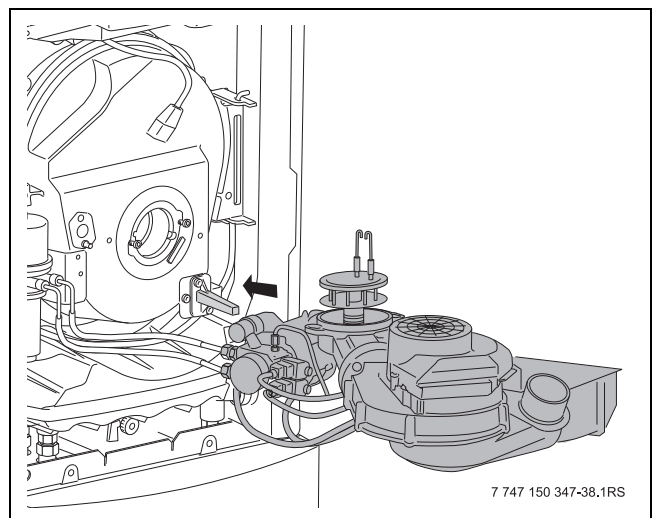
Afb. 55 Brander in servicepositie plaatsen.
