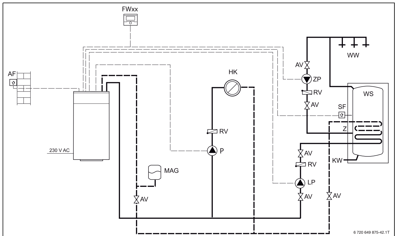
Afb. 14 Vereenvoudigd installatievoorbeeld: een ongemengd cv-circuit met warmwaterbereiding via ketelregeling
