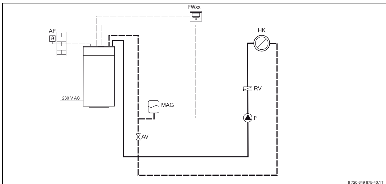
Afb. 12 Vereenvoudigd installatievoorbeeld: een ongemengd cv-circuit
