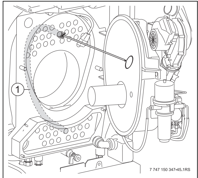
Afb. 68 Rookgaskanalen reinigen
