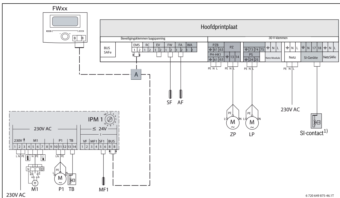
Afb. 17 Aansluitschema gemengd cv-circuit met warmwaterbereiding via ketelregeling
