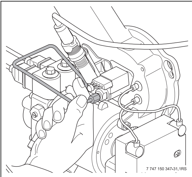
Afb. 63 Olieleiding wegtrekken
