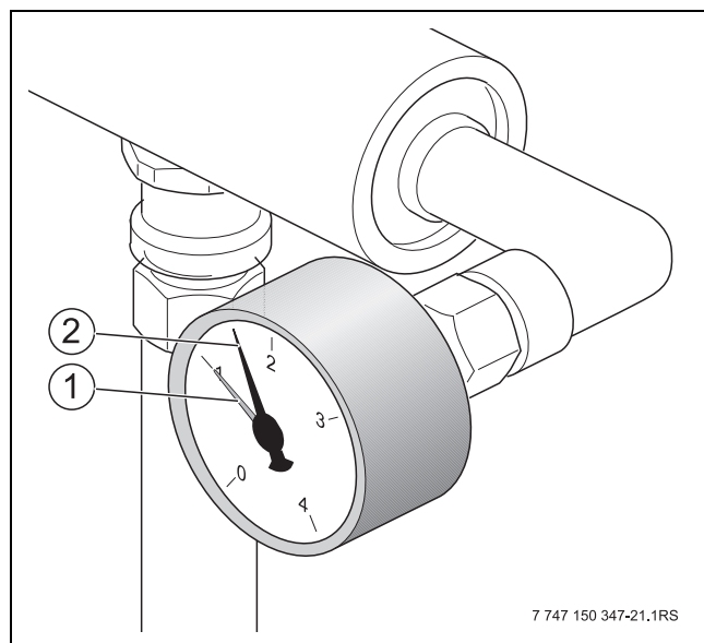
Afb. 27 Manometer
