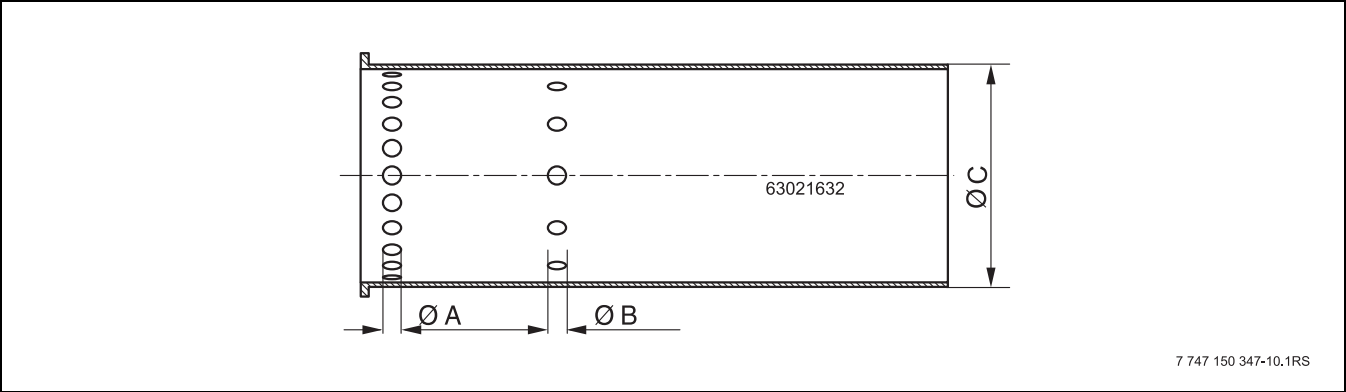
Afb. 7 Branderbuizen
