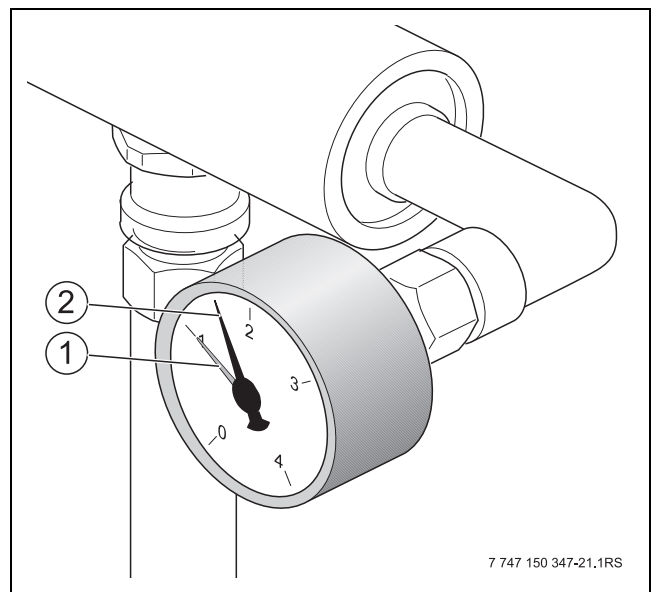
Afb. 72 Manometer
