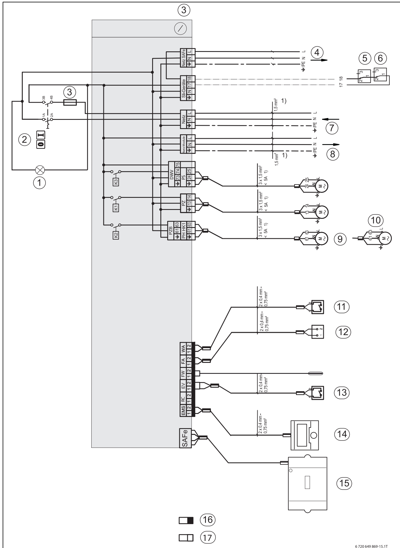
Afb. 34 Aansluitschema hoofdprintplaat
