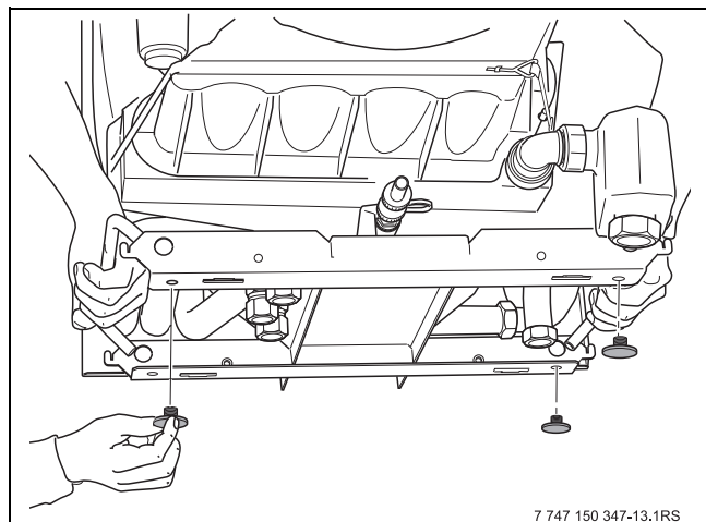
Afb. 22 Stelvoetjes zonder transportmiddel monteren
