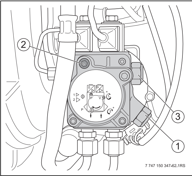
Afb. 46 Druk instellen
