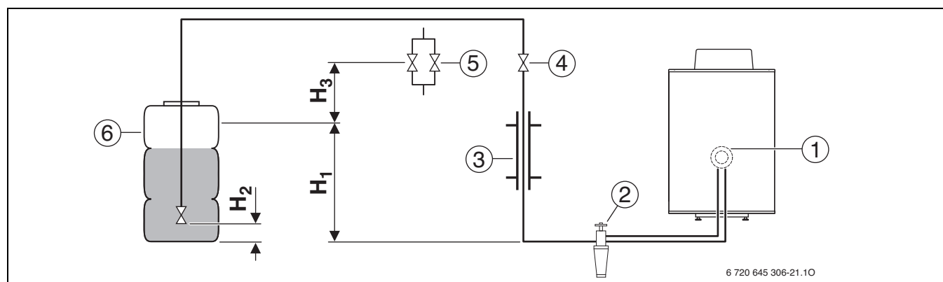
Afb. 31 Installatievoorbeeld
