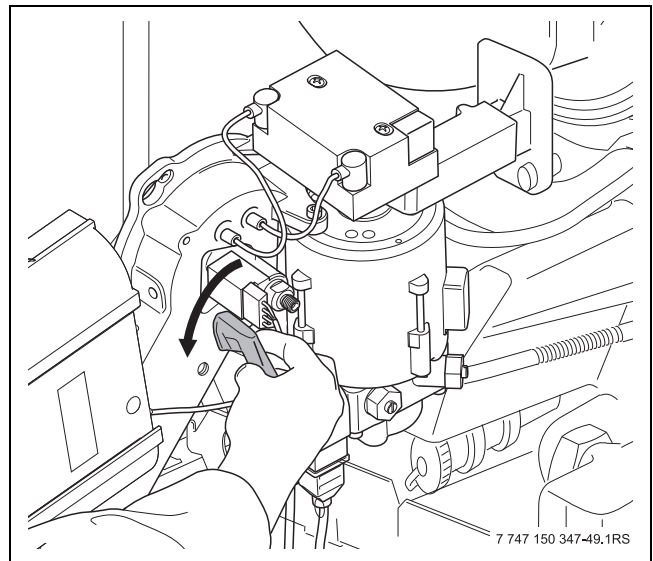
Afb. 77 Hoekvormige houder demonteren
