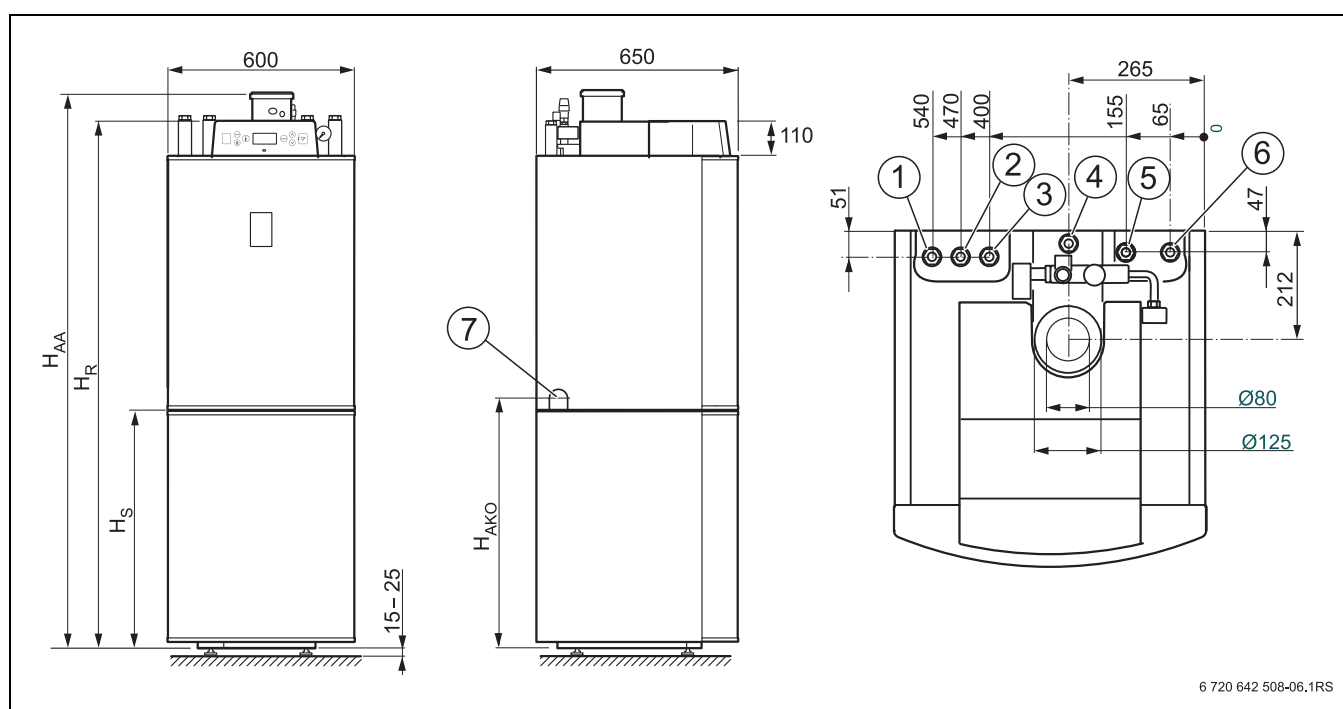
Afb. 5 Aansluitingen en afmetingen van de cv-ketel met optioneel ingebouwde boiler (maten in mm)
