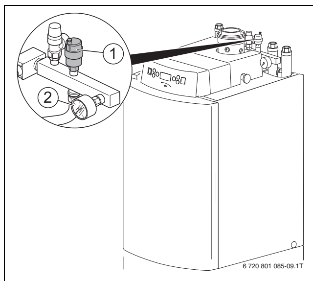
Afb. 28 Vullen cv-installatie
