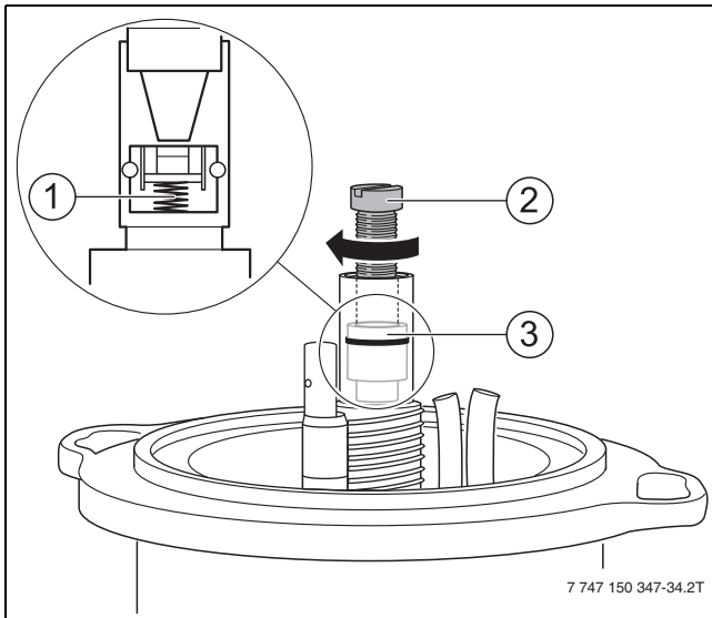
Afb. 59 Afsluitklep vervangen
