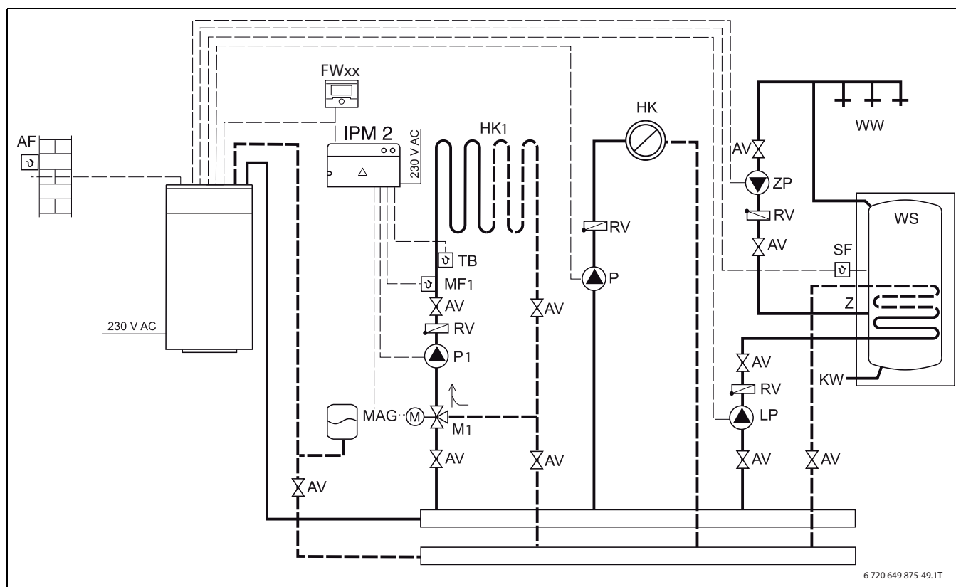
Afb. 18 Vereenvoudigd installatievoorbeeld: een gemengd cv-circuit en een ongemengd cv-circuit met boiler
