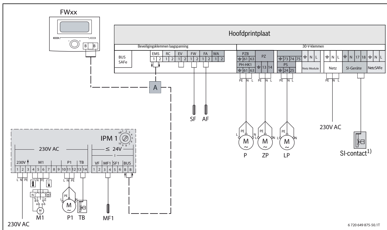
Afb. 19 Aansluitschema gemengd cv-circuit en ongemengd cv-circuit met warmwaterbereiding via ketelregeling
