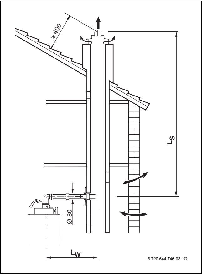
Afb. 10 Parallele buIs naar schacht (B 23 , B 23P )
