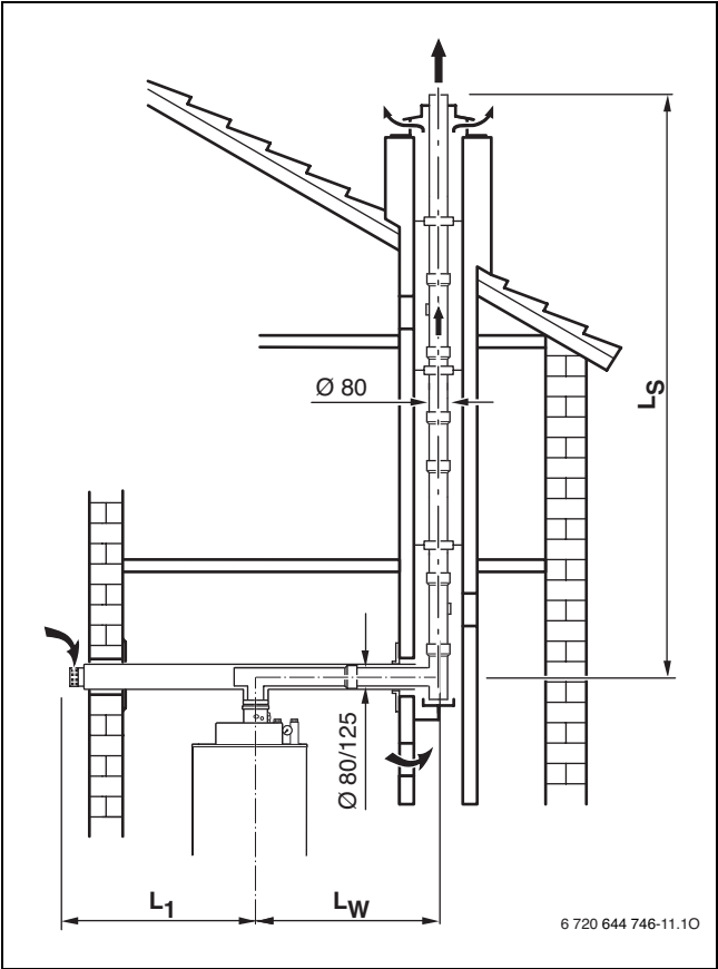
Afb. 18 Gescheiden rookgasafvoer in schacht ( C_{53(x)} )
