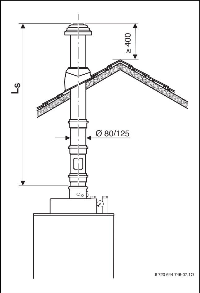
Afb. 14 Concentrische buis verticaal (C 33(x) )
