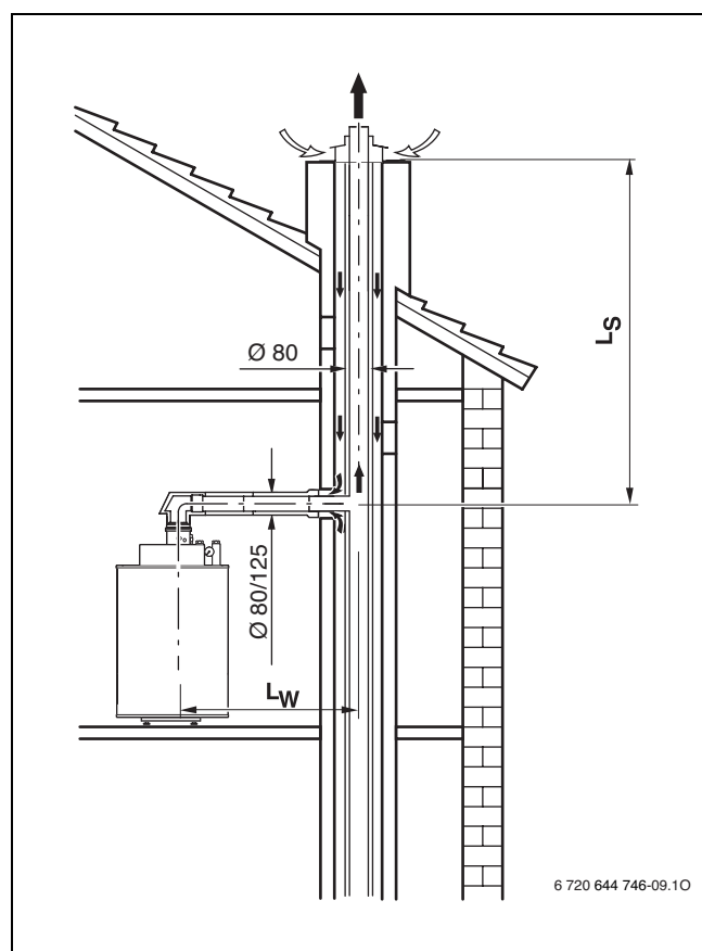
Afb. 16 Concentrische buis tot bestaand rookgasafvoerkanaal (C 43(x) )
