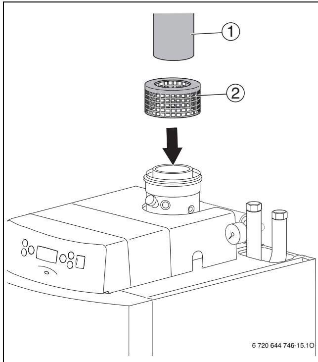
Afb. 1 Montage verbrandingsluchtrooster
