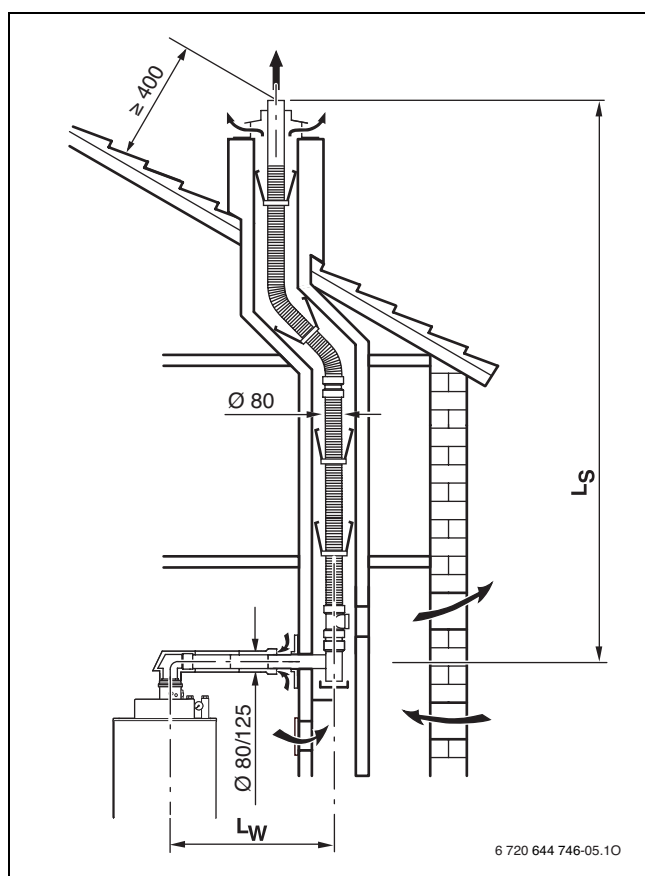
Afb. 12 Parallelle buīs in schacht ( B_{33} , flexibel)
