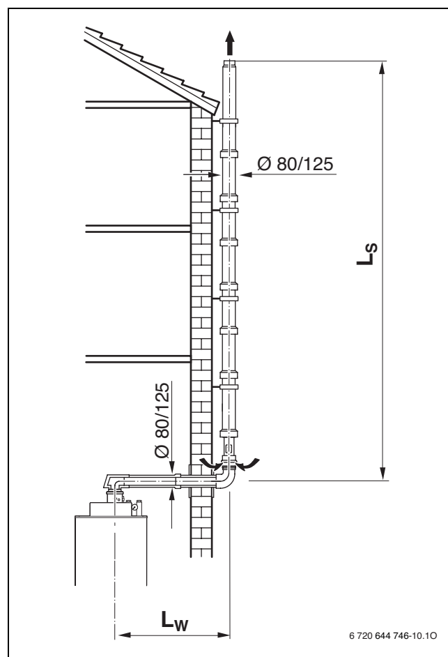
Afb. 17 Concentrische buis tegen de gevel (C 53(x) )
