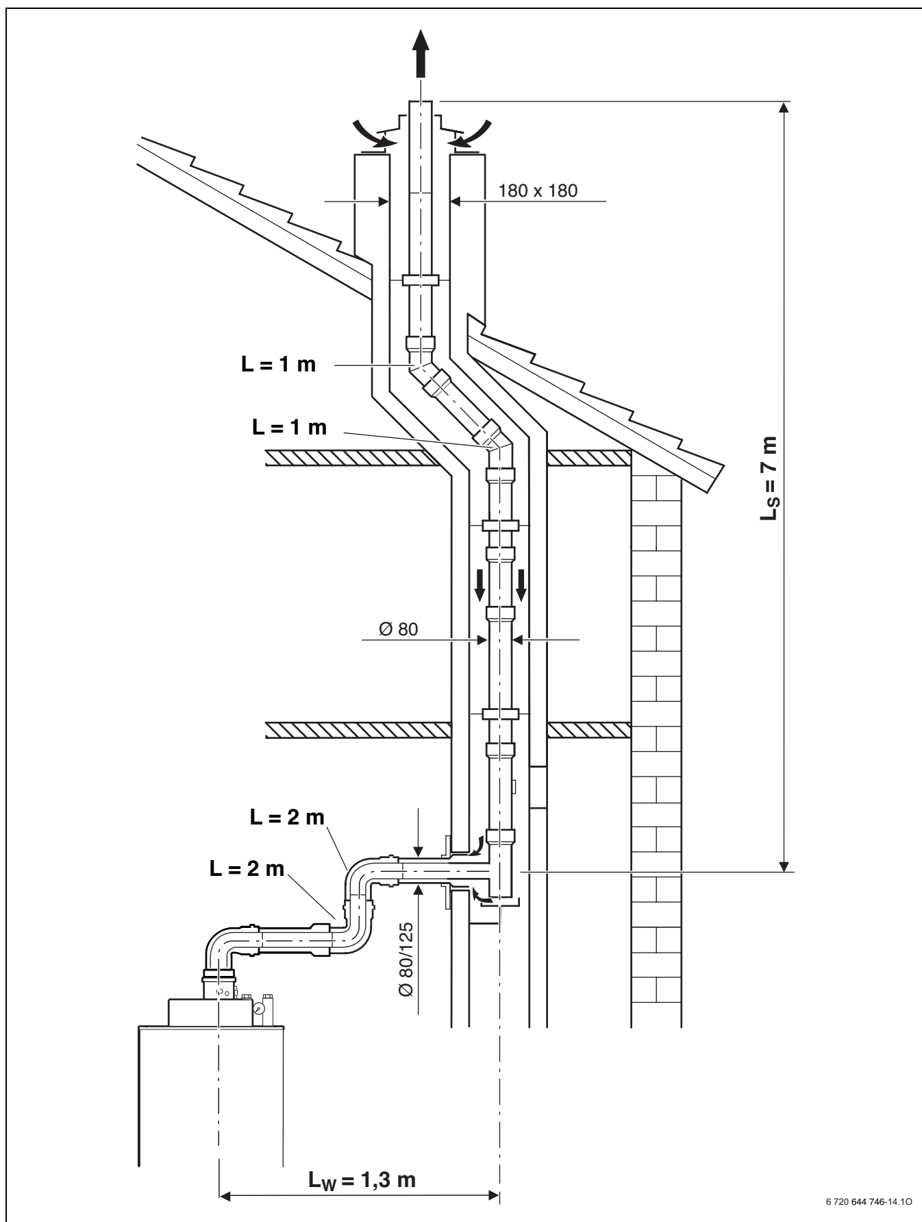
Afb. 20 Voorbeeld lengten rookgasafvoerbuiss
