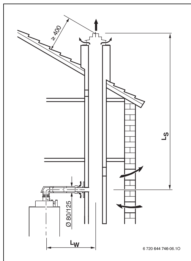
Afb. 13 Concentrische buīs naar schacht ( B_{33} , star)
