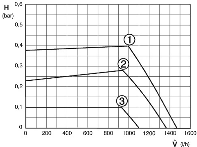
Fig. 76 constante druk TOP 22/275-3 ZBS
