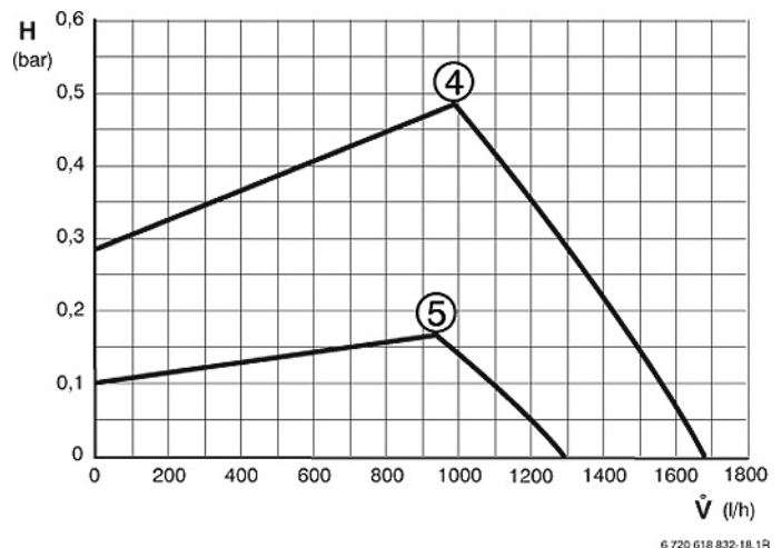
Fig. 79 proportionele druk TOP 30/375-3 ZBS
