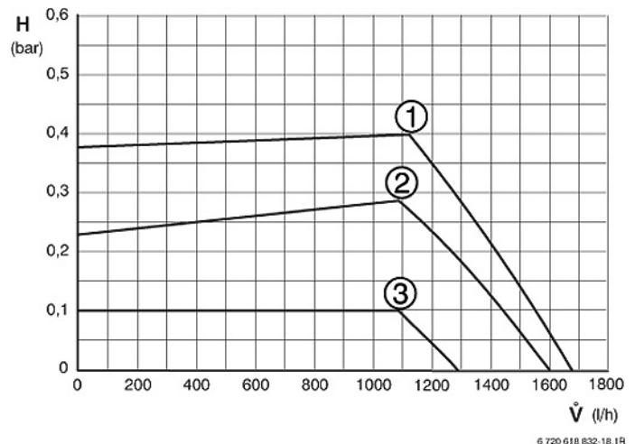
Fig. 77 constante druk TOP 30/375-3 ZBS
