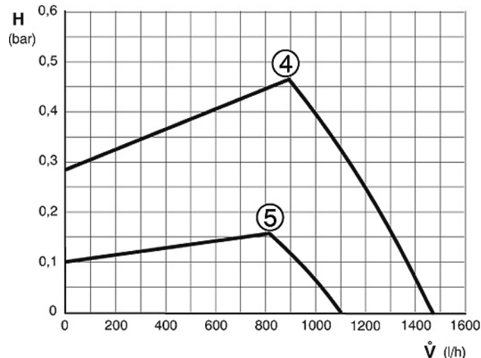
Fig. 78 proportionele druk TOP 22/275-3 ZBS
