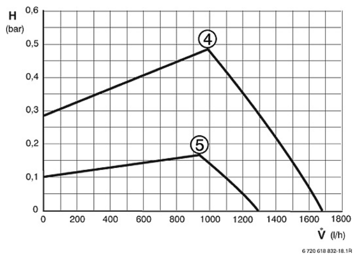
Fig. 68 proportionele druk TOP 30/475-3 ZBS
