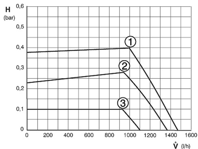
Fig. 65 constante druk TOP 14/400-3 ZBS
