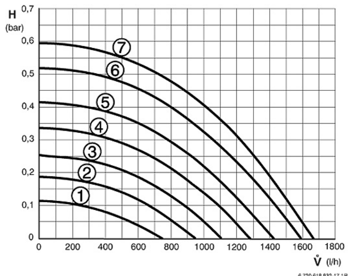
Fig. 70 stand intelligente circulatiepomp TOP 30/475-3 ZBS
