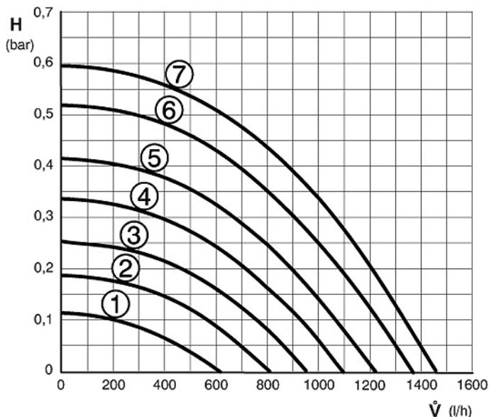
Fig. 69 stand intelligente circulatiepomp TOP 14/400-3 ZBS
