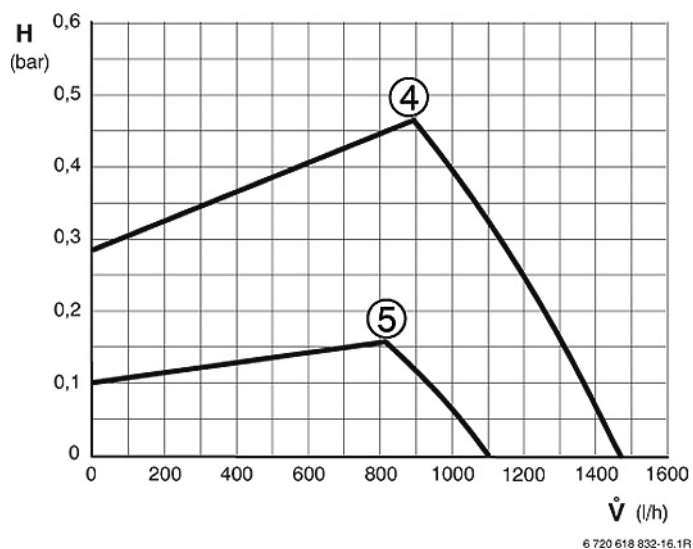
Fig. 67 proportionele druk TOP 14/400-3 ZBS
