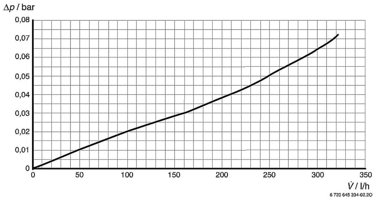
Fig. 15 Warmwaterzijdig drukverlies
