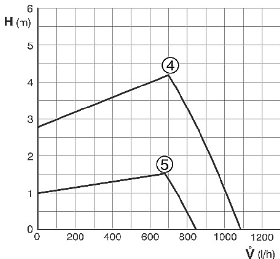
Fig. 50 proportionele druk gasket met buffervat SP 400 SHU en aansluitset Nr. 1463
