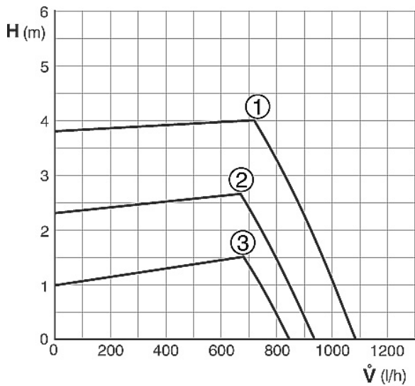
Fig. 48 constante druk gasket met buffervat SP 400 SHU en aansluitset Nr. 1463
