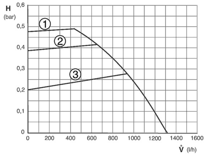
Fig. 64 constante druk TOP 14/400-3 ZBS
