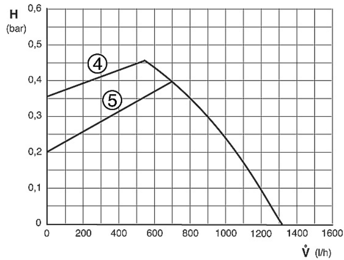
Fig. 66 proportionele druk TOP 14/400-3 ZBS
