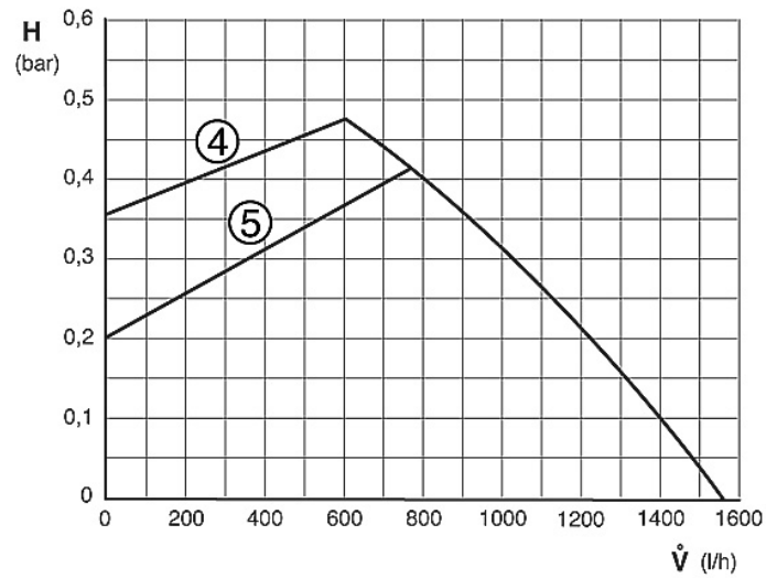
Fig. 67 proportionele druk TOP 30/475-3 ZBS
