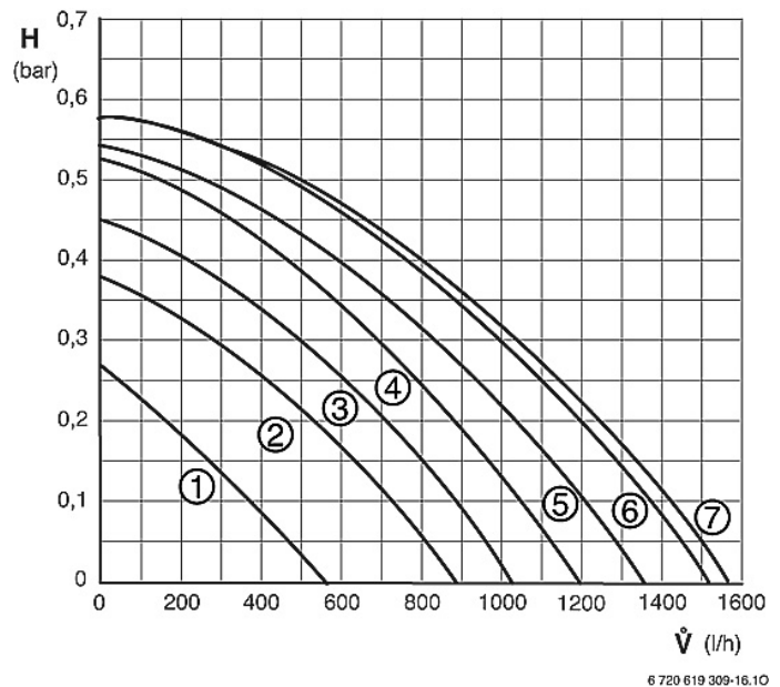
Fig. 69 stand intelligente circulatiepomp TOP 30/475-3 ZBS
