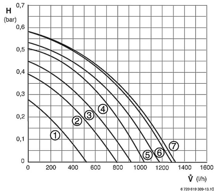
Fig. 68 stand intelligente circulatiepomp TOP 14/400-3 ZBS
