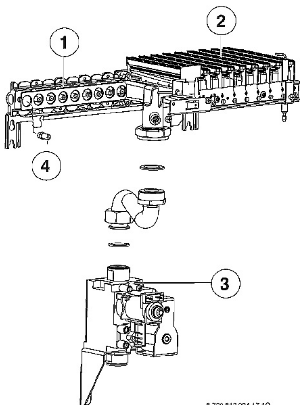
Fig. 50 brander ZSC 24-3, ZWC 24-3 & ZWC 28-3
