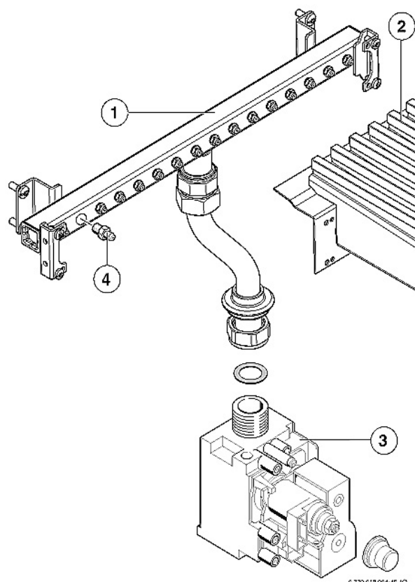
Fig. 51 brander ZWC 35-3
