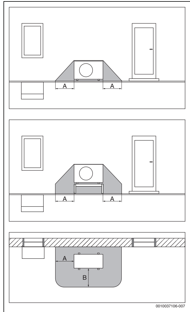
Fig. 1 Volume de protection, placement au sol
