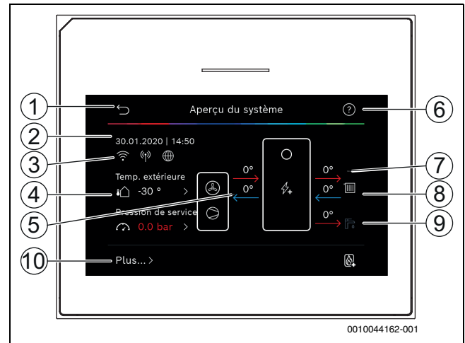
Fig. 12 Vue d'ensemble du système
