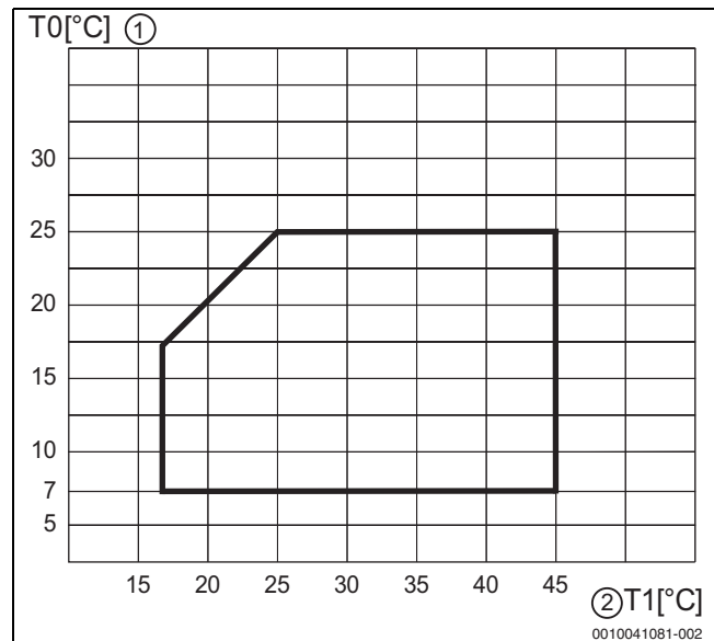
Fig. 5 Pompe à chaleur en mode Refroidissement
