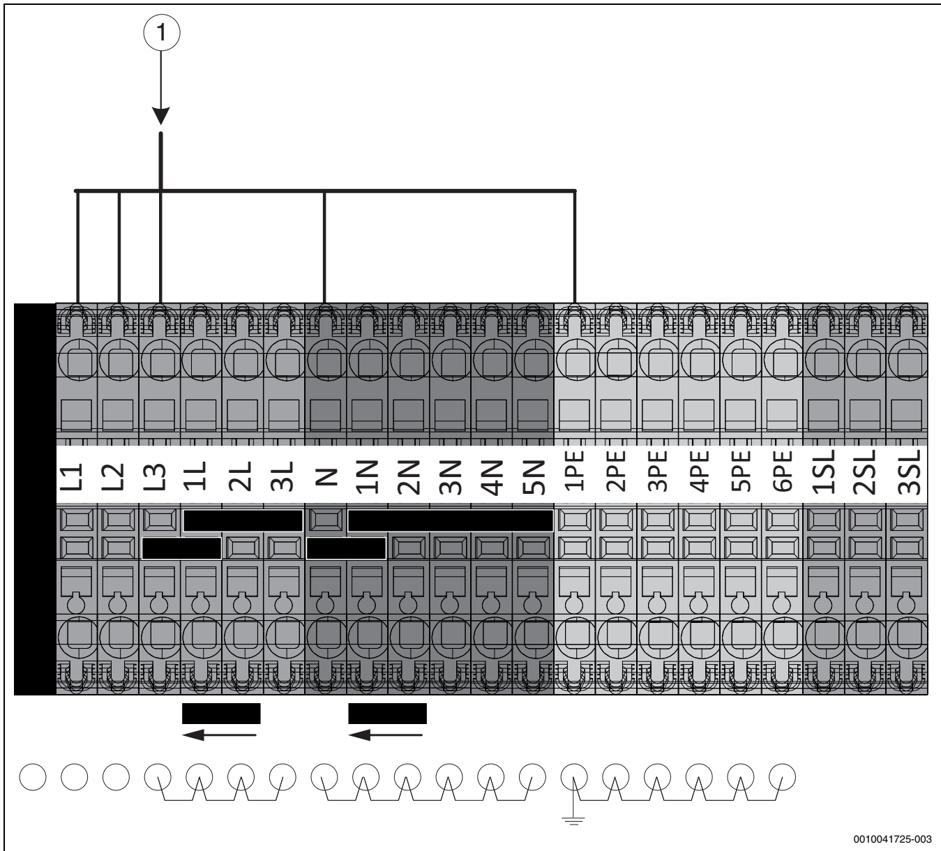
Bild 30 Elektrischer Anschluss
