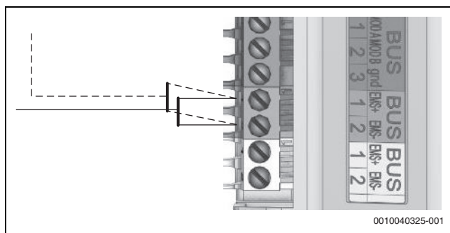
Bild 22 EMS-Anschluss
