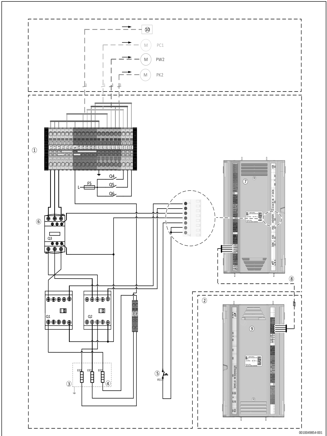
Bild 41 Spannungsversorgung Inneneinheit, Standard
