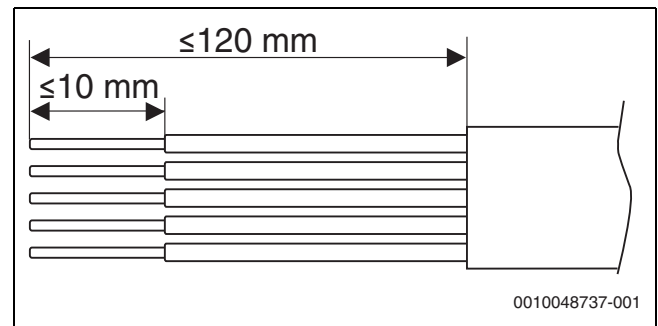
Bild 24 Abisolieren der Adern für den Netzanschluss
