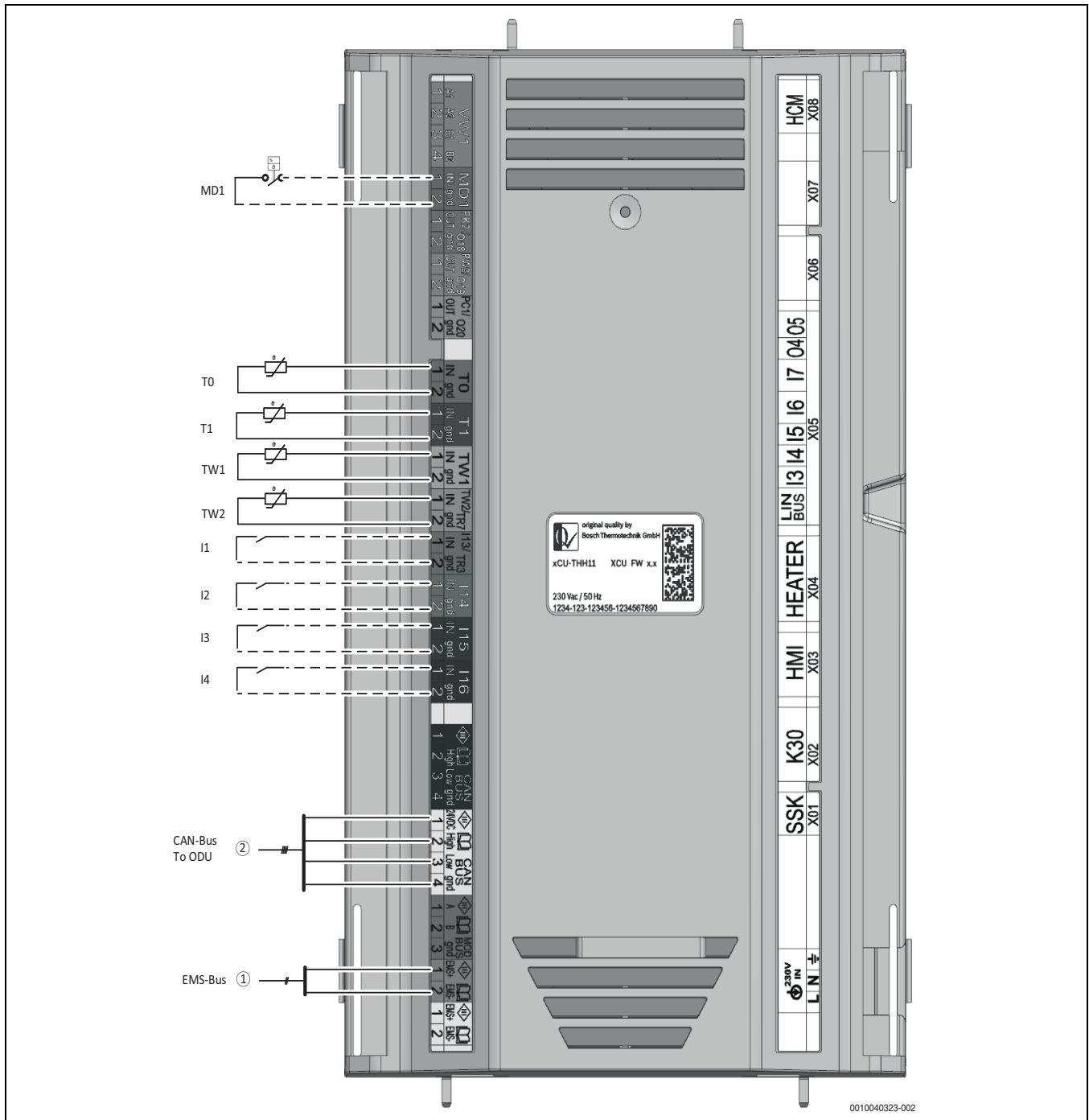
Bild 33 Anschlüsse
