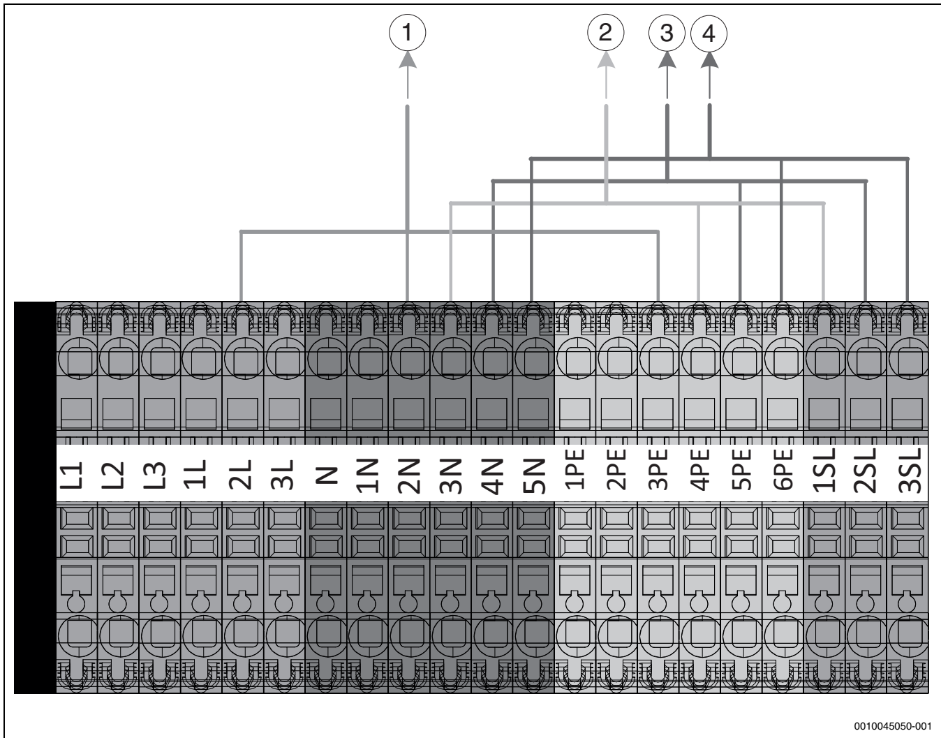
Bild 32 Elektrische Anschlüsse für Zubehör
