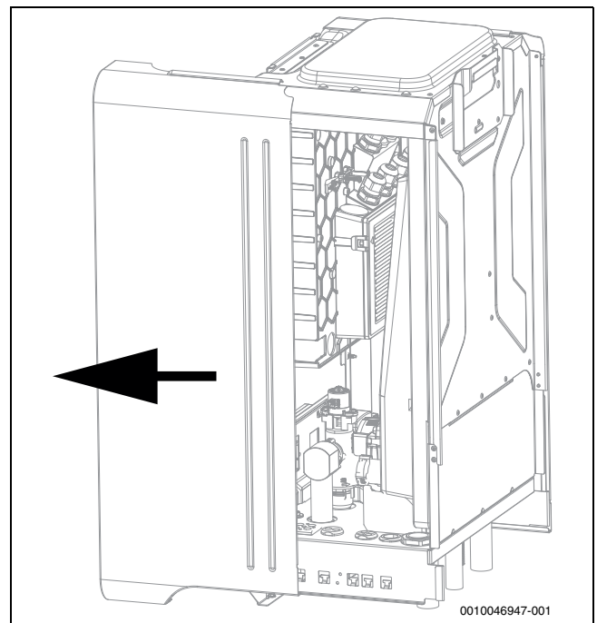
Bild 13 Seitenabdeckung abnehmen
