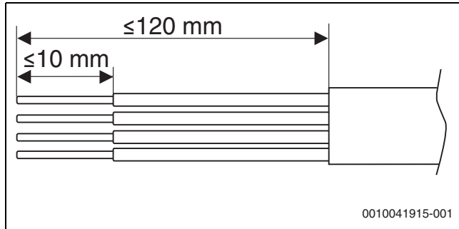
Bild 21 Abisolierung CAN-BUS
