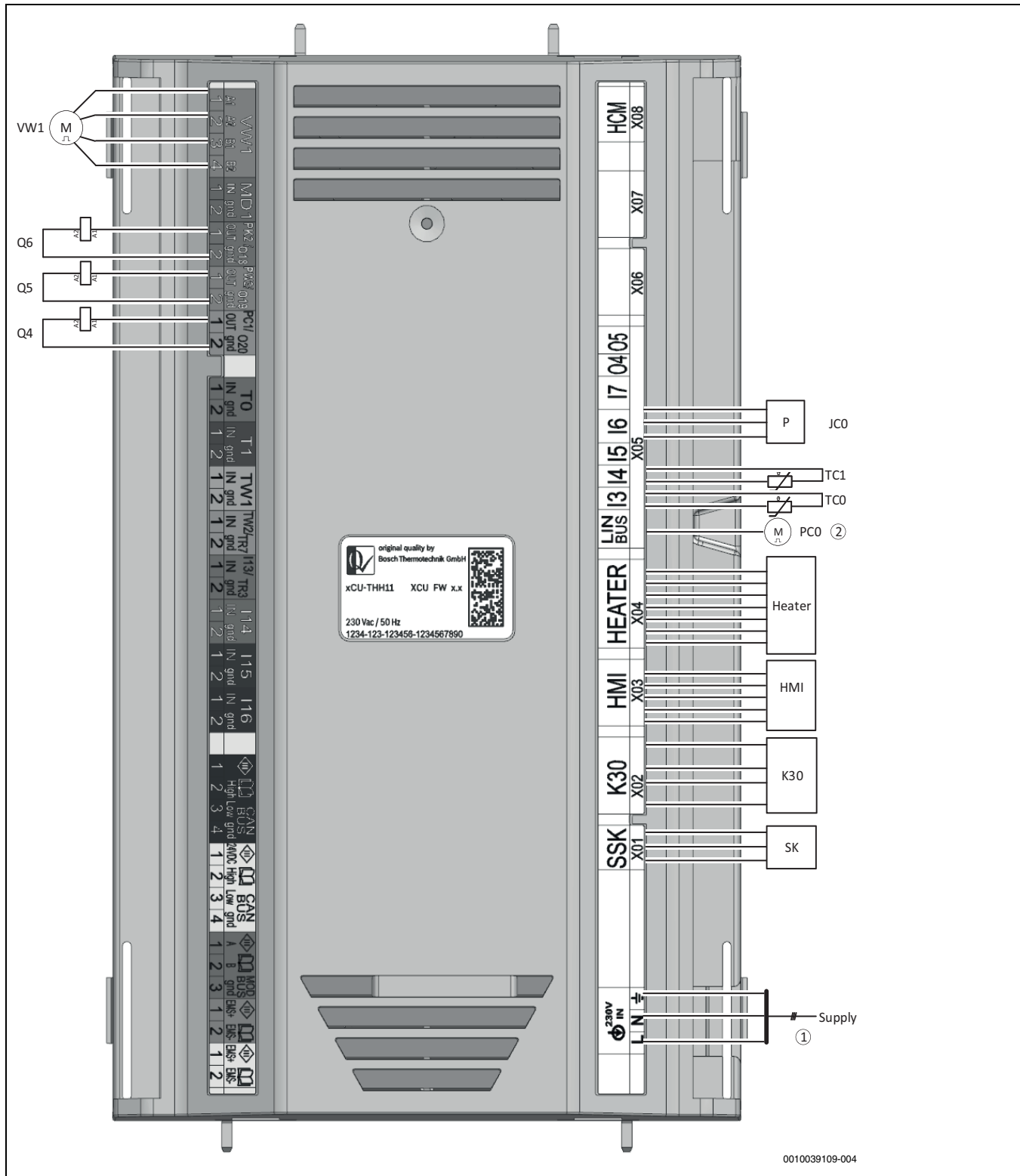
Bild 40 Schaltplan XCU-THH (XCU HY)
