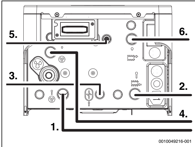
Bild 14 Rohranschlüsse
