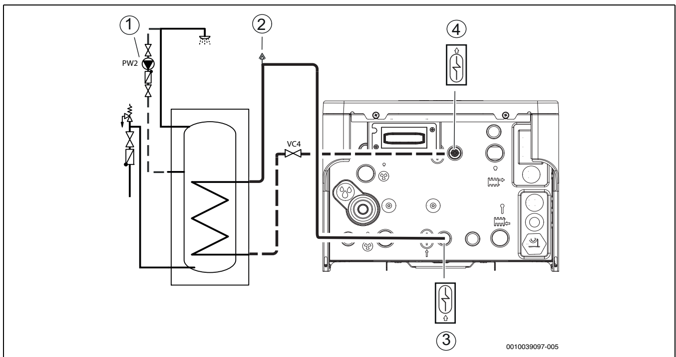
Bild 18 Trinkwasseranschlüsse Inneneinheit
