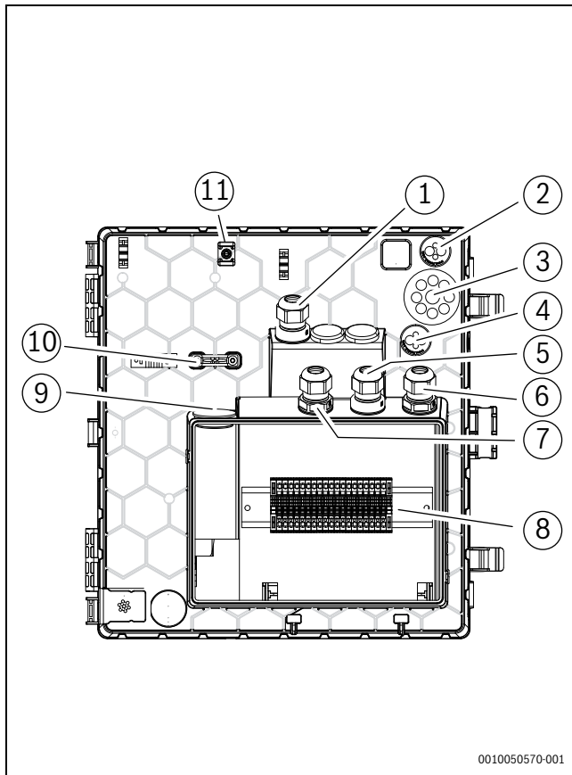
Bild 27 Kabeldurchführungen zum Klemmenkasten
