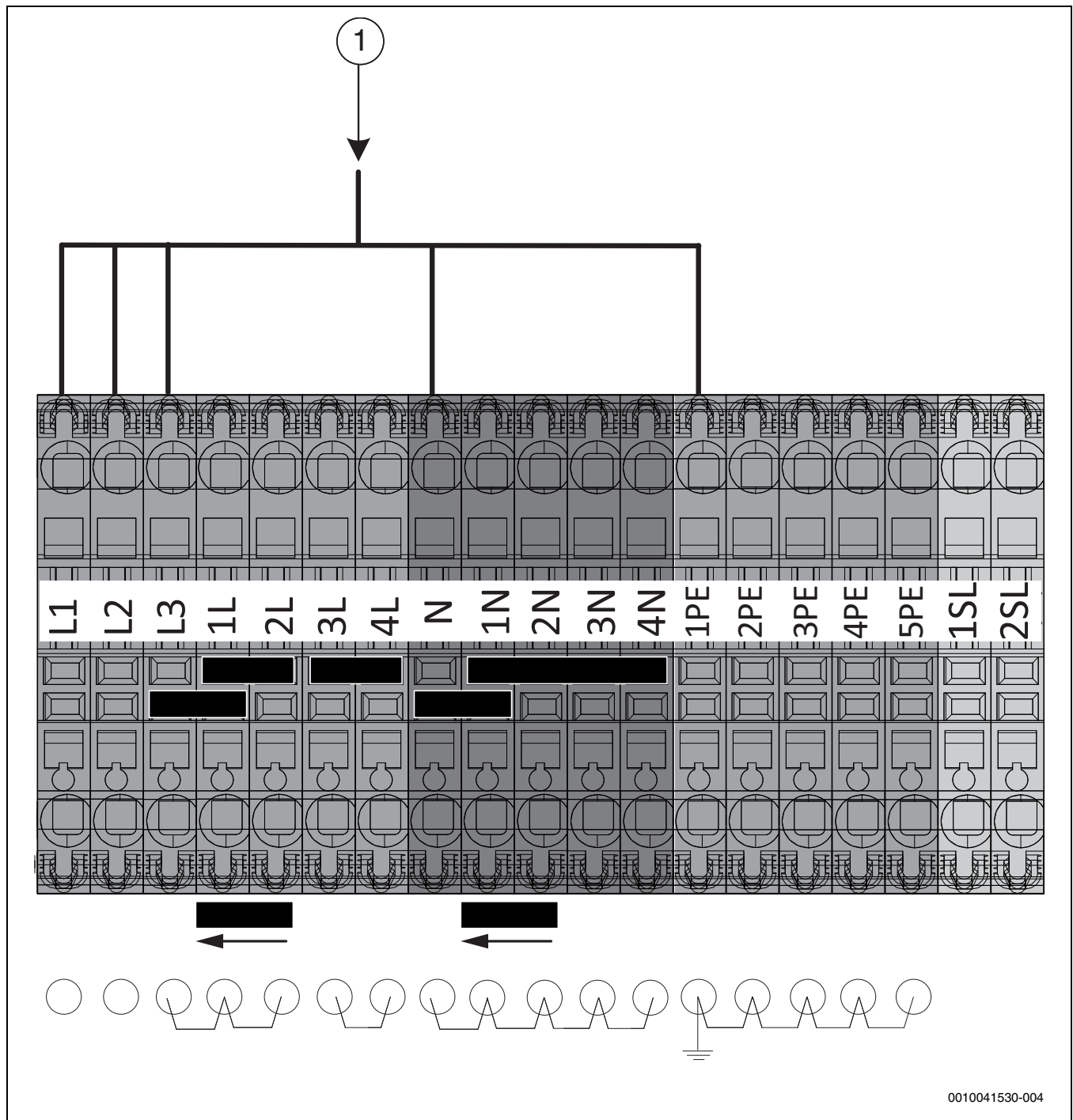
Bild 4 Elektrische Anschlüsse ohne EVU-Sperre
