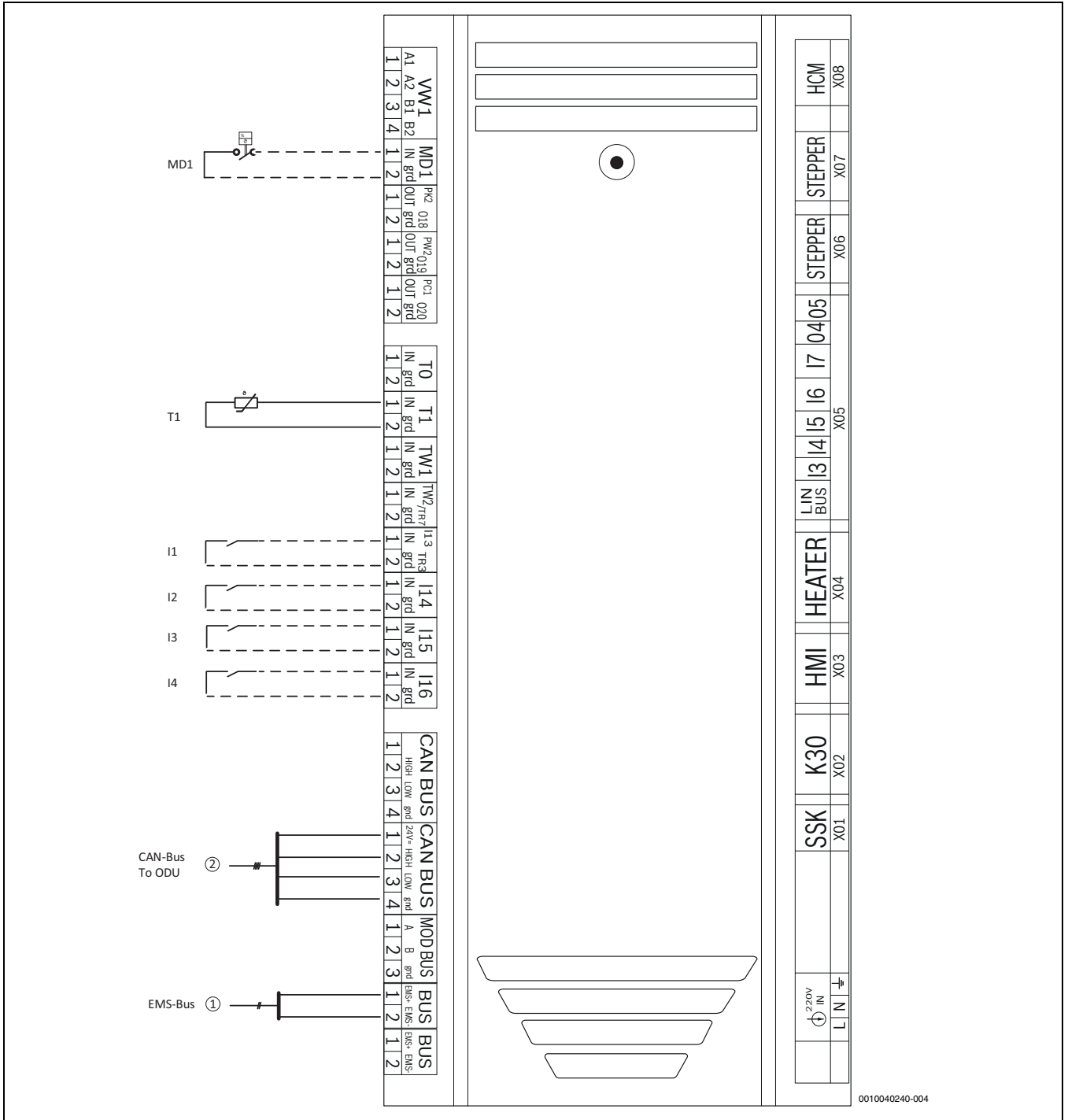
Bild 7 Anschlüsse XCU-THH (XCU HY)
