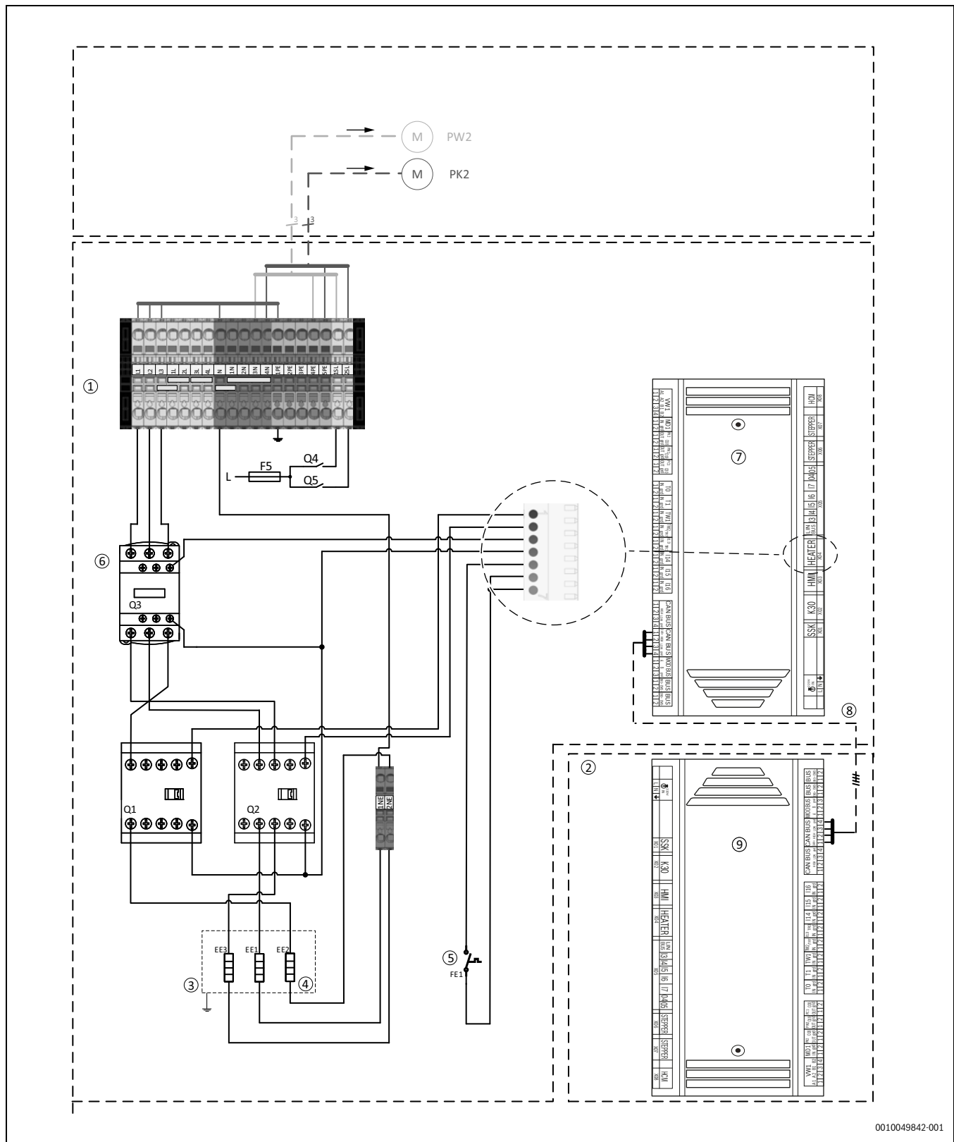
Bild 16 Spannungsversorgung Inneneinheit
