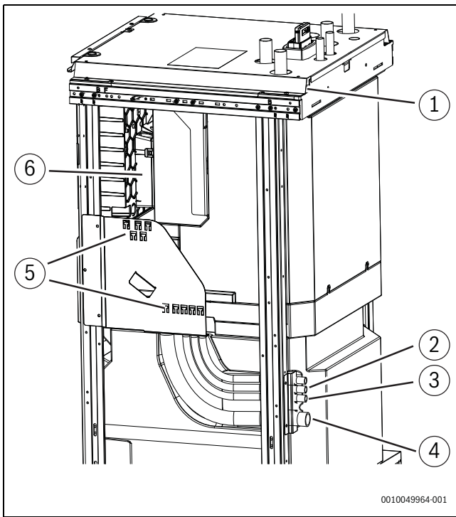
Bild 1 Kabelführungen der Inneneinheit
