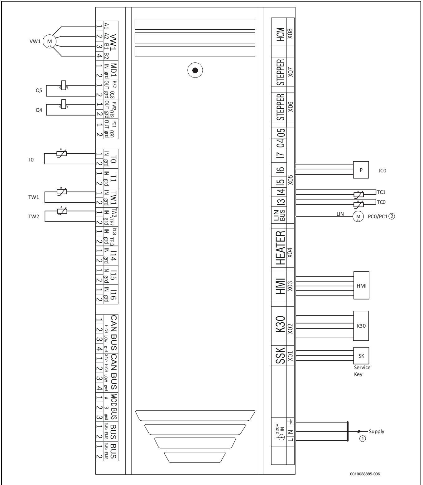
Bild 15 Schaltplan XCU-THH (XCU HY)-Modul
