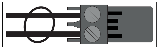
Bild 8 Kabelbinder am Steckverbinder
