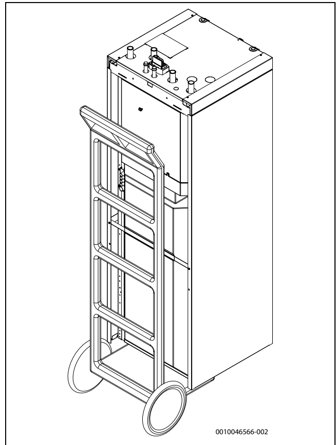
Bild 11 Transportwagen mit Gerät
