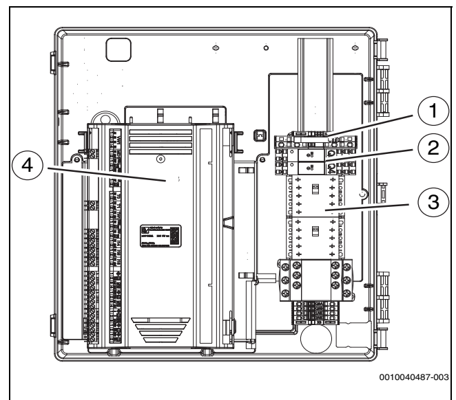
Bild 3 Anordnung der Komponenten im Klemmenkasten
