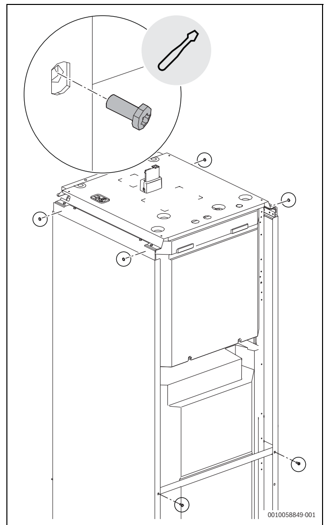
Bild 16 Schrauben für die Seitenwände
