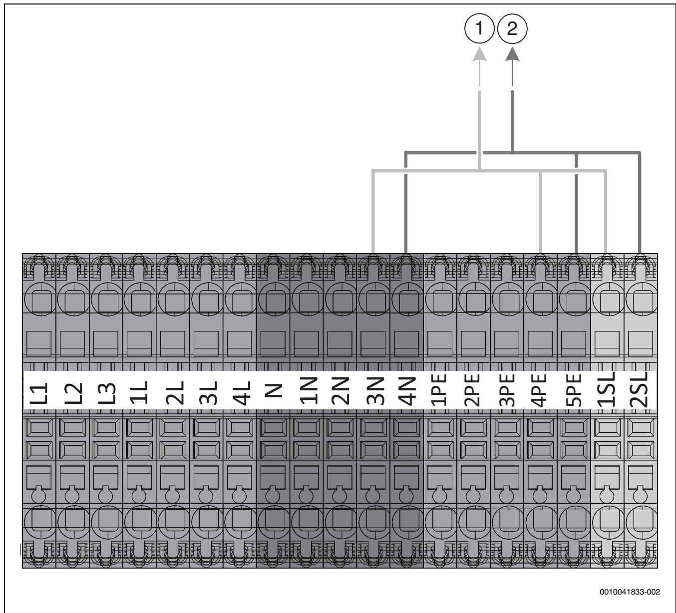
Bild 6 Elektrische Anschlüsse für Zubehör
