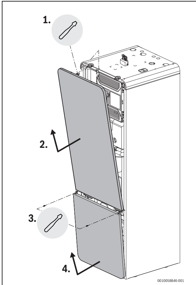
Bild 13 Vorderwand
