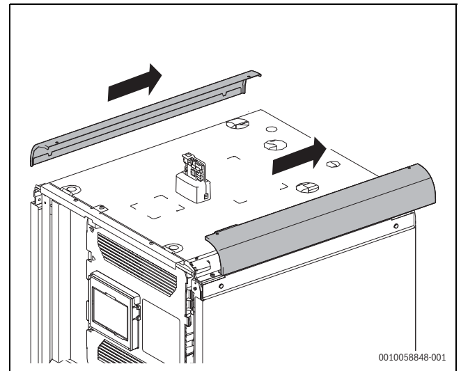
Bild 15 Abdeckleisten
