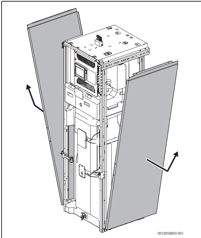
Bild 17 Seitenwand
