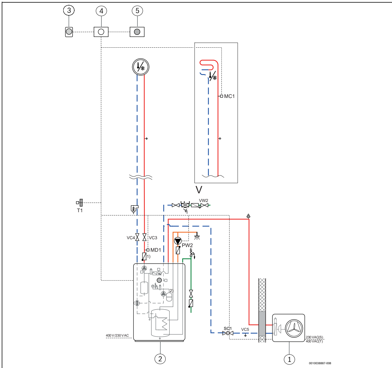
Bild 13 Tower Inneneinheit, Wärmepumpe (ODU), ein ungemischter Heizkreis
