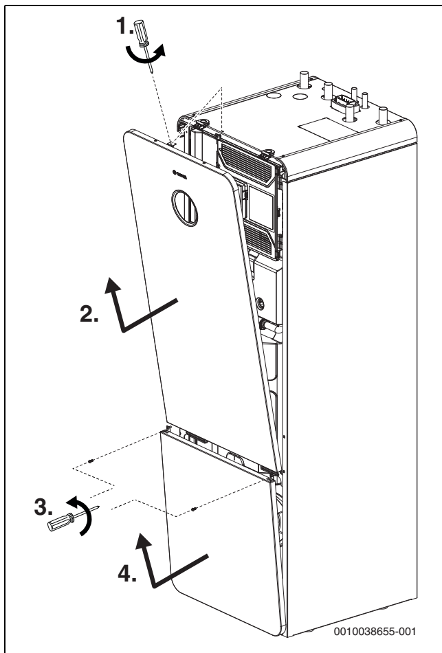
Bild 20 Front abnehmen
