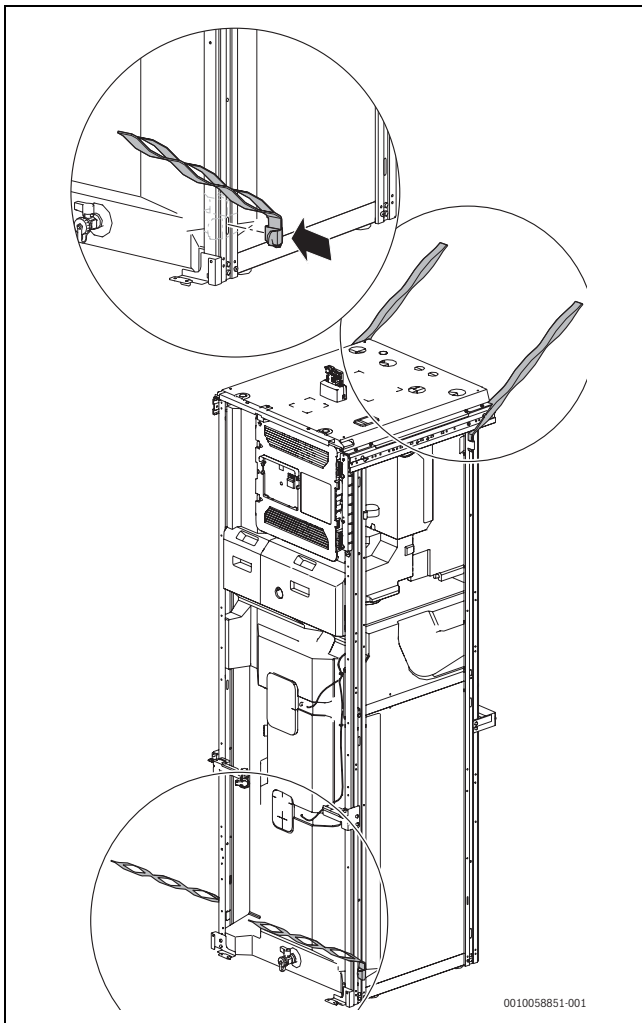
Bild 18 Transportgurte
