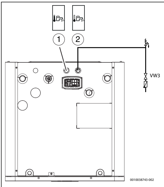
Bild 29 Wärmepumpenanschlüsse Trinkwasser
