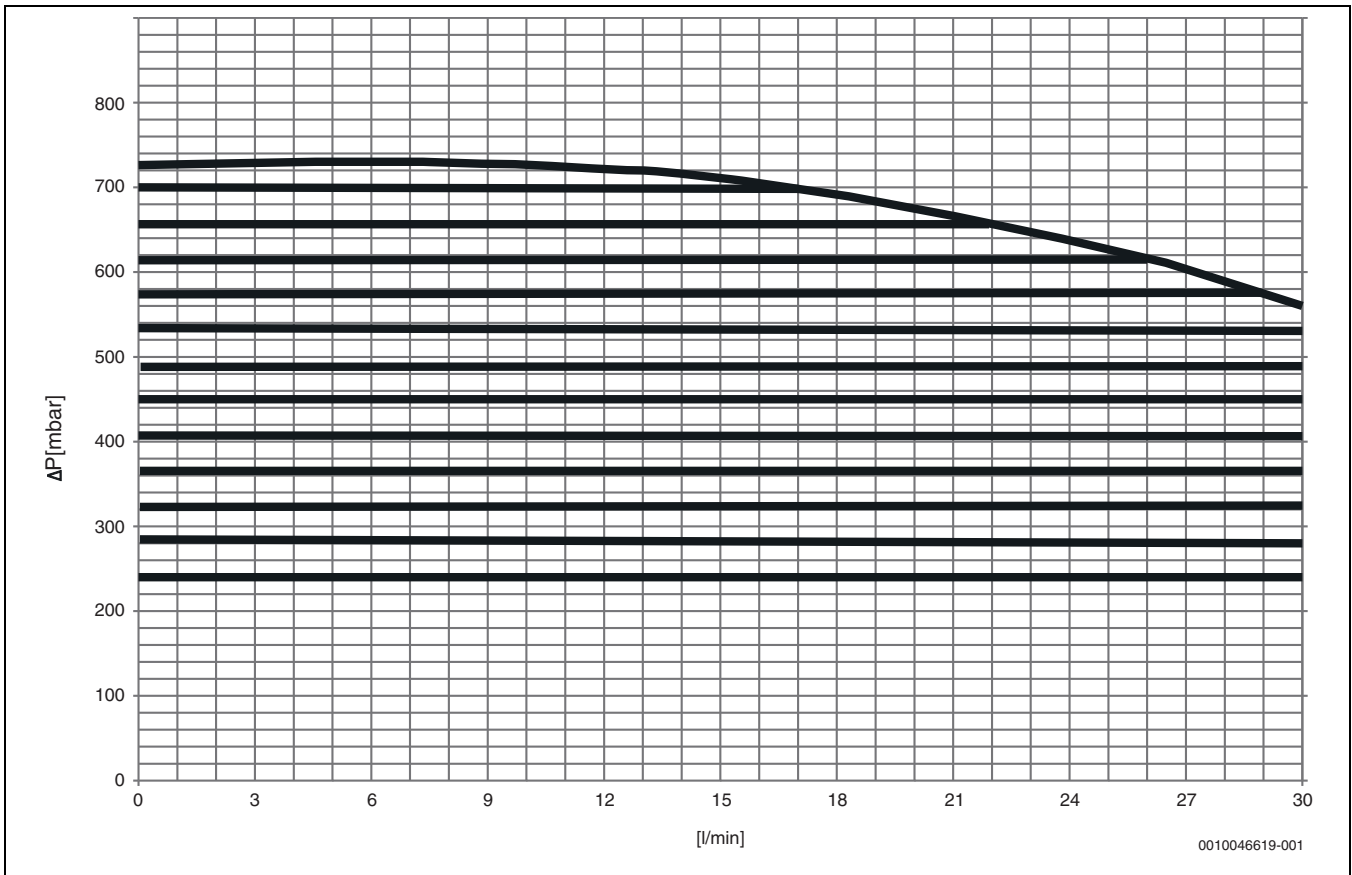
Bild 14 Pumpenkennzahlen für PC1
