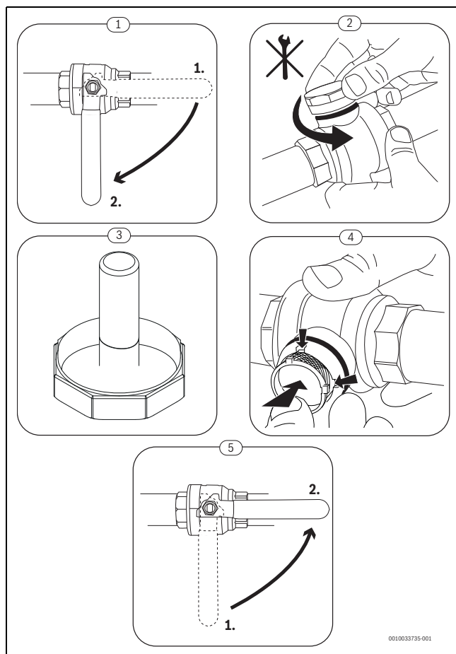
Bild 10 Reinigen des Partikelfilters
