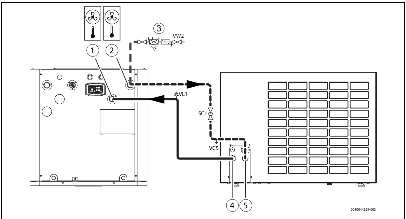
Bild 26 Inneneinheit an die Wärmepumpe anschließen
