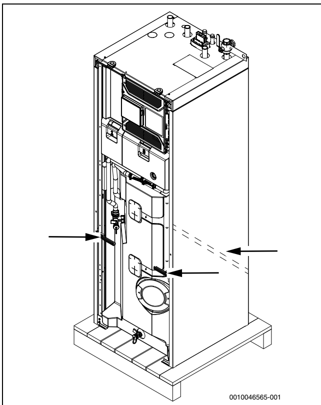
Bild 10 Transportbügel
