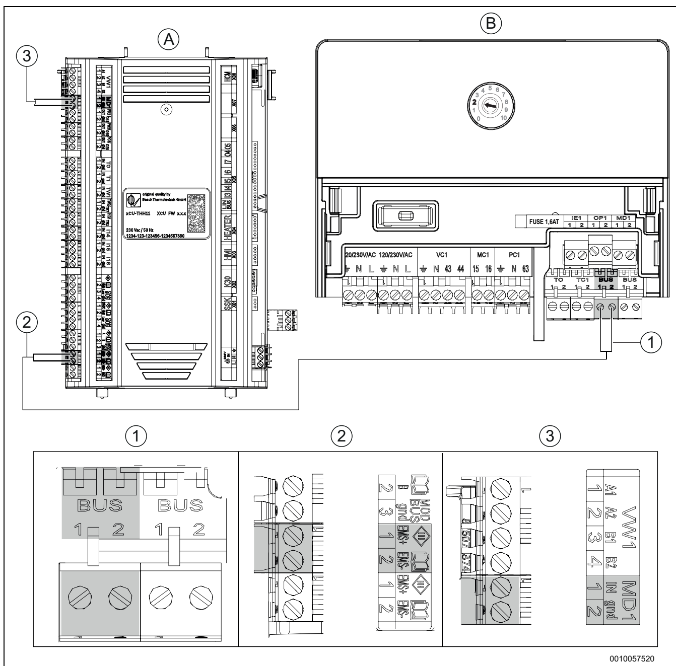
Afb. 10 Aansluiting van EMS-BUS aan dauwpuntsensor MD1, van passief koelstation naar warmtepomp
