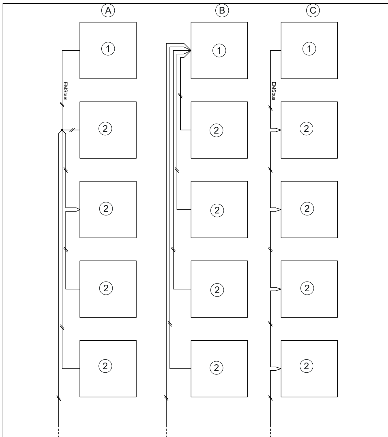
Fig. 45 Alternatives de raccordement pour bus EMS
