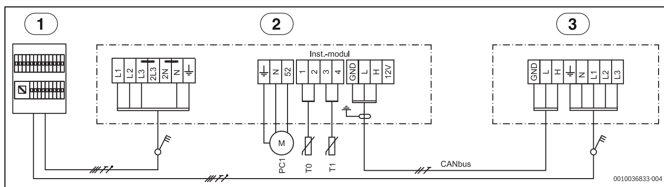
Fig. 42 Schéma de câblage 9 kW 400 V 3N ~
