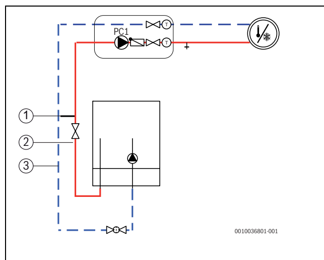
Fig. 31 Unité intérieure avec circuit de chauffage et by-pass
