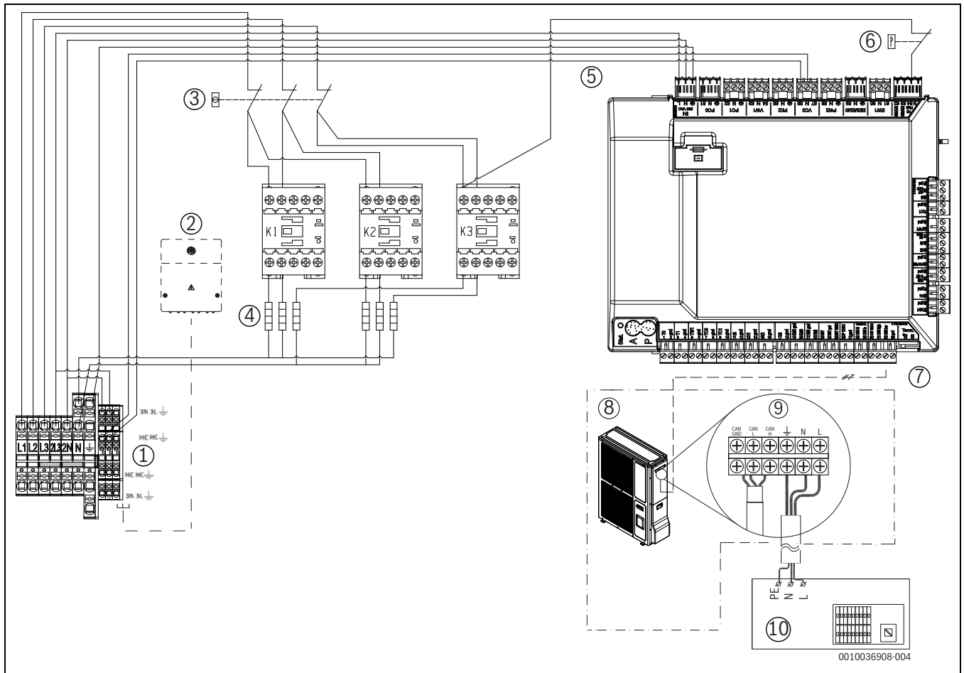
Fig. 43 Unité intérieure 400 V 3 N~ avec unité extérieure 230 V~
