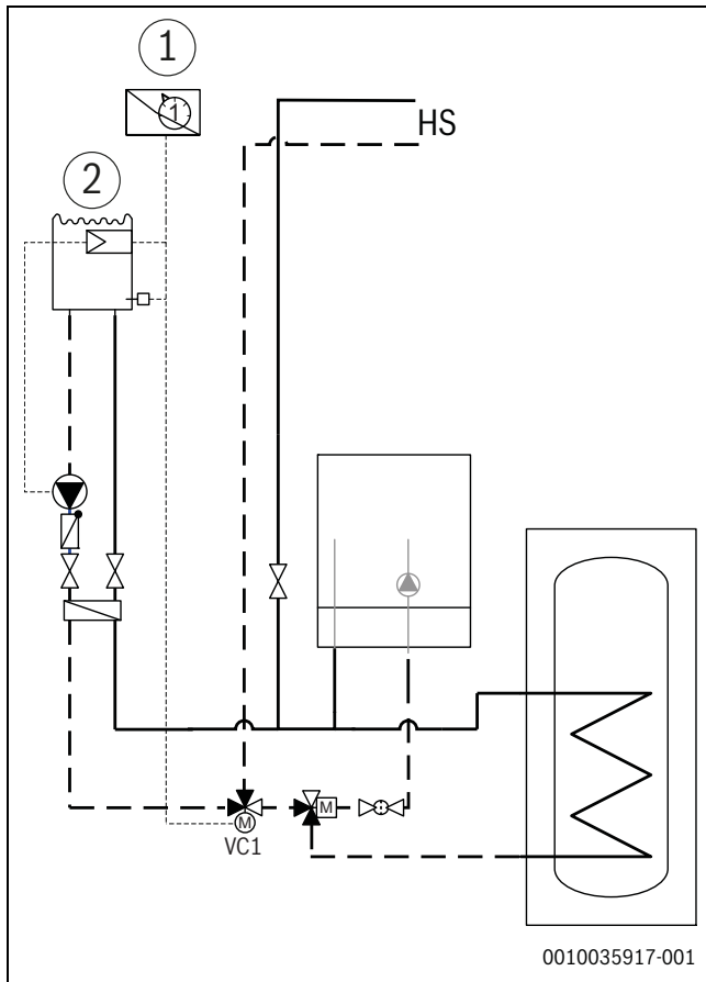
Fig. 25 Exemple d'installation d'une piscine
