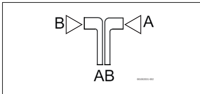
Fig. 22 Hydraulique pour vanne d'inversion TW1
