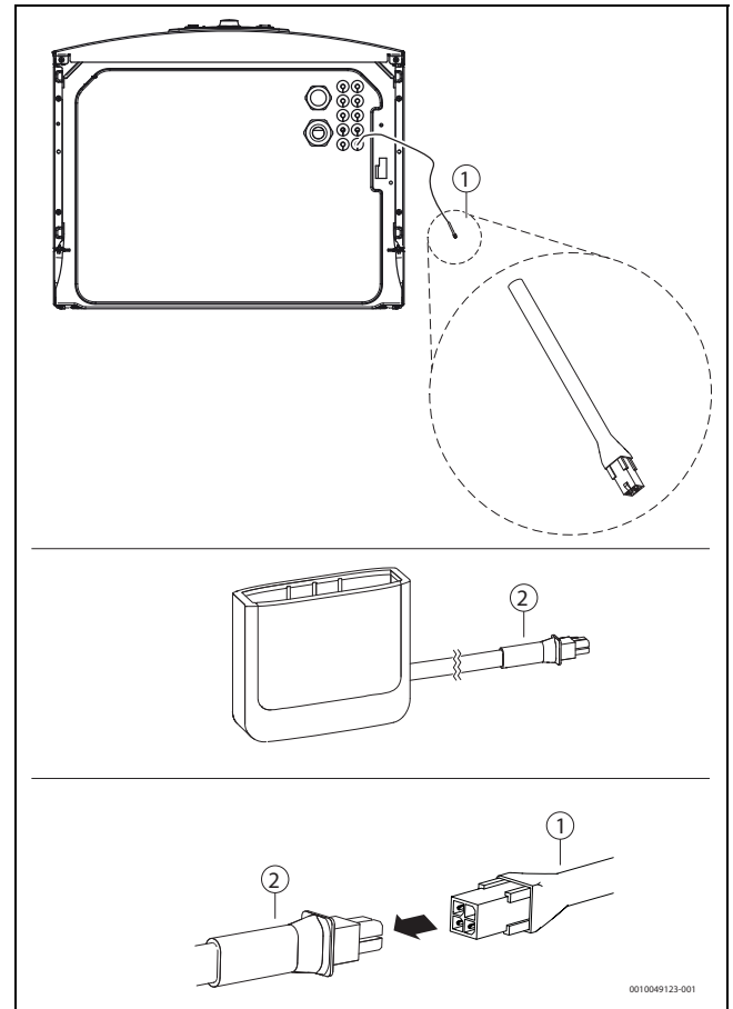
Fig. 26 Raccordement de Module radio.
