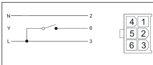
Fig. 21 Connecteur Molex
