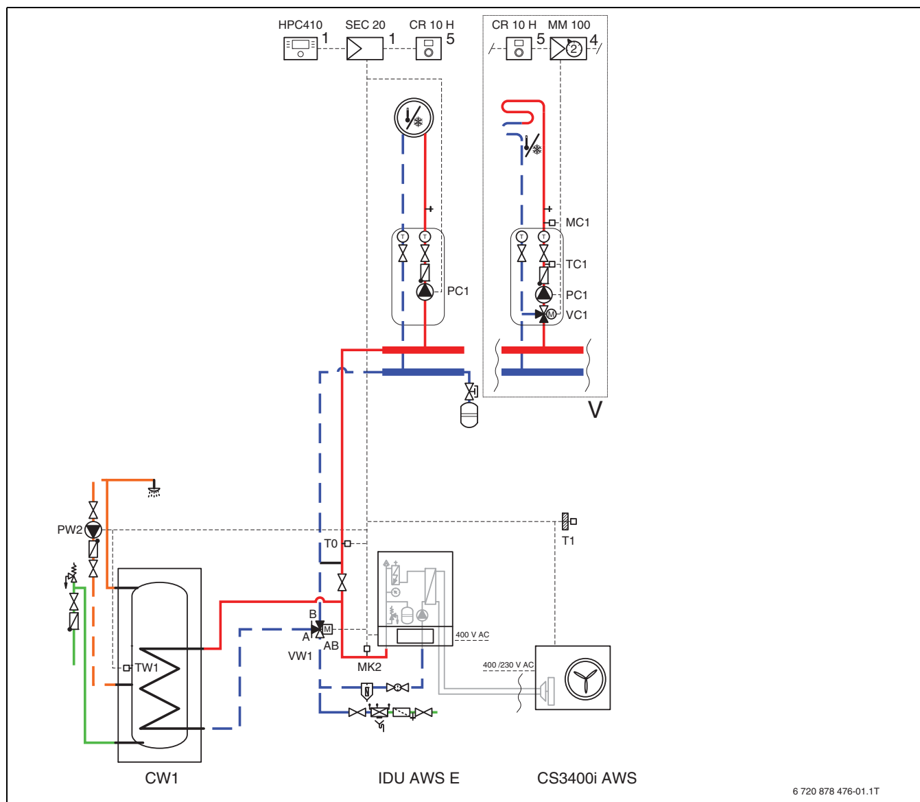
Fig. 36 Unité extérieure avec unité intérieure, ECS et un ou plusieurs circuits de chauffage
