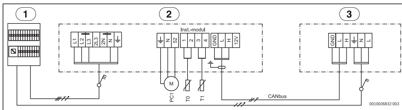
Fig. 41 Schéma de câblage 9 kW 400 V 3 N~
