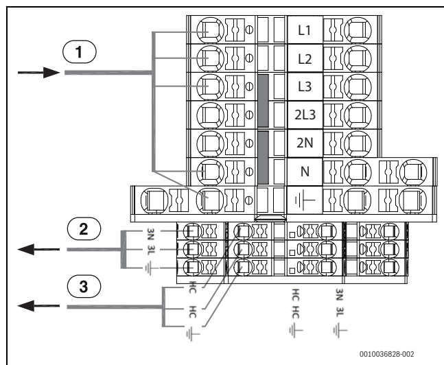
Fig. 14 Bornes de raccordement pour le raccordement électrique, 9 kW 400 V 3 N~
