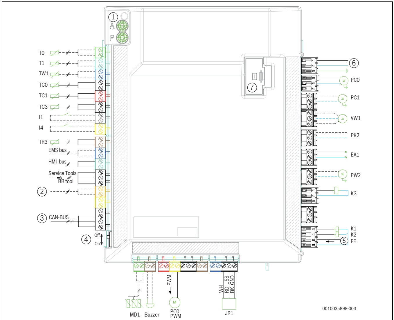
Fig. 38 Carte de circuit imprimé d'installation de l'unité intérieure
