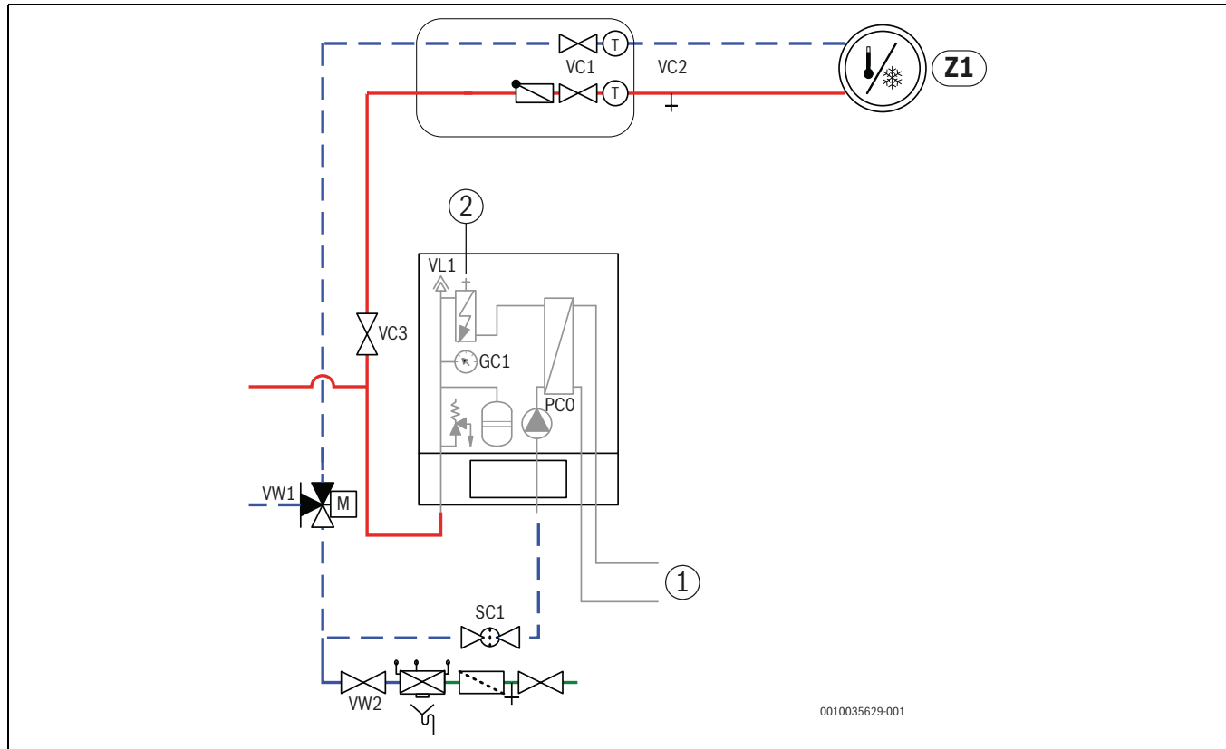
Fig. 9 Unité intérieure avec chauffage d'appoint électrique intégré et système de chauffage
