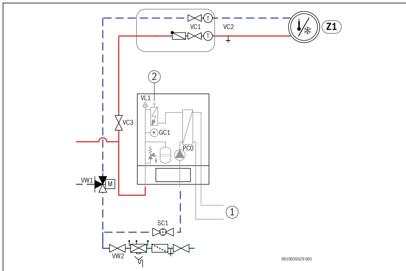
Fig. 16 Unité intérieure avec chauffage d'appoint électrique intégré et système de chauffage
