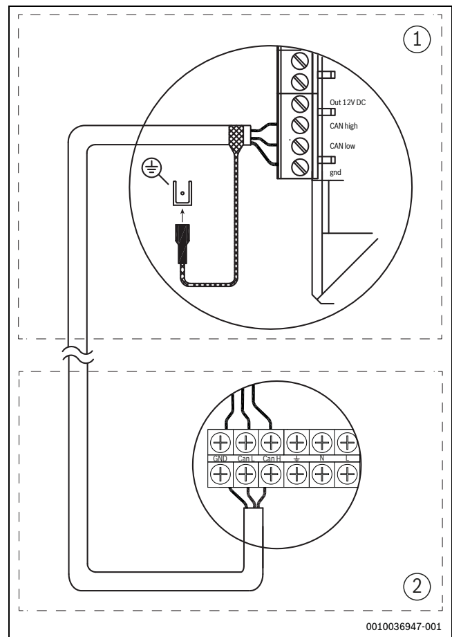
Fig. 12 Connexion CAN-BUS
