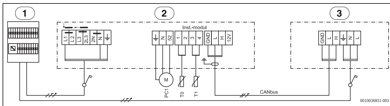
Fig. 40 Schéma de câblage
