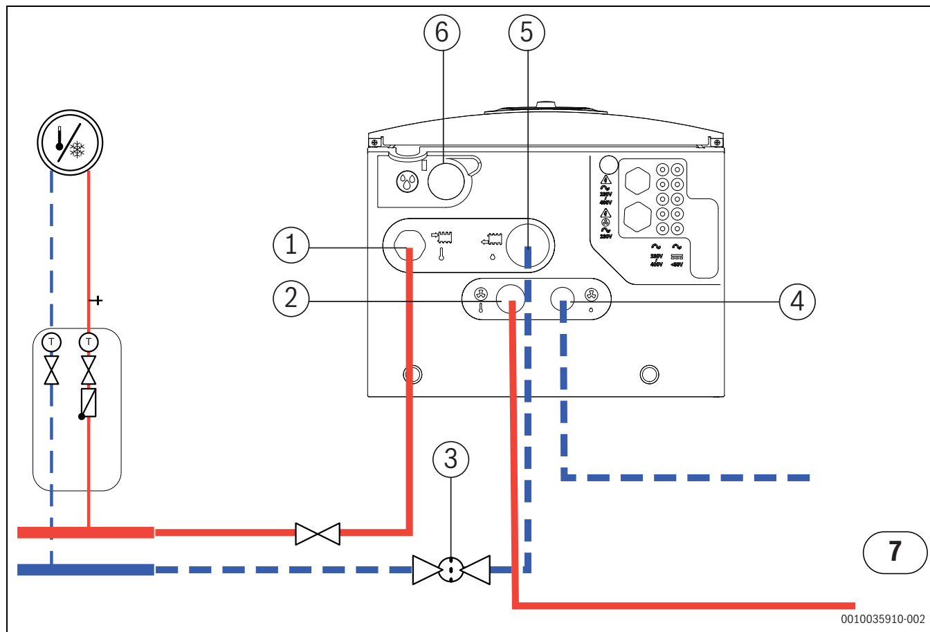
Fig. 8 Raccordement d'une unité intérieure avec chauffage d'appoint électrique intégré à une unité extérieure et un système de chauffage
