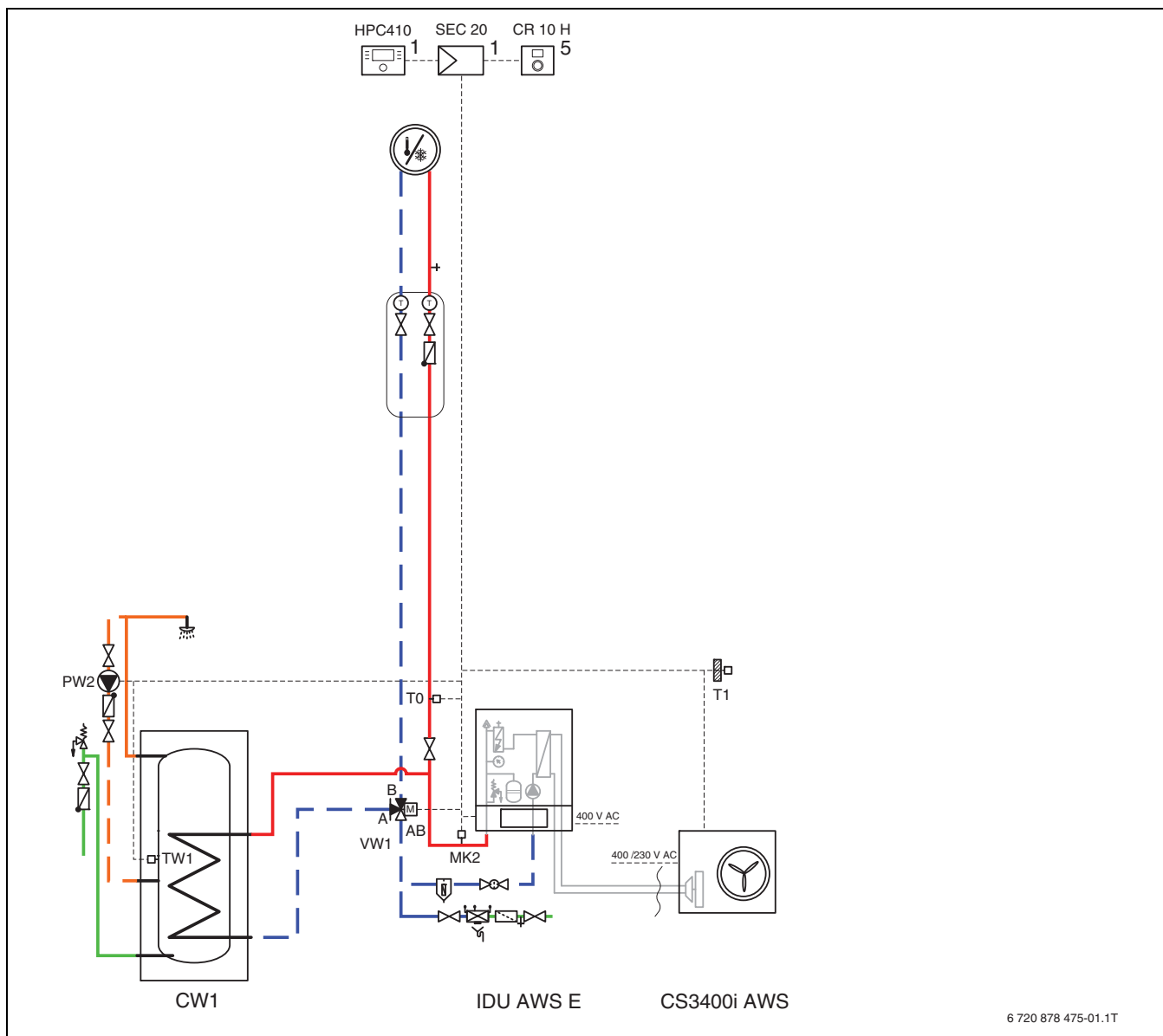
Fig. 35 Unité extérieure avec unité intérieure et un circuit de chauffage
