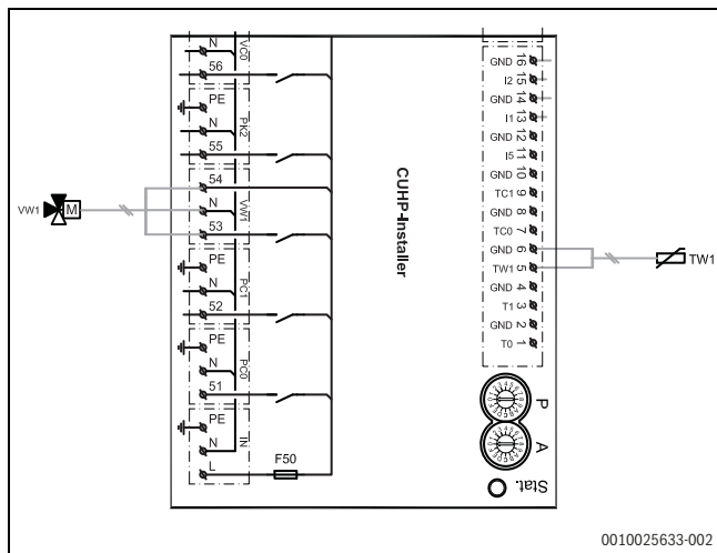
Fig. 20 Raccordement de la vanne d'inversion VW1 sur la carte de circuit imprimé d'installation
