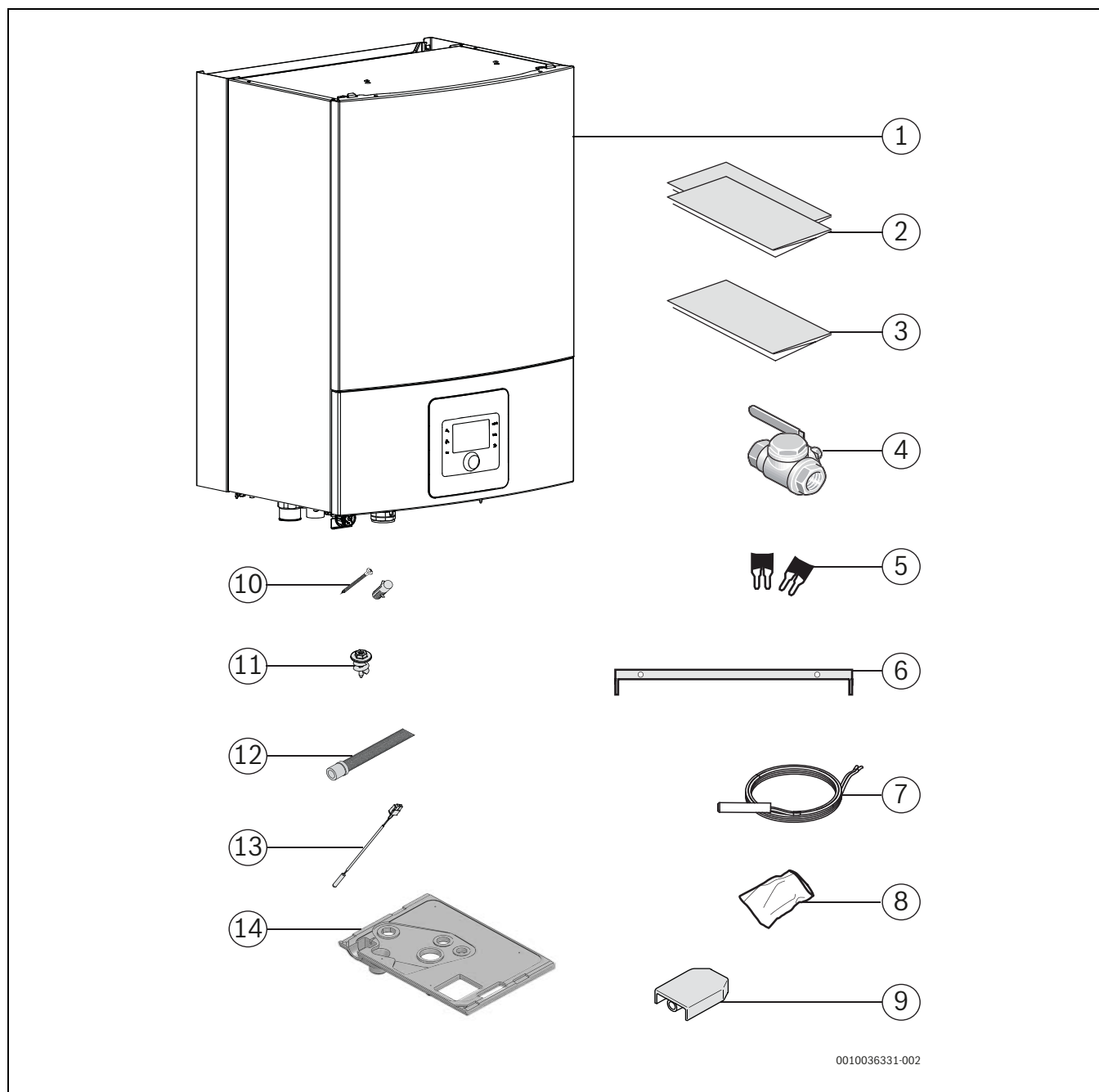
Fig. 2 Pièces fournies
