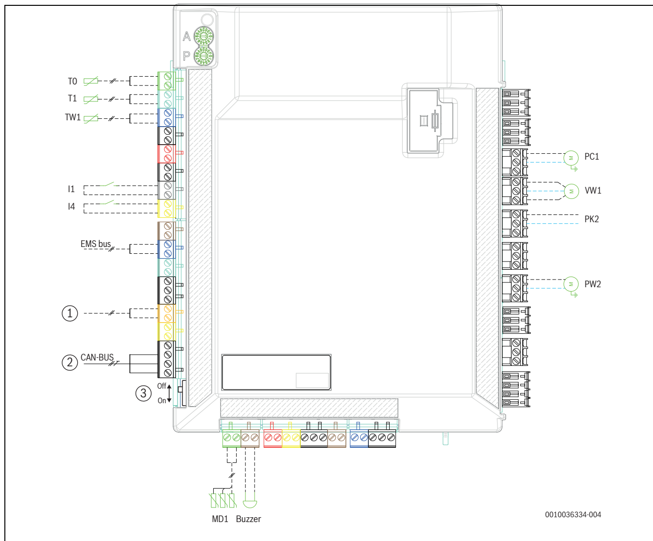
Fig. 11 Carte de circuit imprimé d'installation de l'unité intérieure
