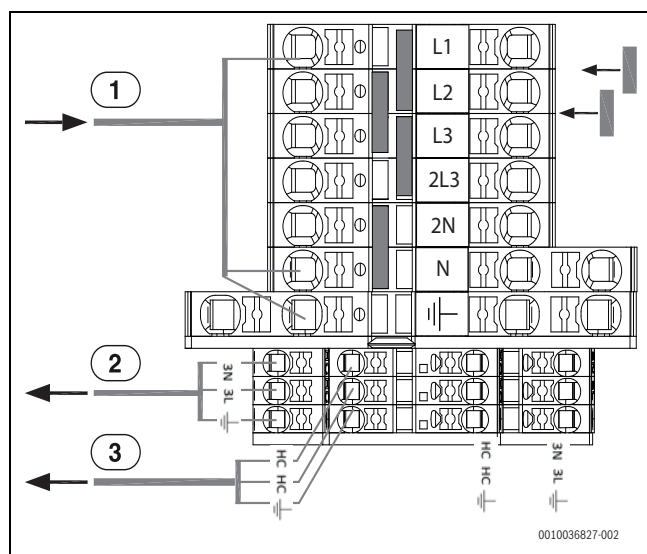
Fig. 15 Bornes de raccordement pour le raccordement électrique, 9 kW 230 V~
