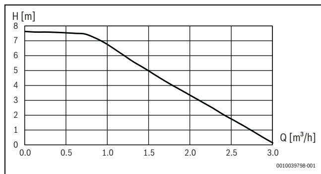
Fig. 30 Courbe caractéristique de capacité pour la pompe de circulation primaire (PC0)
