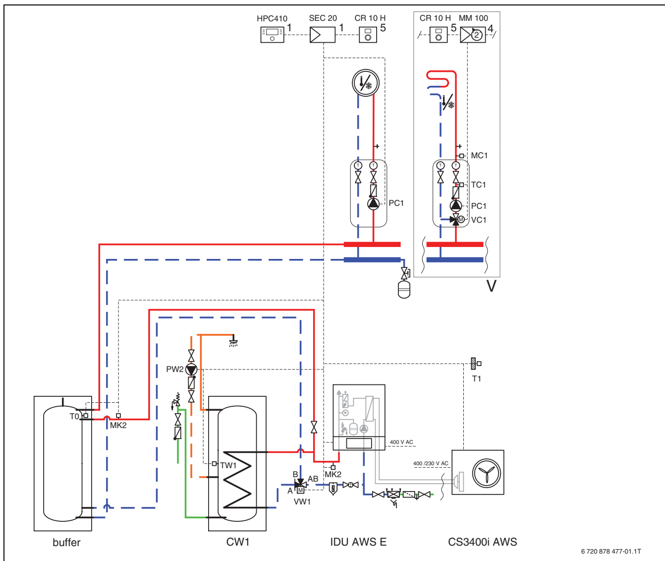
Fig. 37 Unité extérieure avec unité intérieure, tampon et un ou plusieurs circuits de chauffage
