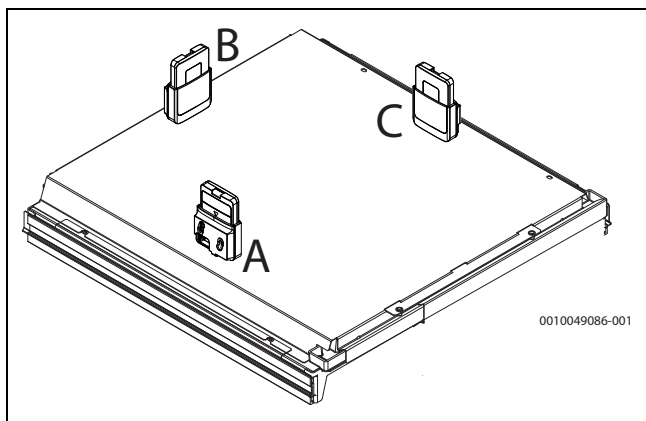
Fig. 27 Fixer le support sur la partie supérieure de l'appareil sur pieds. En plus du support, la figure indique également Module radio qui se trouve à l'intérieur du support
