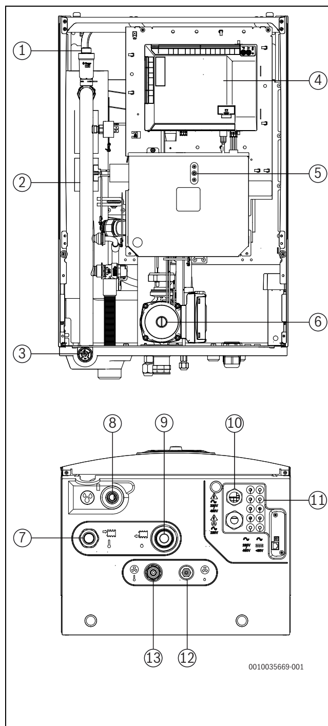
Fig. 3 Composants et raccords de conduites de l'unité intérieure avec chauffage d'appoint électrique (vues avec bac de récupération)
