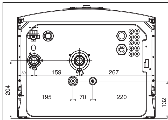
Fig. 5 Dimensions et raccordements (vue sans bac de récupération)
