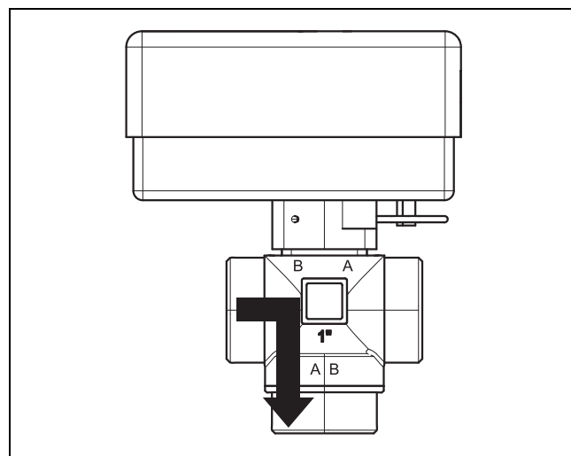
Fig. 24 Contact ouvert, raccordement B ouvert
