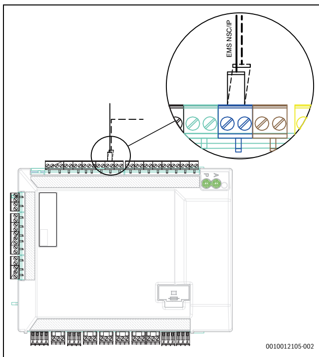
Fig. 18 Raccordement EMS sur le module d'installation
