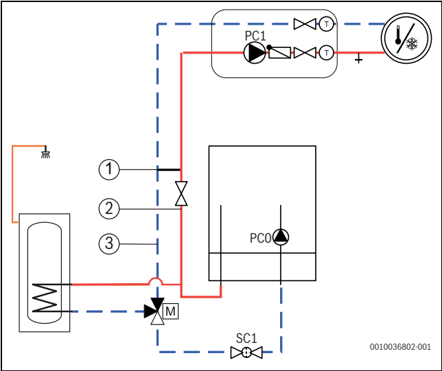
Fig. 32 Unité intérieure avec circuit de chauffage et production d'eau chaude sanitaire
