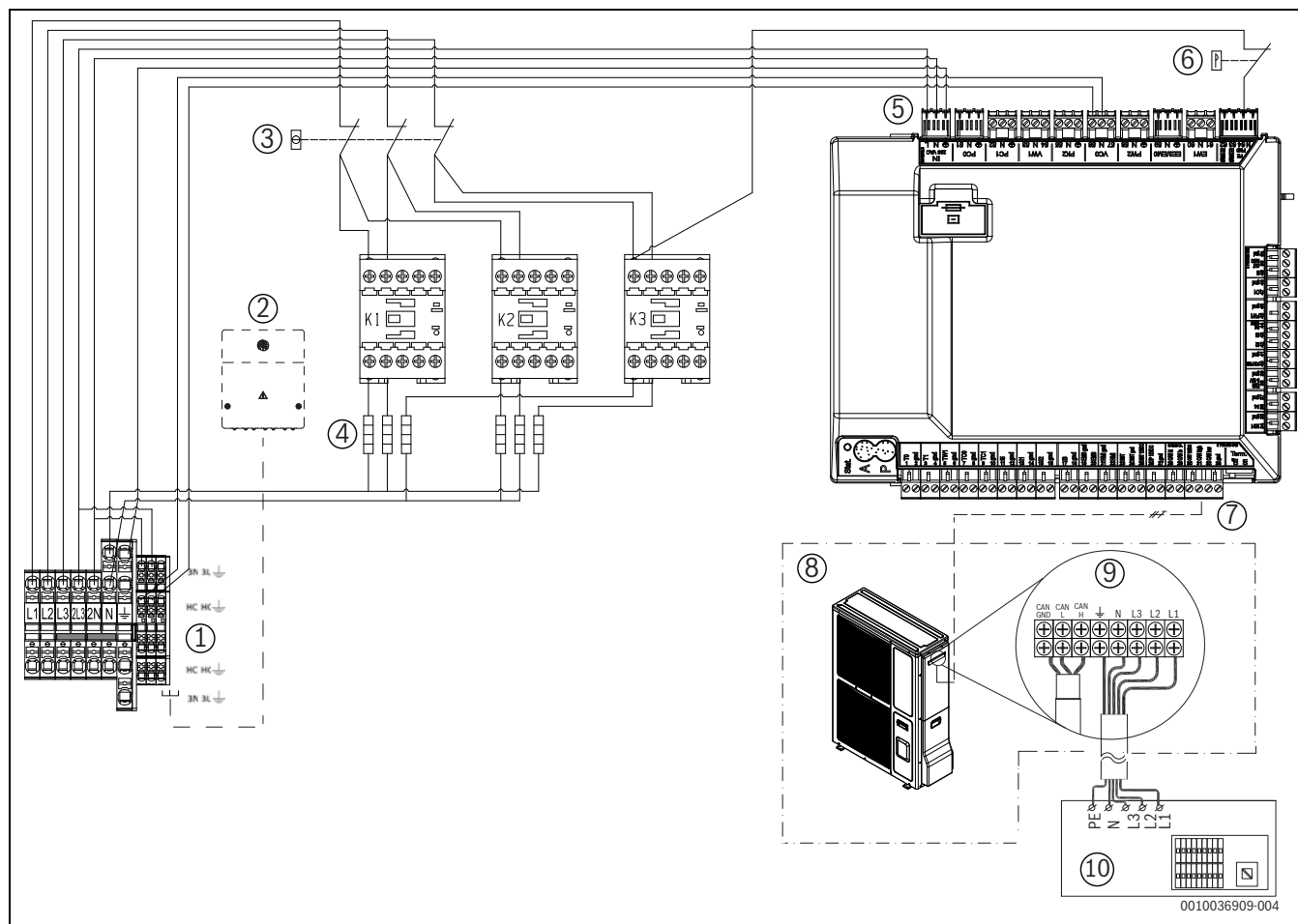
Fig. 44 Unité intérieure 400 V 3 N~ avec unité extérieure 400 V 3 N~
